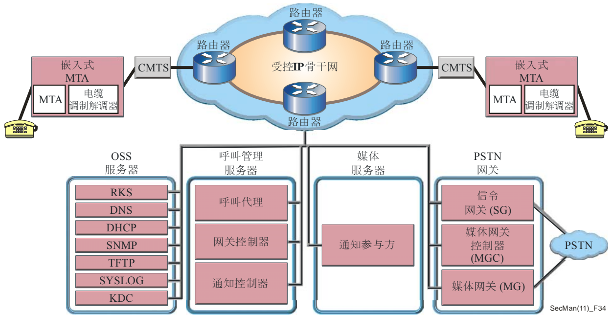
图34 – IP-Cablecom构成参考模型
