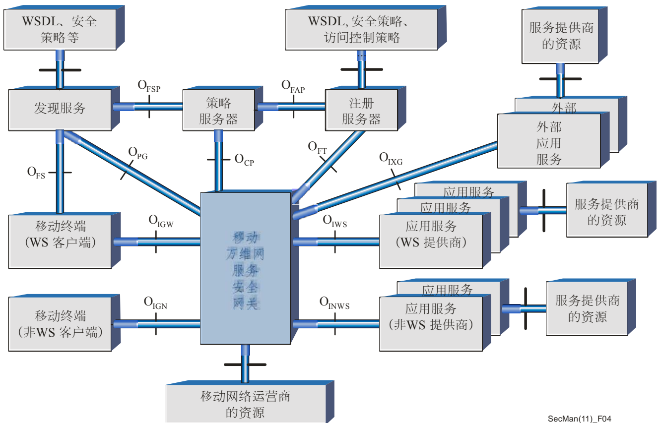
图 4 – 用于移动万维网服务的安全体系结构
