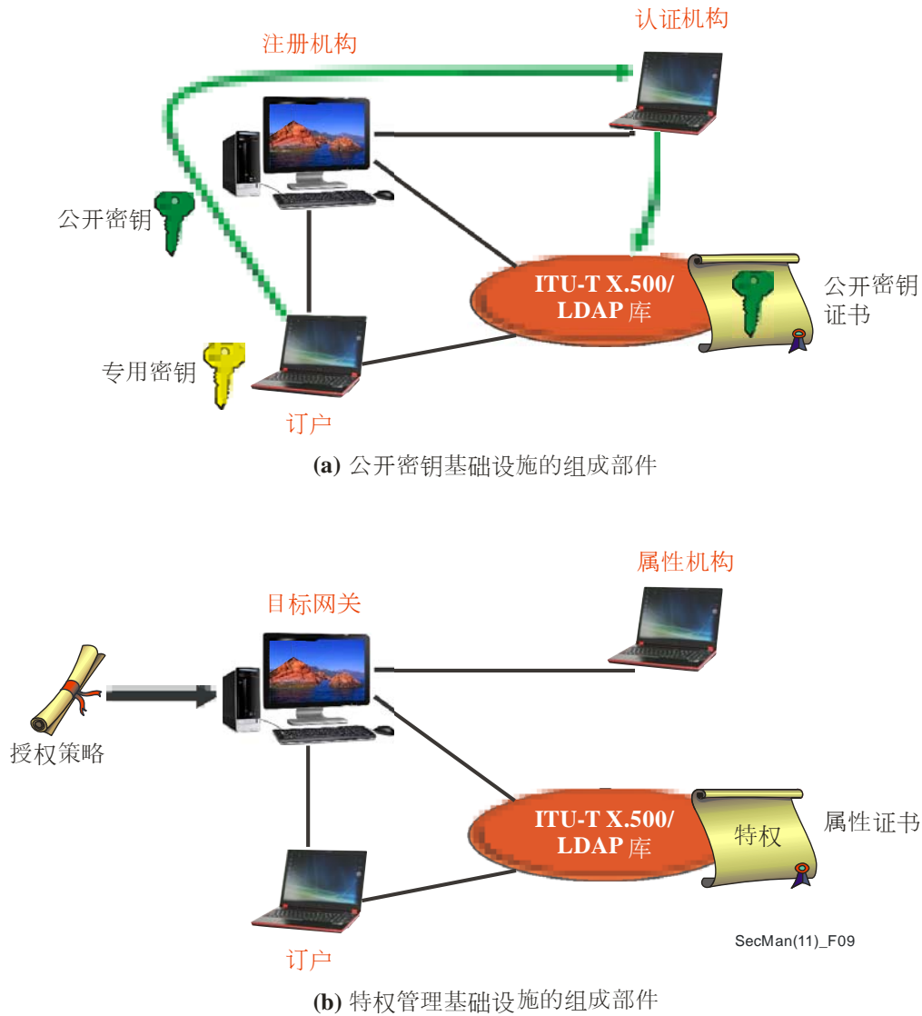
图9 – PKI和PMI的构成
