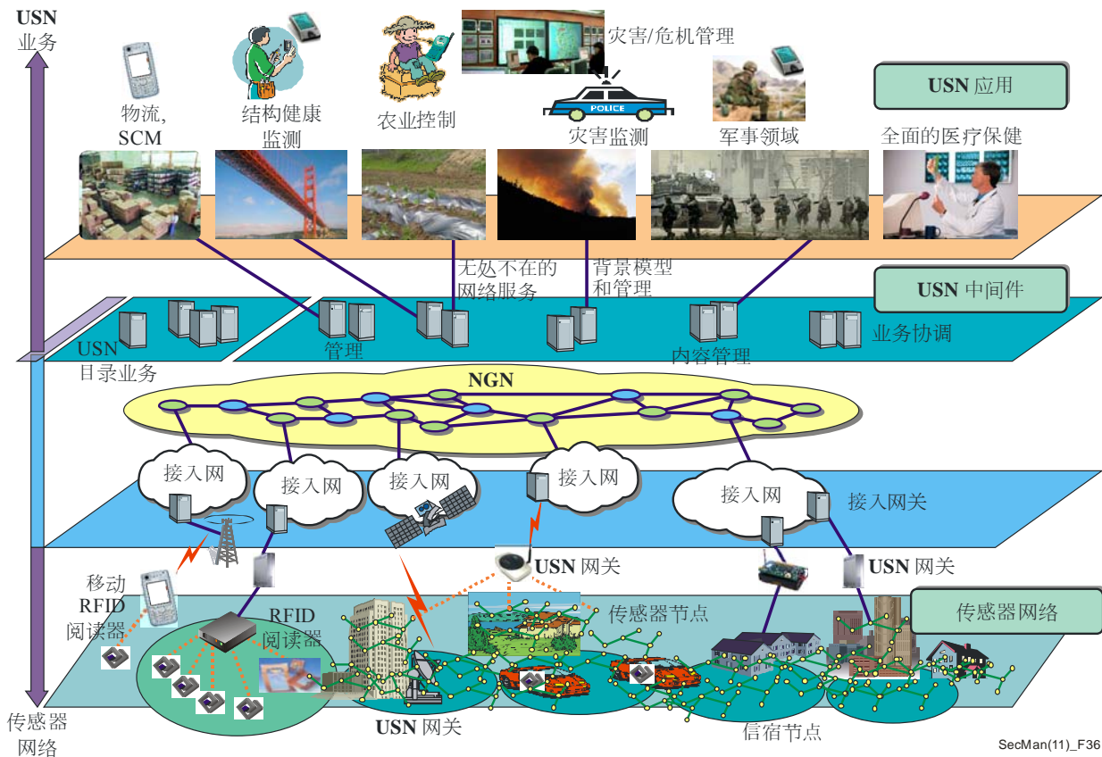
图36 – USN的总体结构
