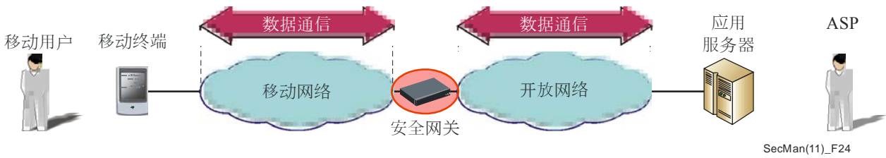
图24 - 移动用户与ASP之间移动端对端数据通信的网关模型
