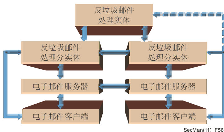
图56 – 反垃圾电子邮件处理域的通用结构
