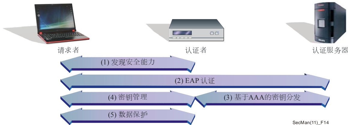
图14 – 低层认证和密钥管理的四个工作阶段
