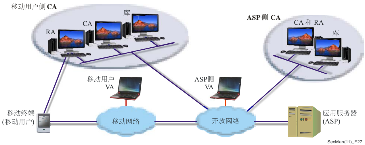
图27 – 移动端对端数据通信的通用PKI模型
