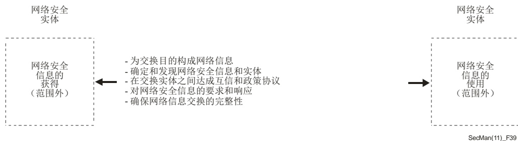
图39 – CYBEX模型
