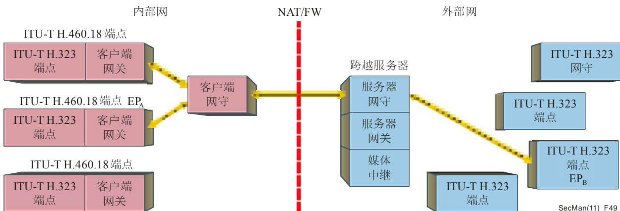
图49 – 网守通信体系结构
