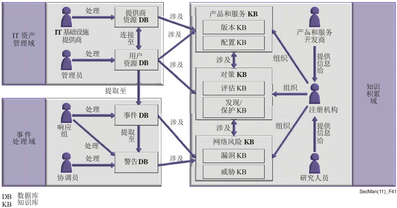
图41 – 网络安全运行信息本体论
