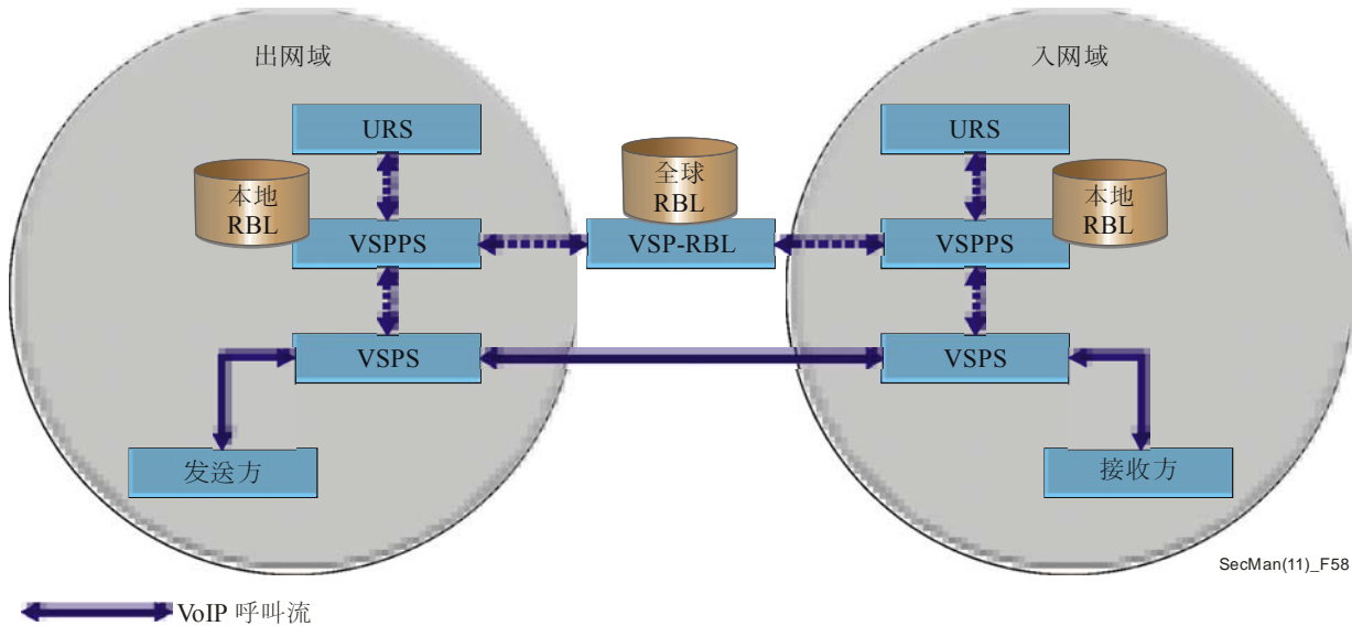
图58 – 打击VoIP垃圾信息的功能架构
