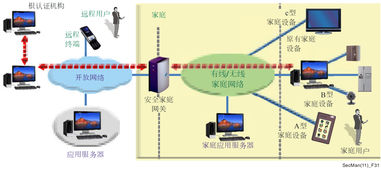
图31 – 安全家庭网络的设备认证模型
