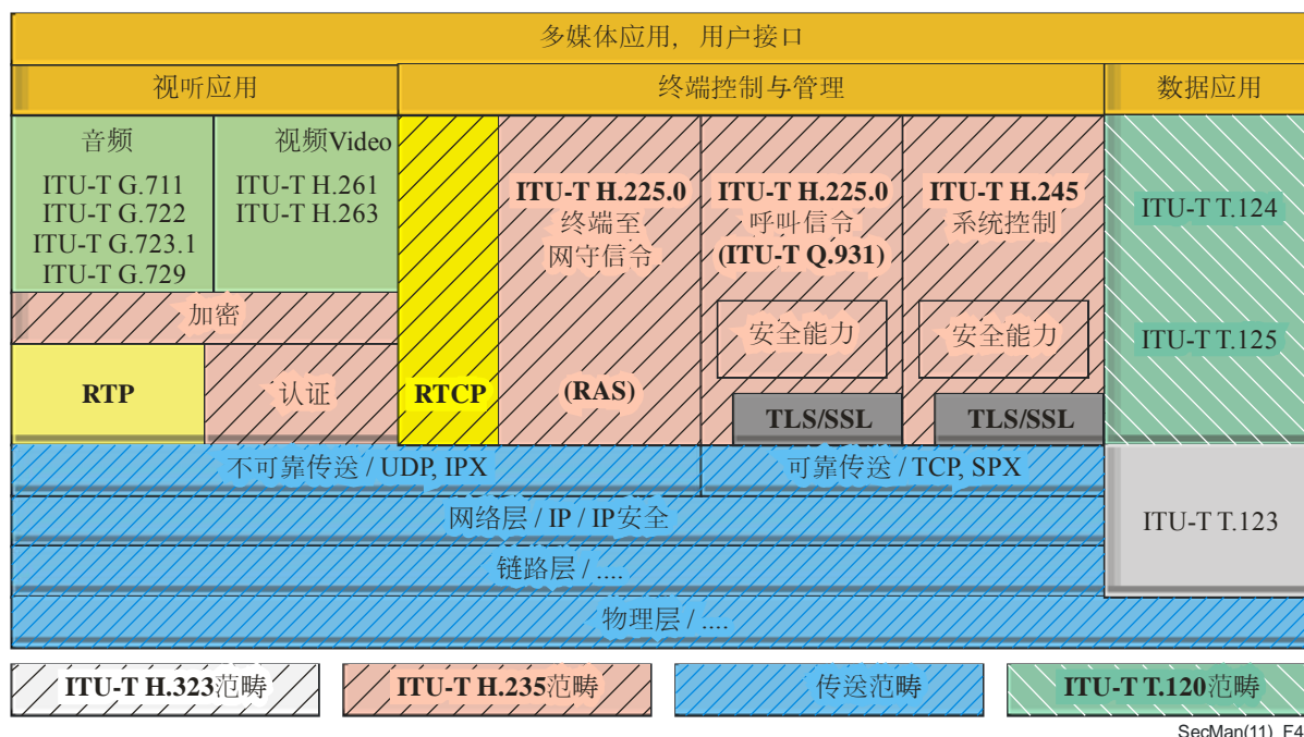
图47- ITU-T H.235提供的ITU-T H.323安全
