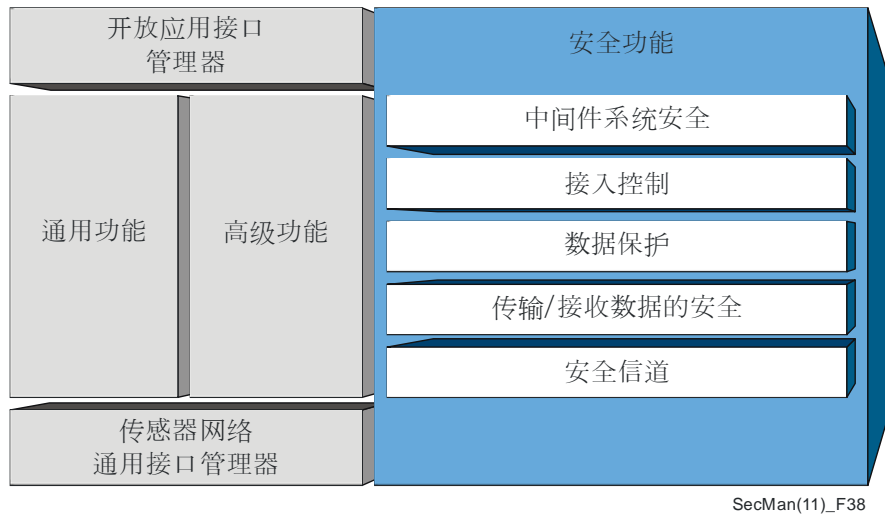
图38 – USN中间件的安全功能
