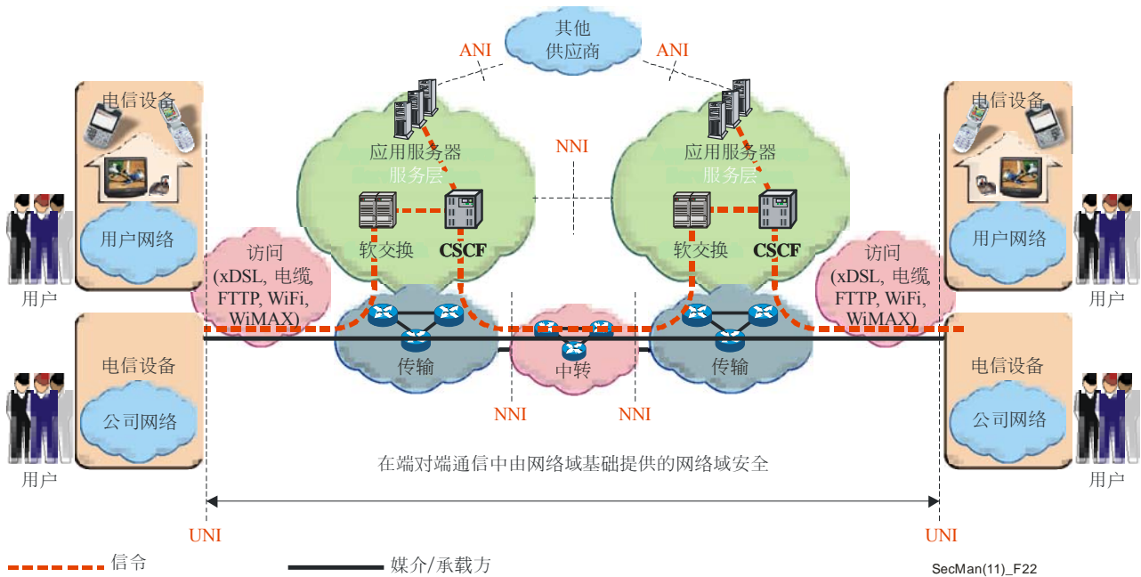
图22 – 跨多个网络的通信安全
