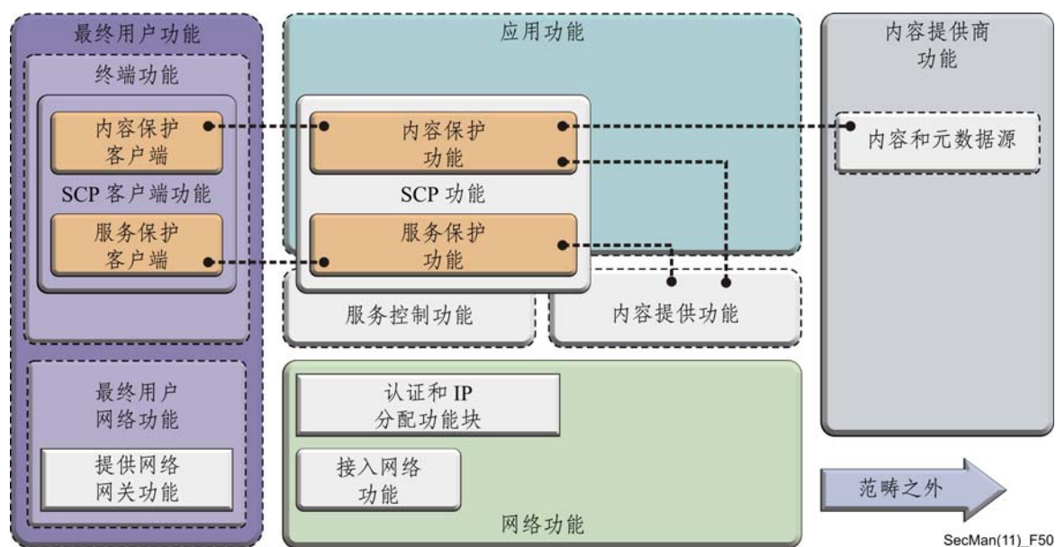
图50 - IPTV通用安全体系结构
