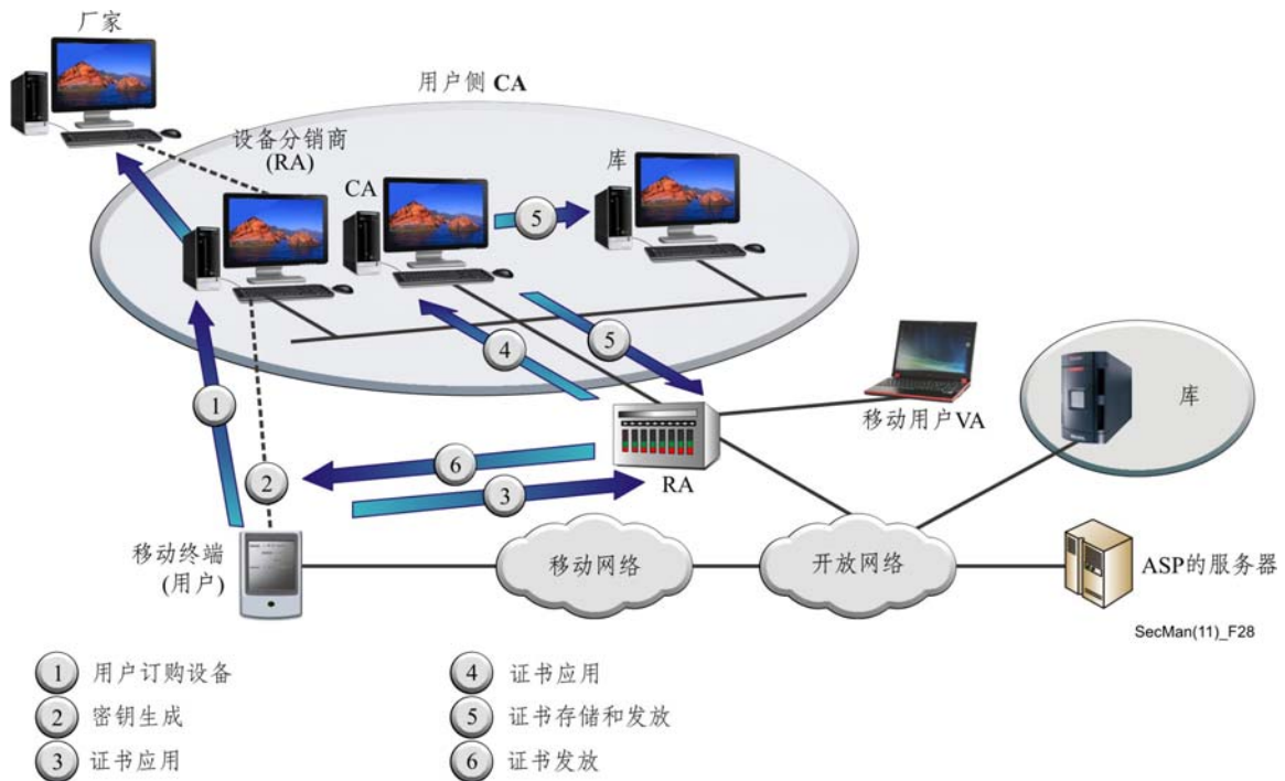
图28 – 移动终端的证书发放程序
