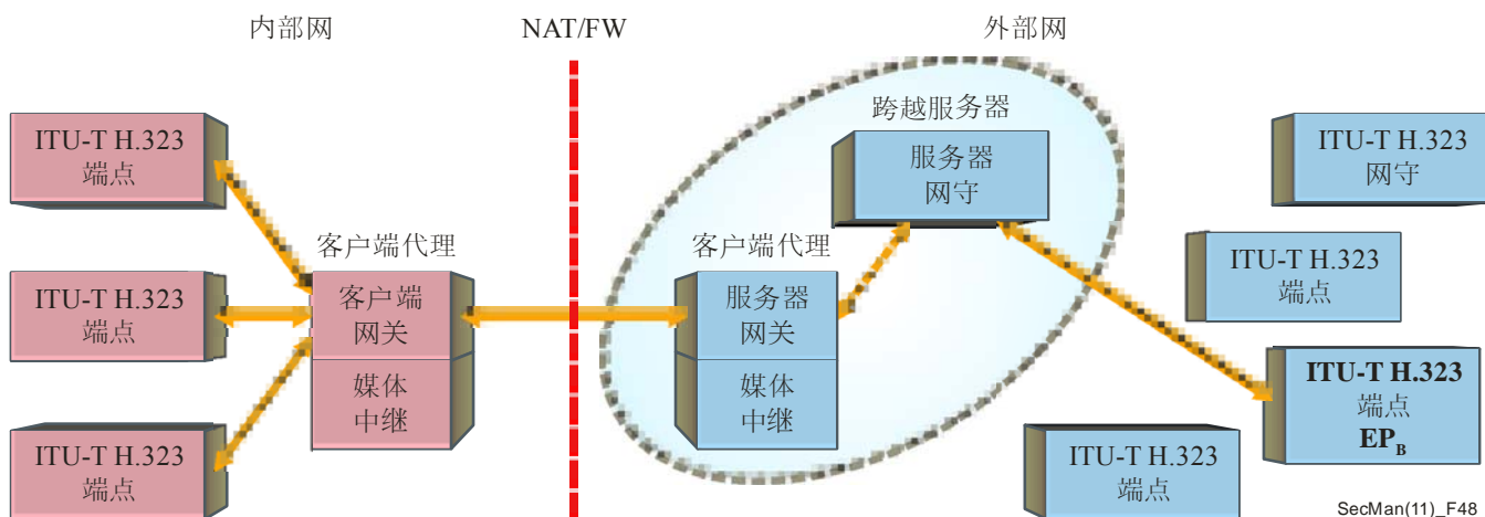
图48 – H.460.18体系结构中的NAT/FW跨越
