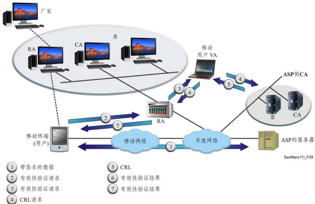
图29 – 移动端对端数据通信的证书验证程序
