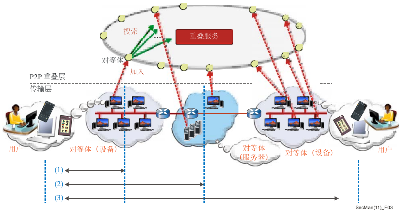
图 3 – P2P网络的体系结构参考模型
