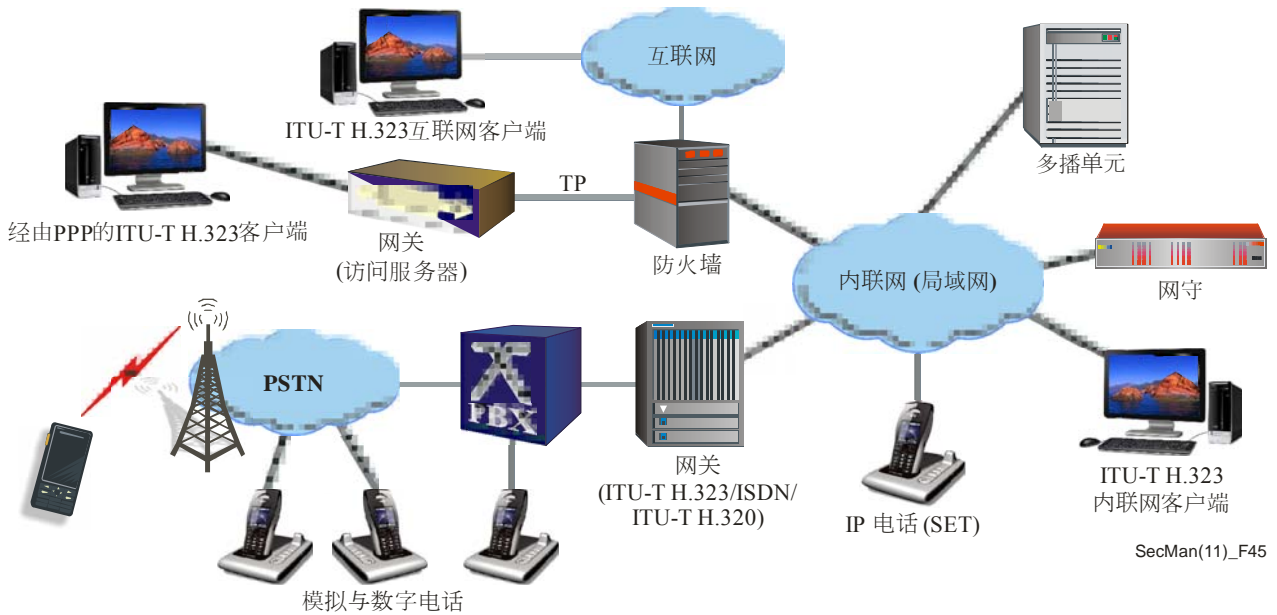
图45 – H.323系统：组成部件和配置方案
