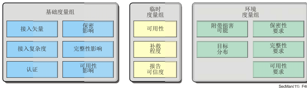
图40 – CVSS度量组
