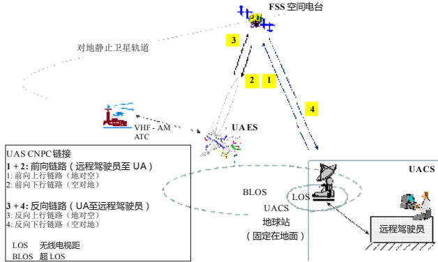
使用FSS的UAS架构组成部分
