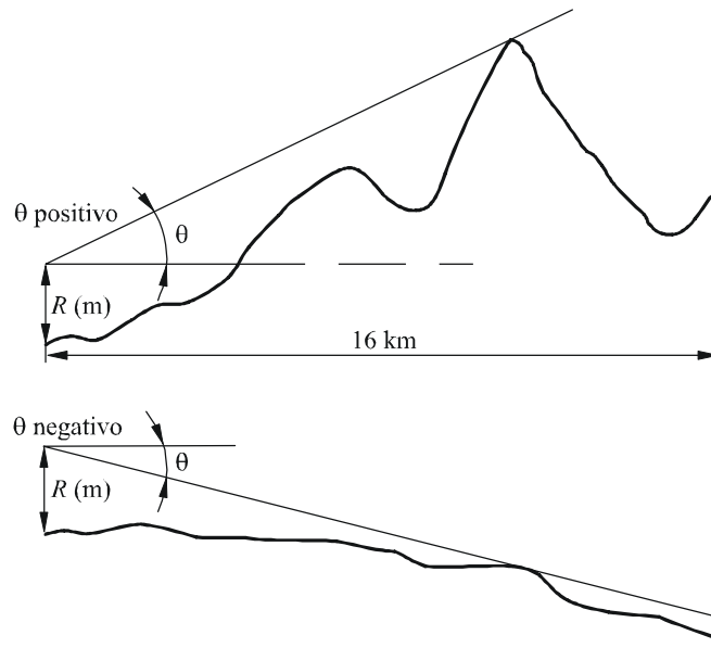
FIGURA A.2.1-3 Ángulo de despejamiento del terreno
