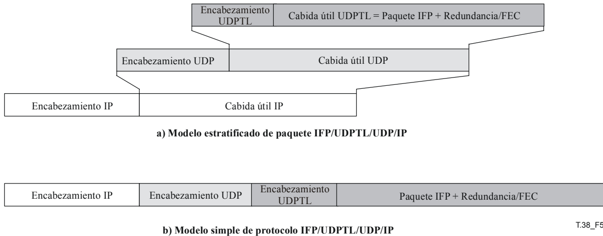
Figura 5/T.38 – Estructura de paquetes UDPTL/UDP/IP de alto nivel
