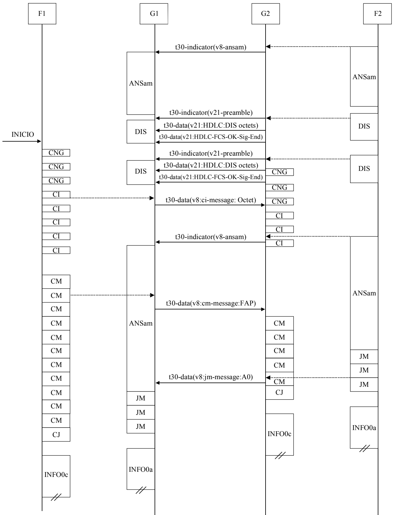
Figura IV.10/T.38 – Transmisión manual (el DIS tiene el bit 6 puesto en 1 para indicar capacidad V.8)
