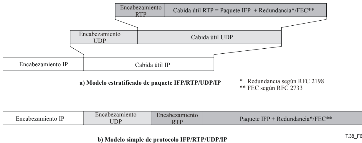
Figura 6/T.38 – Estructura de paquetes RTP/UDP/IP de alto nivel
