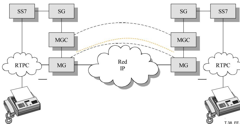
Figura E.1/T.38 – Modelo desglosado típico
