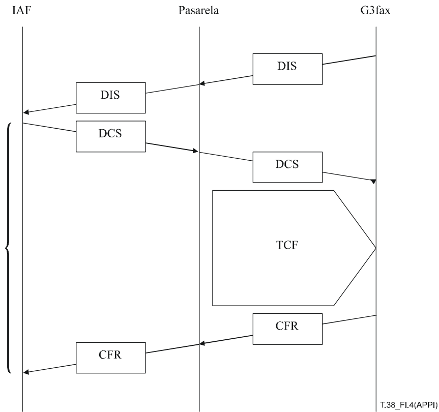
Figura I.4/T.38 – Temporización en emisión, por el dispositivo IAF, desde la DCS hasta la CFR
