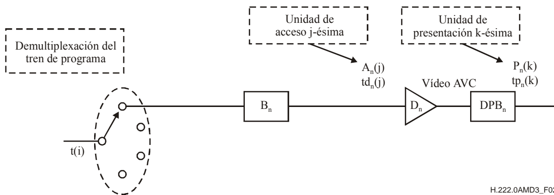
Figura 2-12 – Extensiones del modelo P-STD según la Rec. H.264 | ISO/CEI 14496-10
