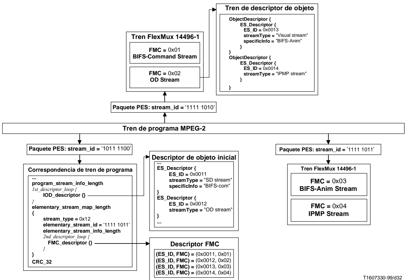
Figura R.1 – Ejemplo de contenido ISO/CEI 14496 en un tren de programa
