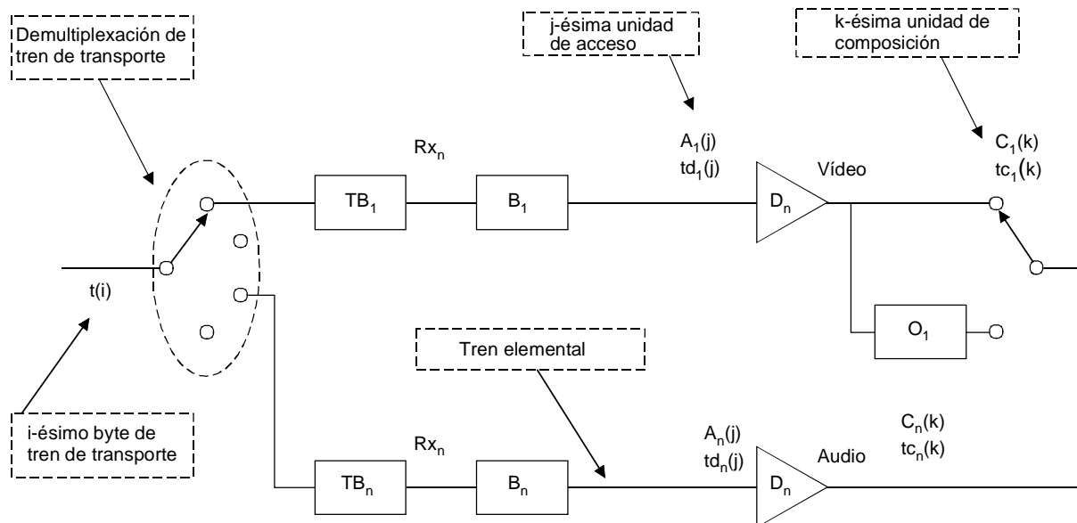
Figura 2-4 – Extensiones del modelo T-STD para trenes elementales ISO/CEI 14496 individuales
