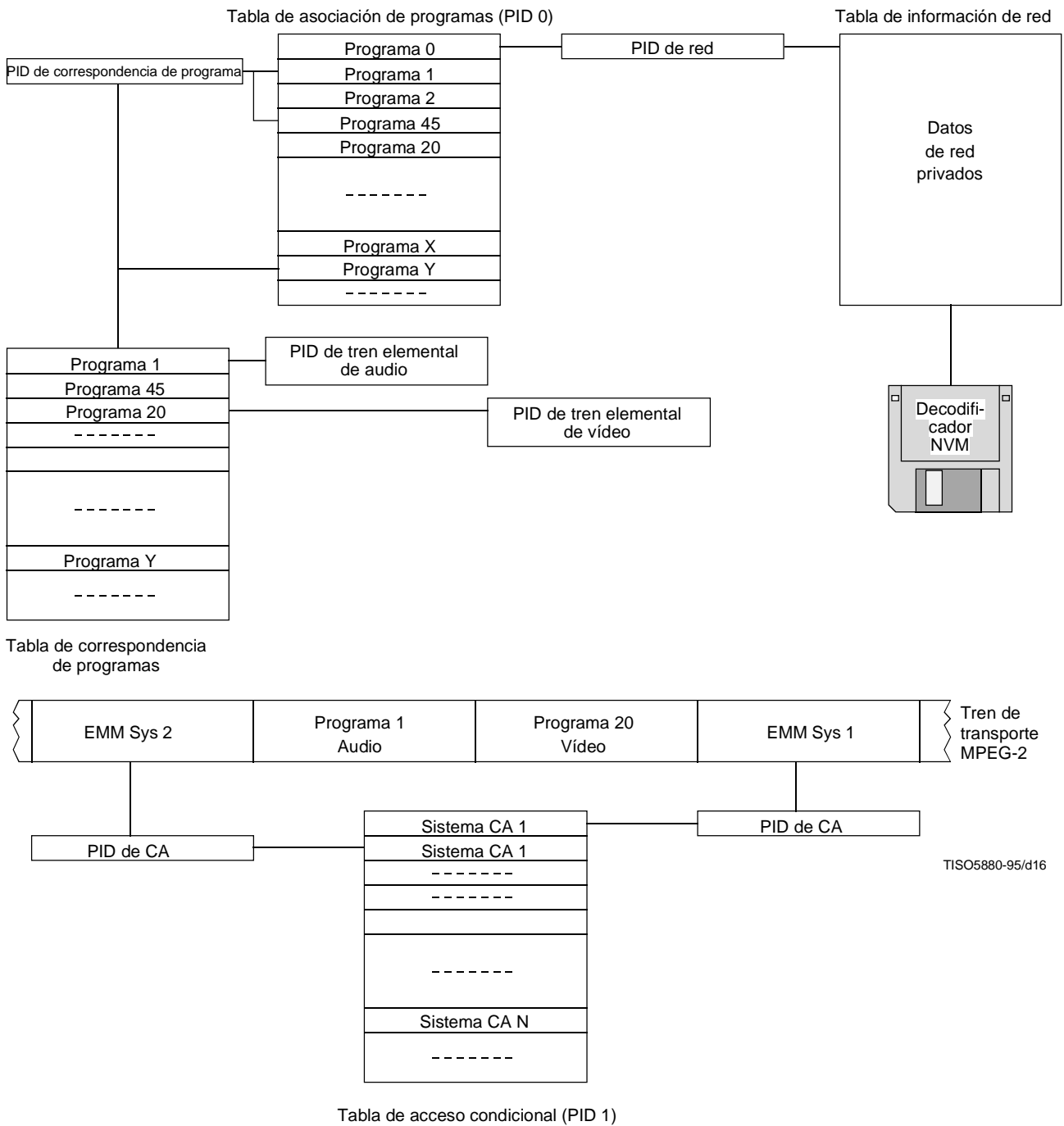
Figura C.1 – Relaciones de correspondencia de programa y red
