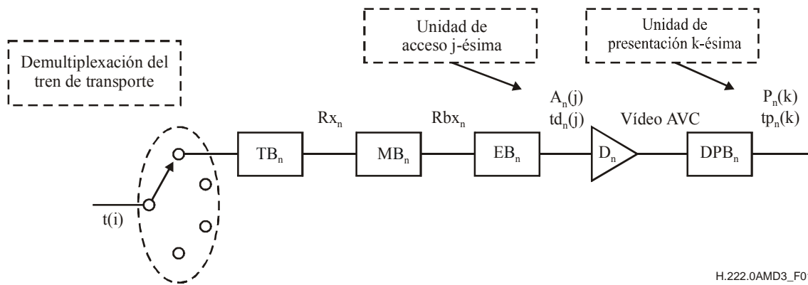
Figura 2-11 – Extensiones del modelo T-STD para vídeo de la Rec. UIT-T H.264 | ISO/CEI 14496-10
