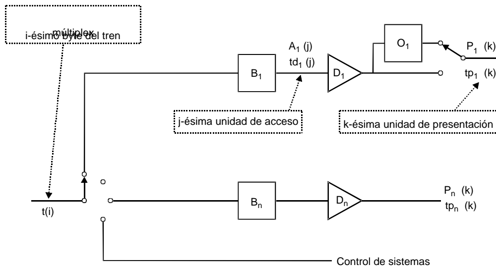
Figura 2-2 – Notación del decodificador-objetivo de sistemas del tren de programa
