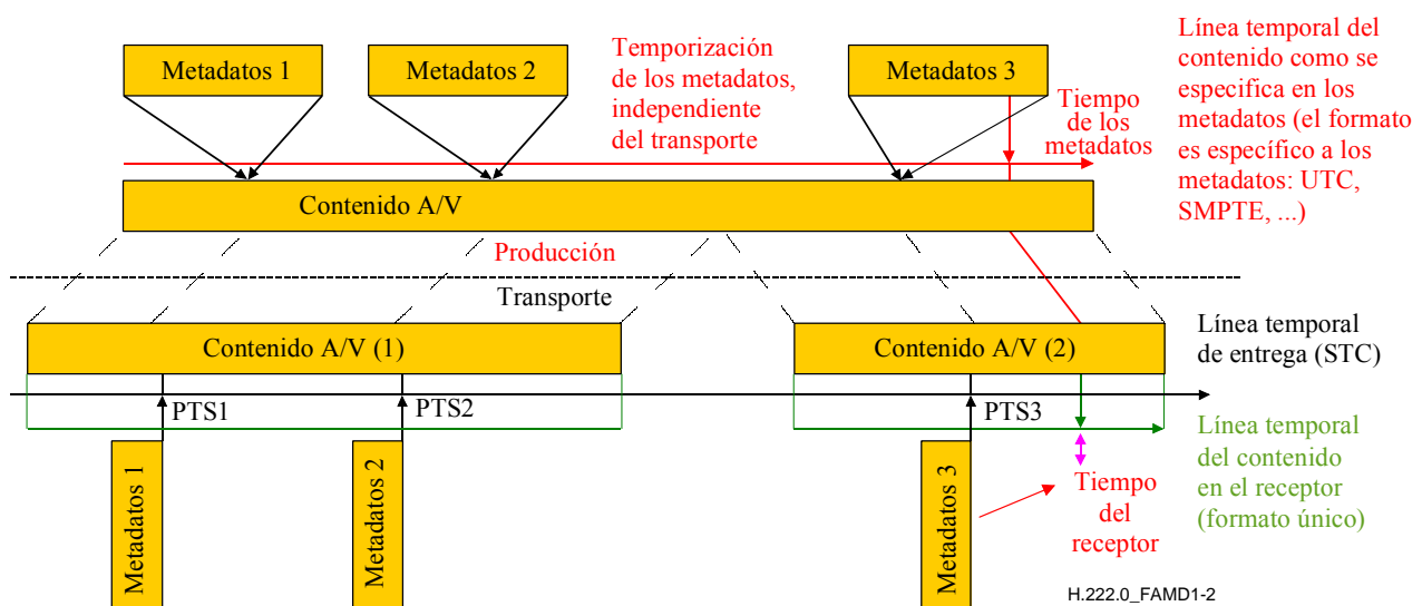
Figura 2-8 – Entrega de los metadatos en paquetes PES
