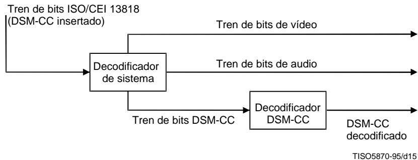
Figura B.3 – Tren de bits DSM-CC decodificado como parte del tren de bits de sistema
