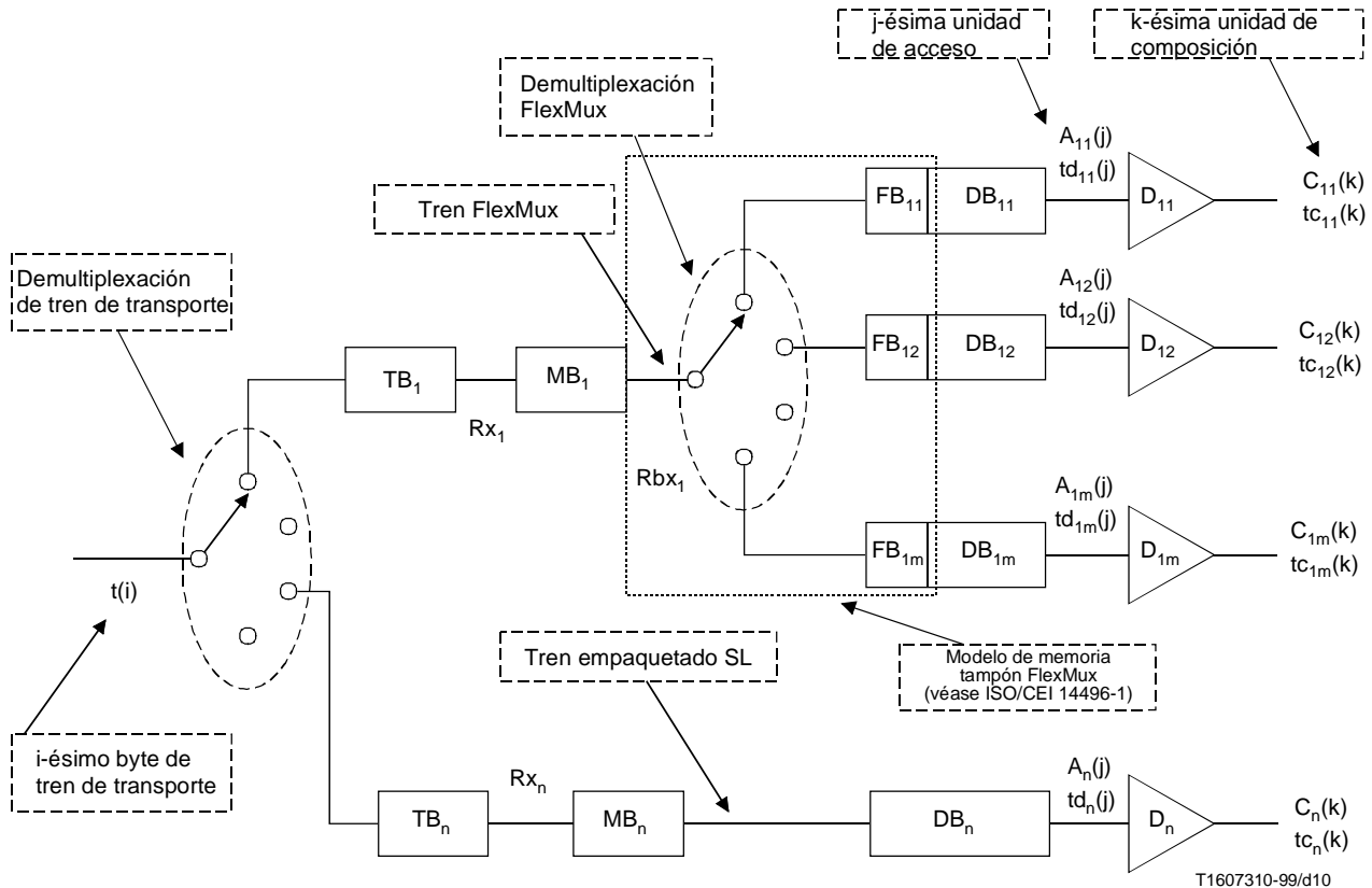
Figura 2-5 – Modelo T-STD para el contenido ISO/CEI 14496
