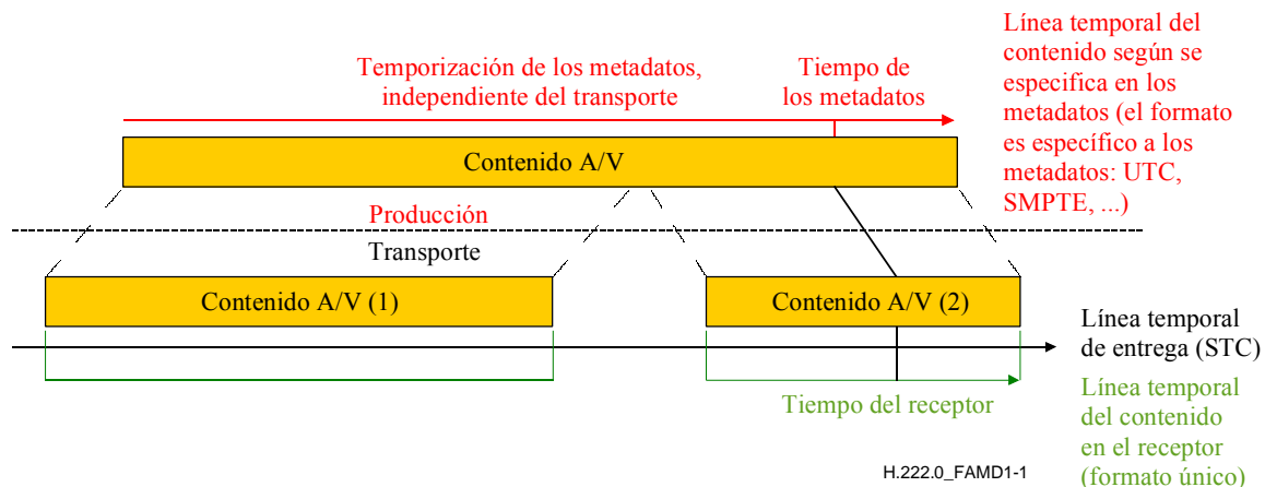
Figura 2-7 – Modelo de temporización para la entrega de contenidos y metadatos
