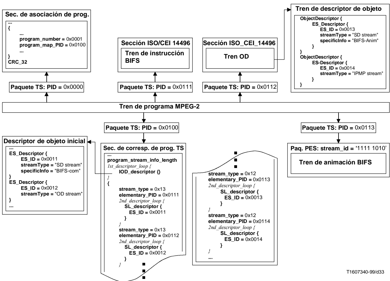
Figura R.2 – Ejemplo de contenido ISO/CEI 14496 en un tren de transporte
