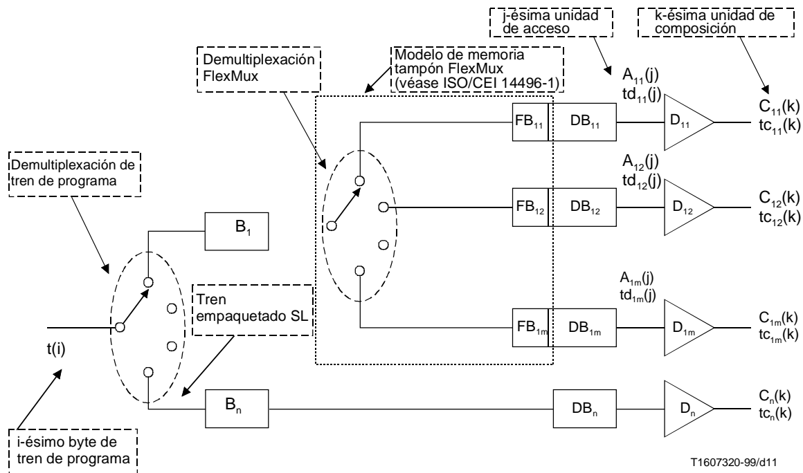
Figura 2-6 – Modelo P-STD para el tren de sistemas ISO/CEI 14496
