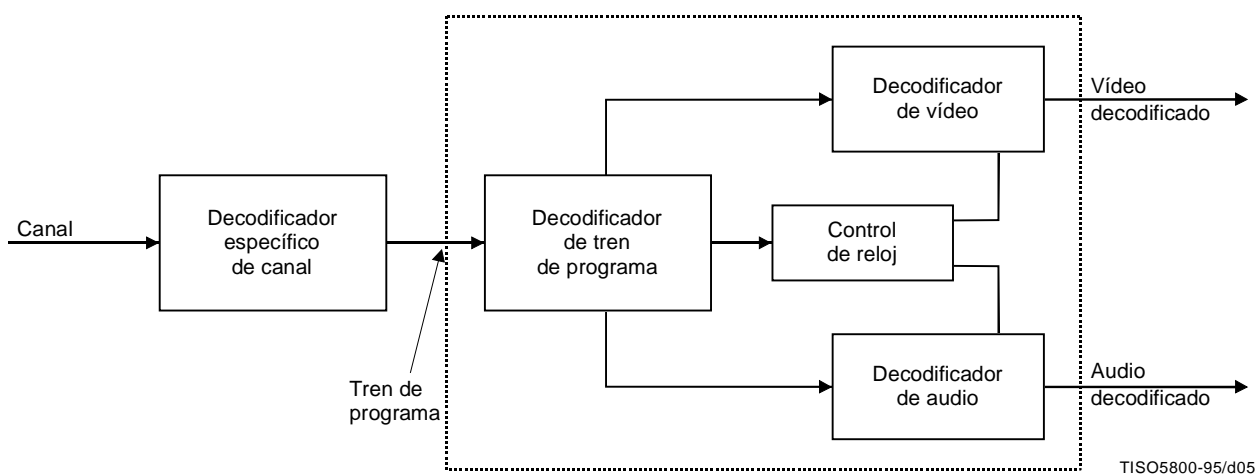
Figura Intro. 5 – Prototipo de decodificador para trenes de programa
