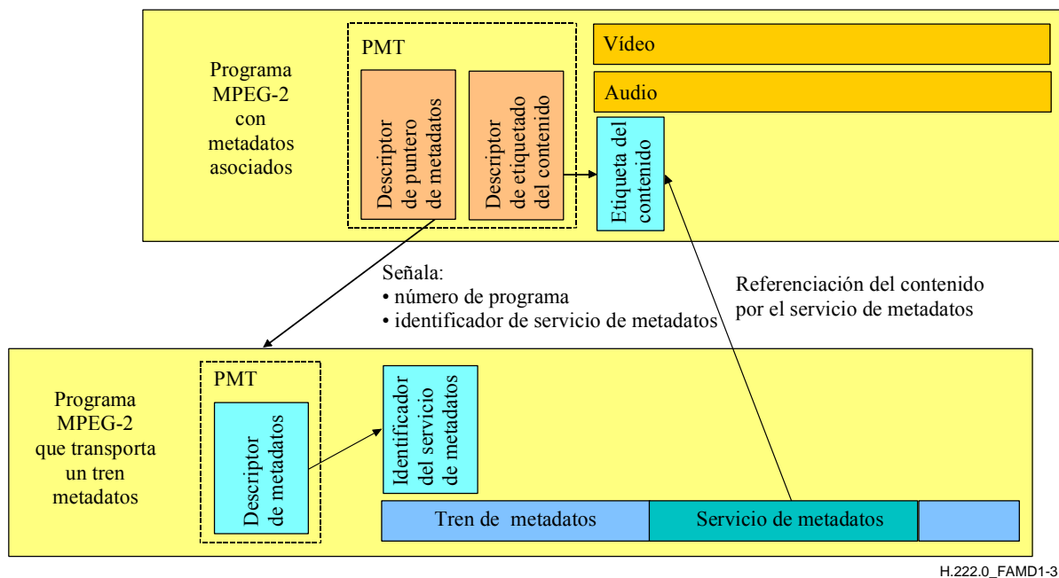
Figura 2-9 – Referenciación y señalización de los metadatos
