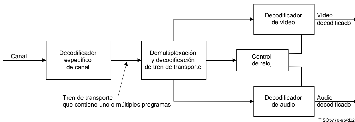
Figura Intro. 2 – Ejemplo de prototipo de demultiplexación y decodificación de tren de transporte
