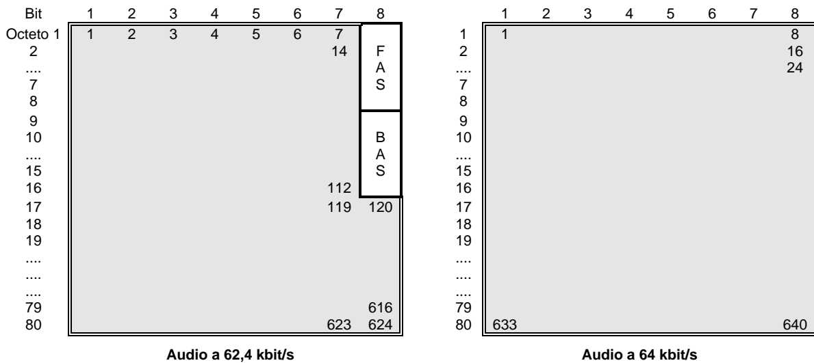
Figura 6/H.221 – Posiciones de bits para audio ISO/CEI 11172-3 en uno o dos canales a 64 kbit/s
