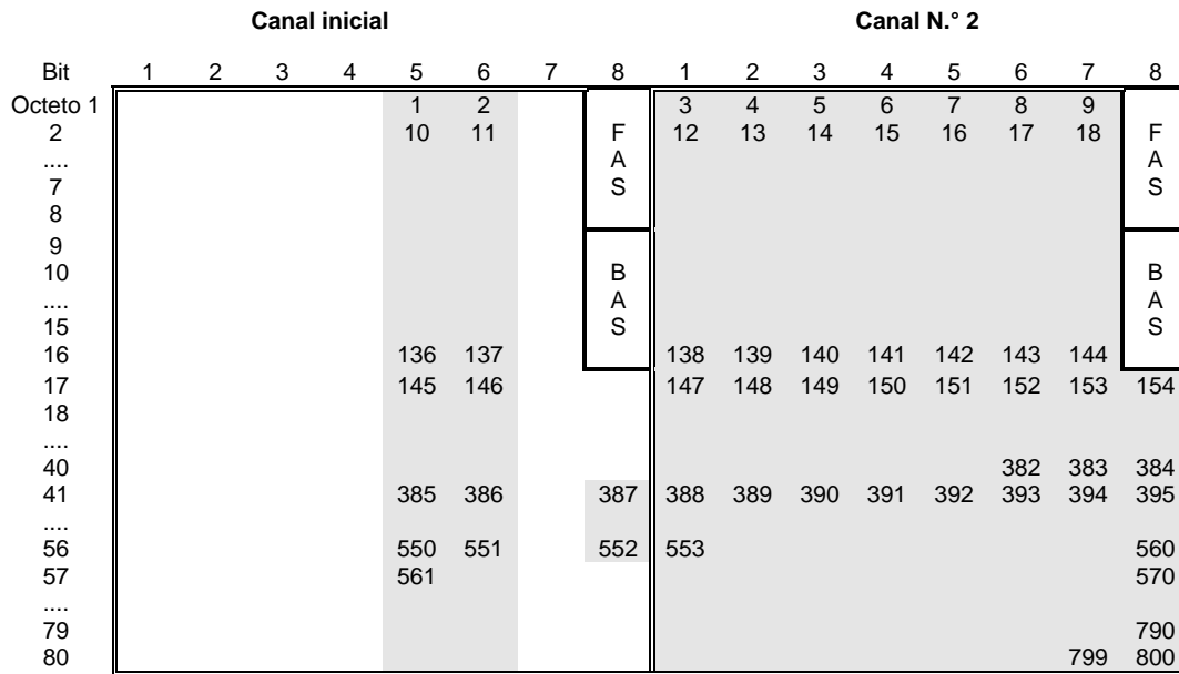
Audio a 80 kbit/s en dos canales a 64 kbit/s
