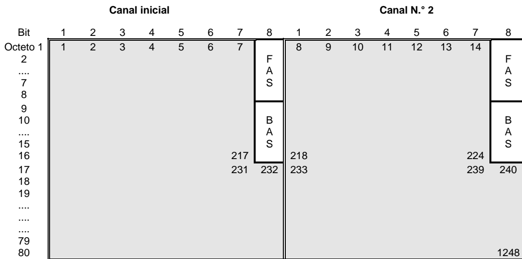
Audio a 124,8 kbit/s en dos canales a 64 kbit/s
