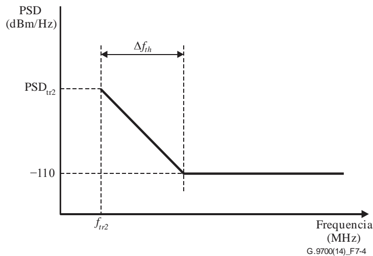
Figura 7-4 – LPM fuera de la banda en altas frecuencias
