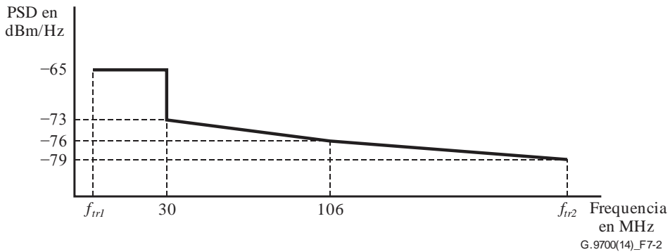
Figura 7-2 – Máscara de PSD límite dentro de la banda para el perfil 212 MHz
