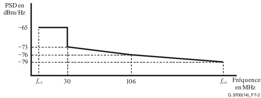
Figure 7-2 – Gabarit limite de densité PSD dans la bande pour le profil à 212 MHz
