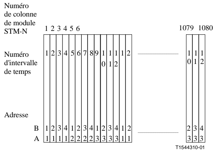
Figure 7-25/G.707/Y.1322 – Schéma de numérotage d'unités AU-3 au sein d'une rangée de pointeurs d'unités AU et des colonnes de charge utile d'un module STM-4
