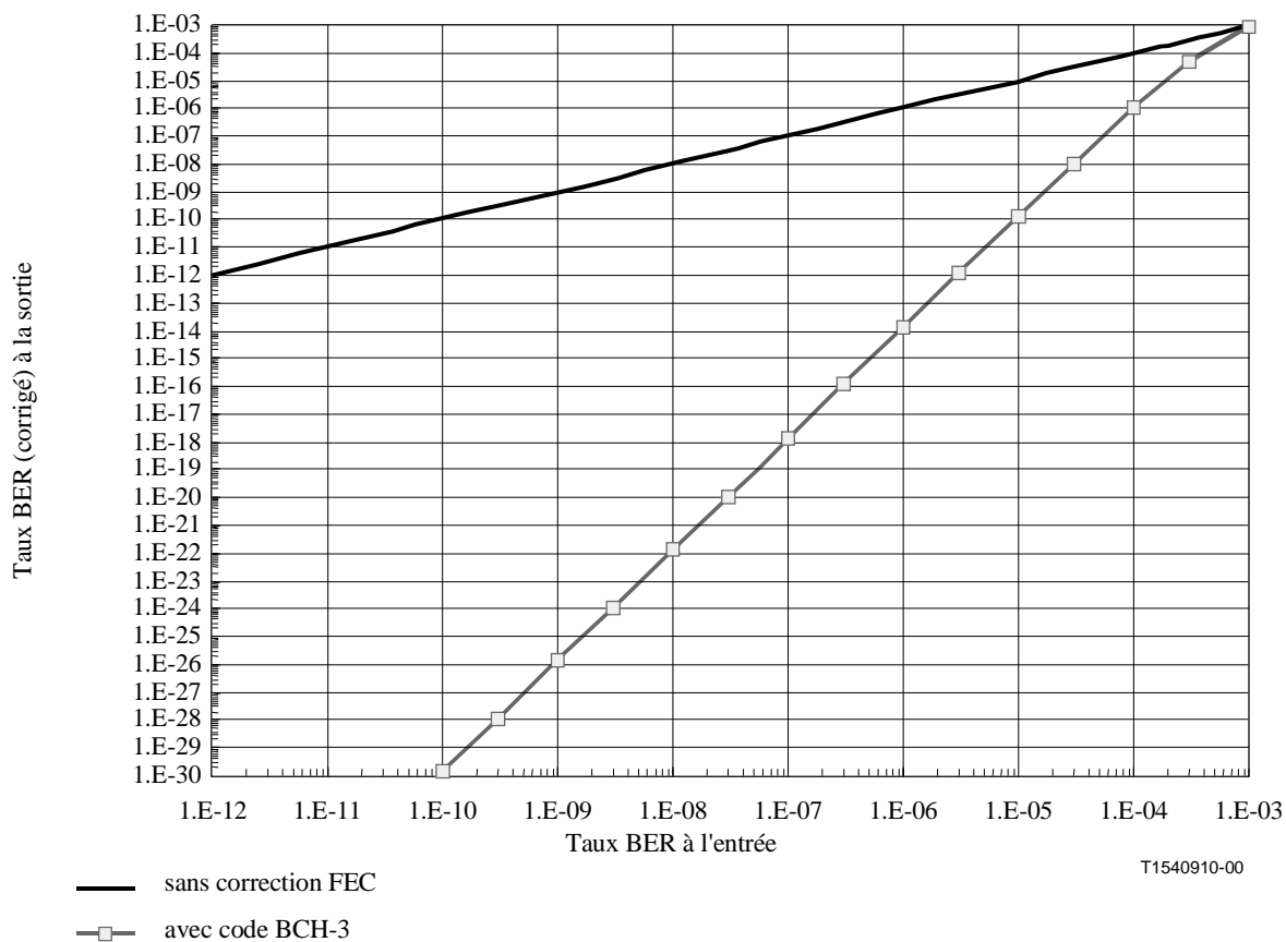
Figure X.1/G.707/Y.1322 – Taux BER (corrigé) théorique à la sortie en fonction du taux BER à l'entrée (code BCH-3)
