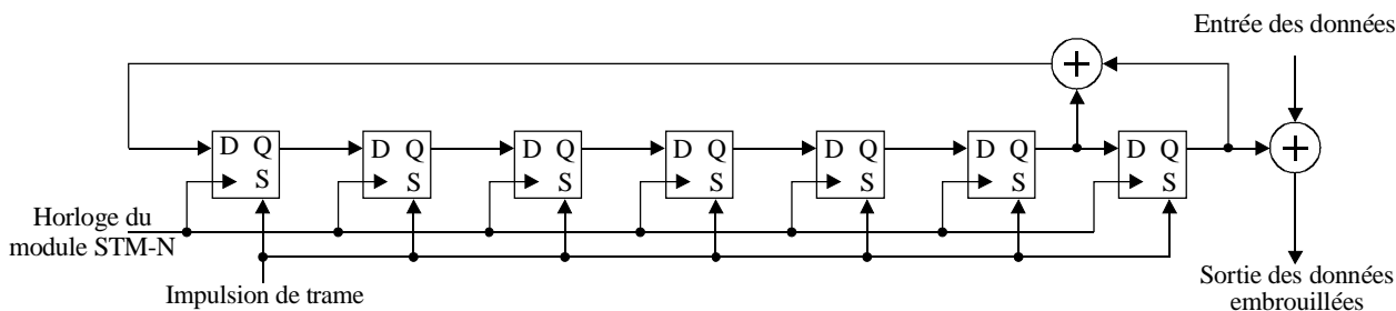
Figure 6-10/G.707/Y.1322 – Embrouilleur synchrone de trames (diagramme fonctionnel)
