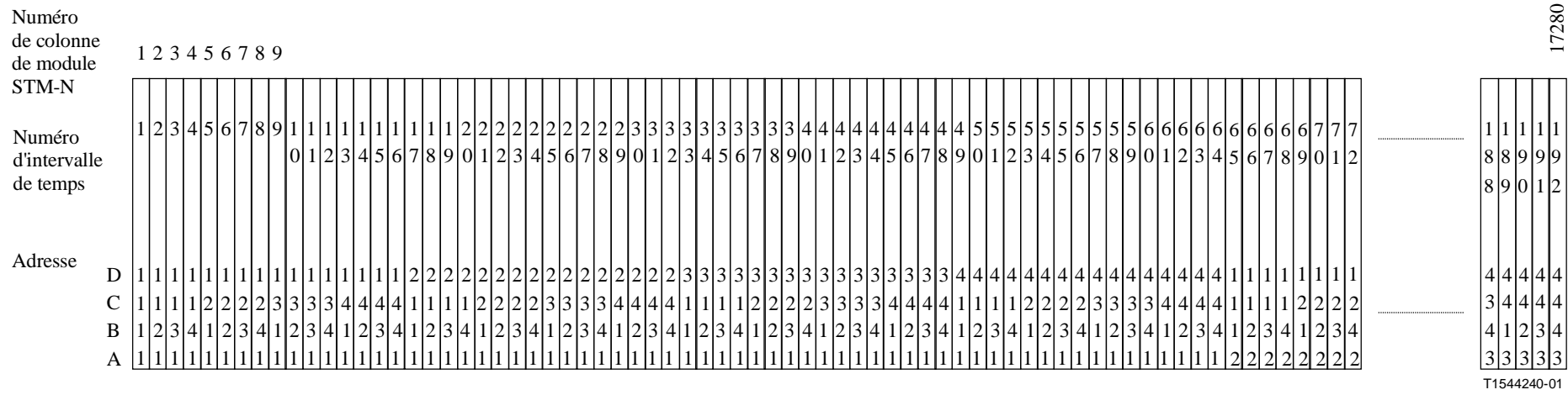
Figure 7-18/G.707/Y.1322 – Schéma de numérotage d'unités AU-3 au sein d'une rangée de pointeurs d'unités AU et des colonnes de charge utile d'un module STM-64
