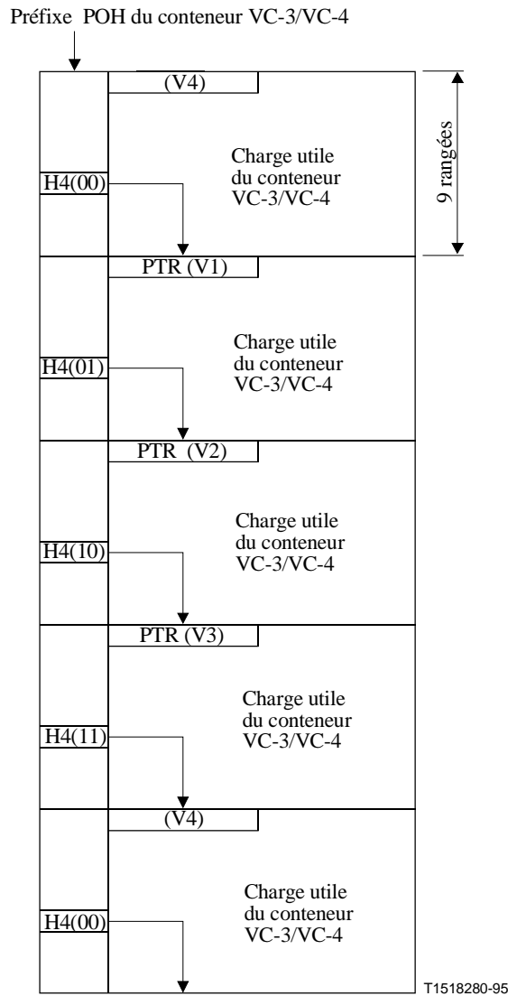
Figure 8-12/G.707/Y.1322 – Exemple d'indication de multitrames 500 µs d'unité TU-1/2 utilisant l'octet H4
