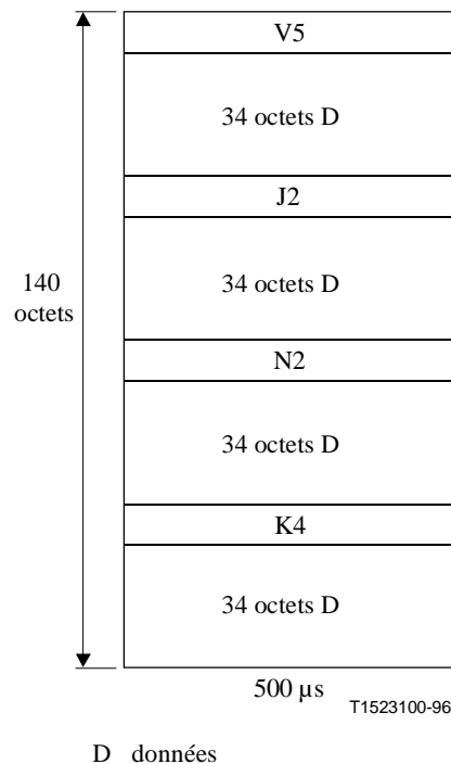
Figure 10-22/G.707/Y.1322 – Mappage de cellules ATM dans un conteneur VC-12
