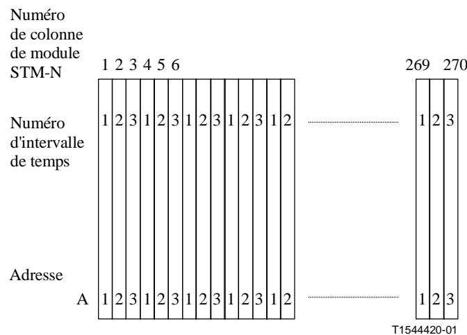
Figure 7-26/G.707/Y.1322 – Schéma de numérotage d'unités AU-3 au sein d'une rangée de pointeurs d'unités AU et des colonnes de charge utile d'un module STM-1
