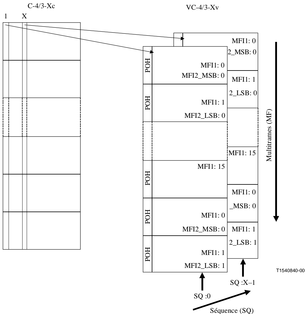
Figure 11-4/G.707/Y.1322 – Indicateur de multitrames et de séquence du conteneur VC-3/4-Xv
