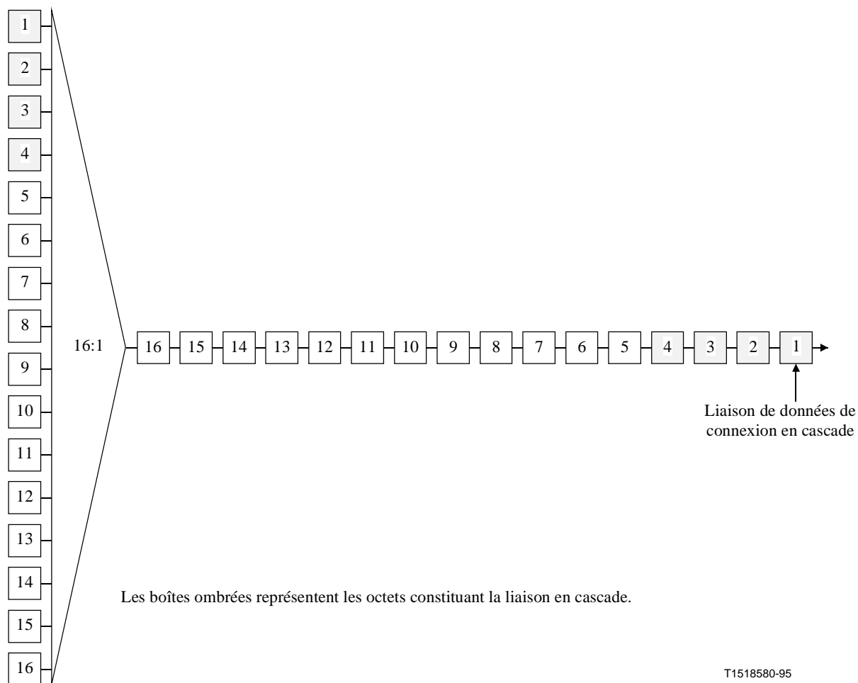
Figure C.3/G.707/Y.1322 – Exemple de connexion en cascade au débit STM-4 dans un module STM-16
