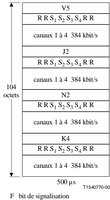
Figure 10-15/G.707/Y.1322 – Mappage synchrone d'octets pour des affluents à 384 kbit/s
