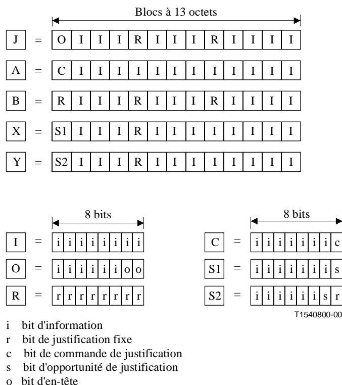
Figure 10-25/G.707/Y.1322 – Contenu des blocs pour le mappage asynchrone de l'interface FDDI
