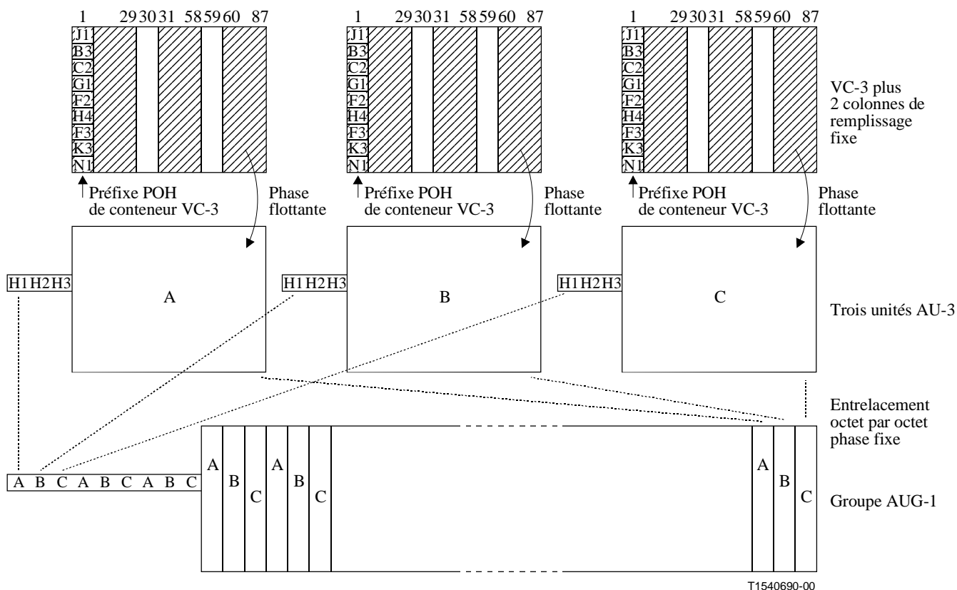
Figure 7-4/G.707/Y.1322 – Multiplexage d'unités AU-3 au moyen d'un groupe AUG-1
