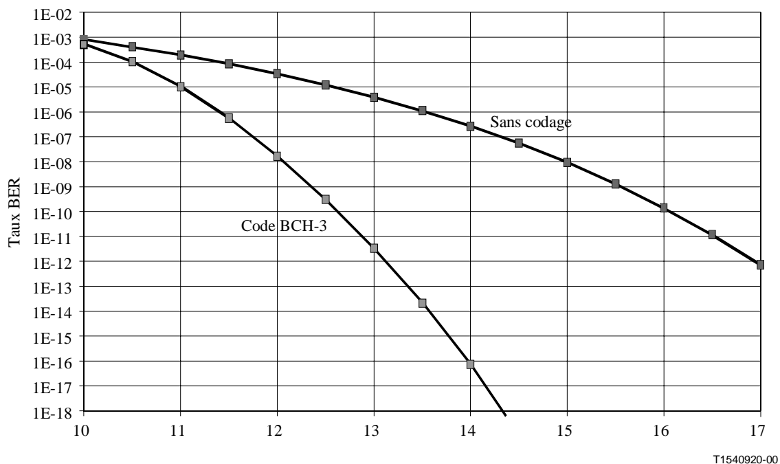
Figure X.2/G.707/Y.1322 – Taux BER (corrigé) théorique à la sortie en fonction de la valeur Q (code BCH-3)
