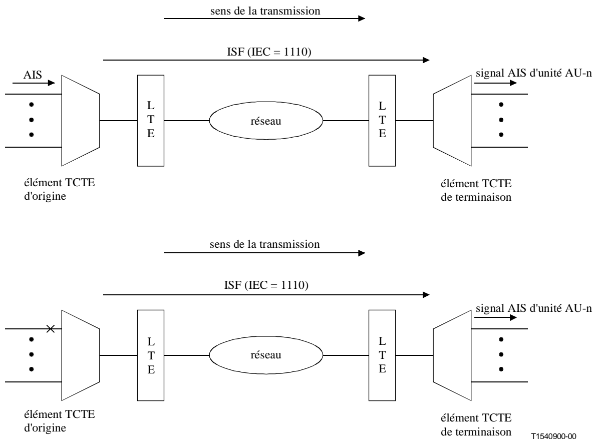
Figure C.8/G.707/Y.1322 – Connexion en cascade avec défaillances de signal entrant
