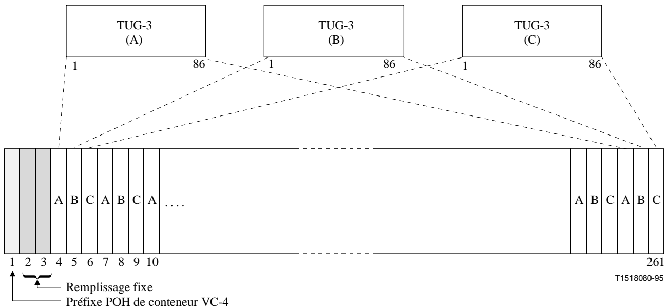
Figure 7-6/G.707/Y.1322 – Multiplexage de trois groupes TUG-3 dans un conteneur VC-4
