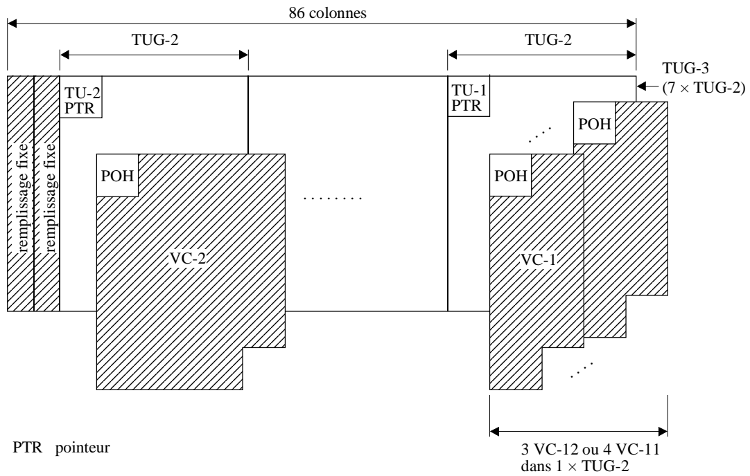
Figure 7-8/G.707/Y.1322 – Multiplexage de sept groupes TUG-2 au moyen d'un groupe TUG-3
