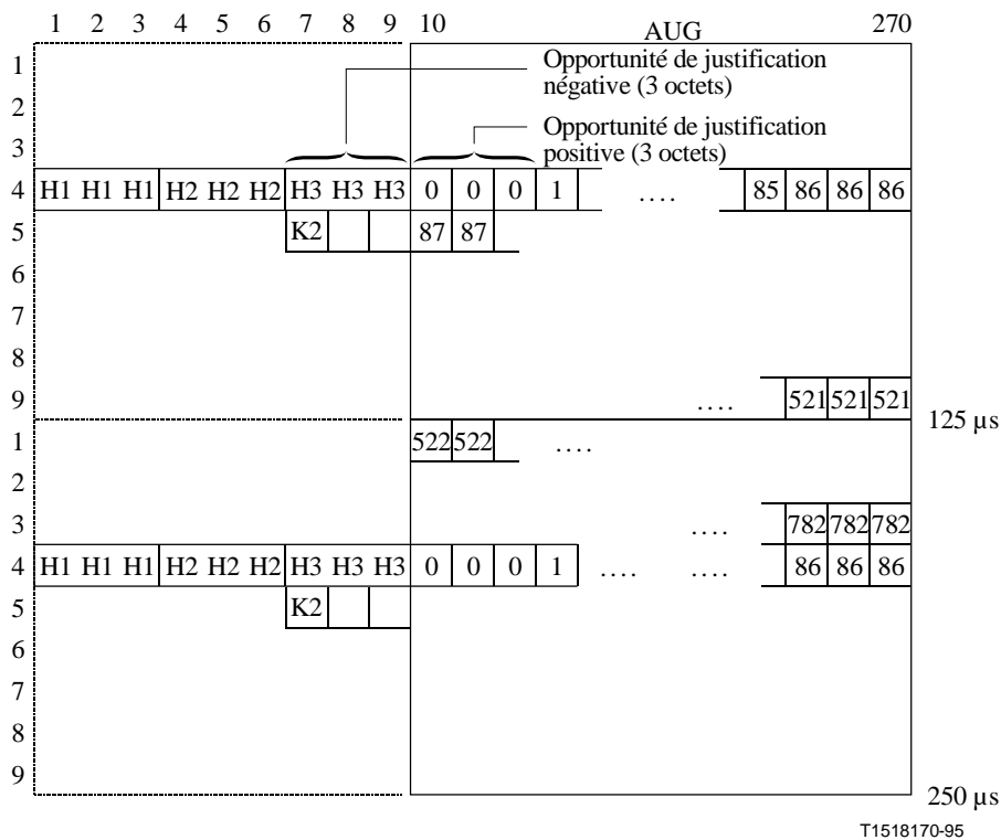
Figure 8-2/G.707/Y.1322 – Numérotage du décalage de pointeur d'unité AU-3
