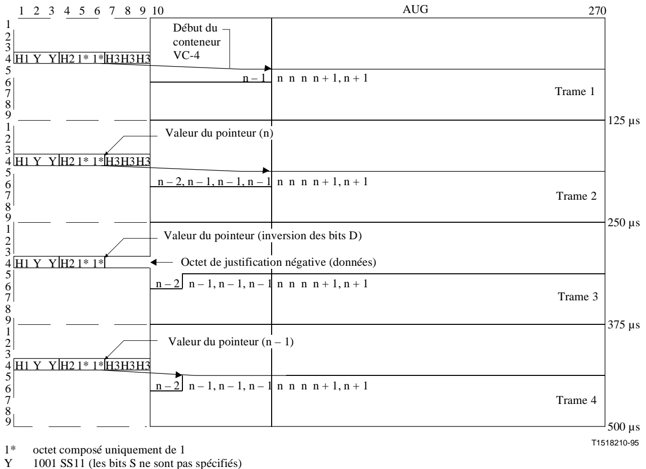
Figure 8-6/G.707/Y.1322 – Opération d'ajustement du pointeur d'unité AU-4 – Justification négative
