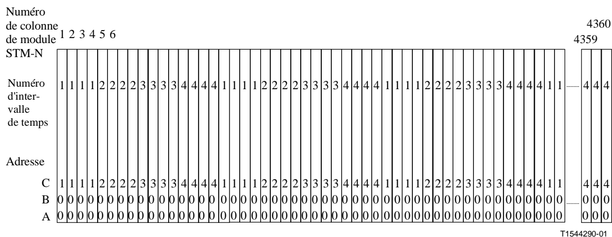
Figure 7-23/G.707/Y.1322 – Schéma de numérotage d'unités AU-4-4c au sein d'une rangée de pointeurs d'unités AU et des colonnes de charge utile d'un module STM-16
