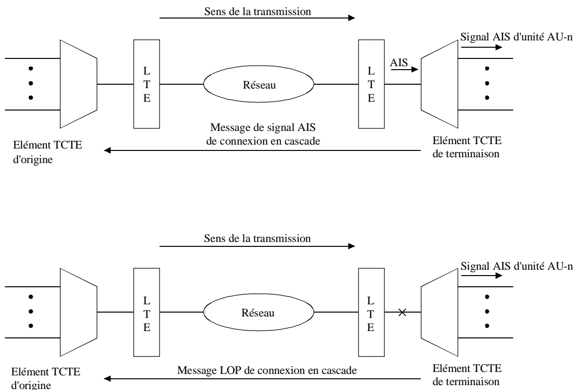
Figure C.9/G.707/Y.1322 – Défaillances de signal au sein de la connexion en cascade
