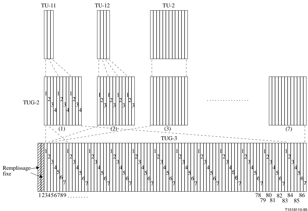
Figure 7-9/G.707/Y.1322 – Multiplexage de sept groupes TUG-2 au moyen d'un groupe TUG-3
