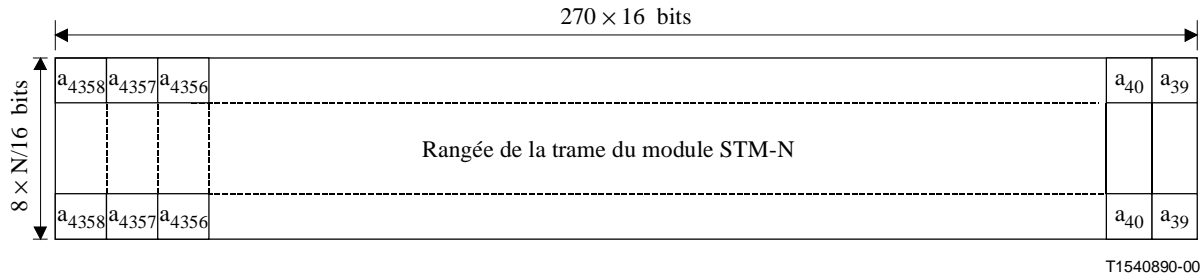
Figure A.1/G.707/Y.1322 – Bits d'information de correction FEC dans la rangée K de la trame du module STM-N
