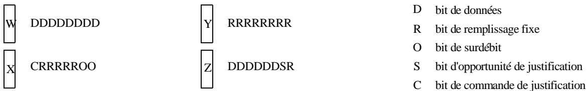
Figure 10-3/G.707/Y.1322 – Mappage asynchrone d'un affluent à 139 264 kbit/s dans un conteneur VC-4
