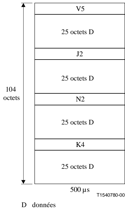
Figure 10-23/G.707/Y.1322 – Mappage de cellules ATM dans un conteneur VC-11
