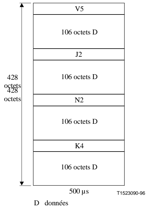
Figure 10-21/G.707/Y.1322 – Mappage de cellules ATM dans un conteneur VC-2
