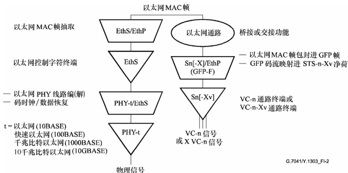
图 I.2/G.7041/Y.1303—使用GFP-F帧映射进SDH网元的以太网 分支接口端口
