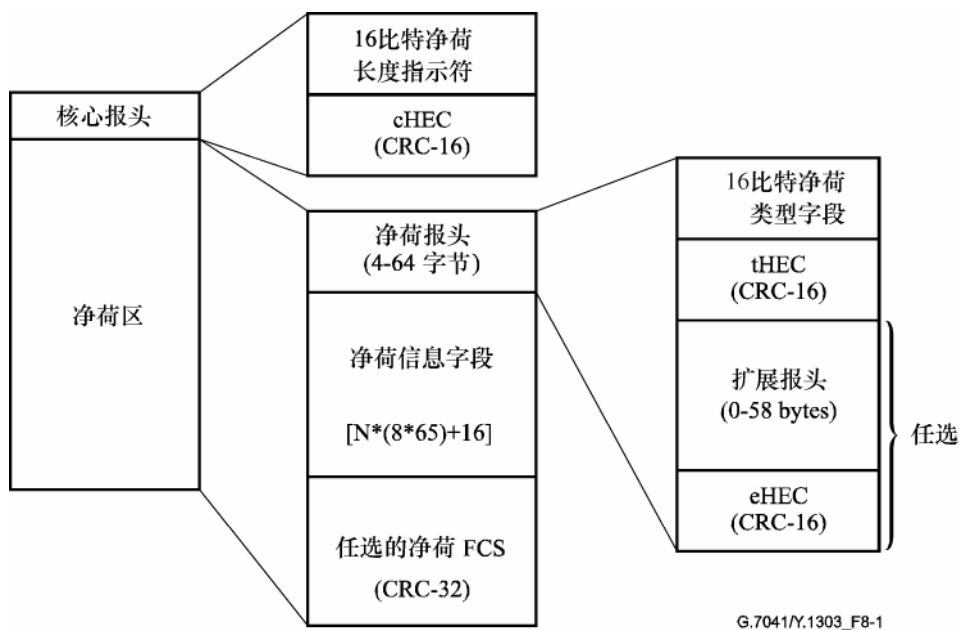
图 8-1/G.7041/Y.1303—透明GFP帧的格式
