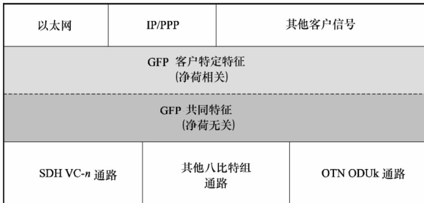
图 1/G.7041/Y.1303—GFP与客户信号和传送通路的关系
