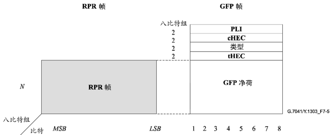
图 7-5/G.7041/Y.1303—RPR帧和GFP帧的关系
