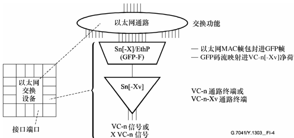
图 I.4/G.7041/Y.1303— 以太网交换或以太网交换功能上的VC-n-Xv端口嵌入混合SDH/以太网设备
