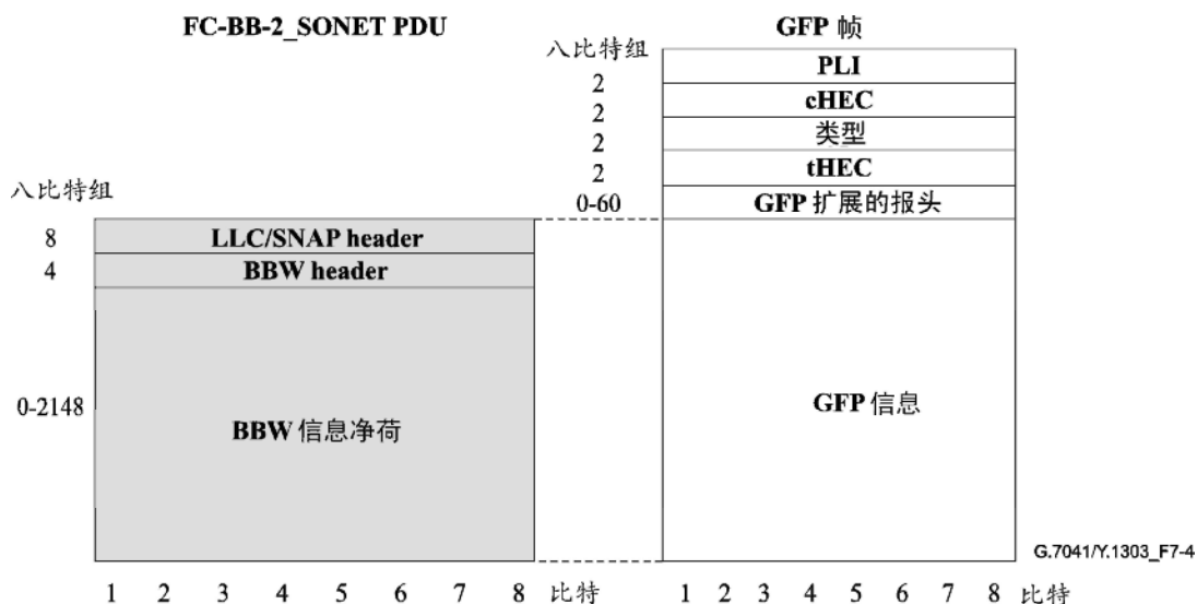
图 7-4/G.7041/Y.1303—光纤通道宽带-2 SONET (FC-BBW_SONET) 和GFP帧的关系
