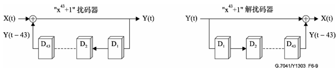
图 6-9/G.7041/Y.1303—GFP用的 x^{43}+1 扰码器和解扰码器过程
