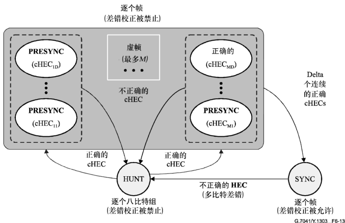
图 6-13/G.7041/Y.1303—GFP帧描述状态图
