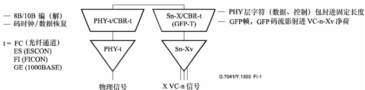
图 I.1/G.7041/Y.1303—采用全速率GFP-T 映射进SDH网元的FC/ES/FI/GE分支接口端口
