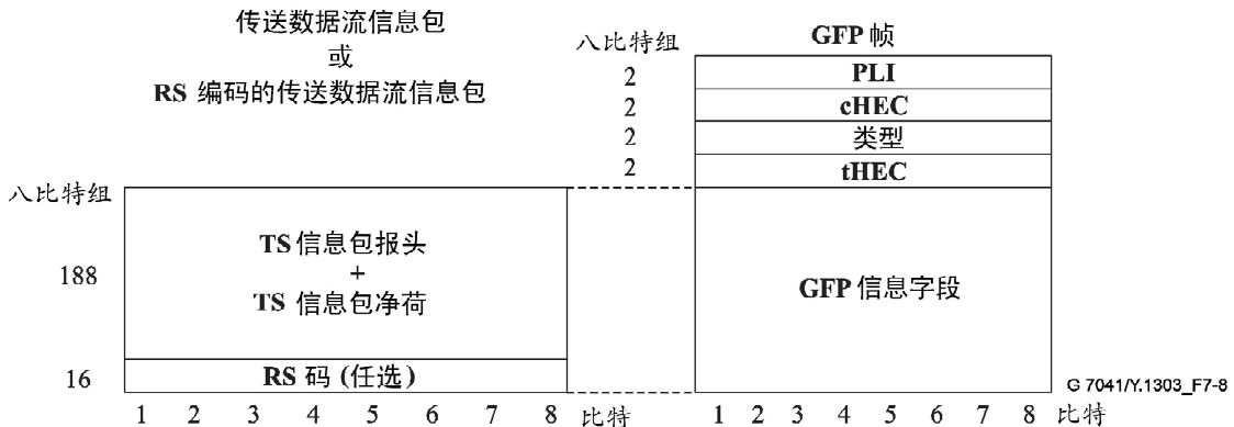
图 7-8/G.7041/Y.1303 — TS信息包和GFP帧的关系
