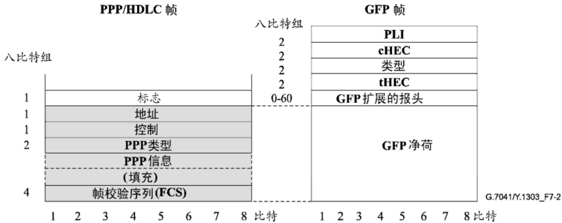
图 7-2/G.7041/Y.1303—HDLC/PPP和GFP帧的关系
