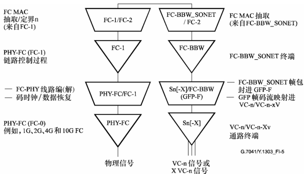
图 I.5/G.7041/Y.1303 – 利用FC-BBW_SONET和GFP-F映射进SDH网元的光纤通道支路接口端口
