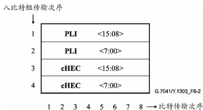
图 6-2/G.7041/Y.1303—GFP核心报头格式
