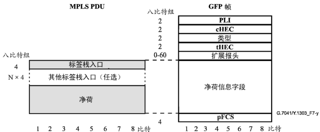
图 7-6/G.7041/Y.1303—MPLS PDU和GFP帧的关系
