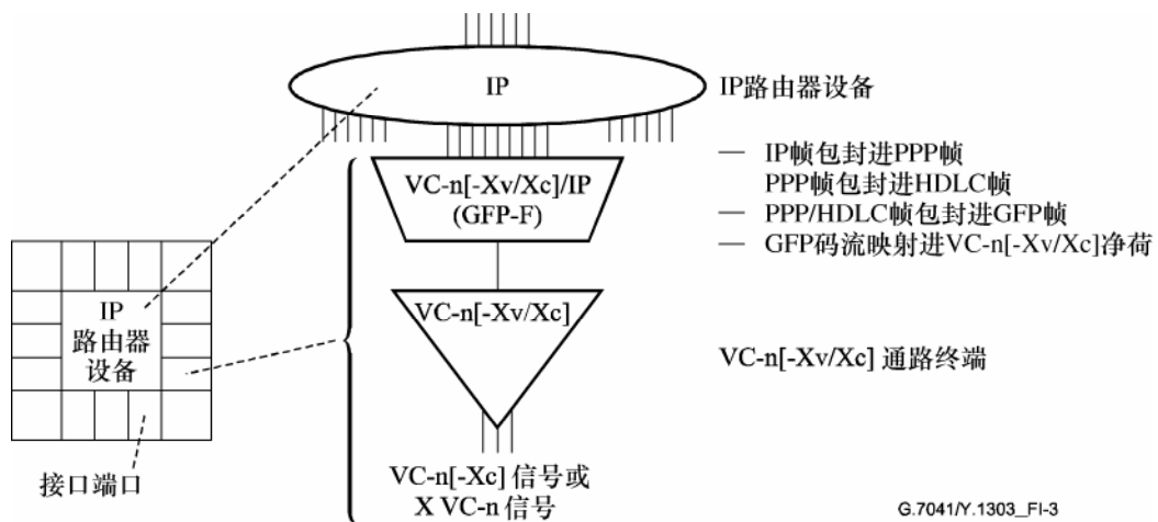
图 I.3/G.7041/Y.1303— 在IP路由器或IP路由器功能上VC-n/VC-n-Xv/VC-n-Xc端口嵌进混合SDH/IP设备
