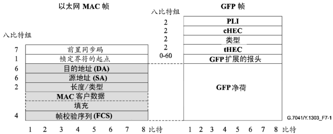
图 7-1/G.7041/Y.1303—以太网和GFP帧的关系
