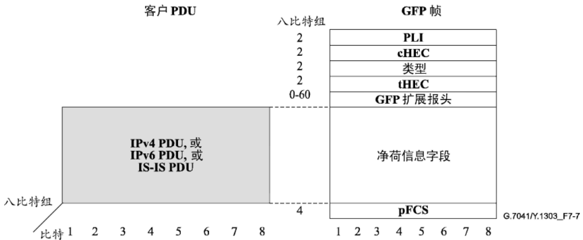
图 7-7/G.7041/Y.1303 — IPv4/IPv6/IS-IS PDU和GFP帧的关系
