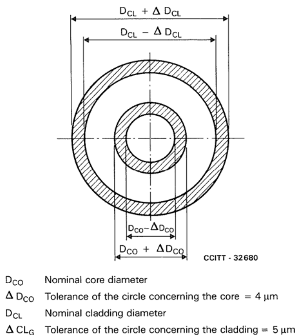
FIGURE B-1/G.651
