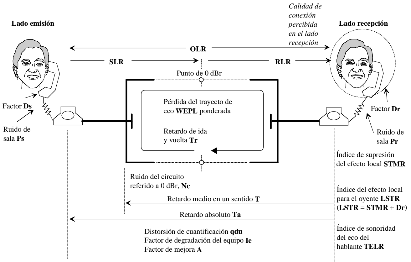
Figura 1/G.107 – Conexión de referencia del modelo E
