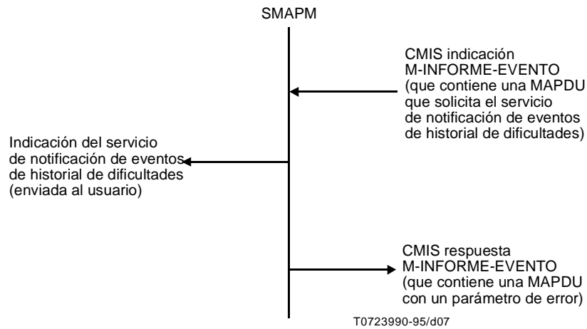
Figura 9-3/X.791 – Recepción de petición (Cometido de gestor)
