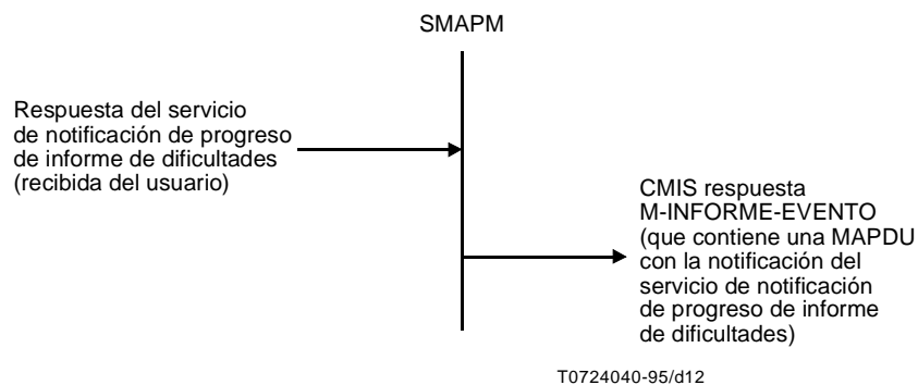
Figura 9-8/X.791 – Respuesta (Cometido de gestor)
