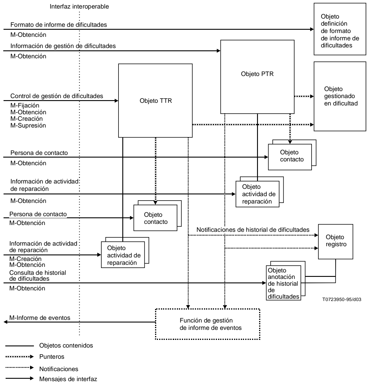
Figura 7-3/X.791 – Visión general del modelo teórico de gestión de dificultades
