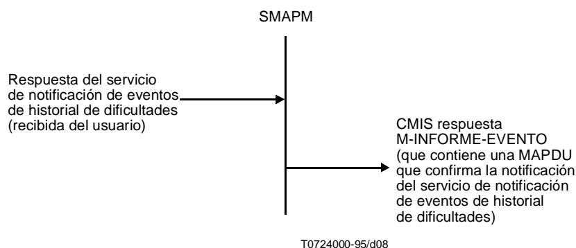
Figura 9-4/X.791 – Respuesta (Cometido de gestor)
