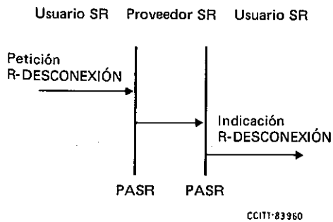
FIGURA A-11/T.70 Liberación de una CR iniciada por el usuario SR
