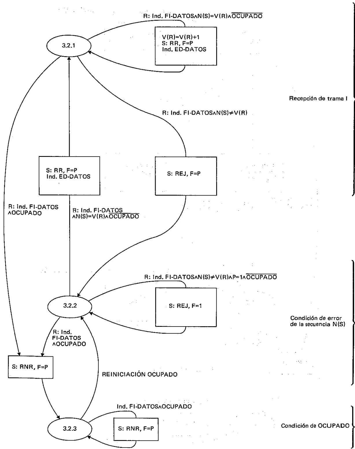
FIGURA D-15/T.70 Diagrama de transición de estados HDLC (3.2 Fase de transferencia de información, acuse de recibo de las tramas I en condiciones excepcionales)
