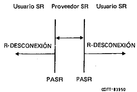
FIGURA A-12/T.70 Liberación de una CR iniciada por el proveedor SR
