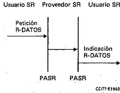
FIGURA A-9/T.70 Transferencia R-DATOS
