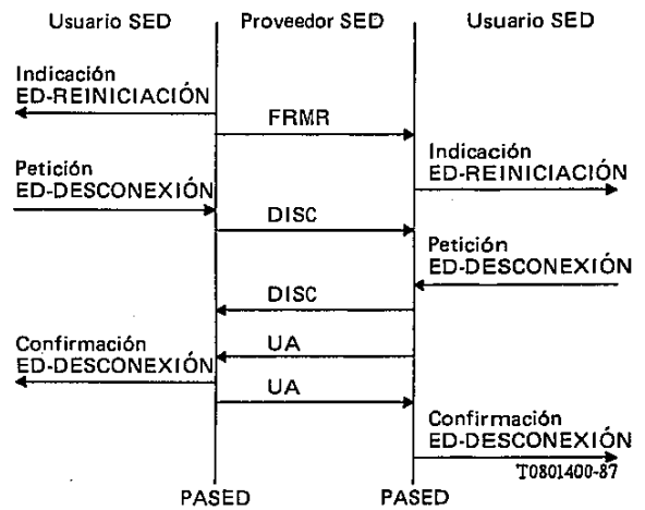
FIGURA D-10/T.70 Reiniciación no aceptada por ninguno
