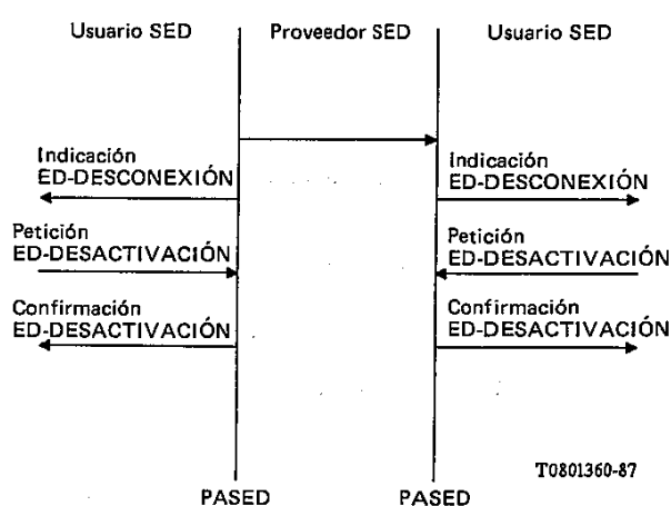
FIGURA D-6/T.70 Liberación del enlace de datos iniciada por el proveedor del enlace de datos
