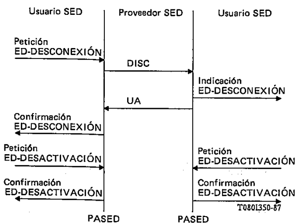
FIGURA D-5/T.70 Liberación del enlace de datos iniciada por un usuario ED
