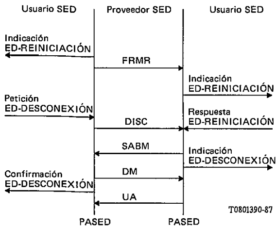
FIGURA D-9/T.70 Reiniciación no soportada por el emisor de FRMR
