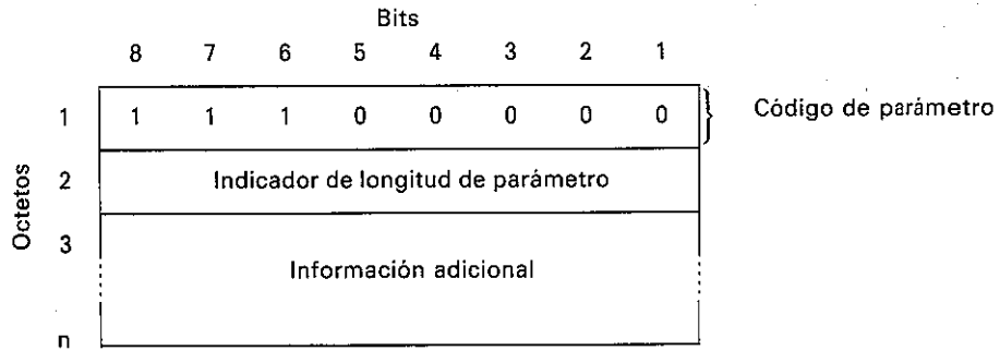
FIGURA 14/T.70 Parámetro de información adicional de liberación
