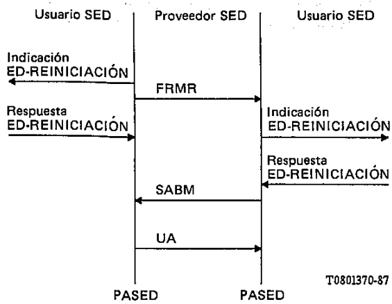
FIGURA D-7/T.70 Reiniciación fructuosa
