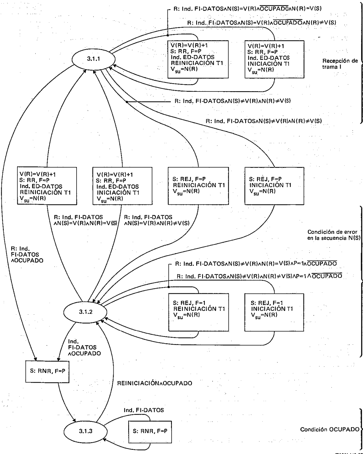
FIGURA D-14/T.70 Diagrama de transición de estados HDLC (3.1 Fase de transferencia de información, acuse de recibo de las tramas I)
