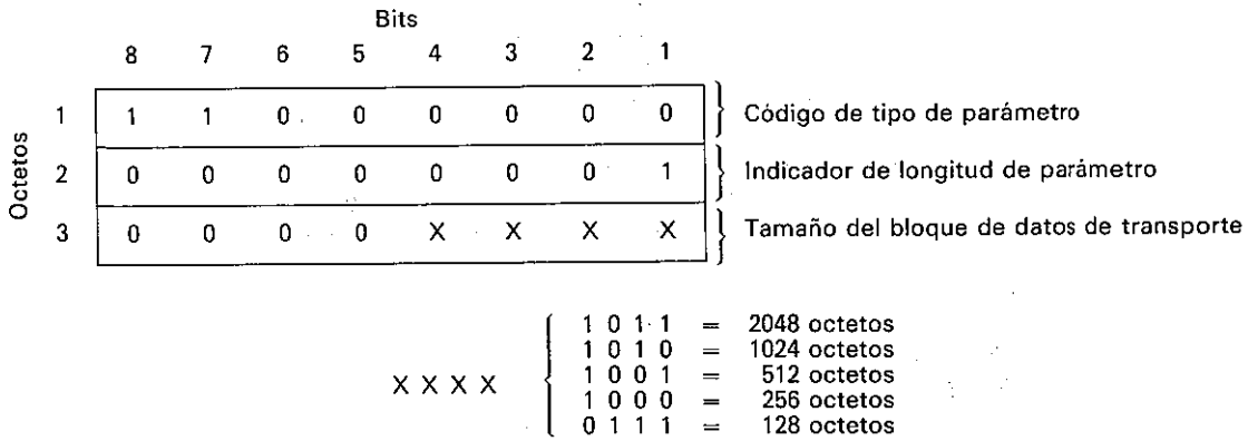
FIGURA 11/T.70 Parámetro del tamaño del bloque de datos de transporte
