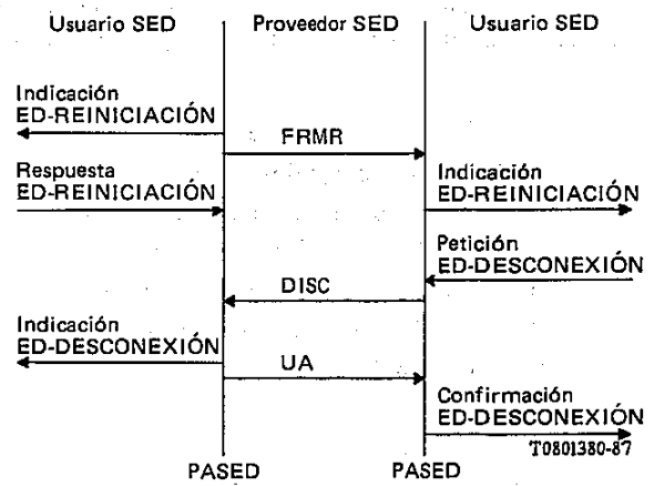
FIGURA D-8/T.70 Reiniciación no aceptada por el receptor de FRMR
