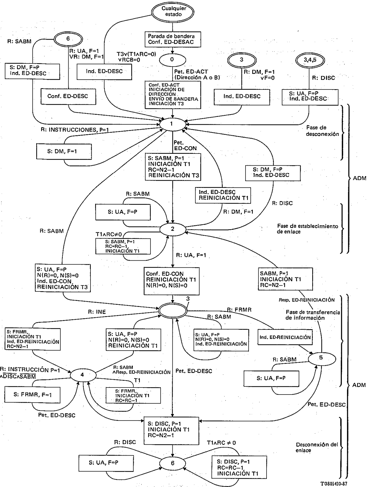
FIGURA D-11/T.70 Diagrama de transición de estados HDLC (control del enlace de datos)
