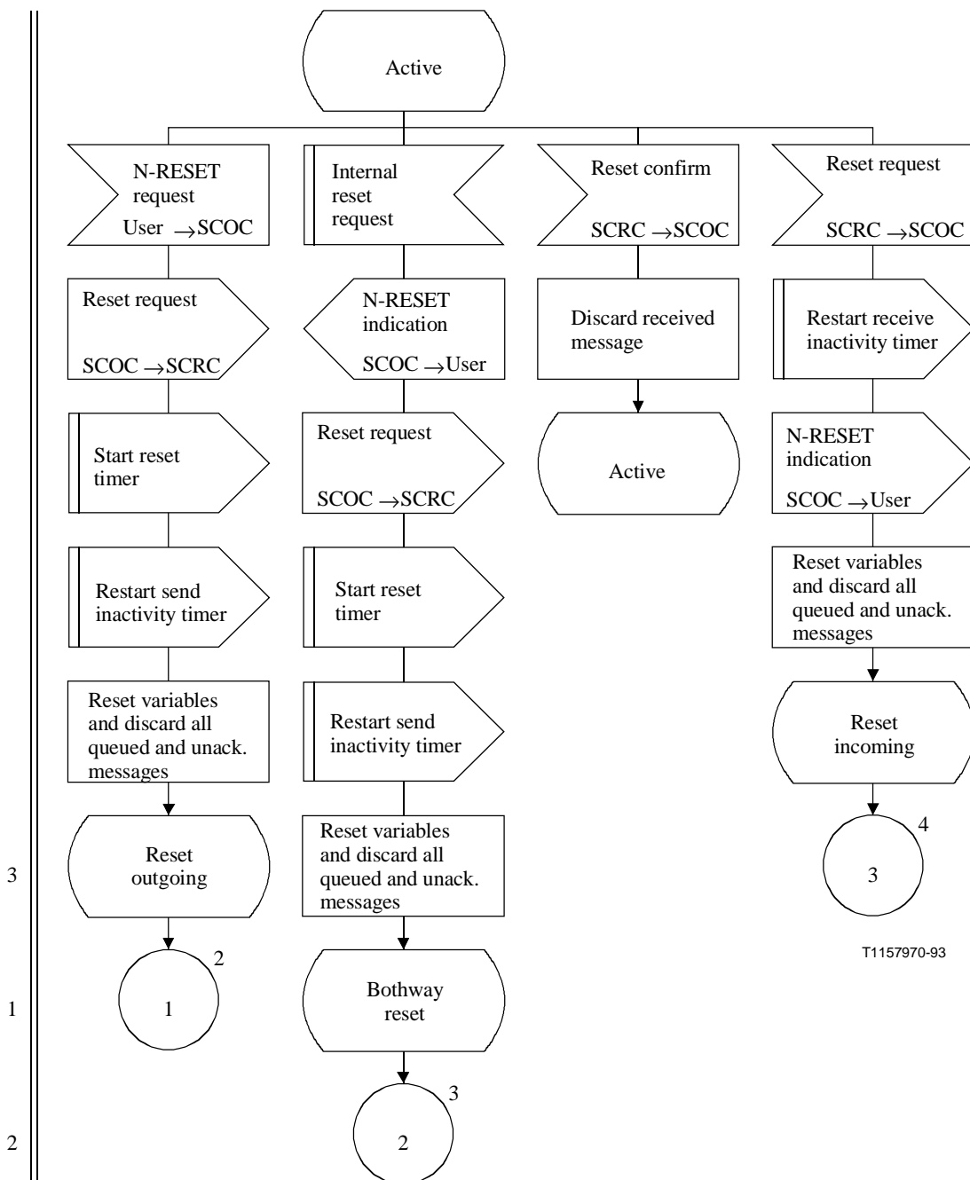
Figura C.6/Q.714 (hoja 1 de 4) – Procedimientos de reiniciación en los nodos de origen y de destino para el control orientado a la conexión de la SCCP (SCOC)
