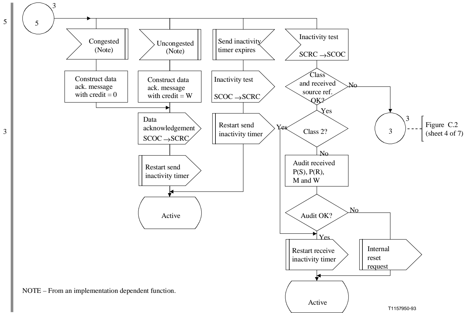
Figura C.4/Q.714 (hoja 4 de 4) – Procedimientos de transferencia de datos en los nodos de origen y de destino para el control orientado a la conexión de la SCCP (SCOC)
