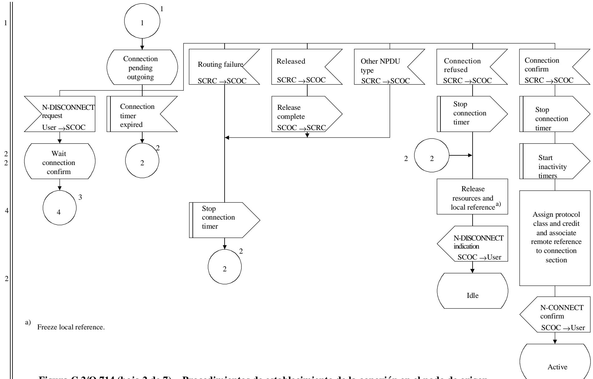
Figura C.2/Q.714 (hoja 2 de 7) – Procedimientos de establecimiento de la conexión en el nodo de origen para el control con conexión de la SCCP (SCOC)
