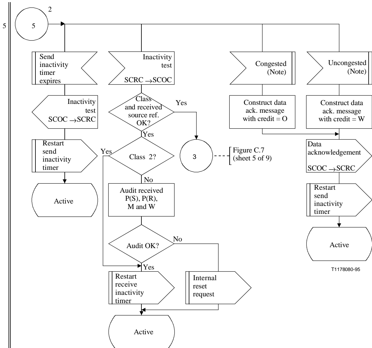
Figura C.8/Q.714 (hoja 4 de 4) – Procedimientos de transferencia de datos en un nodo intermedio para el control orientado a la conexión de la SCCP (SCOC)
