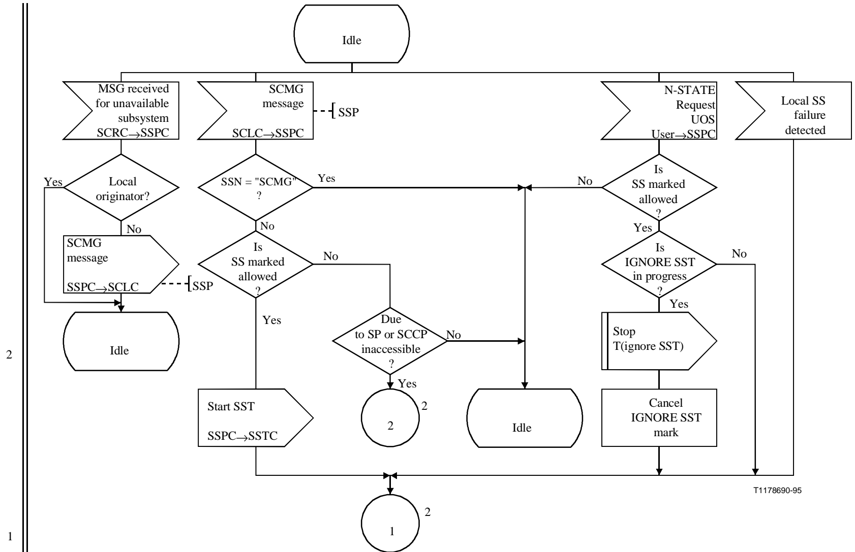
Figura D.5/Q.714 (hoja 1 de 2) – Control de subsistema prohibido (SSPC)
