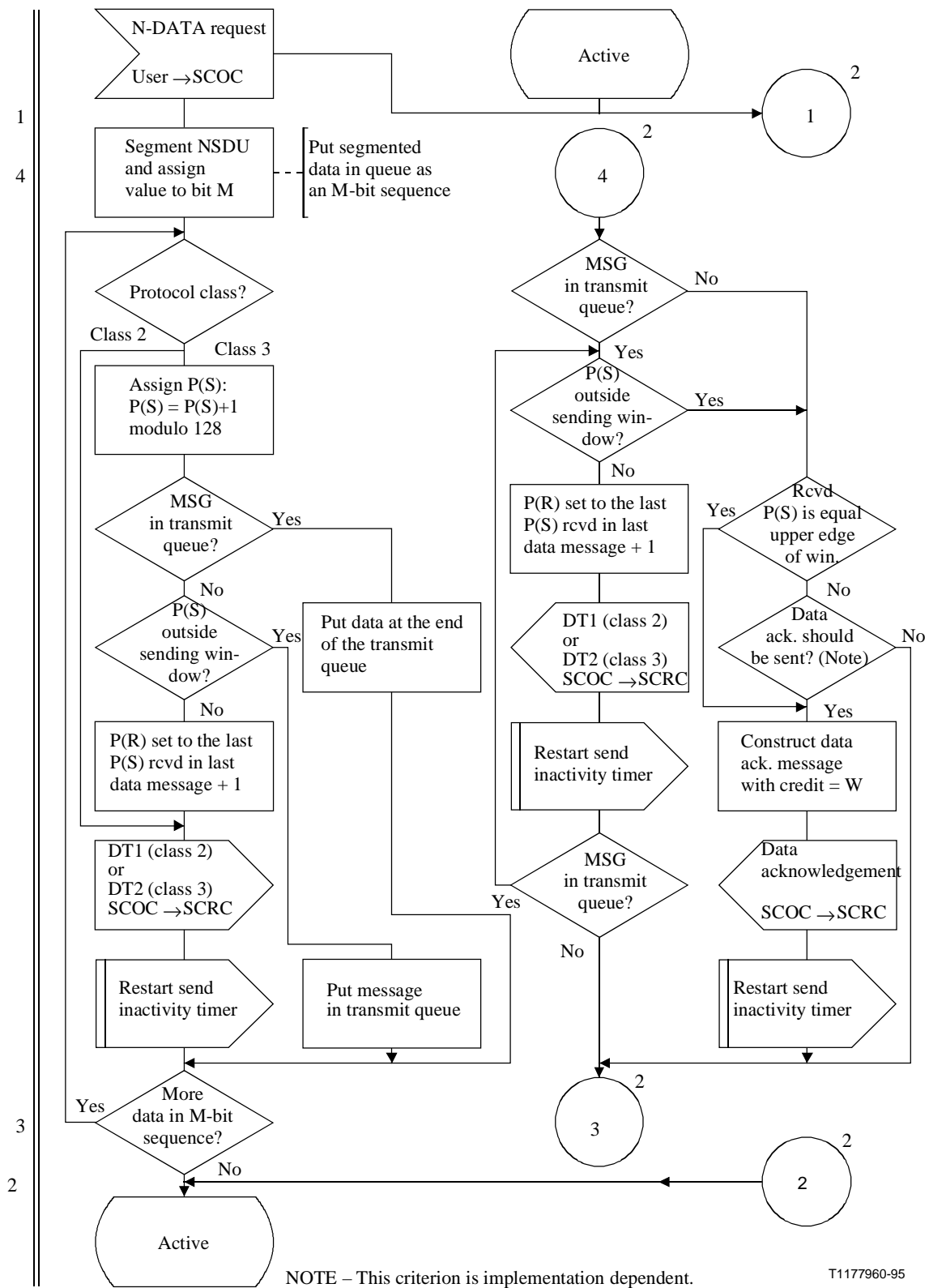
Figura C.4/Q.714 (hoja 1 de 4) – Procedimientos de transferencia de datos en los nodos de origen y de destino para el control orientado a la conexión de la SCCP (SCOC)
