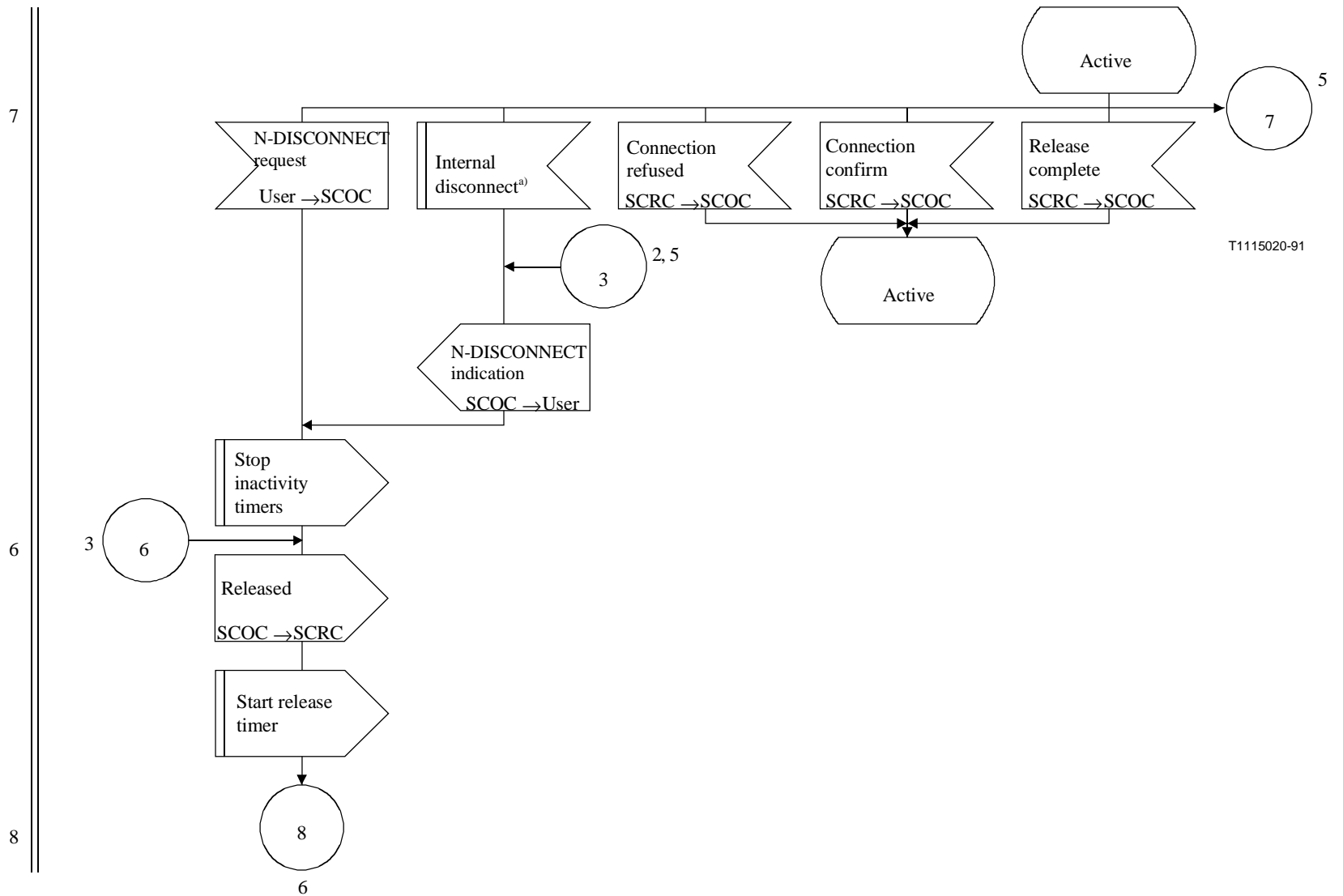
Figura C.2/Q.714 (hoja 4 de 7) – Procedimientos de liberación de la conexión en el nodo de origen para el control orientado a la conexión de la SCCP (SCOC)
