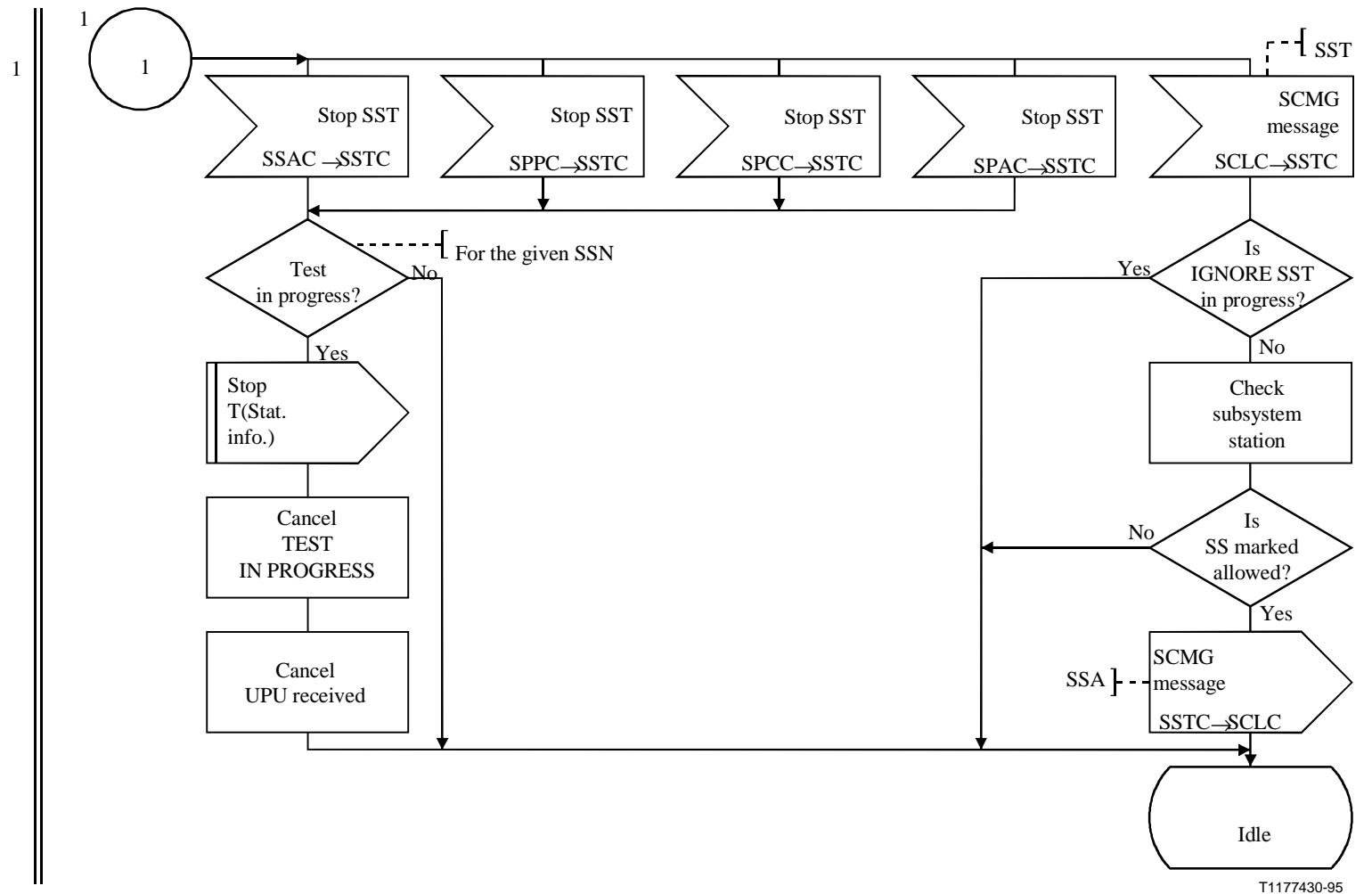
Figura D.7/Q.714 (hoja 2 de 2) – Control de prueba de estado de subsistema (SSTC)
