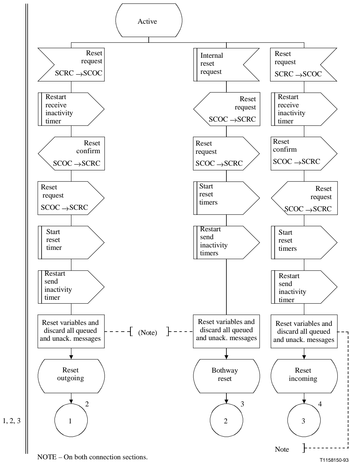
Figura C.10/Q.714 (hoja 1 de 4) – Procedimientos de reiniciación en un nodo intermedio para el control orientado a la conexión de la SCCP (SCOC)
