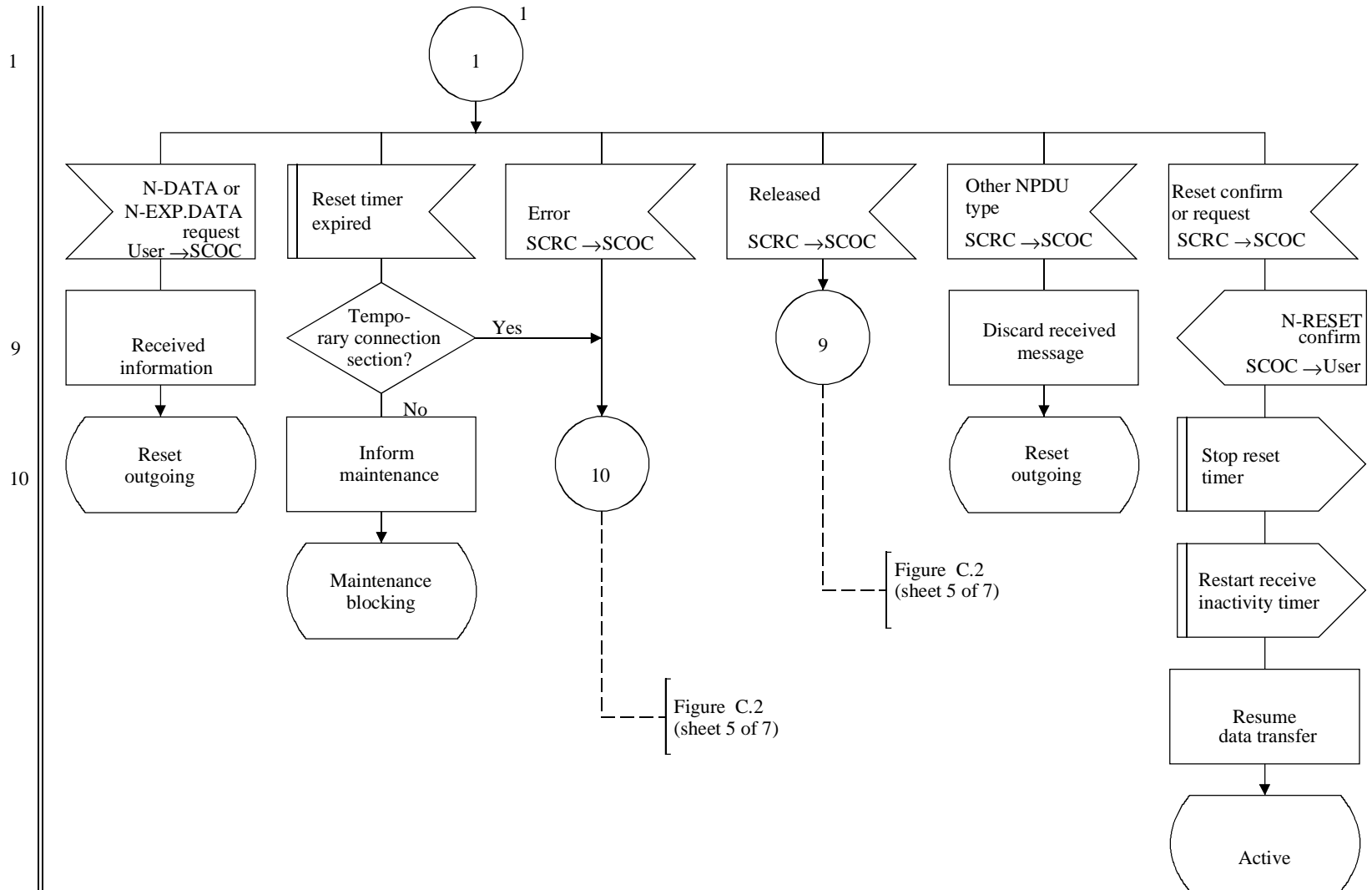
Figura C.6/Q.714 (hoja 2 de 4) – Procedimientos de reiniciación en los nodos de origen y de destino para el control orientado a la conexión de la SCCP (SCOC)
