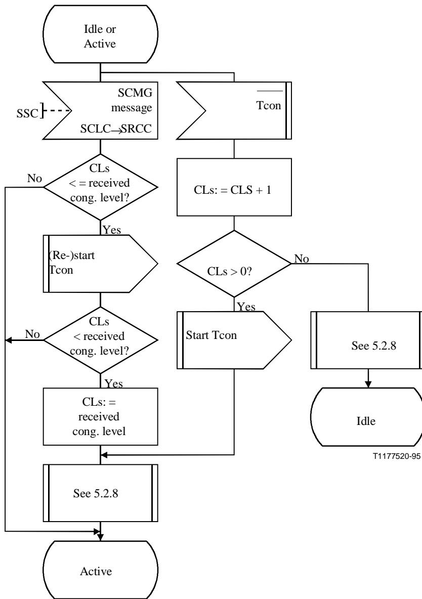
Figura D.13/Q.714 (hoja 1 de 2) – Control de la congestión de la SCCP y nodal distantes (SRCC)
