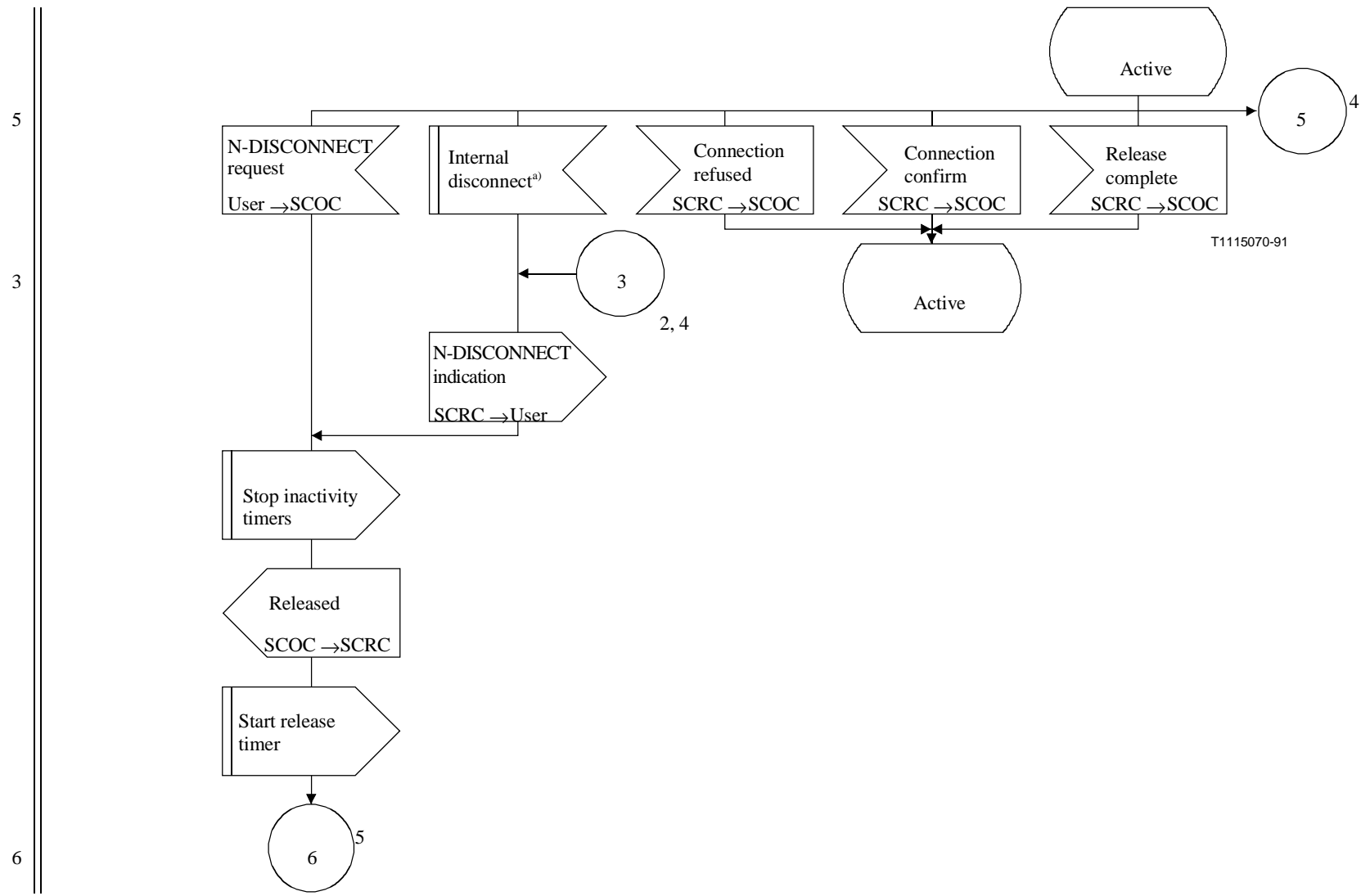
Figura C.3/Q.714 (hoja 3 de 6) – Procedimientos de liberación de la conexión en el nodo de destino para el control orientado a la conexión de la SCCP (SCOC)
