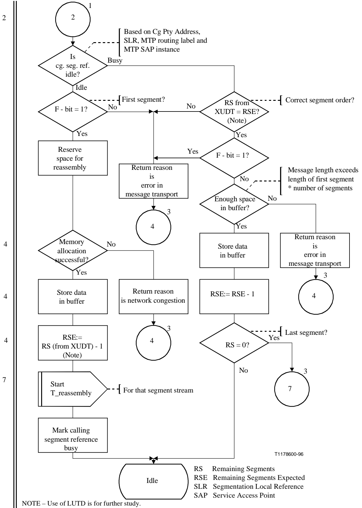
Figura C.12/Q.714 (hoja 2 de 9) – Control sin conexión de la SCCP (SCLC)
