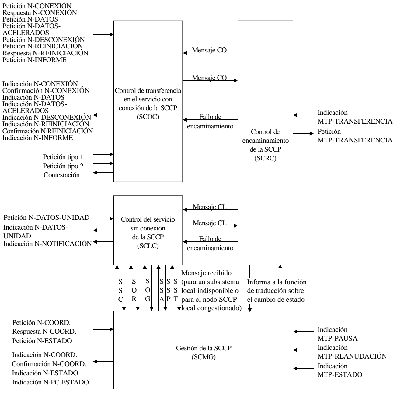
Figura 1/Q.714 – Estructura básica de la SCCP
