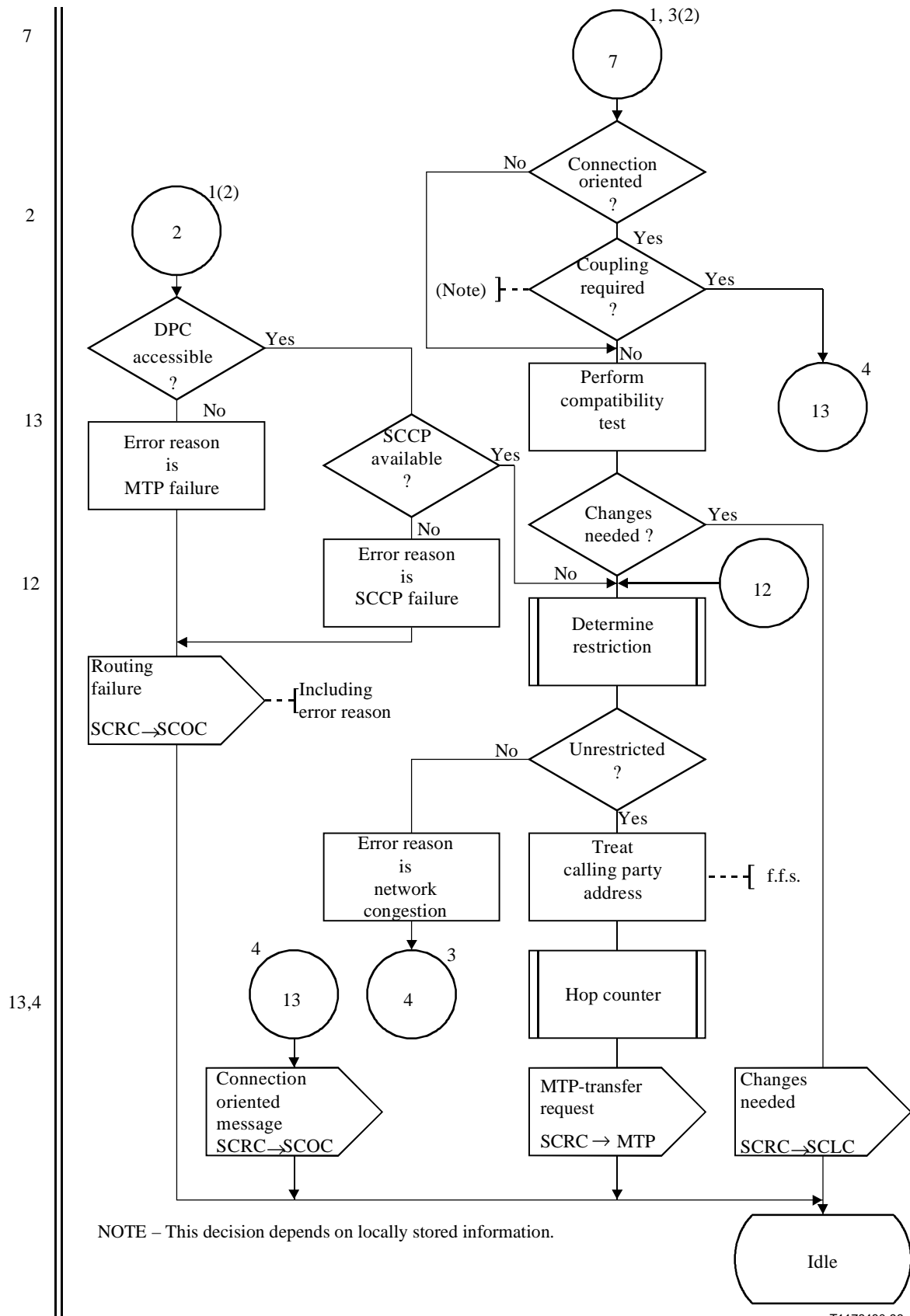
Figura C.1/Q.714 (hoja 4 de 11) – Procedimientos de control de encaminamiento de la SCCP (SCRC)
