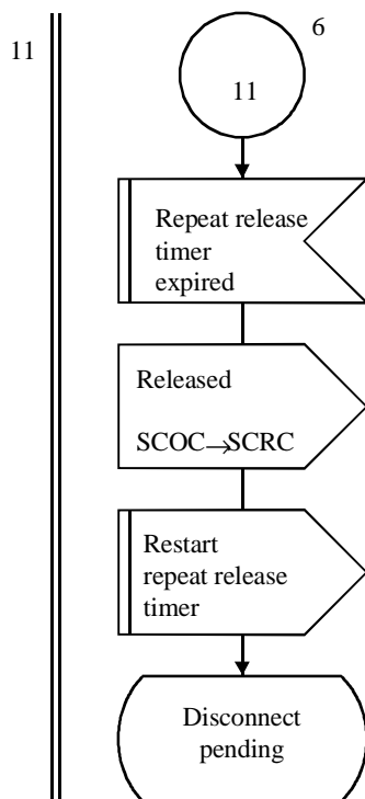
Figura C.2/Q.714 (hoja 7 de 7) – Procedimientos de establecimiento de la conexión en el nodo de origen para el control orientado a la conexión de la SCCP (SCOC)
