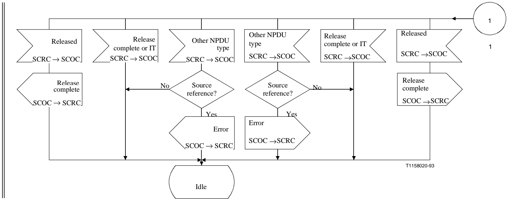
Figura C.7/Q.714 (hoja 2 de 9) – Procedimientos de establecimiento de la conexión en un nodo intermedio para el control orientado a la conexión de la SCCP (SCOC)
