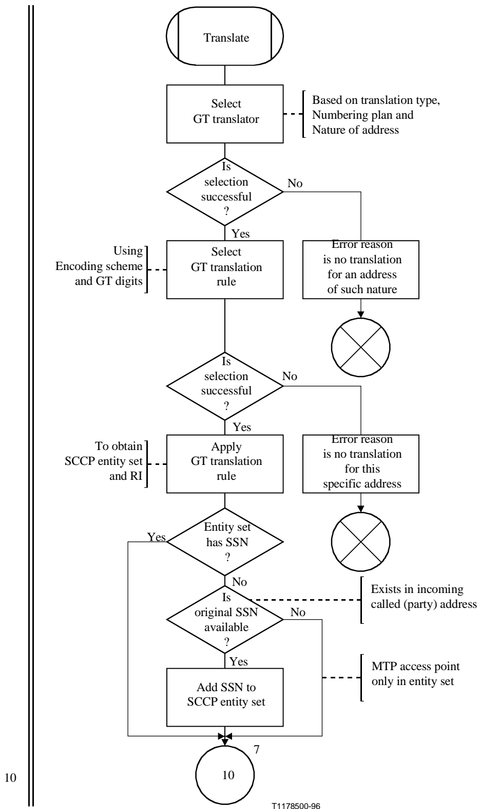
Figura C.1/Q.714 (hoja 6 de 11) – Procedimientos de control de encaminamiento de la SCCP (SCRC)
