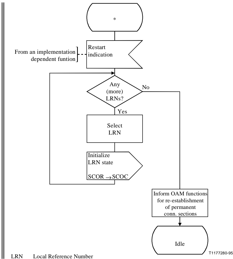
Figura C.13/Q.714 – Control de re arranque para el control orientado a la conexión de la SCCP (SCOR)
