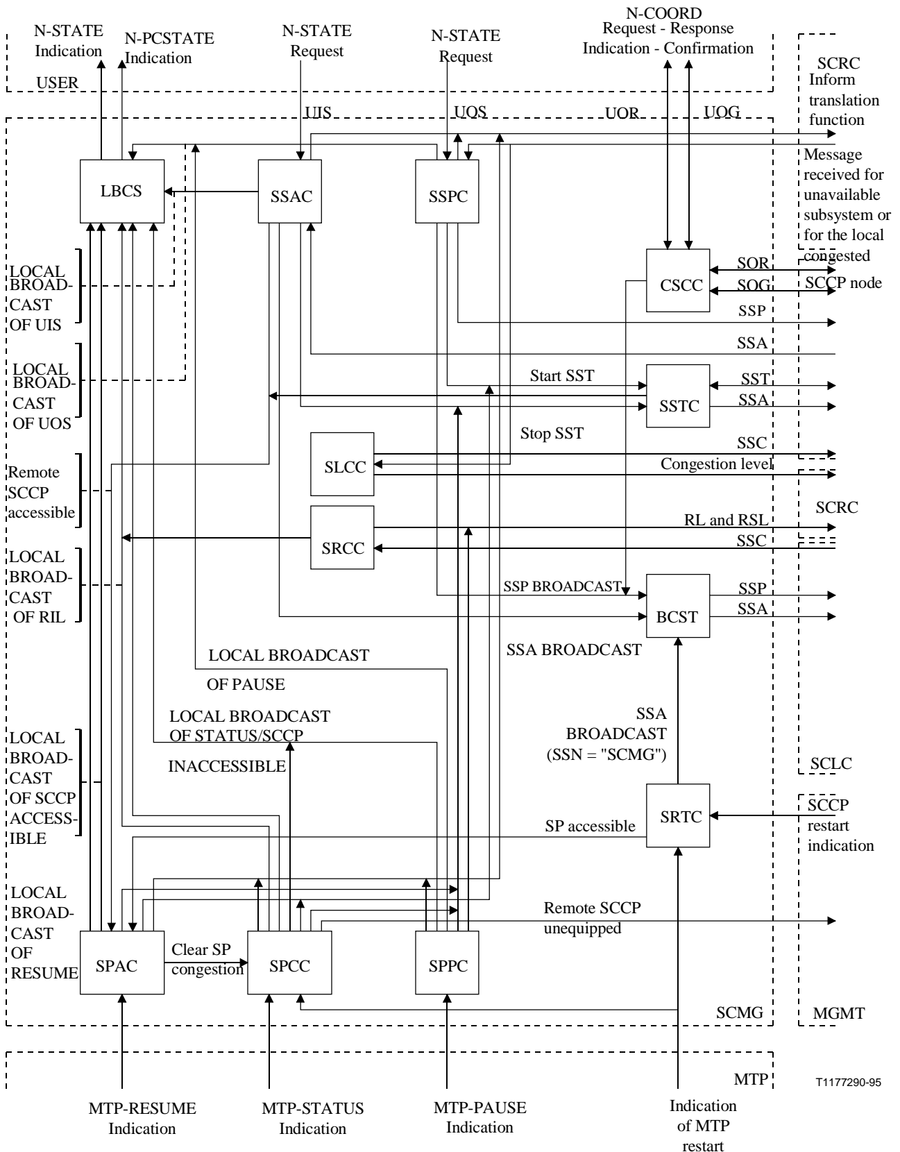
Figura D.1/Q.714 – Visión de conjunto de la función de gestión de la SCCP (SCMG)
