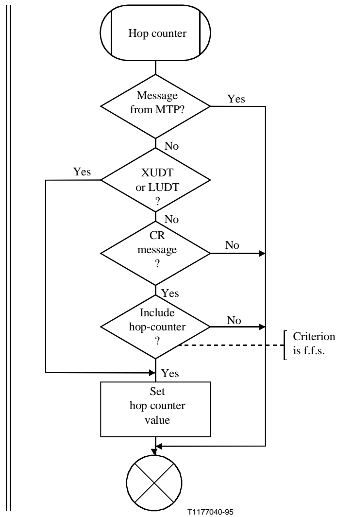
Figura C.1/Q.714 (hoja 8 de 11) – Procedimientos de control de encaminamiento de la SCCP (SCRC)
