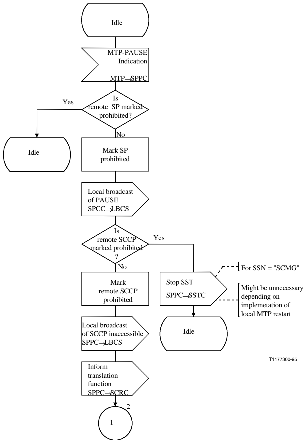
Figura D.2/Q.714 (hoja 1 de 2) – Control de punto de señalización prohibido (SPPC)
