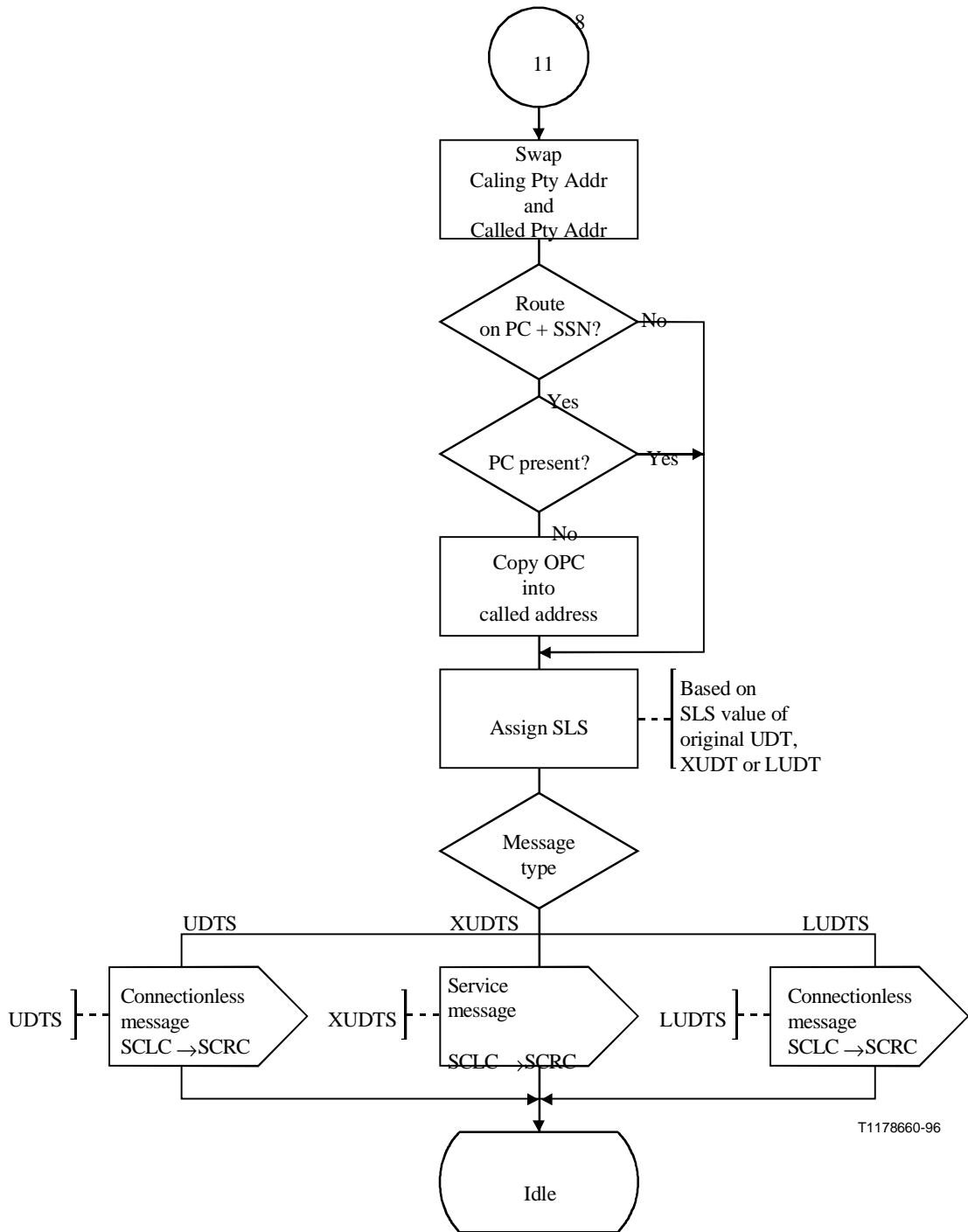
Figura C.12/Q.714 (hoja 9 de 9) – Control sin conexión de la SCCP (SCLC)
