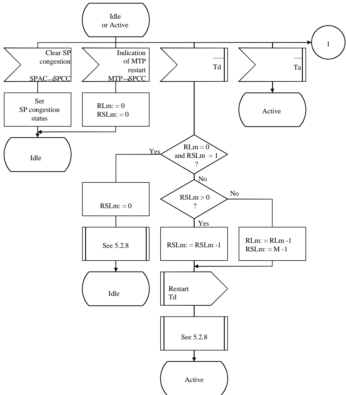
Figura D.4/Q.714 (hoja 1 de 4) – Control de punto de señalización congestionado (SPCC)
