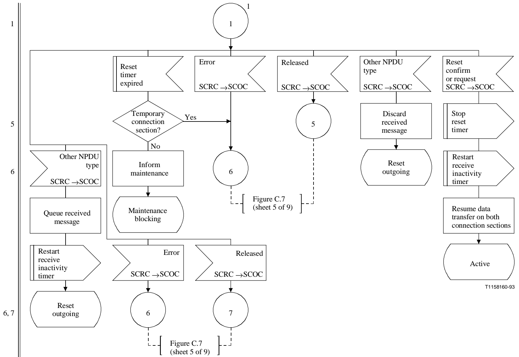
Figura C.10/Q.714 (hoja 2 de 4) – Procedimientos de reiniciación en un nodo intermedio para el control orientado a la conexión de la SCCP (SCOC)
