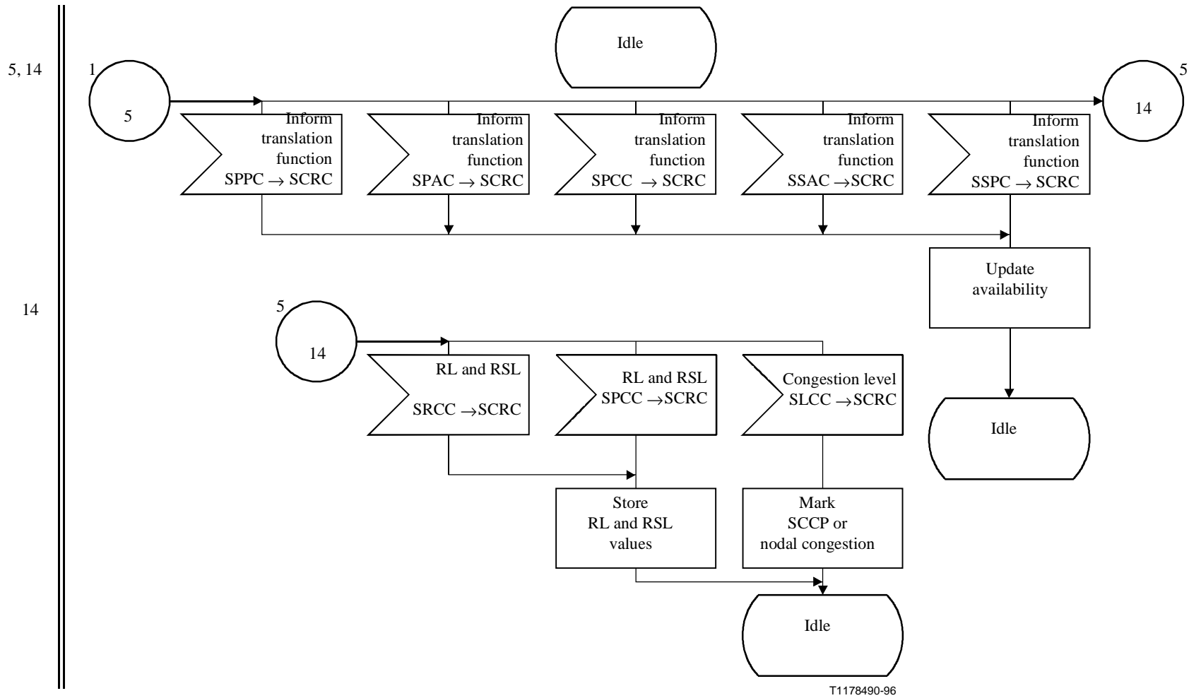
Figura C.1/Q.714 (hoja 5 de 11) – Procedimientos de control de encaminamiento de la SCCP (SCRC)
