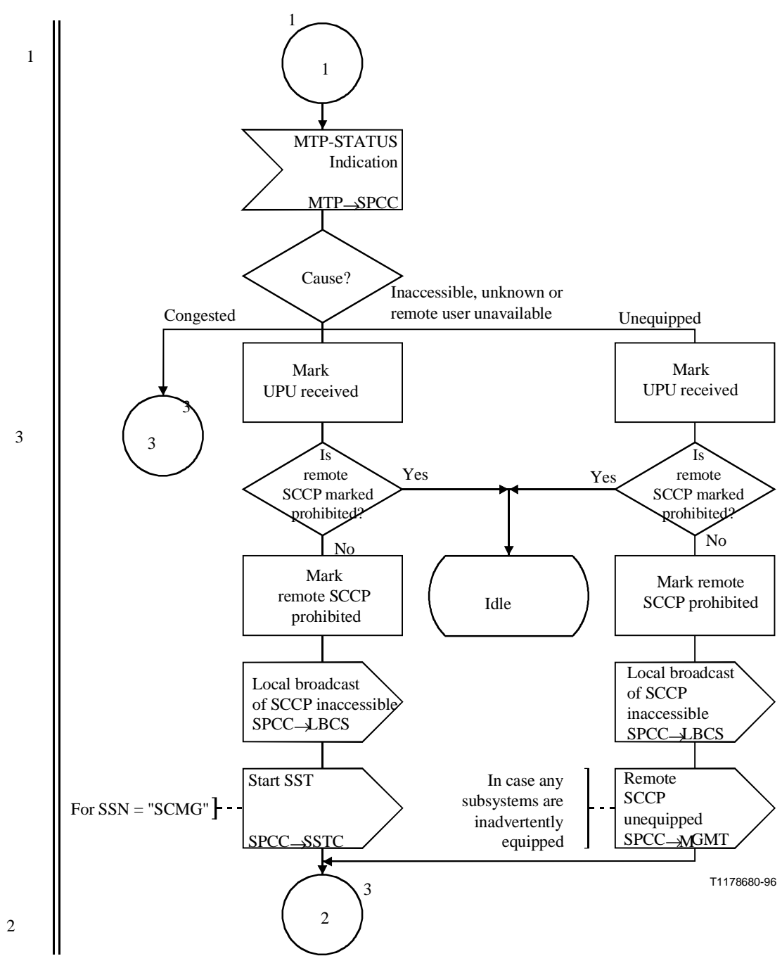
Figura D.4/Q.714 (hoja 2 de 4) – Control de punto de señalización congestionado (SPCC)
