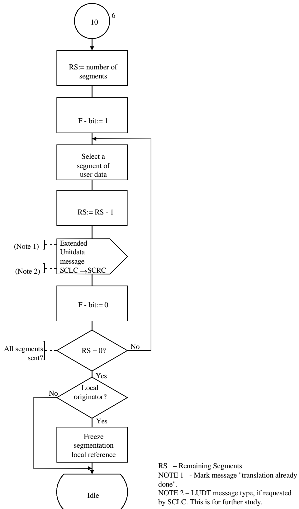
Figura C.12/Q.714 (hoja 7 de 9) – Control sin conexión de la SCCP (SCLC)
