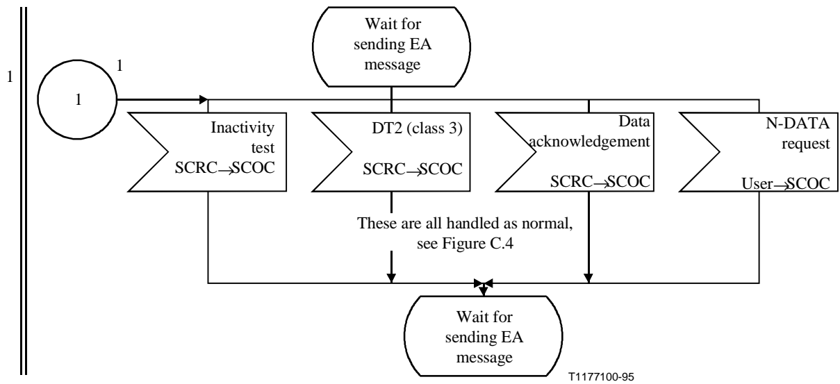
Figura C.5/Q.714 (hoja 2 de 2) – Procedimientos de transferencia de datos acelerados en los nodos de origen y de destino para el control orientado a la conexión de la SCCP (SCOC)
