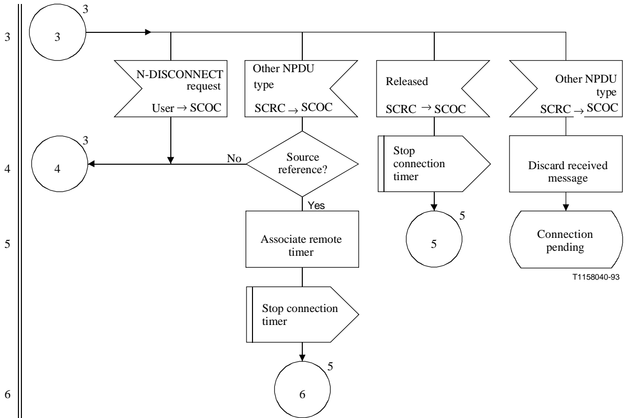
Figura C.7/Q.714 (hoja 4 de 9) – Procedimientos de establecimiento de la conexión en un nodo intermedio para el control orientado a la conexión de la SCCP (SCOC)
