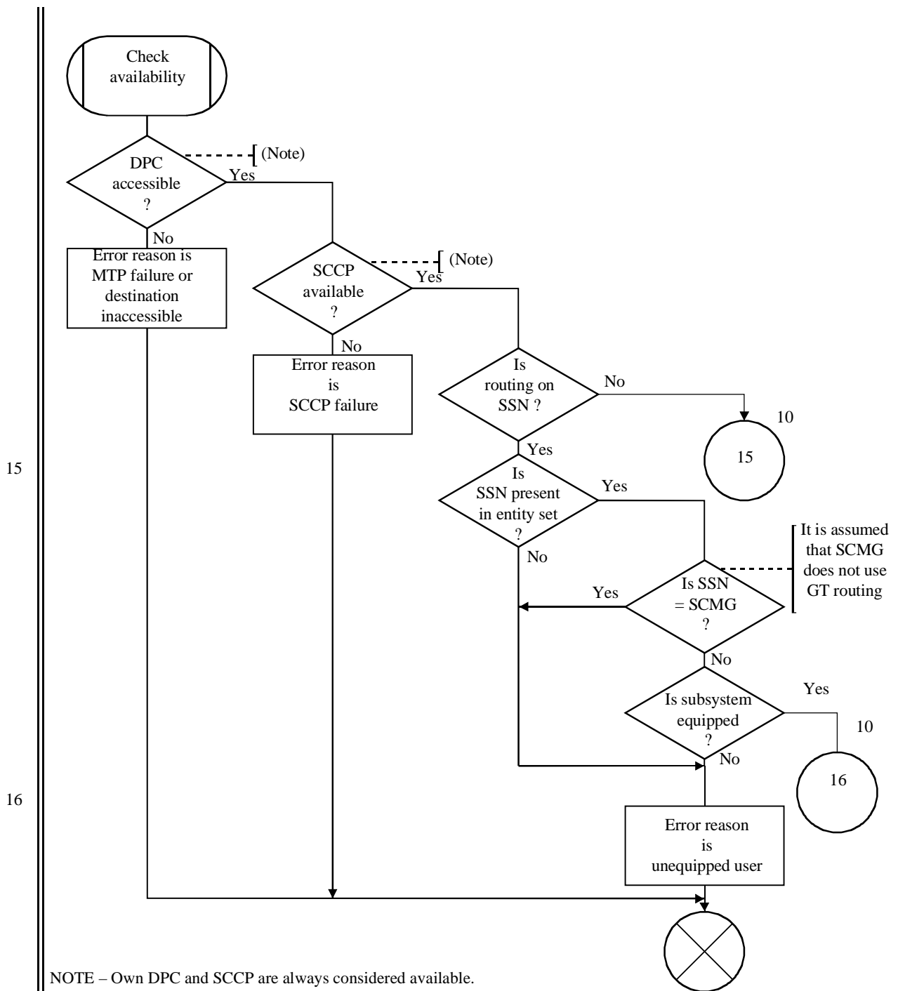
Figura C.1/Q.714 (hoja 9 de 11) – Procedimientos de control de encaminamiento de la SCCP (SCRC)
