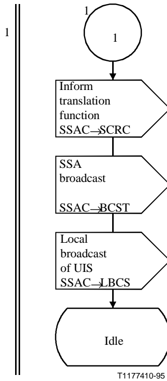
Figura D.6/Q.714 (hoja 2 de 2) – Control de subsistema autorizado (SSAC)
