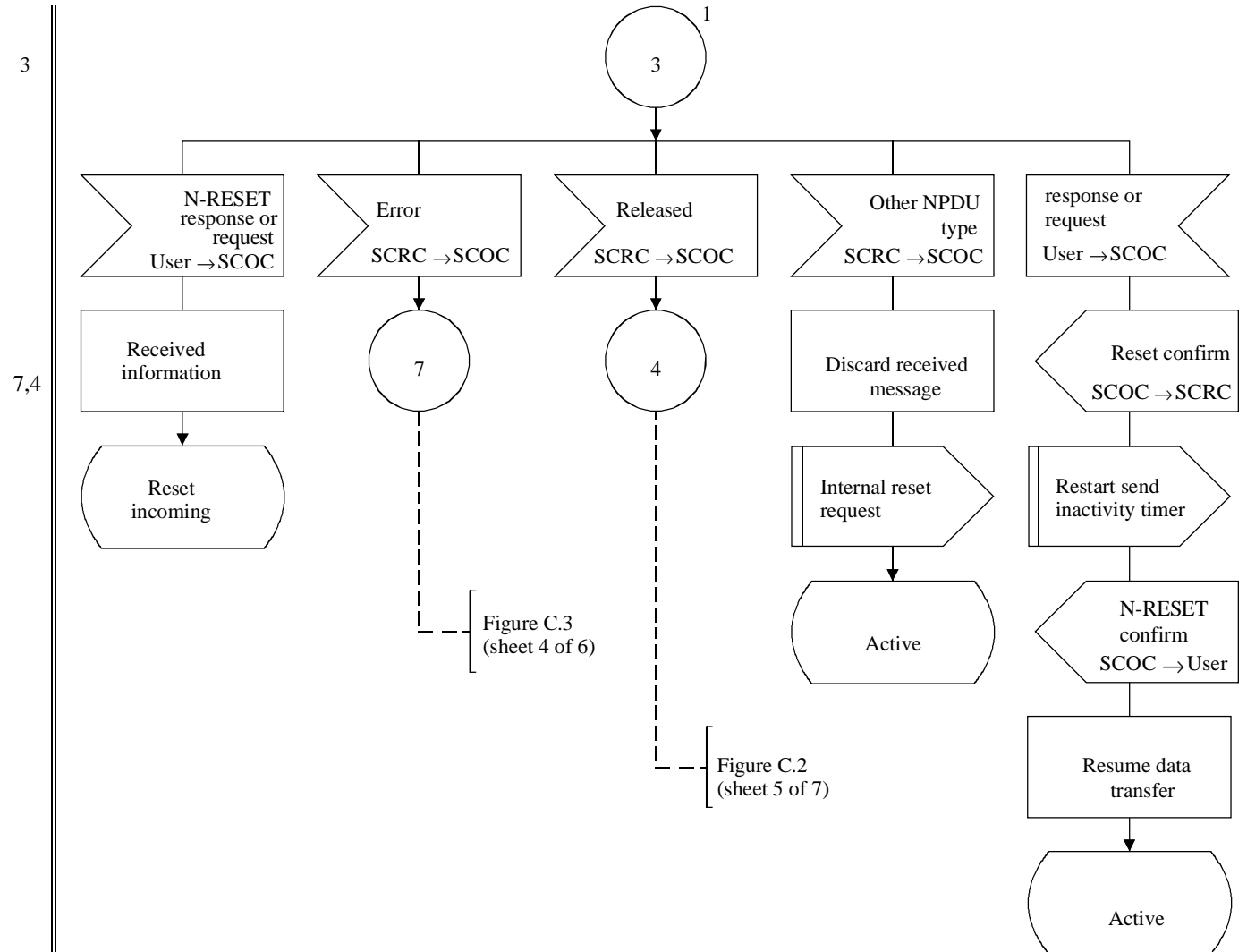
Figura C.6/Q.714 (hoja 4 de 4) – Procedimientos de reiniciación en los nodos de origen y de destino para el control orientado a la conexión de la SCCP (SCOC)
