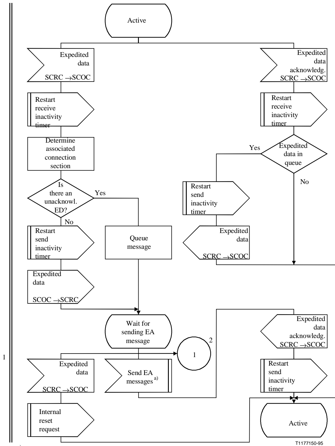
Figura C.9/Q.714 (hoja 1 de 2) – Procedimientos de transferencia de datos en un nodo intermedio para el control orientado a la conexión de la SCCP (SCOC)
