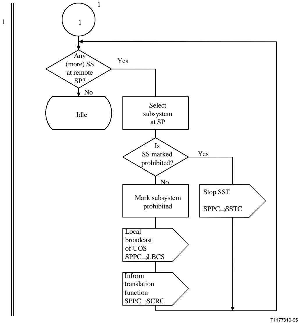
Figura D.2/Q.714 (hoja 2 de 2) – Control de punto de señalización prohibido (SPPC)
