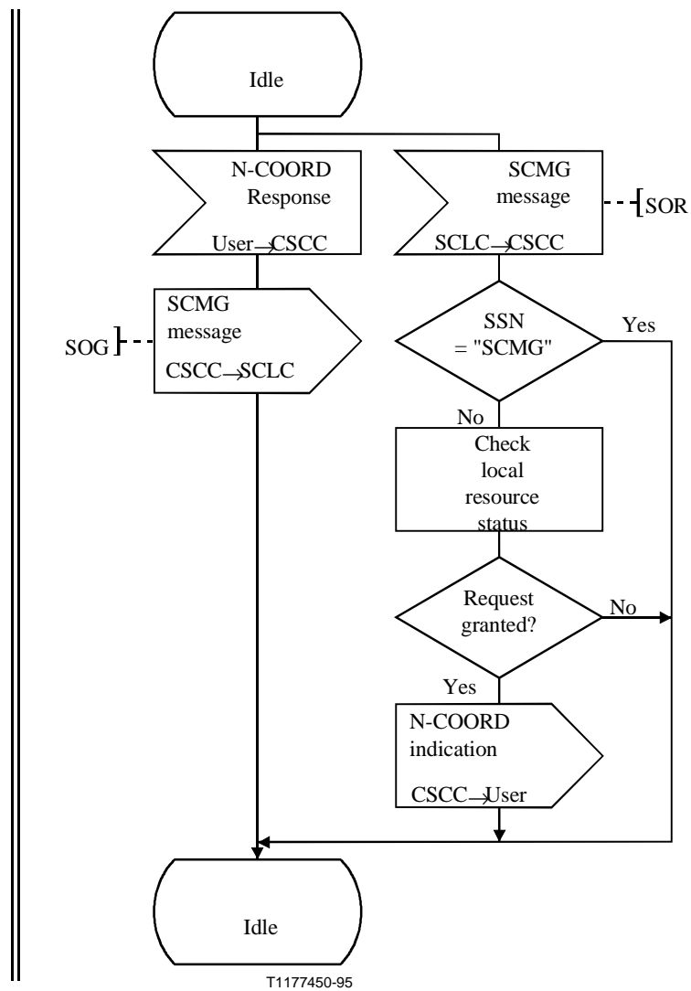
Figura D.8/Q.714 (hoja 2 de 2) – Control de cambio de estado coordinado (CSCC) en el nodo solicitante
