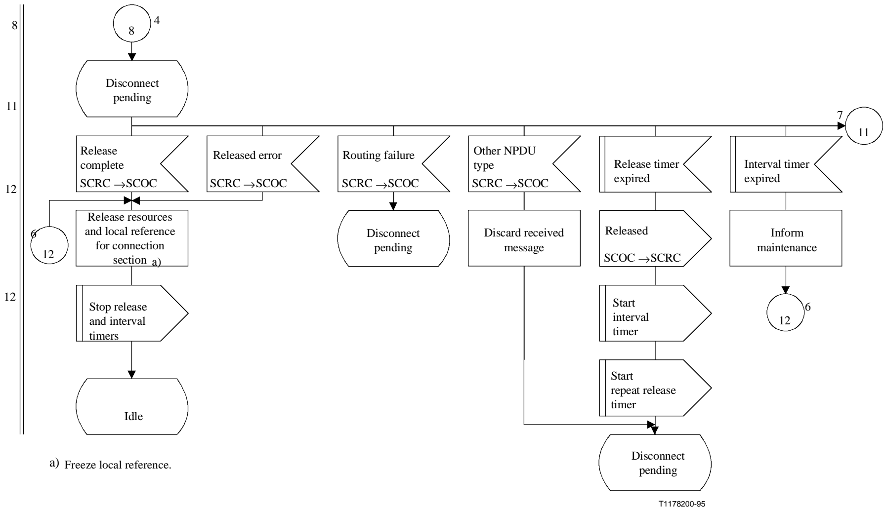
Figura C.2/Q.714 (hoja 6 de 7) – Procedimientos de liberación de la conexión en el nodo de origen para el control orientado a la conexión de la SCCP (SCOC)
