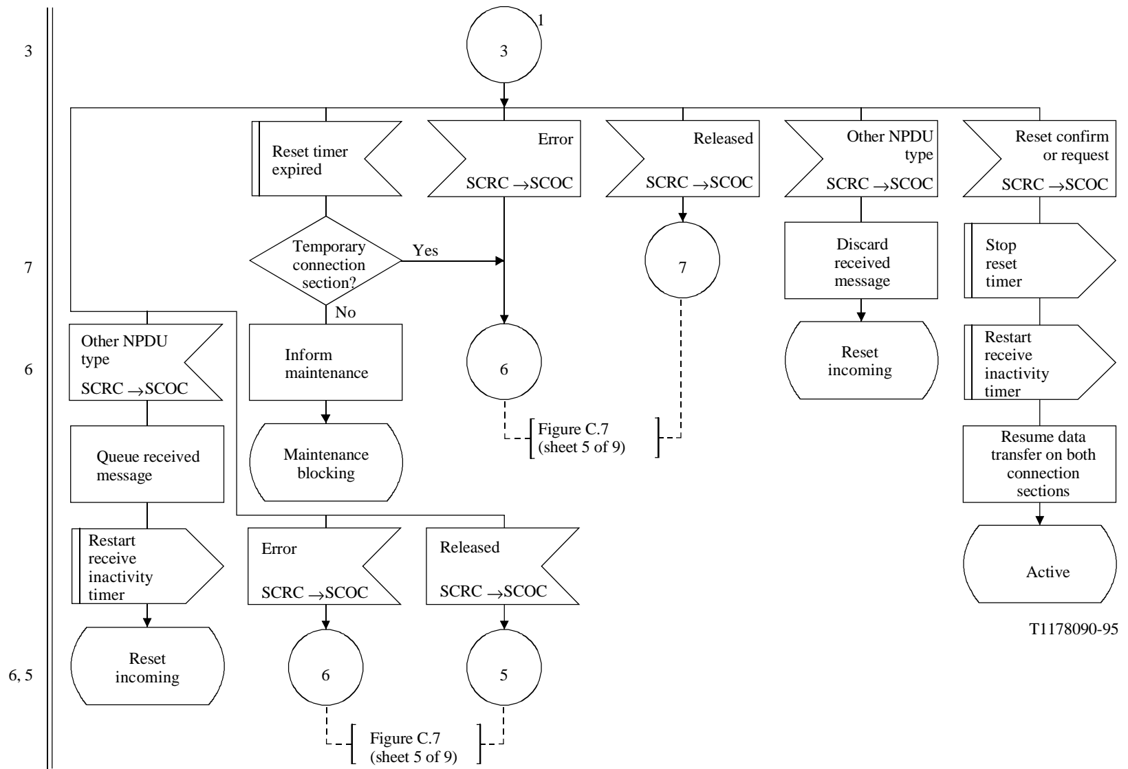
Figura C.10/Q.714 (hoja 4 de 4) – Procedimientos de reiniciación en un nodo intermedio para el control orientado a la conexión de la SCCP (SCOC)
