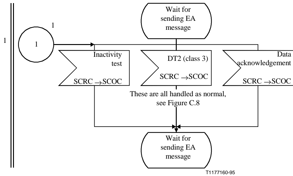
Figura C.9/Q.714 (hoja 2 de 2) – Procedimientos de transferencia de datos en un nodo intermedio para el control orientado a la conexión de la SCCP (SCOC)
