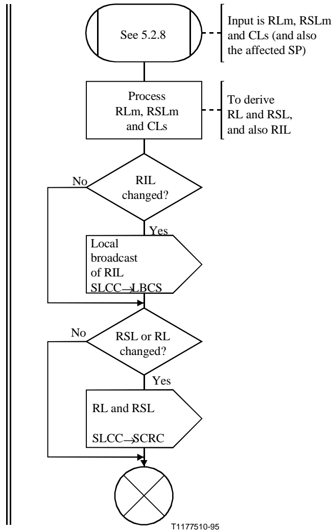
Figura D.12/Q.714 (hoja 2 de 2) – Control de la congestión de la SCCP y nodal locales (SLCC)
