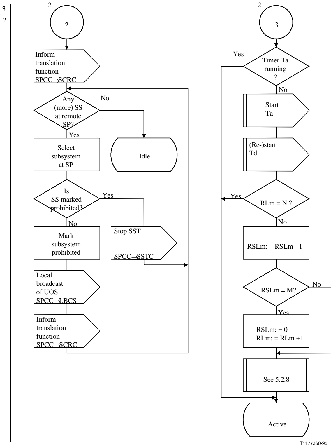
Figura D.4/Q.714 (hoja 3 de 4) – Control de punto de señalización congestionado (SPCC)
