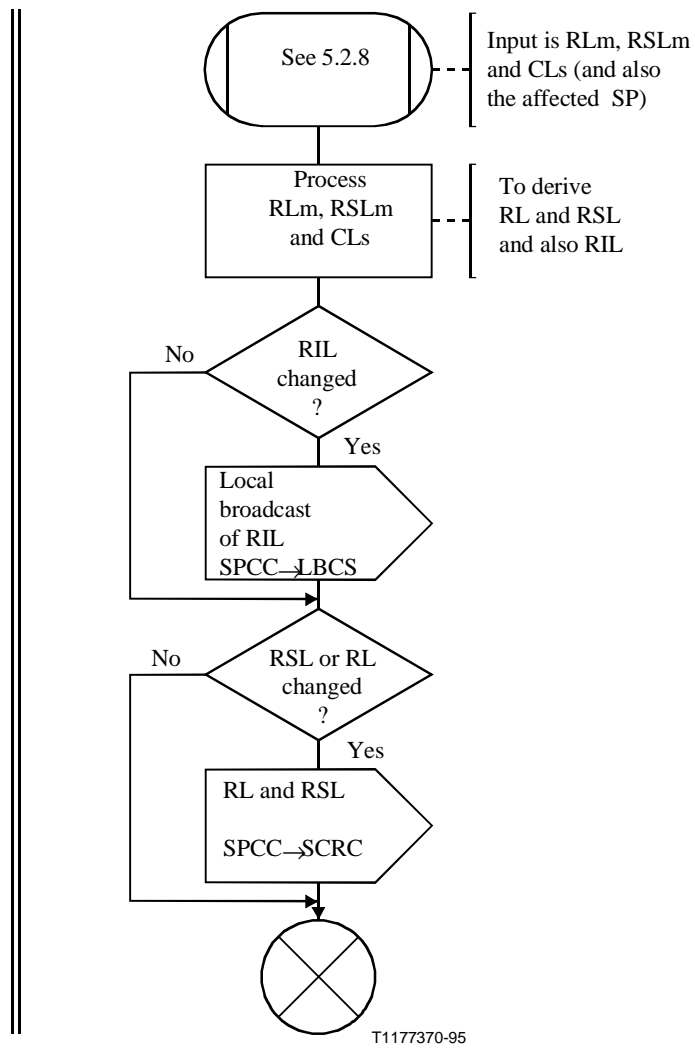
Figura D.4/Q.714 (hoja 4 de 4) – Control de punto de señalización congestionado (SPCC)
