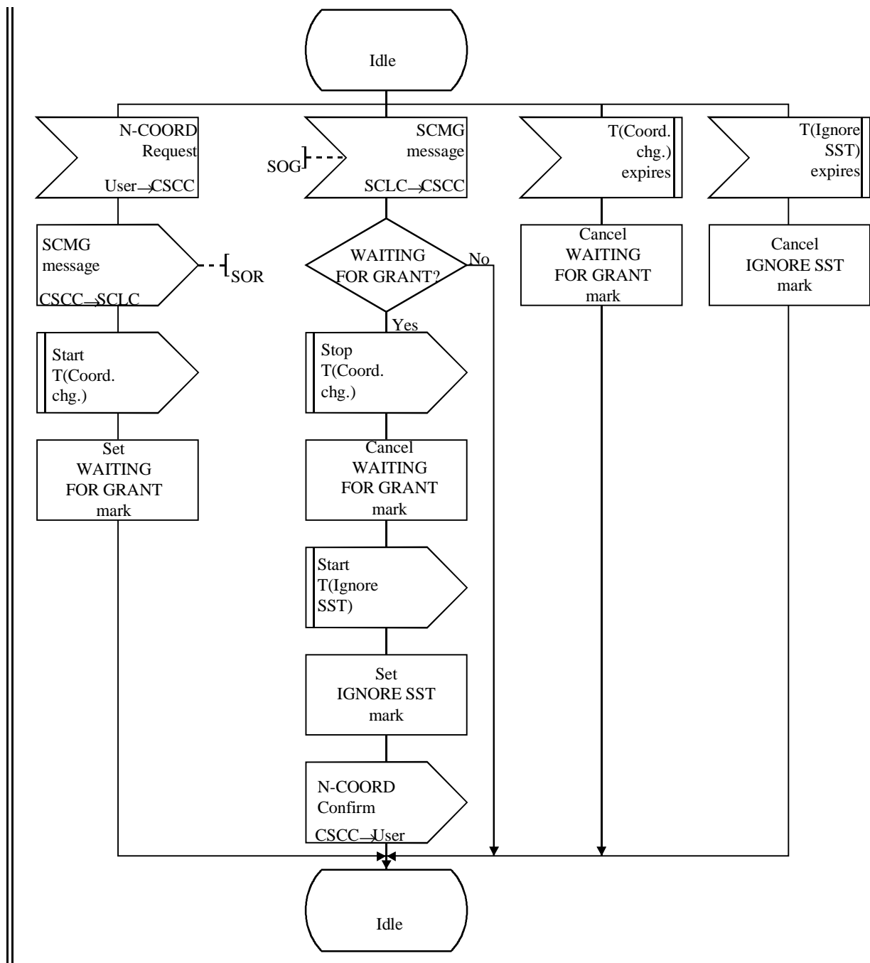
Figura D.8/Q.714 (hoja 1 de 2) – Control de cambio de estado coordinado (CSCC) en el nodo solicitante
