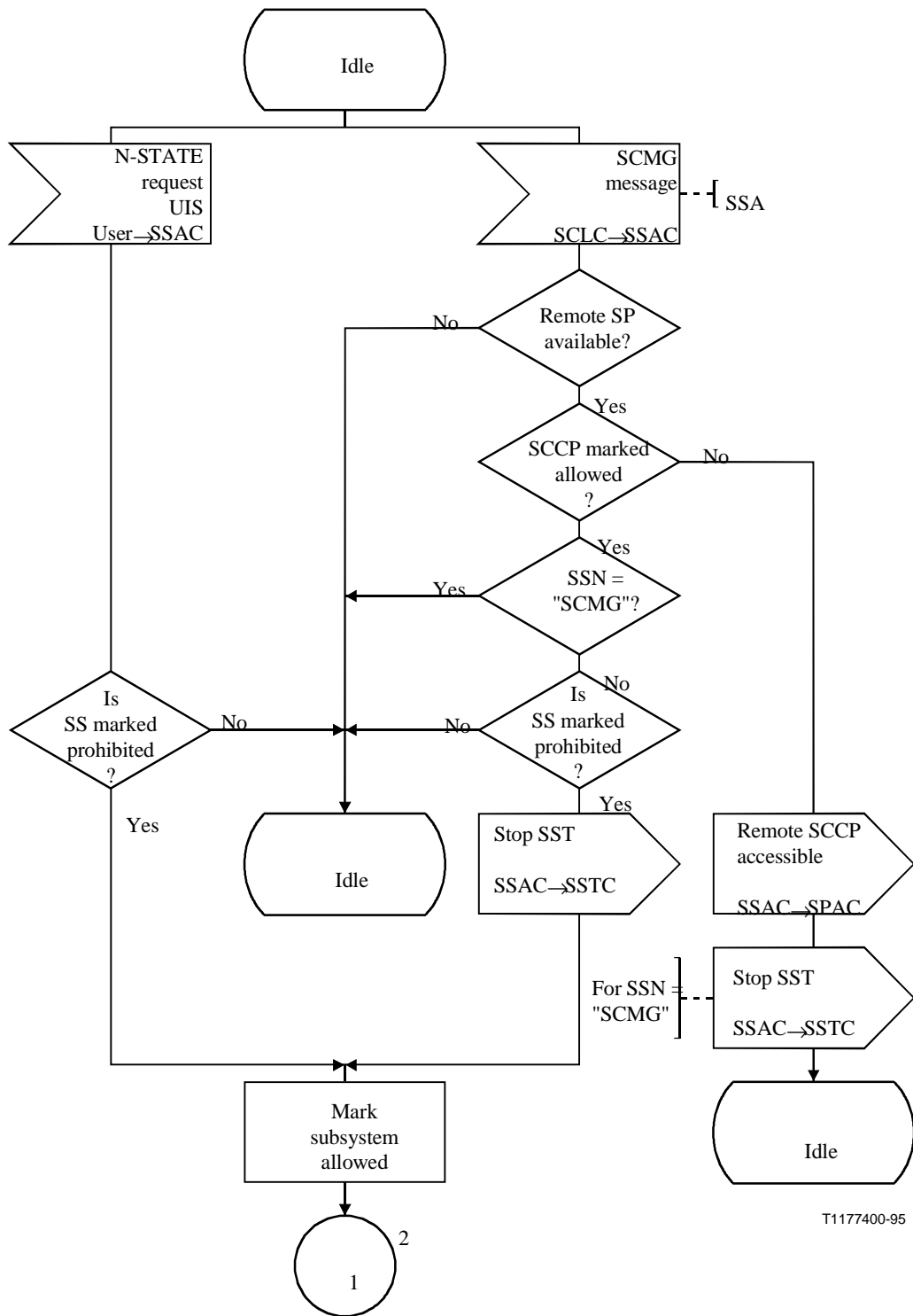
Figura D.6/Q.714 (hoja 1 de 2) – Control de subsistema autorizado (SSAC)
