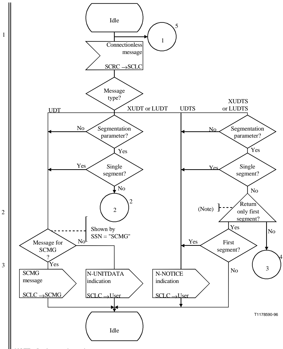
Figura C.12/Q.714 (hoja 1 de 9) – Control sin conexión de la SCCP (SCLC)
