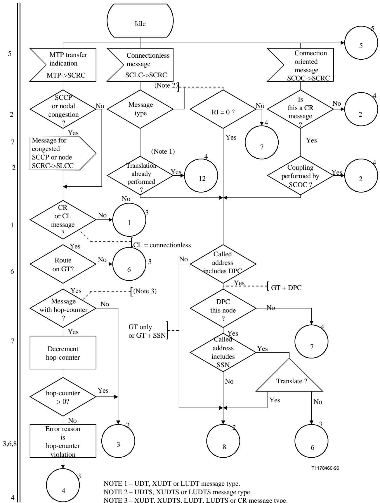
Figura C.1/Q.714 (hoja 1 de 11) – Procedimientos de control de encaminamiento de la SCCP (SCRC)
