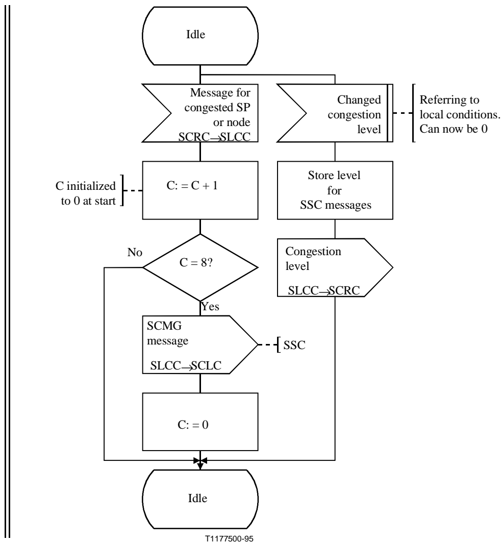
Figura D.12/Q.714 (hoja 1 de 2) – Control de la congestión de la SCCP y nodal locales (SLCC)
