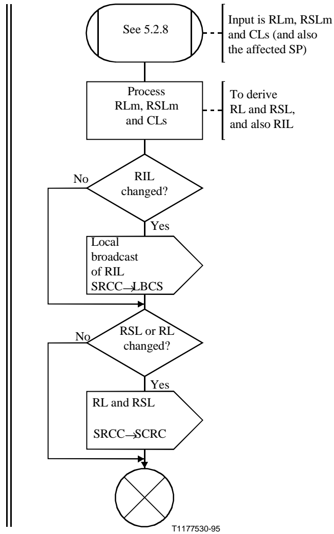
Figura D.13/Q.714 (hoja 2 de 2) – Control de la congestión de la SCCP y nodal distantes (SRCC)
