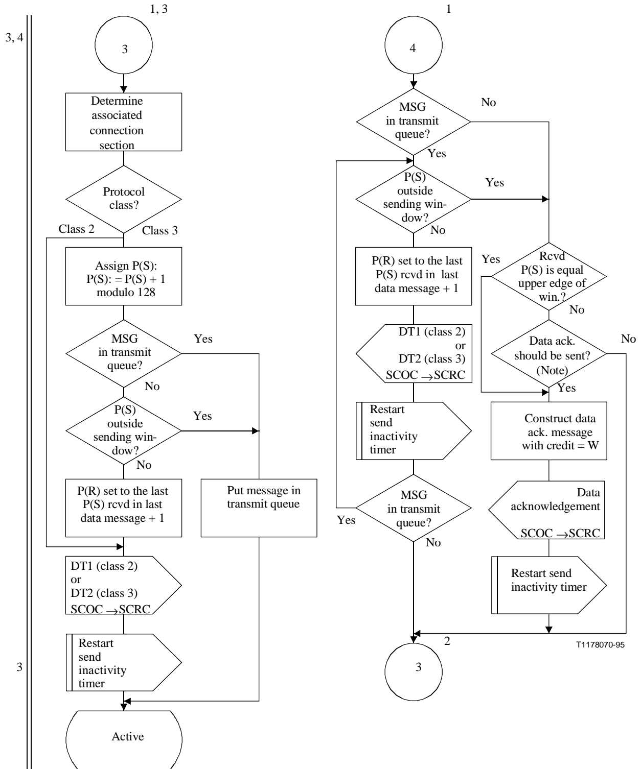
Figura C.8/Q.714 (hoja 3 de 4) – Procedimientos de transferencia de datos en un nodo intermedio para el control orientado a la conexión de la SCCP (SCOC)
