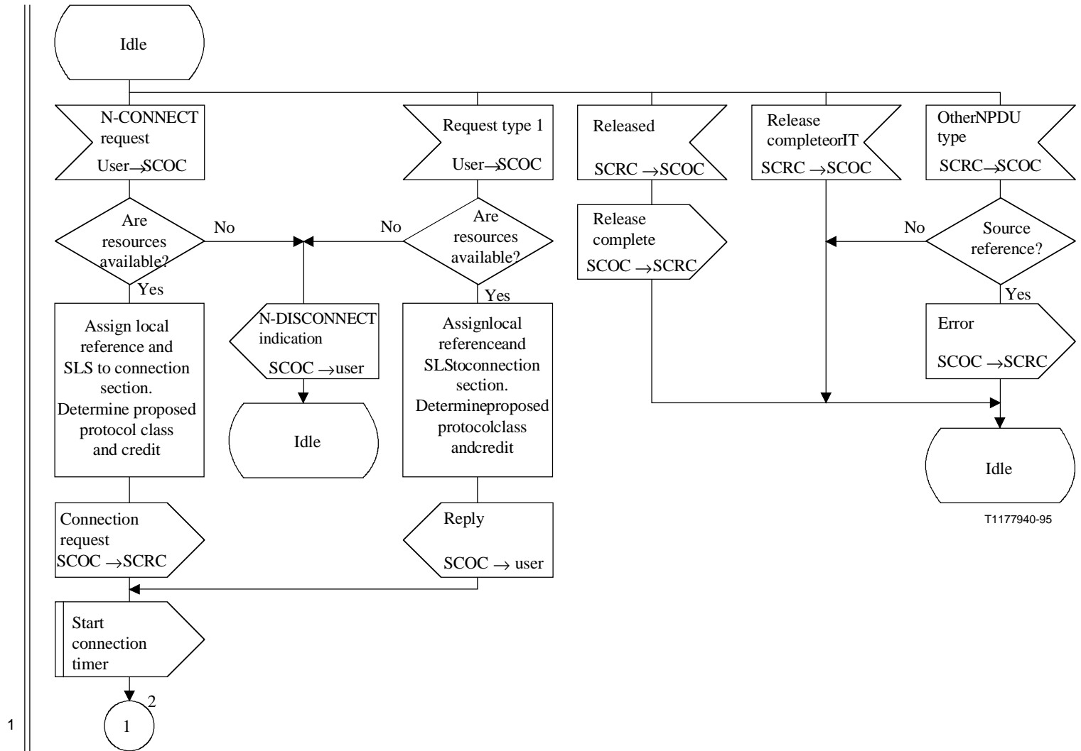
Figura C.2/Q.714 (hoja 1 de 7) – Procedimientos de establecimiento de la conexión en el nodo de origen para el control orientado a la conexión de la SCCP (SCOC)
