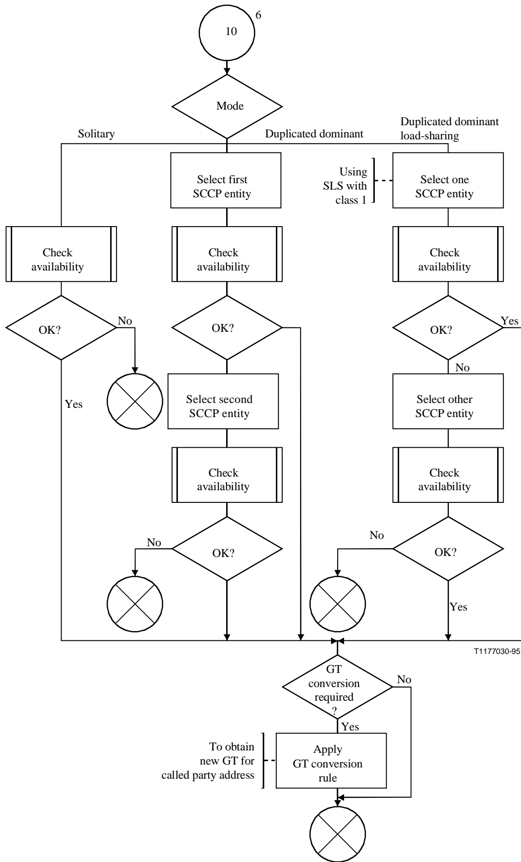
Figura C.1/Q.714 (hoja 7 de 11) – Procedimientos de control de encaminamiento de la SCCP (SCRC)
