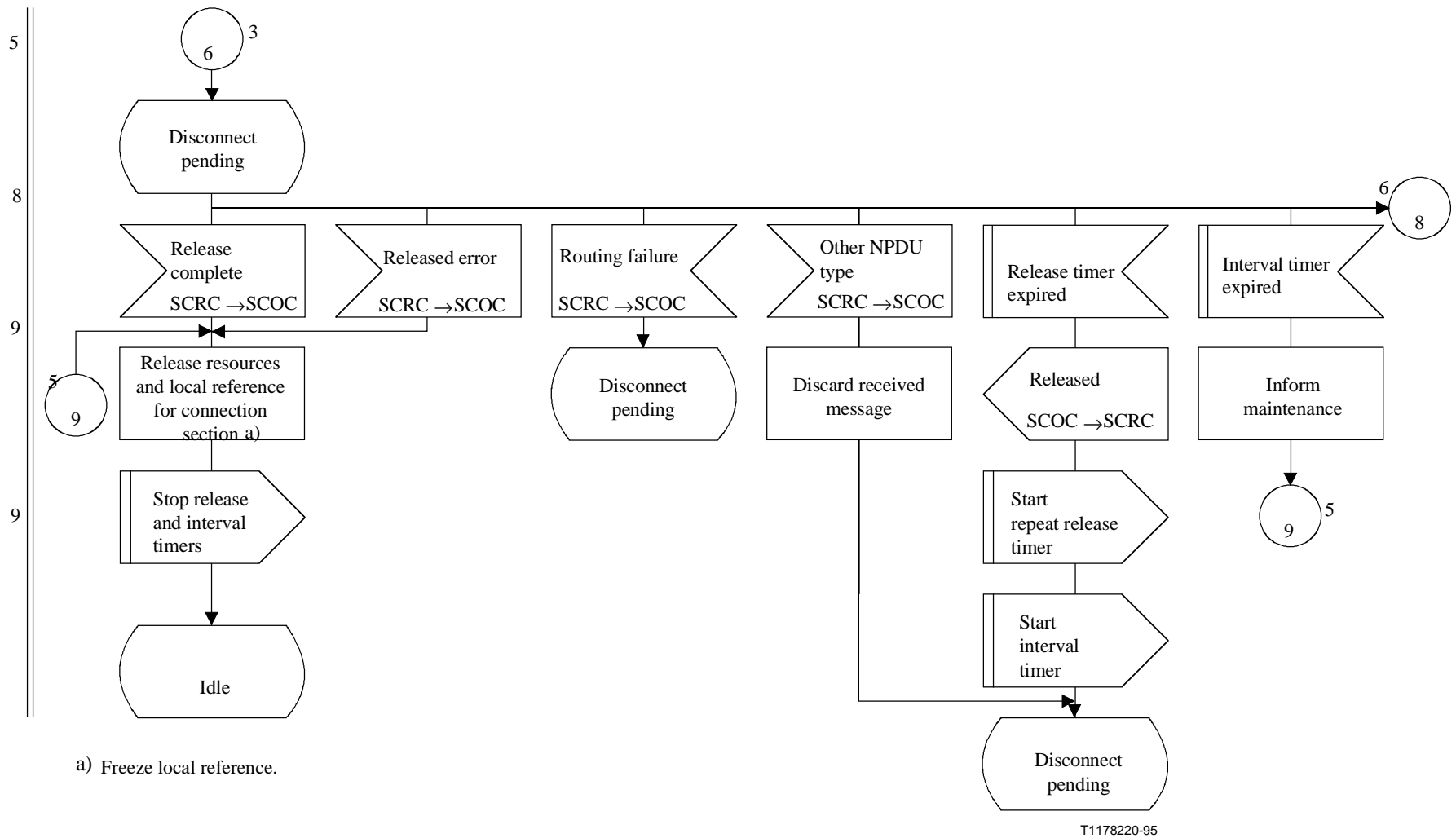
Figura C.3/Q.714 (hoja 5 de 6) – Procedimientos de liberación de la conexión en el nodo de destino para el control orientado a la conexión de la SCCP (SCOC)
