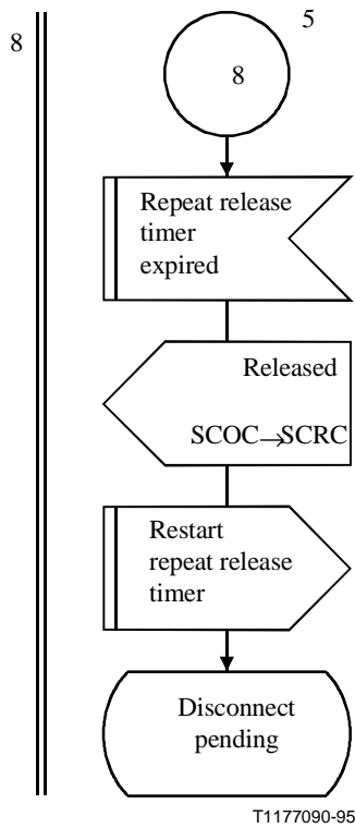
Figura C.3/Q.714 (hoja 6 de 6) – Procedimientos de liberación de la conexión en el nodo de destino para el control orientado a la conexión de la SCCP (SCOC)
