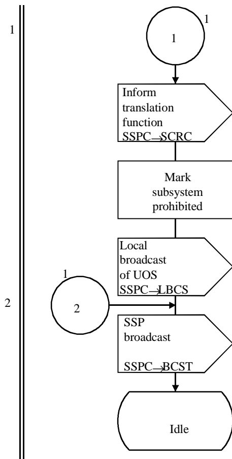
Figura D.5/Q.714 (hoja 2 de 2) – Control de subsistema prohibido (SSPC)
