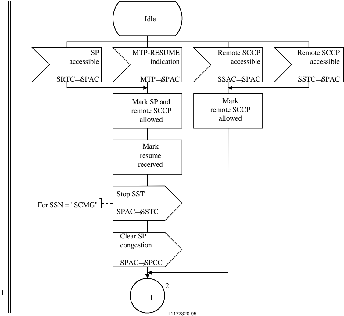
Figura D.3/Q.714 (hoja 1 de 2) – Control de punto de señalización autorizado (SPAC)
