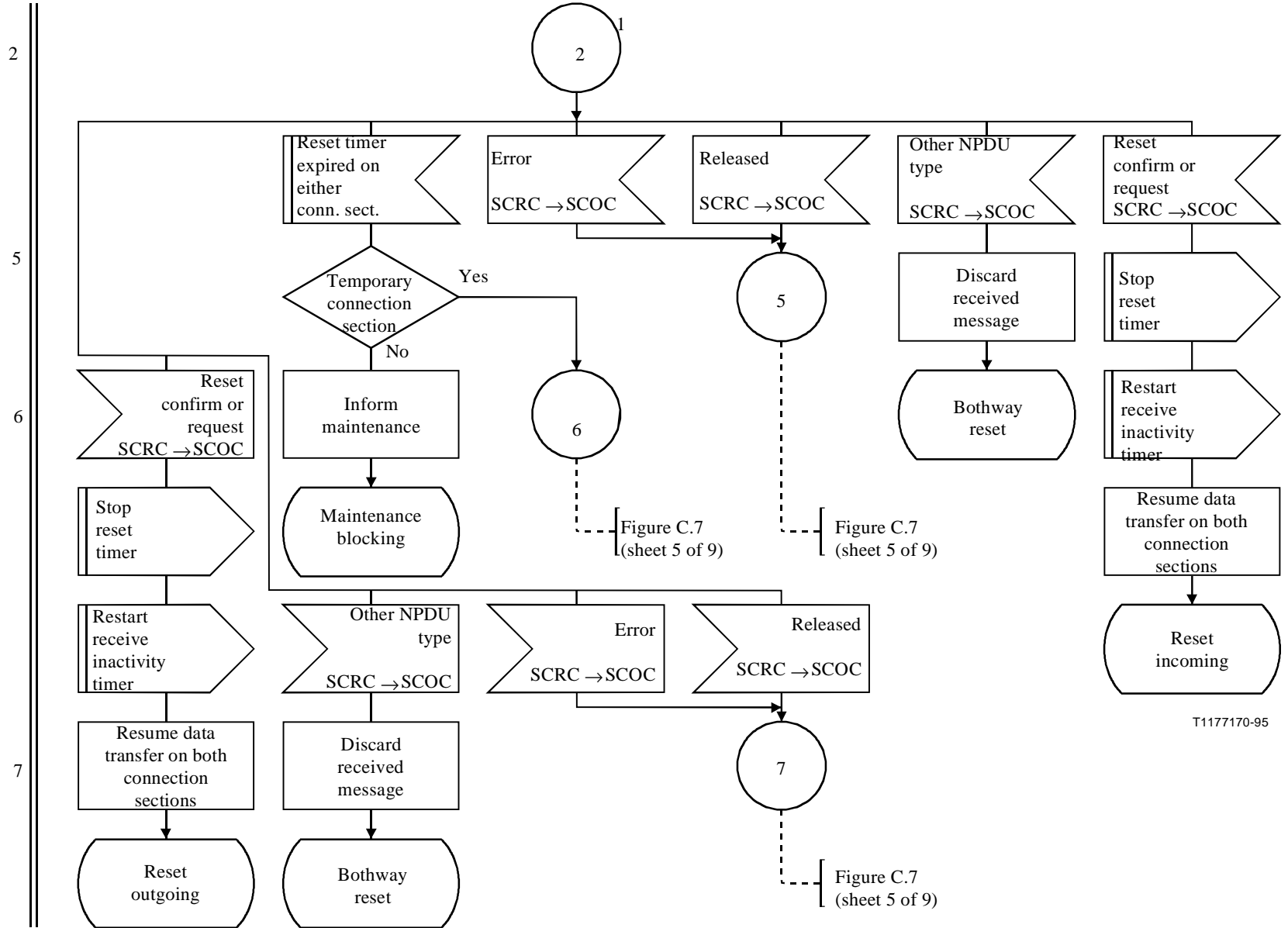
Figura C.10/Q.714 (hoja 3 de 4) – Procedimientos de reiniciación en un nodo intermedio para el control orientado a la conexión de la SCCP (SCOC)
