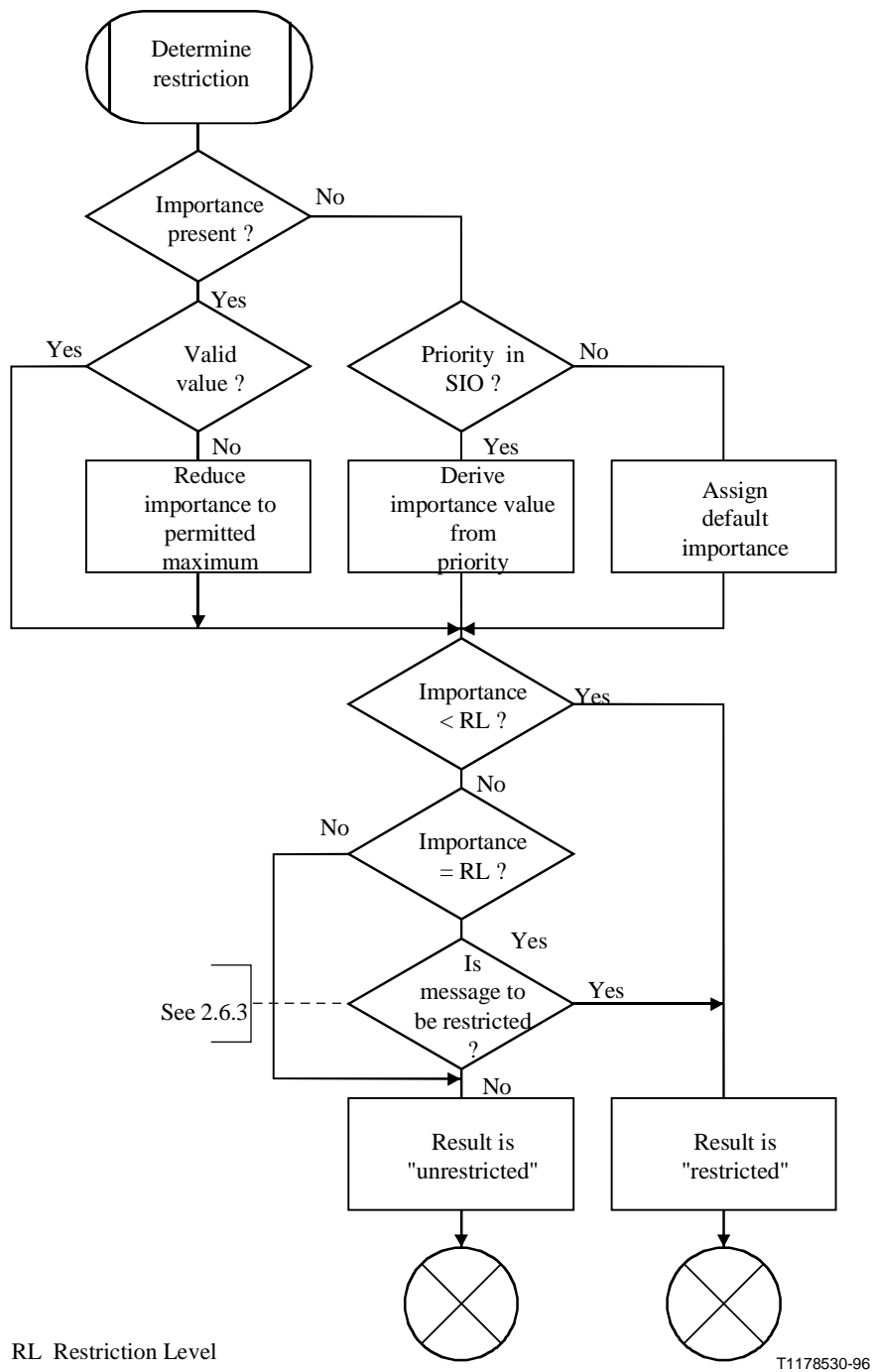
Figura C.1/Q.714 (hoja 11 de 11) – Procedimientos de control de encaminamiento de la SCCP (SCRC)
