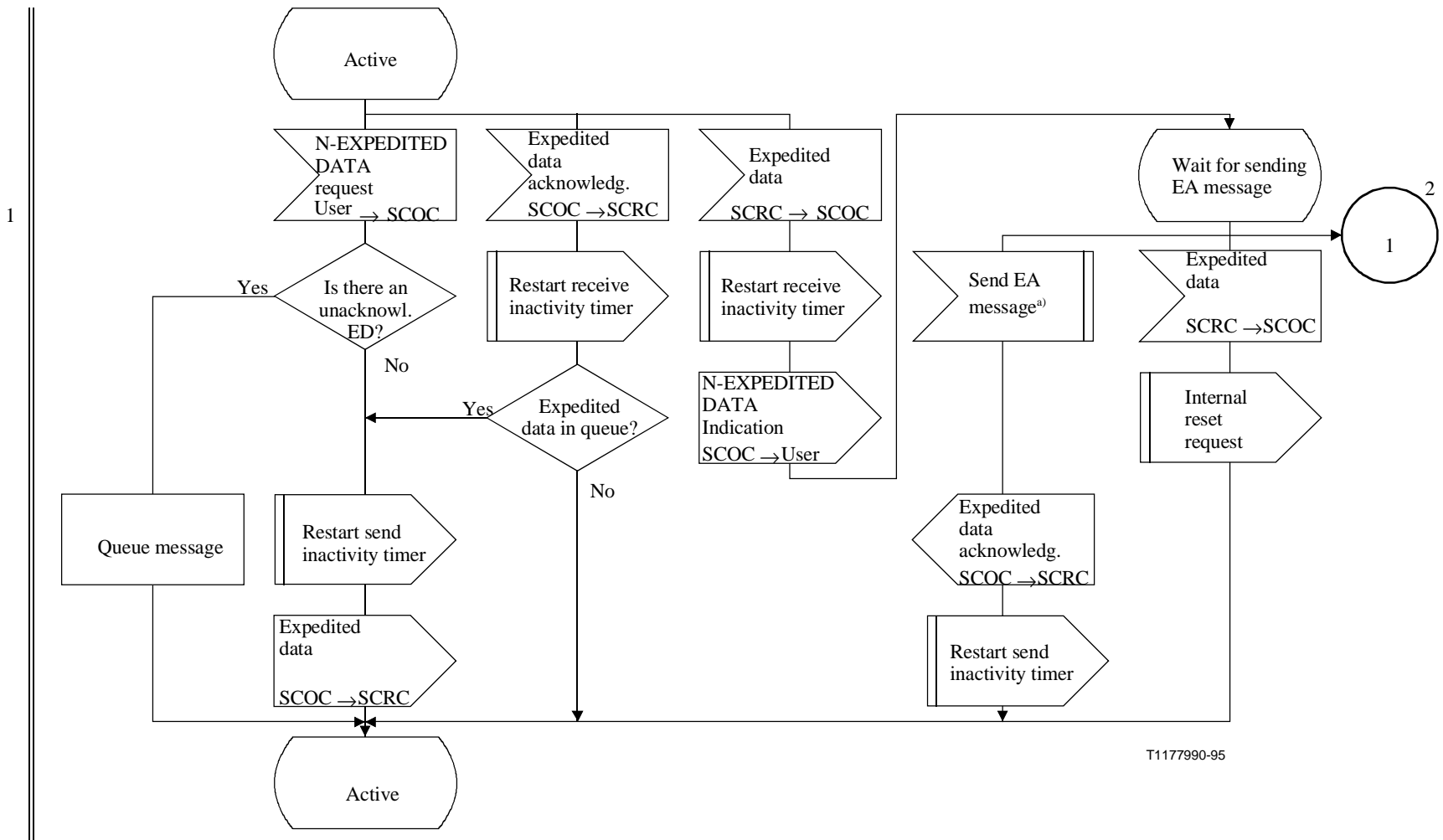
Figura C.5/Q.714 (hoja 1 de 2) – Procedimientos de transferencia de datos acelerados en los nodos de origen y de destino para el control orientado a la conexión de la SCCP (SCOC)
