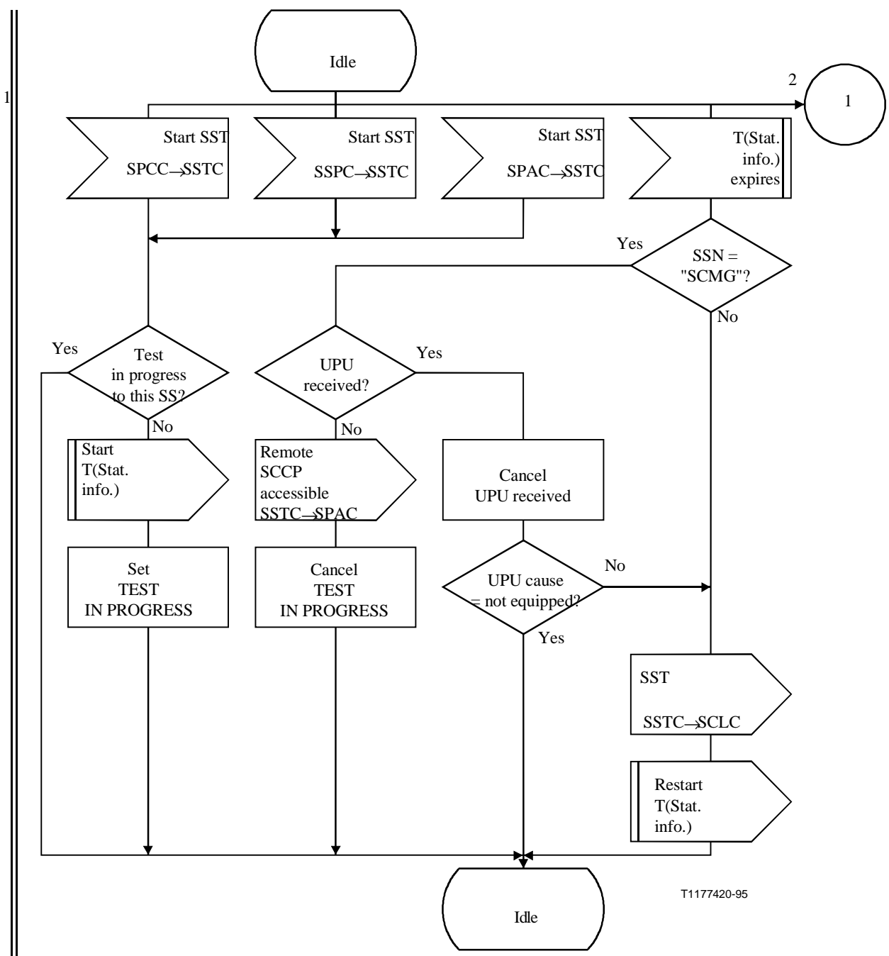
Figura D.7/Q.714 (hoja 1 de 2) – Control de prueba de estado de subsistema (SSTC)
