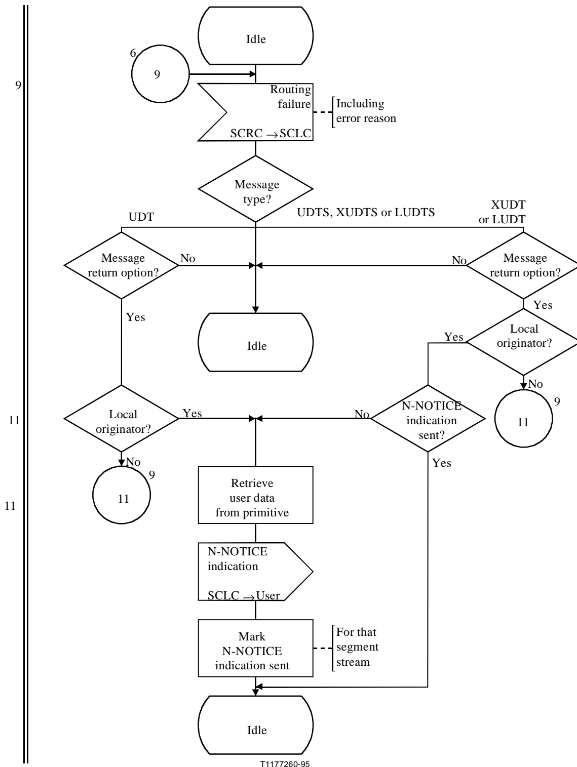
Figura C.12/Q.714 (hoja 8 de 9) – Control sin conexión de la SCCP (SCLC)
