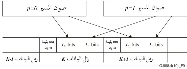
الشكل 9-1 - تعدد إرسال قناة RRC ومسيرات الكمون بالتوصية ITU-T G.993.2
