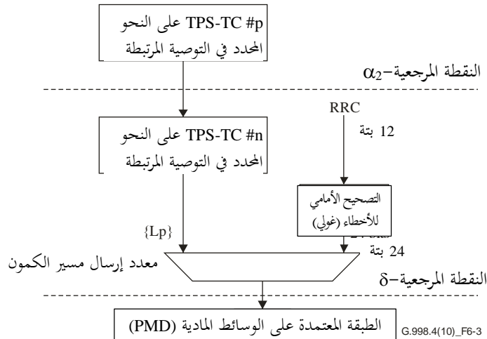
الشكل 3-6: النموذج المرجعي في اتجاه العودة عند تفعيل إعادة الإرسال في اتجاه واحد
