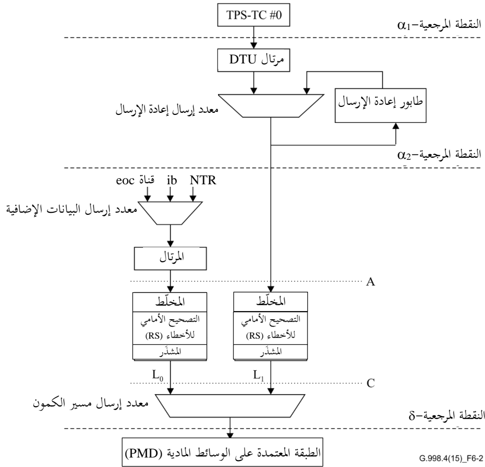
الشكل 2-6: النموذج المرجعي في الاتجاه الأمامي عند تفعيل إعادة الإرسال في اتجاه واحد
