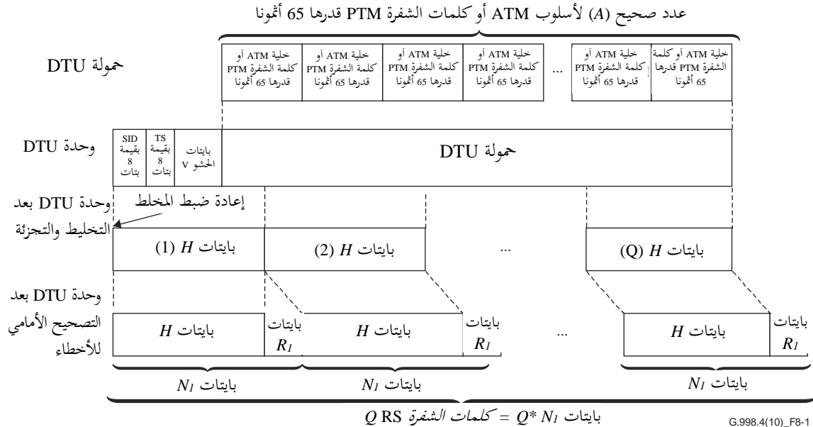
الشكل 1-8- بنية وحدات نقل البيانات بدون تحقق من الإطناب الدوري (نوع الترتيل 1) والمزامنة مع شفرات ريد-سولومون
