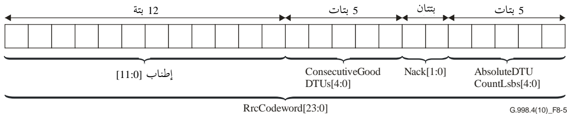
الشكل 5-8 - بنية ومحتوى مشفر قناة عودة إعادة الاتصال
