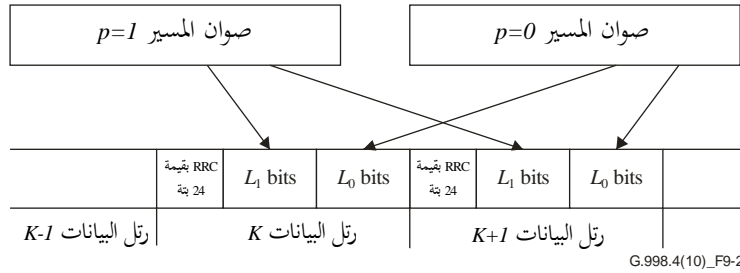
الشكل 9-2 - تعدد إرسال قناة RRC ومسيرات الكمون في التوصيتين ITU-T G.992.3 و ITU-T G.992.5
