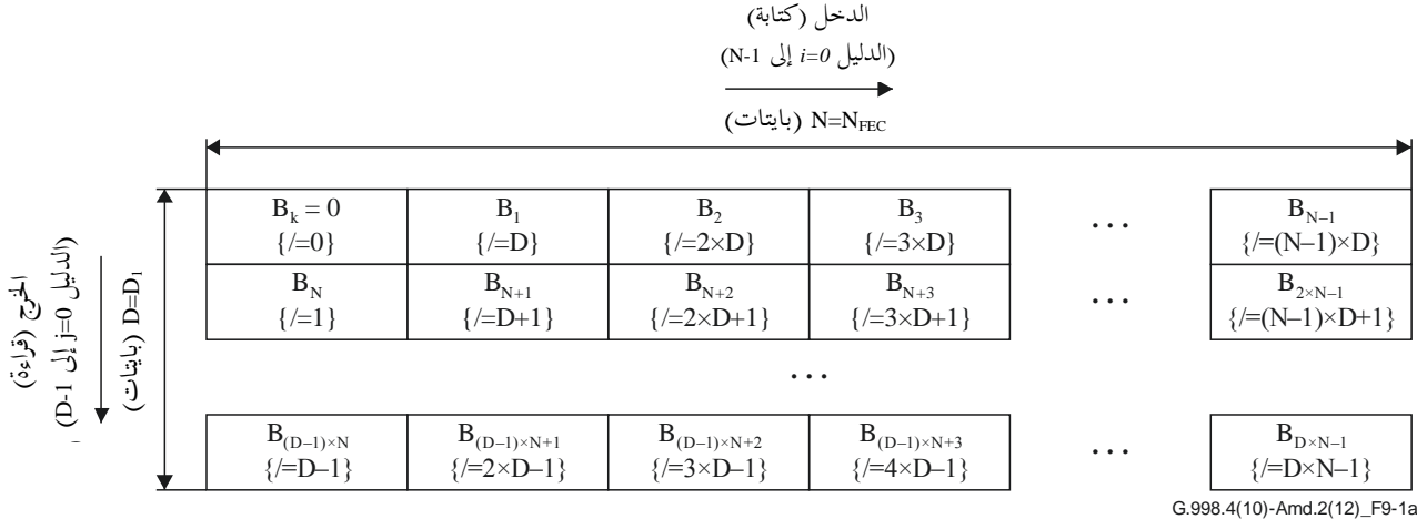
الشكل 9-a1 - توضيح مشدّر القدرات
