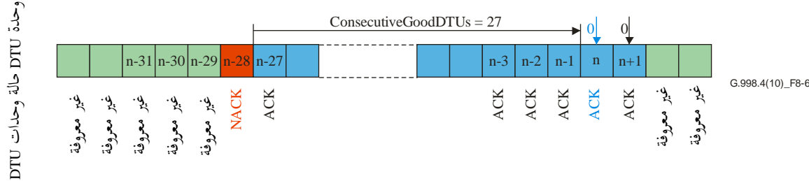
الشكل 6-8 – أمثلة على تقييم الحقل ConsecutiveGoodDtus حيث ib = 31
