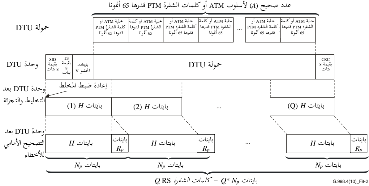
الشكل 2-8 - بنية وحدة نقل البيانات المصحوبة بتحقيق من الإطناب الدوري عند الدليل (نوع الترتيل 2) ومزامنتها مع كلمات الشفرة ريد-سولومون
