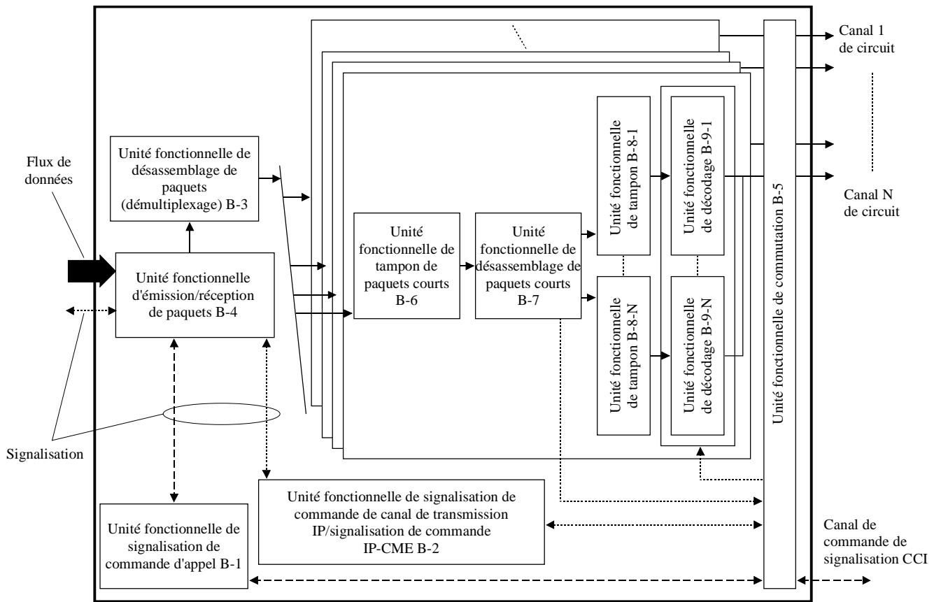
Figure I.2/G.769/Y.1242 – Exemple de schéma fonctionnel de multiplication de la partie réception d'un équipement IP-CME
