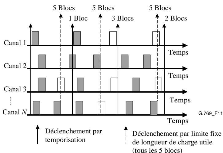
Figure 11/G.769/Y.1242 – Mécanisme de mise en paquets selon l'algorithme 4
