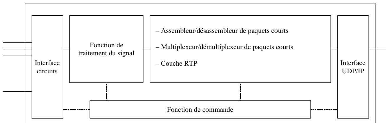
Figure 5/G.769/Y.1242 – Fonctions de base liées au traitement du flux audio
