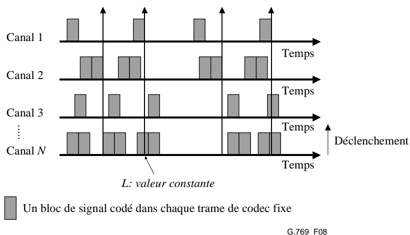
Figure 8/G.769/Y.1242 – Multiplexage et mise en paquets avec déclenchement par une limite fixe de longueur de charge utile
