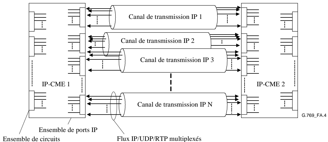
Figure A.4/G.769/Y.1242 – Configuration de la connexion RTP entre deux équipements IP-CME
