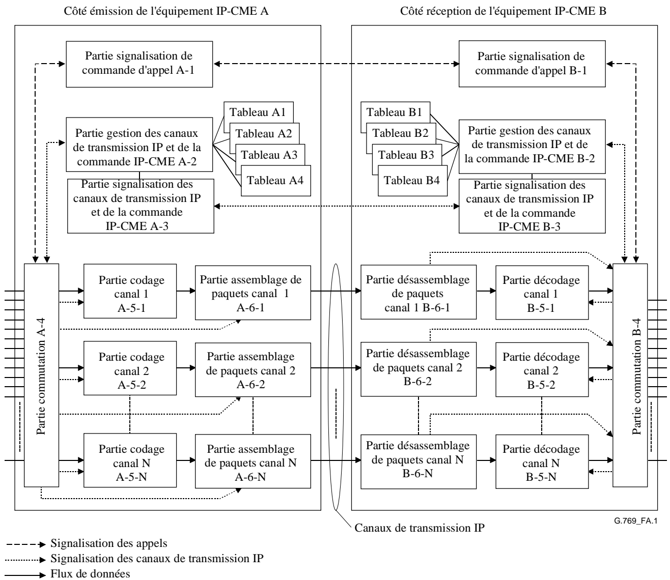
Figure A.1/G.769/Y.1242 – Schéma fonctionnel de la commande des canaux de transmission IP
