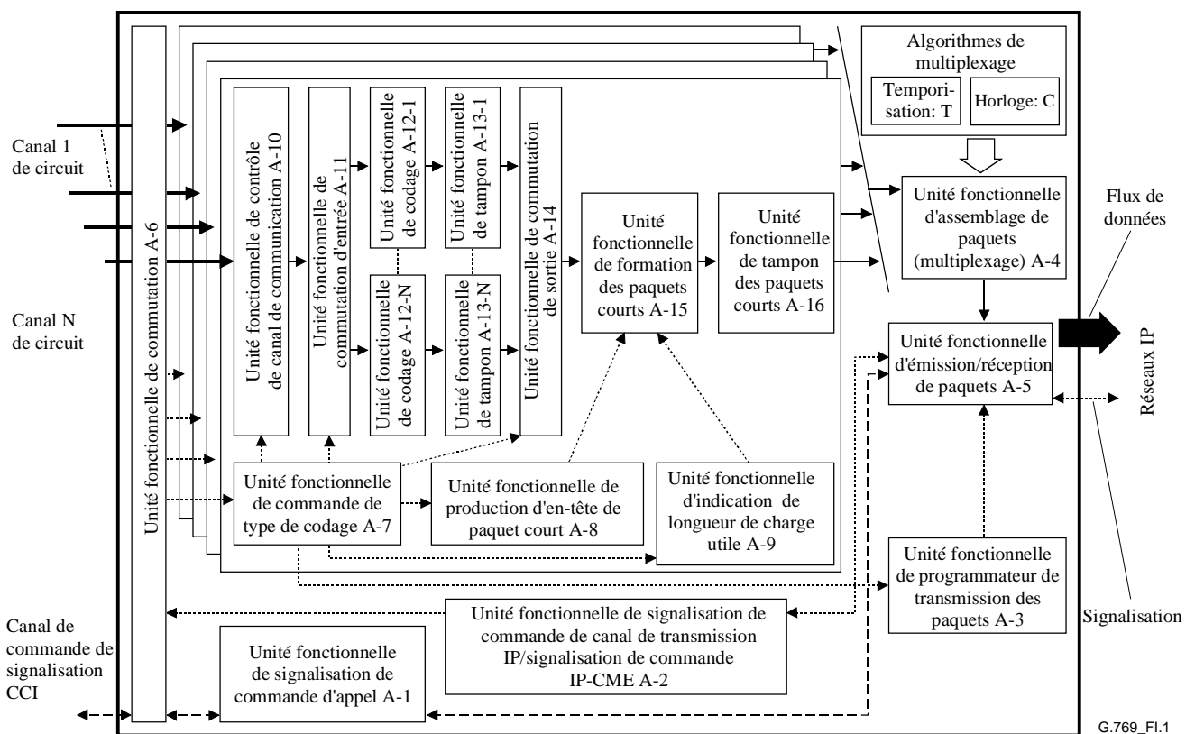
Figure I.1/G.769/Y.1242 – Exemple de schéma fonctionnel de multiplication de la partie émission d'un équipement IP-CME
