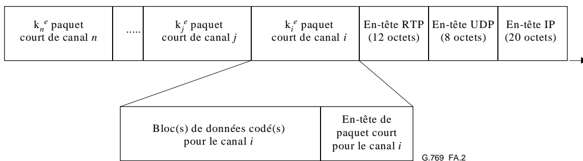
Figure A.2/G.769/Y.1242 – Eléments de structure de paquet IP et d'en-tête de paquet court
