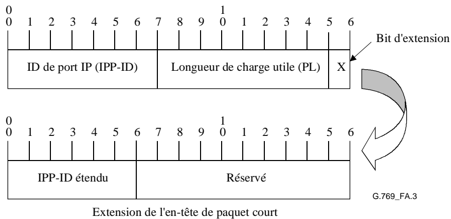
Figure A.3/G.769/Y.1242 – Format de l'en-tête de paquet court
