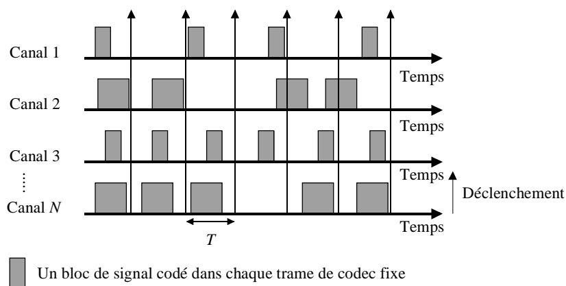
Figure 10/G.769/Y.1242 – Multiplexage et mise en paquets avec déclenchement par temporisation périodique
