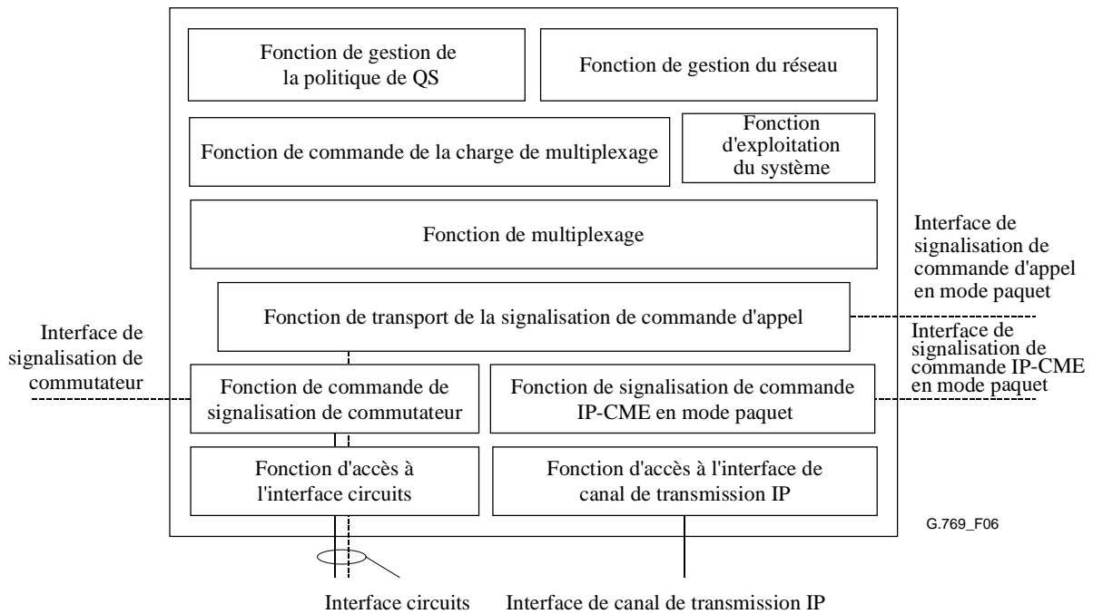
Figure 6/G.769/Y.1242 – Fonctions des équipements IP-CME
