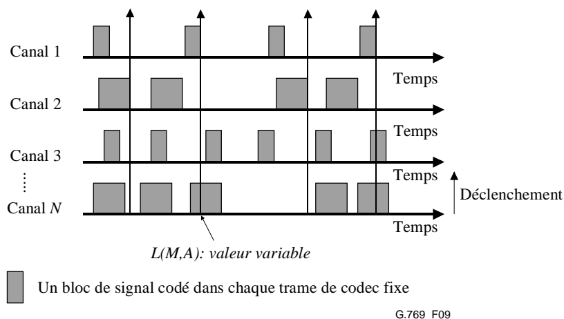
Figure 9/G.769/Y.1242 – Multiplexage et mise en paquets avec déclenchement par une limite dynamique de longueur de charge utile
