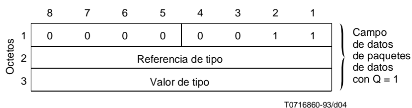
Figura 4/X.29 – Formato de mensaje de PAD de indicación de corte
