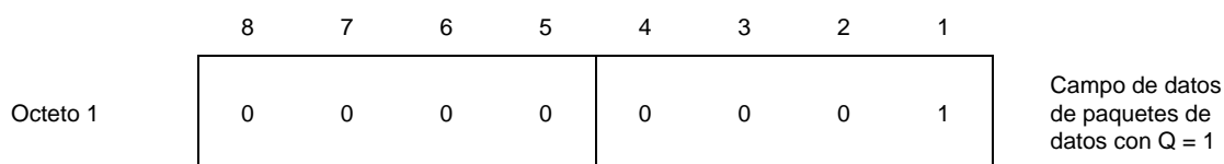
Figura 5/X.29 – Formato de mensaje de PAD de invitación a liberar
