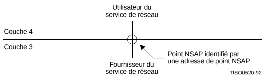
Figure A.2 – Adresse de point NSAP
