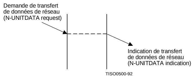
Figure 21 – Enchaînement des primitives dans une transmission sur le réseau en mode sans connexion
