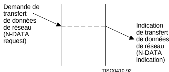
Figure 12 – Enchaînement de primitives correspondant à un transfert de données
