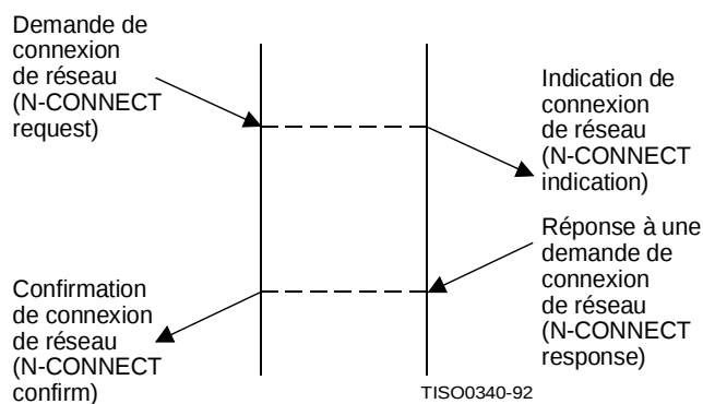
Figure 5 – Enchaînement de primitives pour un établissement de connexion de réseau réussi
