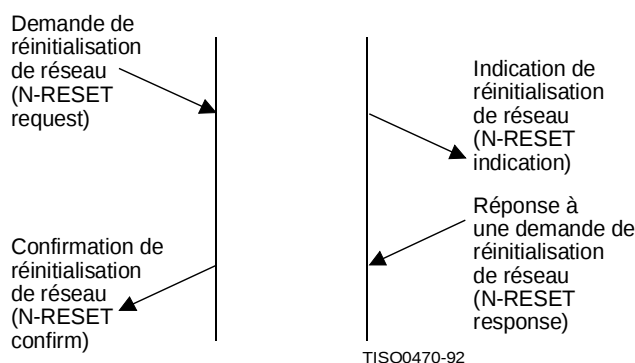
Figure 18 – Enchaînement de primitives correspondant à une réinitialisation provoquée simultanément par un utilisateur et par le fournisseur du service de réseau
