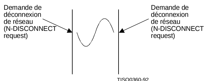
Figure 7 – Enchaînement de primitives correspondant à une libération de la connexion de réseau provoquée simultanément par les deux utilisateurs du service de réseau
