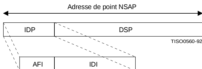
Figure A.6 – Structure de l'adresse de point NSAP
