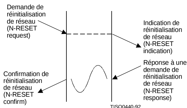
Figure 15 – Enchaînement de primitives correspondant à une réinitialisation provoquée par un utilisateur du service de réseau
