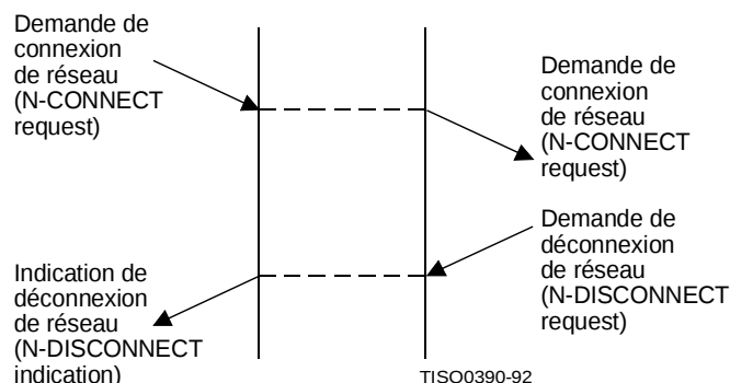
Figure 10 – Enchaînement de primitives correspondant au refus par un utilisateur du service de réseau d'une tentative d'établissement d'une connexion de réseau
