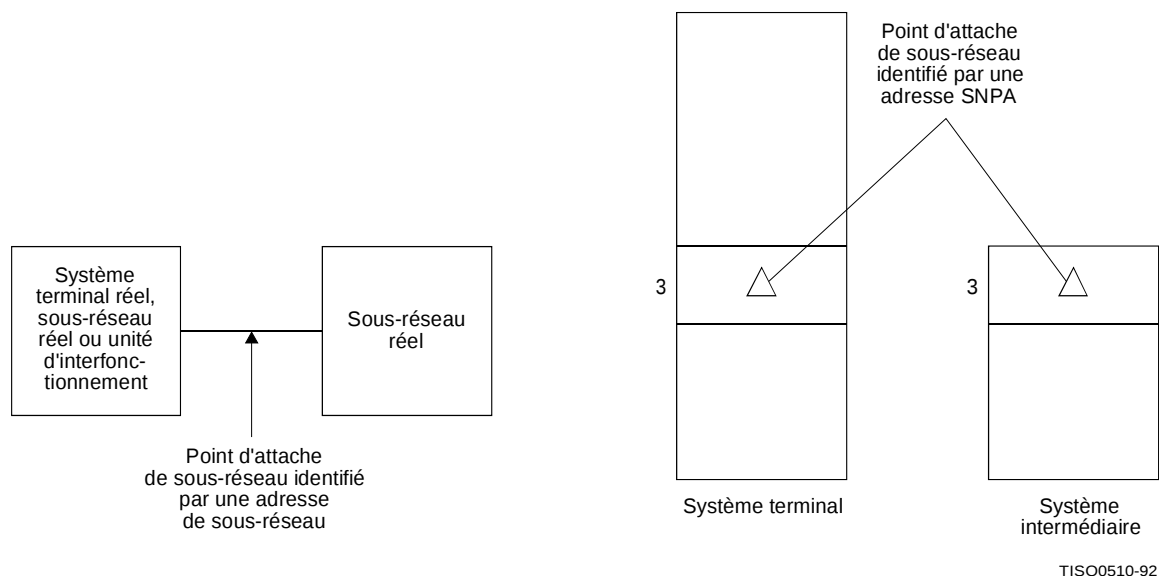
Figure A.1 – Adresse de sous-réseau
