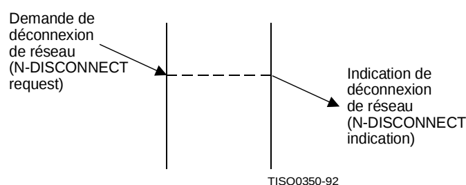
Figure 6 – Enchaînement de primitives correspondant à une libération de la connexion de réseau provoquée par un utilisateur du service de réseau
