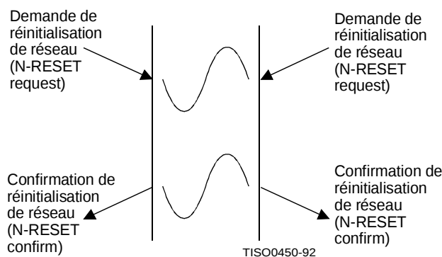
Figure 16 – Enchaînement de primitives correspondant à une réinitialisation provoquée simultanément par les deux utilisateurs du service de réseau
