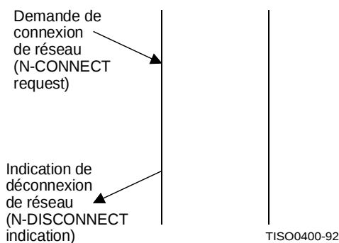
Figure 11 – Enchaînement de primitives correspondant au refus par le fournisseur du service de réseau d'une tentative d'établissement d'une connexion de réseau
