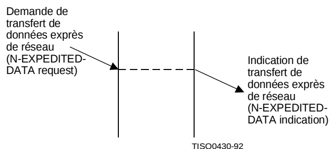
Figure 14 – Enchaînement de primitives correspondant à un transfert de données exprès
