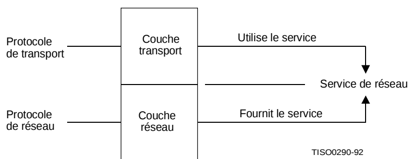
Relation entre le service de réseau et le réseau OSI et les protocoles de transport
