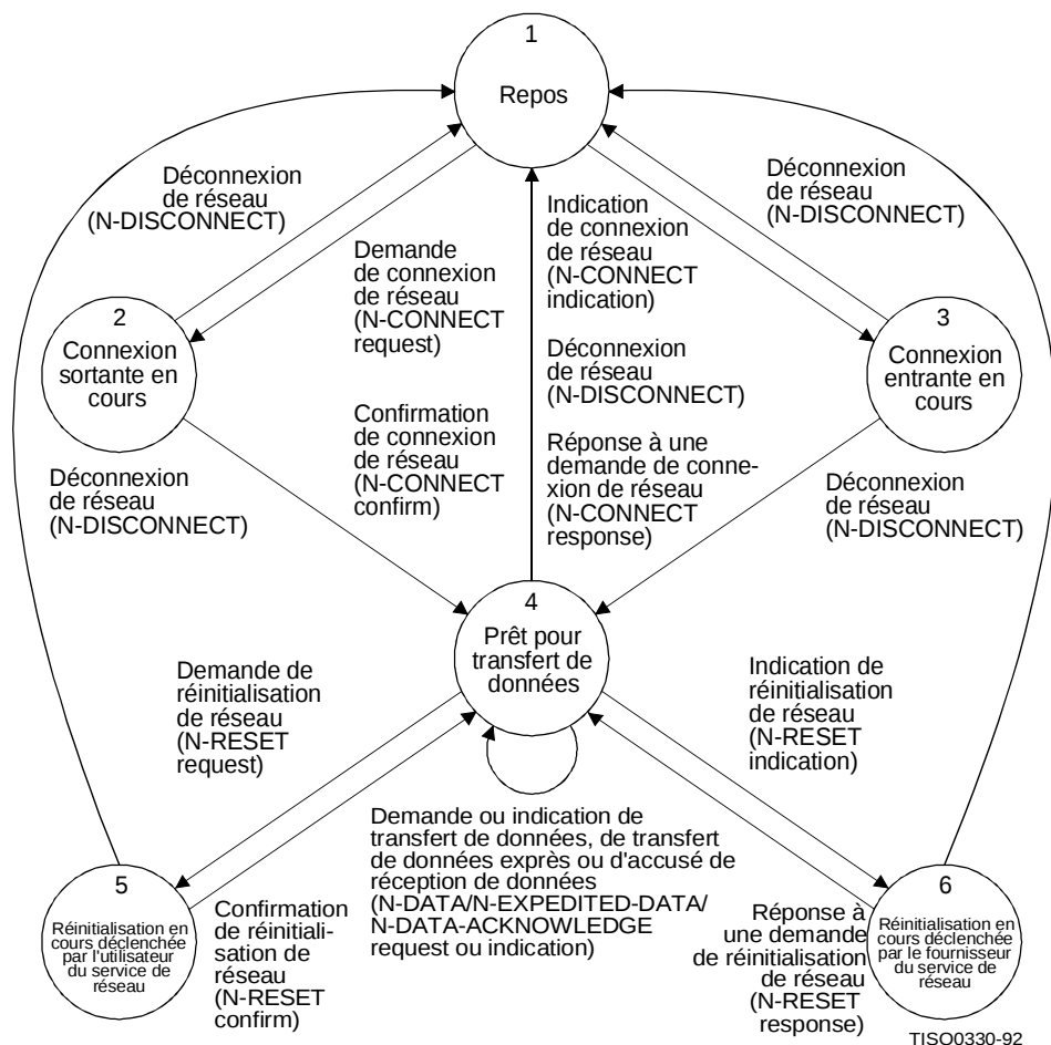
Figure 4 – Diagramme de transitions d'états correspondant aux enchaînements de primitives au niveau d'une extrémité de connexion de réseau
