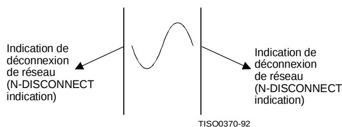
Figure 8 – Enchaînement de primitives correspondant à une libération de la connexion de réseau provoquée par le fournisseur du service de réseau
