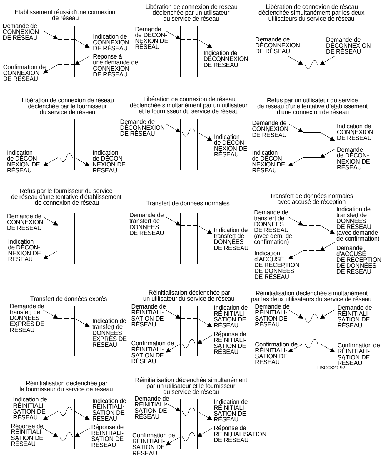
Figure 3 – Diagrammes d'enchaînement des primitives du service de réseau
