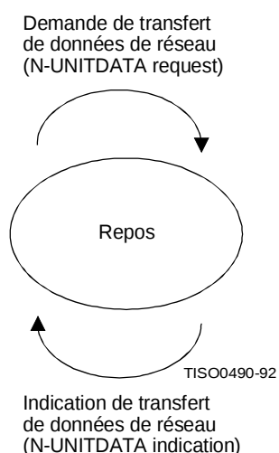
Figure 20 – Diagramme de transition d'état représentant les enchaînements de primitives en mode sans connexion au niveau d'un point NSAP
