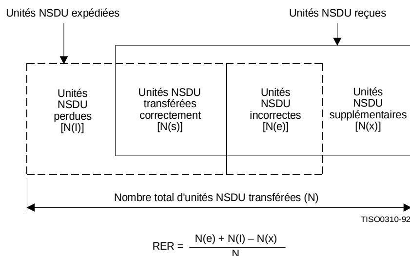
Figure 2 – Composantes du taux d'erreur résiduel
