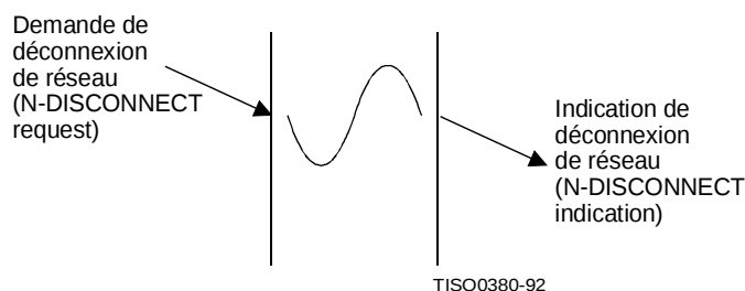
Figure 9 – Enchaînement de primitives correspondant à une libération de la connexion de réseau provoquée simultanément par un utilisateur et par le fournisseur du service de réseau
