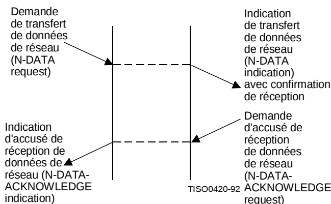
Figure 13 – Enchaînement de primitives correspondant à un transfert de données correct avec confirmation de réception
