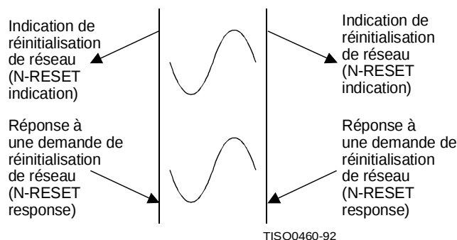
Figure 17 – Enchaînement de primitives correspondant à une réinitialisation provoquée par le fournisseur du service de réseau
