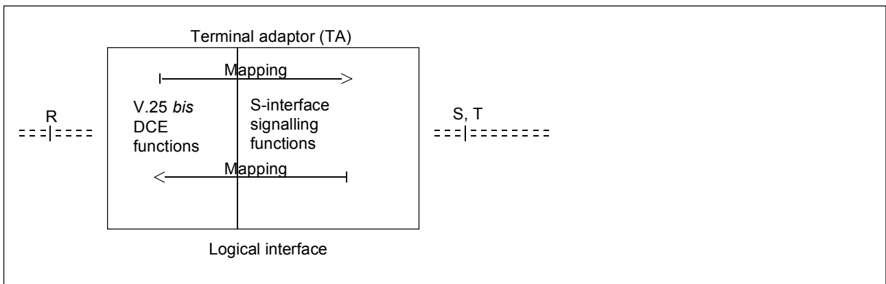
FIGURE II-1/V.110 Terminal adaptor V.25 bis mapping
