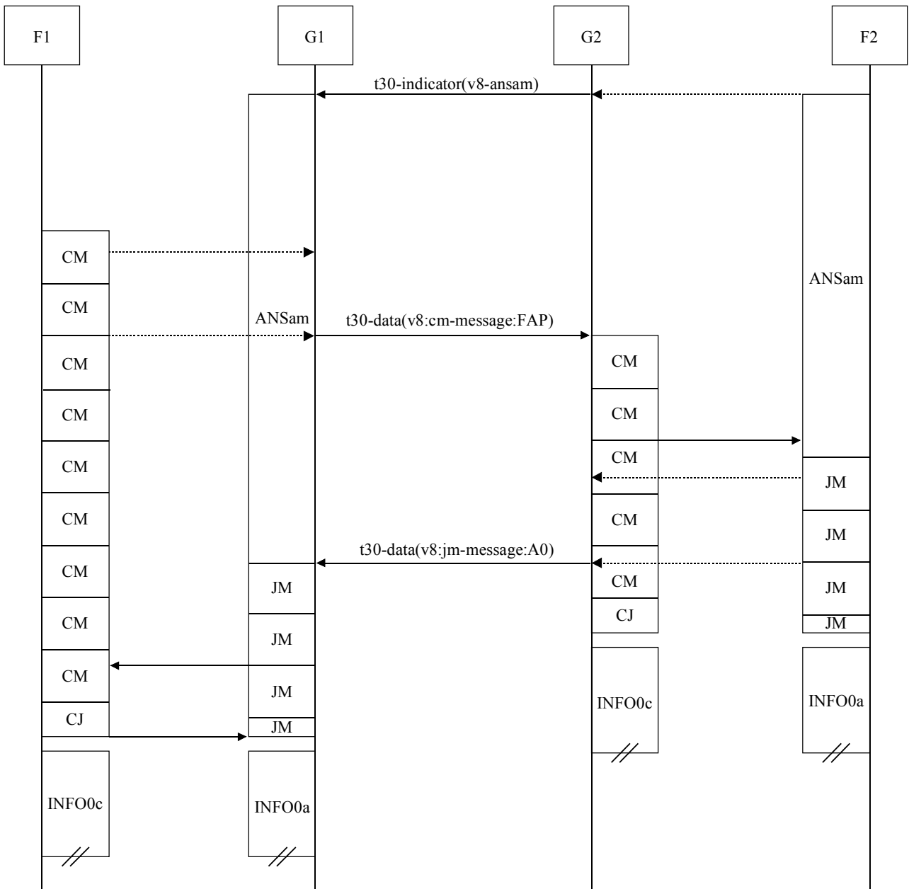
Figure IV.1/T.38 – Signalisation V.8 utilisant les profils et accusés de réception
