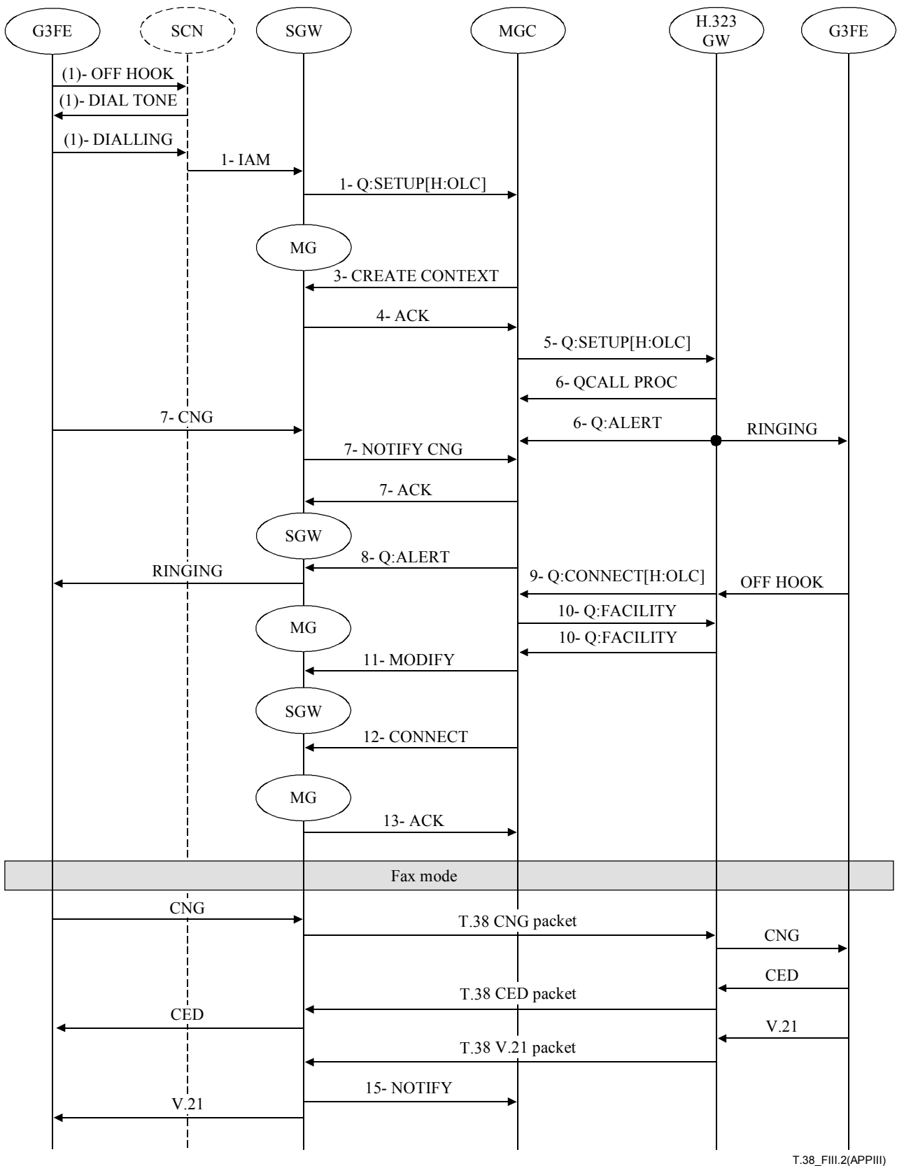
Figure III.2/T.38 – Appel de télécopie seulement entre points d'extrémité H.248 et H.323
