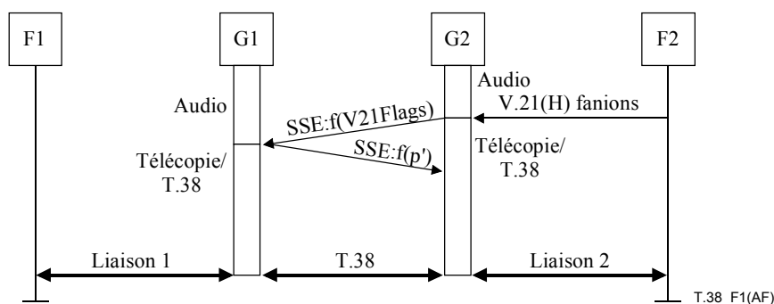
Figure F.1/T.38 – Mode FoIP T.38 (passage du mode MoIP au mode télécopie T30)
