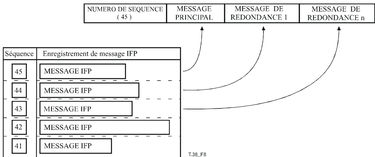
Figure 8/T.38 – Inclusion de paquets (champs) IFP antérieurs (redondants) dans un paquet UDPTL
