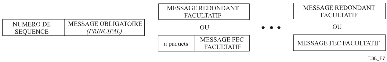
Figure 7/T.38 – Format de base de la section de charge utile UDPTL (en-tête UDP non représenté)
