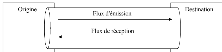
Figure B.1/T.38 – Paire de voies unidirectionnelles
