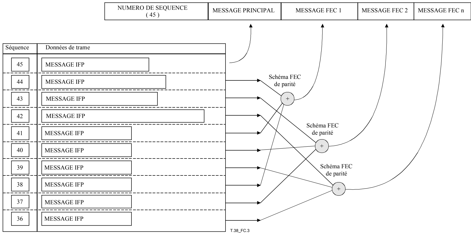
Figure C.3/T.38 – Génération de plusieurs messages FEC assurant une protection contre les erreurs en rafale
