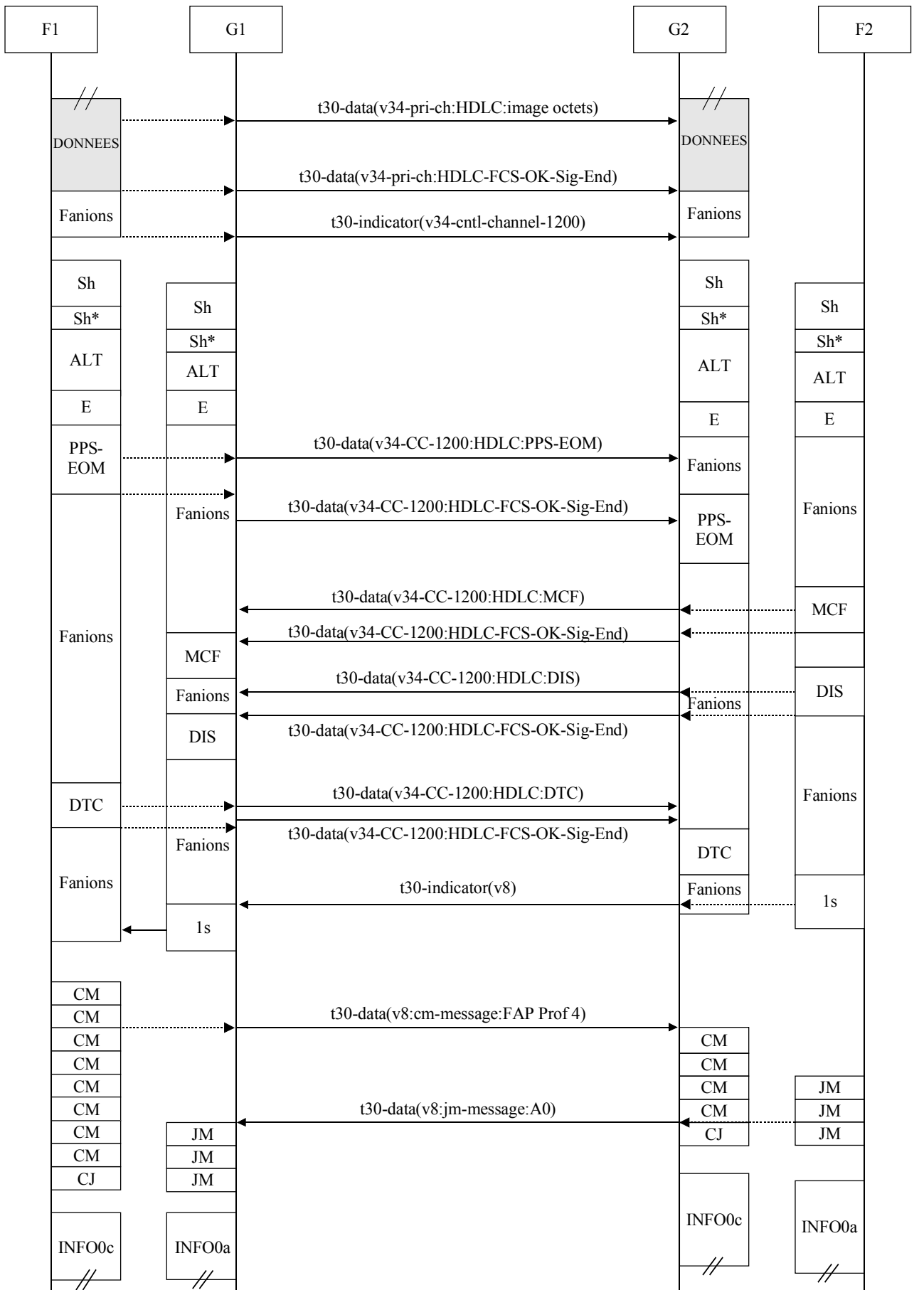
Figure IV.9/T.38 – Relève dans les deux sens
