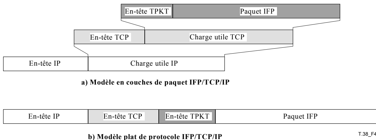
Figure 4/T.38 – Structure d'un paquet TCP/TPKT/IP de niveau élevé
