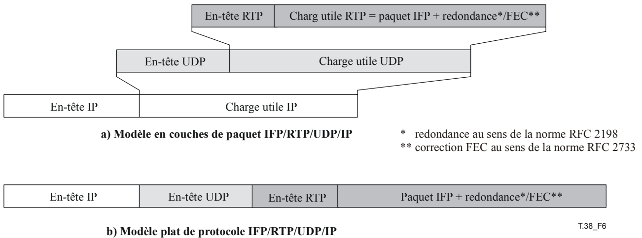
Figure 6/T.38 – Structure d'un paquet RTP/UDP/IP de niveau élevé
