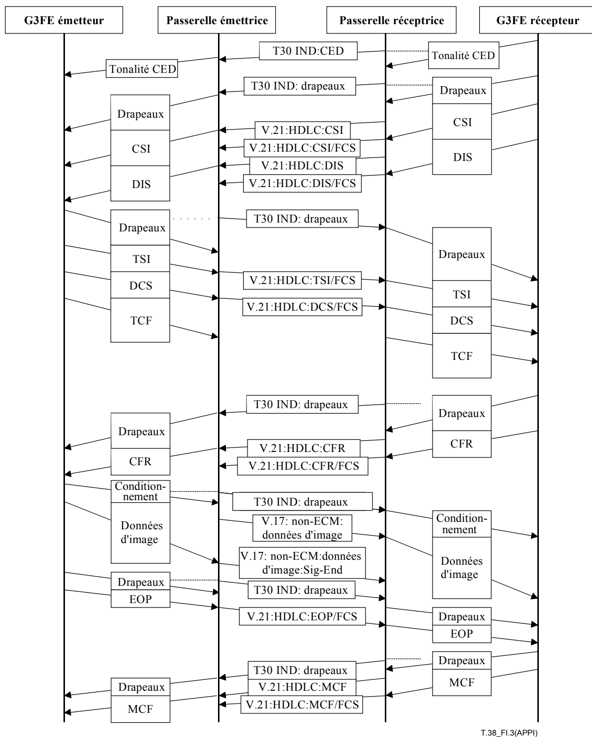
Figure I.3/T.38 – Utilisation de nombreuses trames pour chaque séquence BCS
