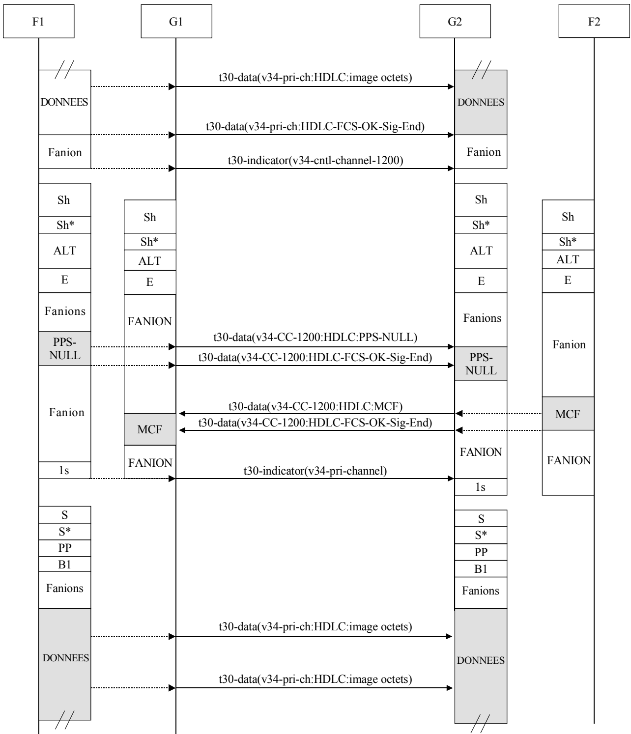
Figure IV.3/T.38 – Entre parties de pages
