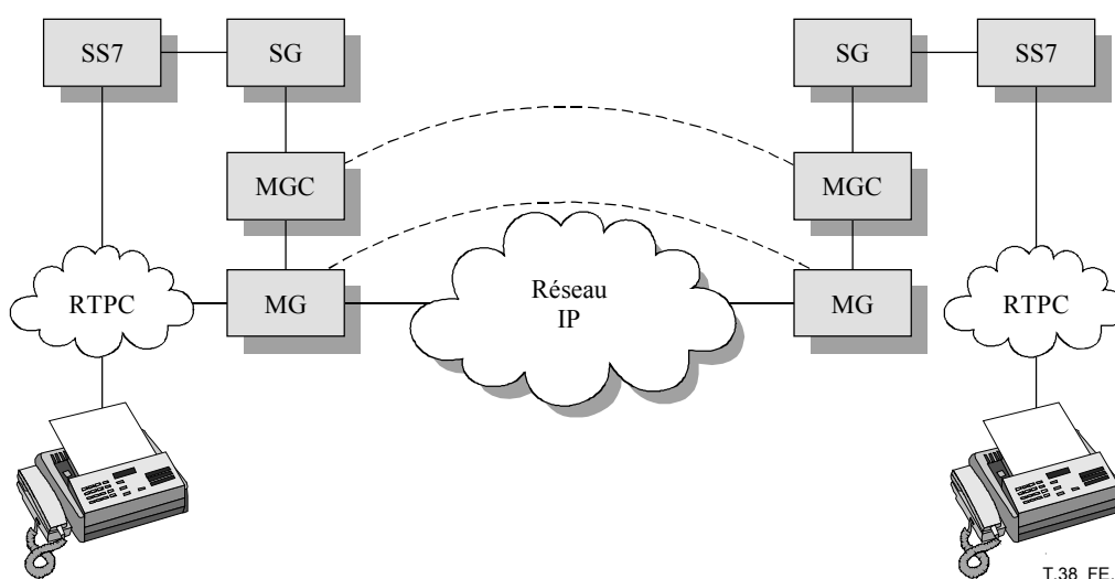
Figure E.1/T.38 – Modèle décomposé type
