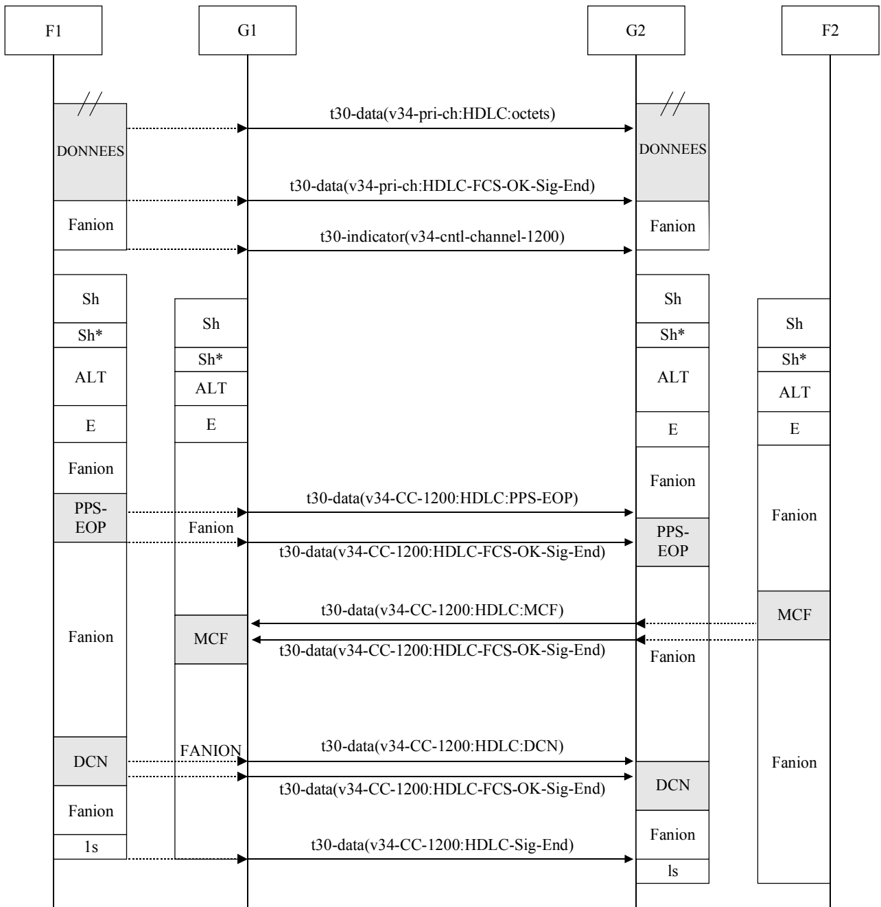
Figure IV.4/T.38 – Dernière page
