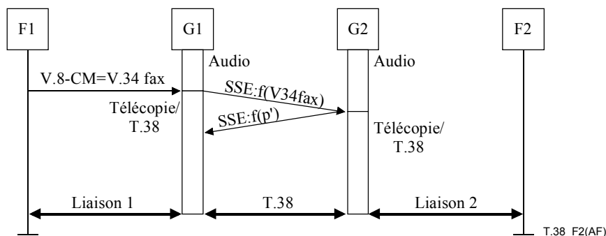
Figure F.2/T.38 – Mode FoIP T.38 (passage du mode MoIP au mode télécopie V34)
