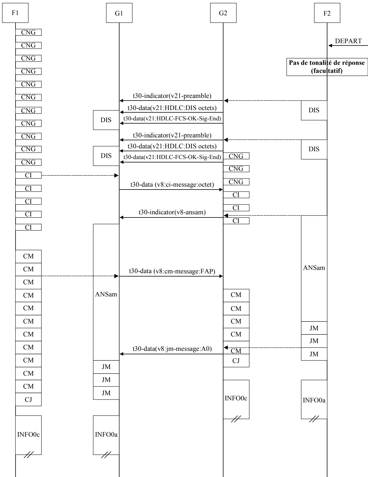
Figure IV.11/T.38 – Réception manuelle (le signal DIS a le bit 6 mis à 1 pour indiquer la capacité V.8)
