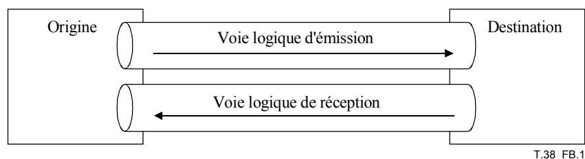
Figure B.1/T.38 – Paire de voies unidirectionnelles
