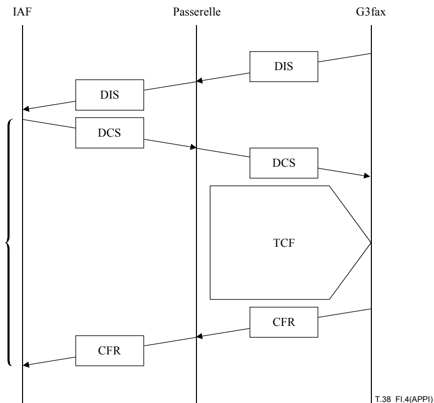
Figure I.4/T.38 – IAF structure temporelle de l'envoi des signaux DCS et CFR
