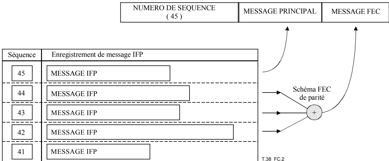
Figure C.2/T.38 – Génération et paquets d'une trame FEC de parité unique
