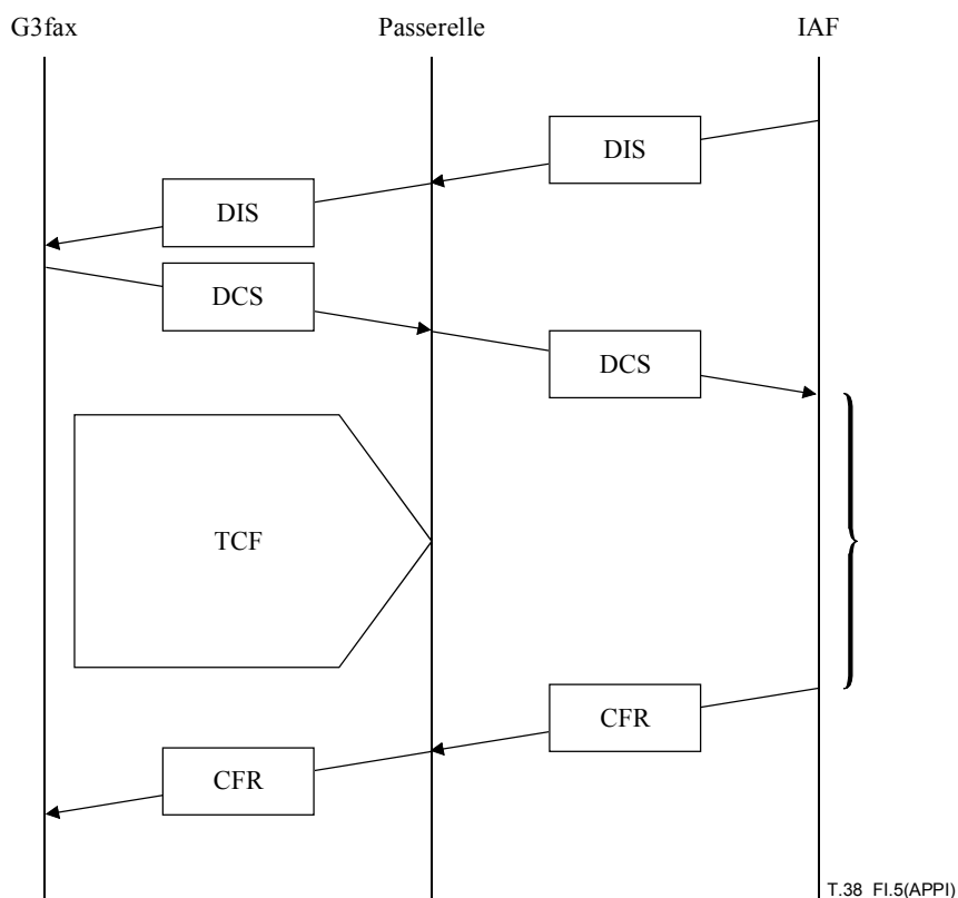
Figure I.5/T.38 – IAF Structure temporelle de la réception des signaux DCS et CFR
