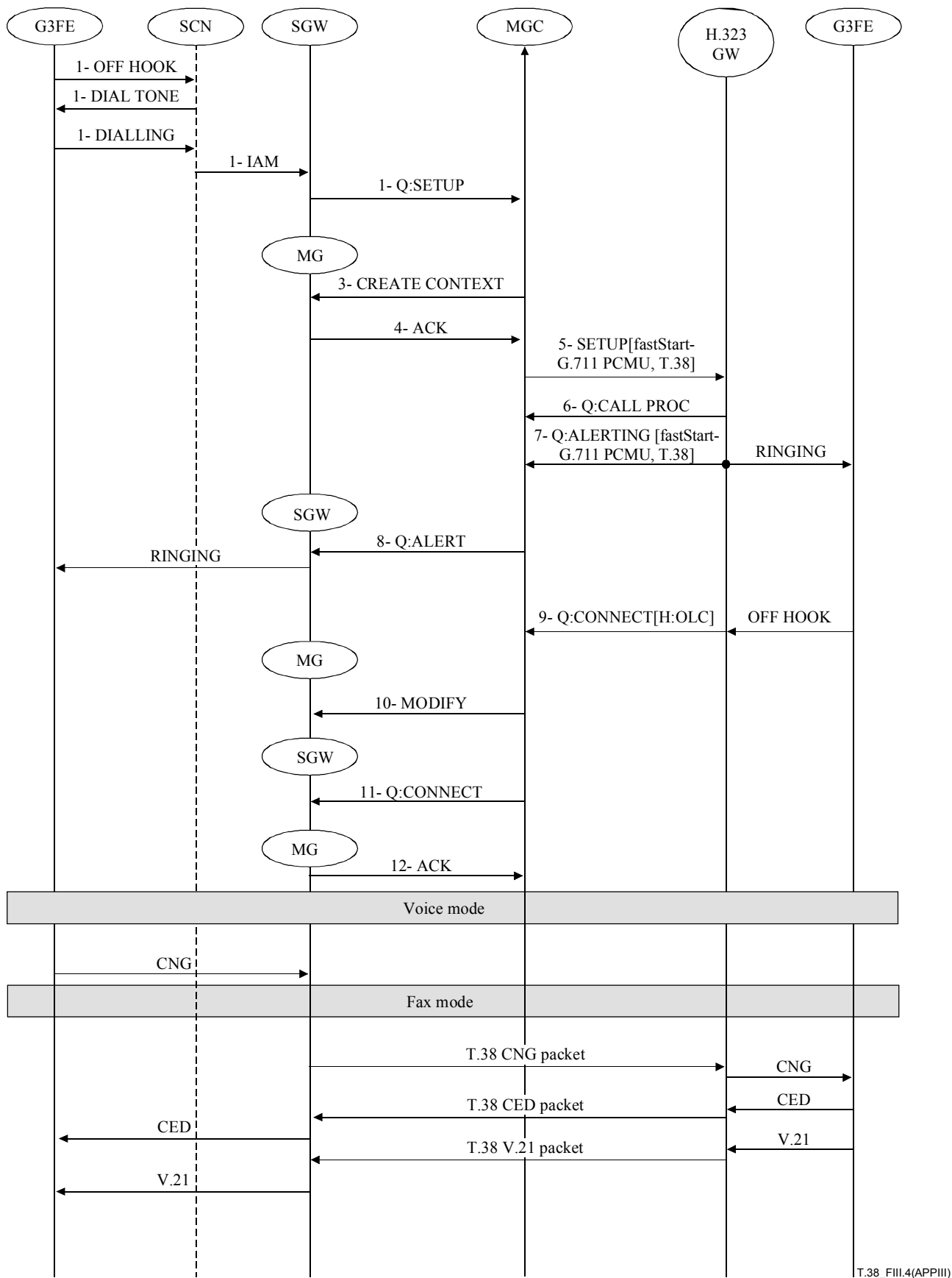
Figure III.4/T.38 – Appel vocal à télécopieur entre points d'extrémité H.248 et H.323 assurant la méthode T.38 du passage autonome entre les modes VoIP et FoIP
