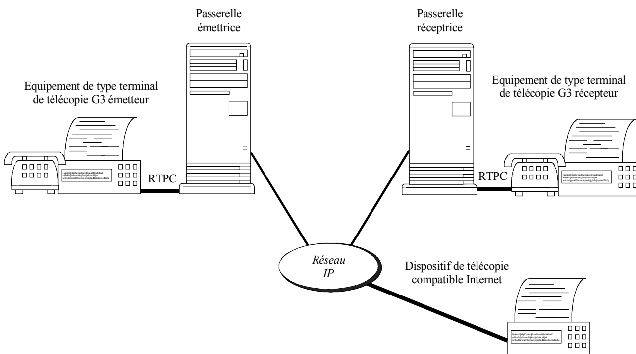
Figure 1/T.38 – Modèle pour la transmission de télécopie sur les réseaux IP
