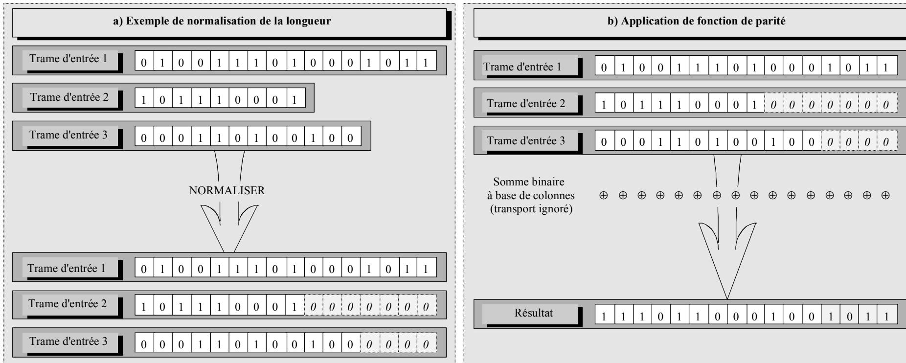
Figure C.1/T.38 – Illustration de la normalisation de la longueur et de l'organisation de la fonction de parité
