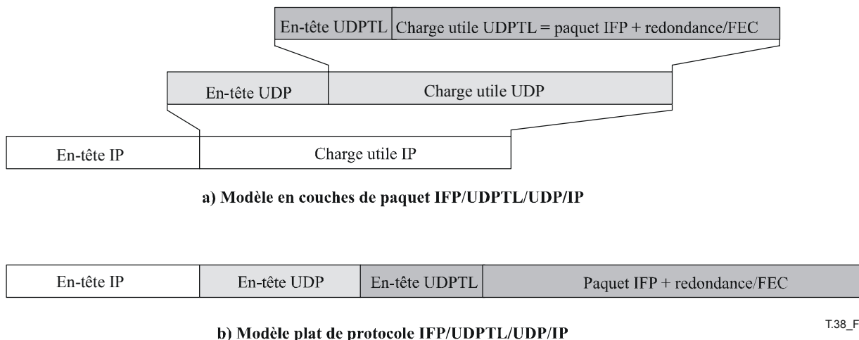
Figure 5/T.38 – Structure d'un paquet UDPTL/UDP/IP de niveau élevé
