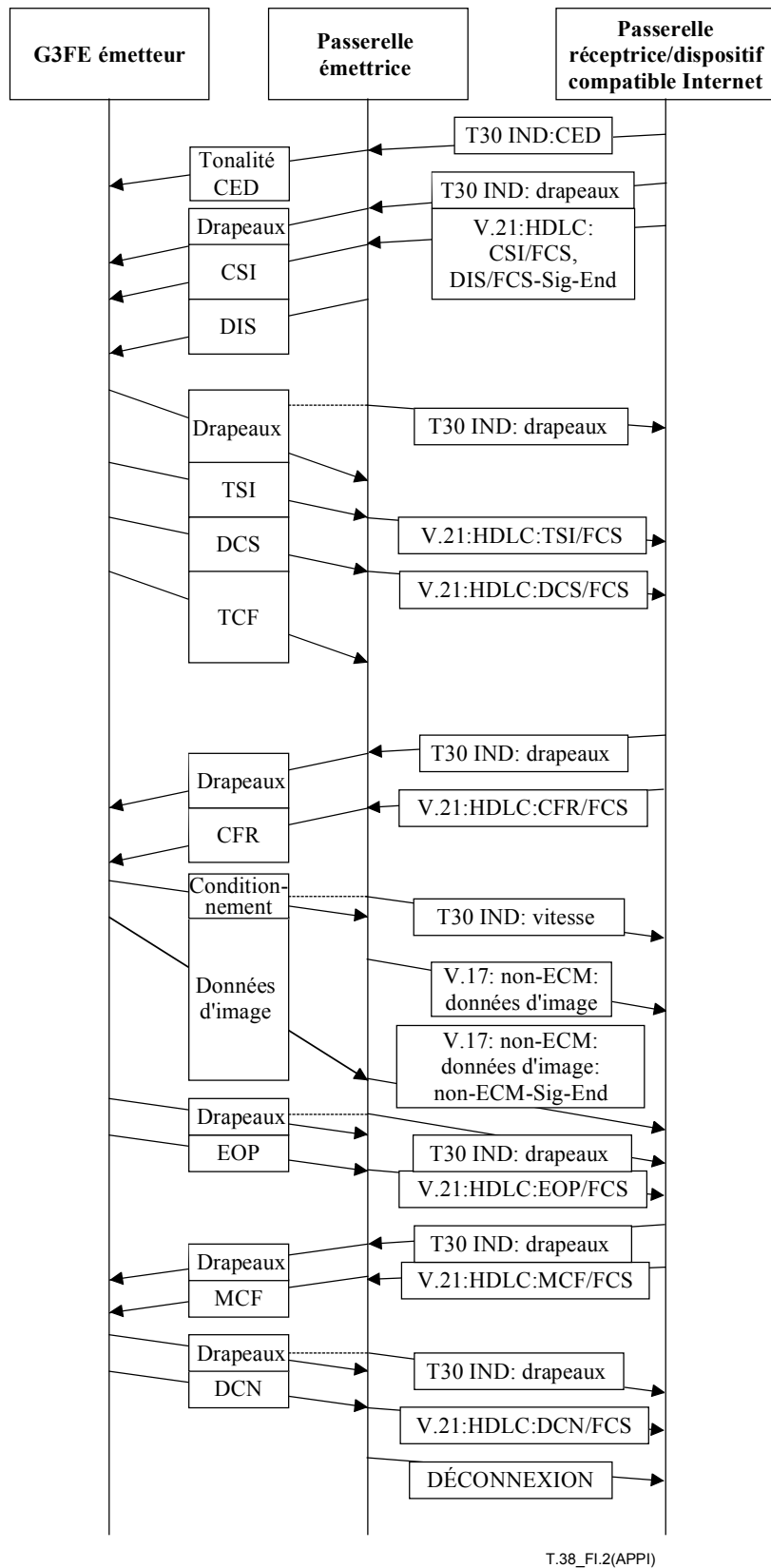
Figure I.2/T.38 – Dispositif de télécopie traditionnel et dispositif compatible Internet
