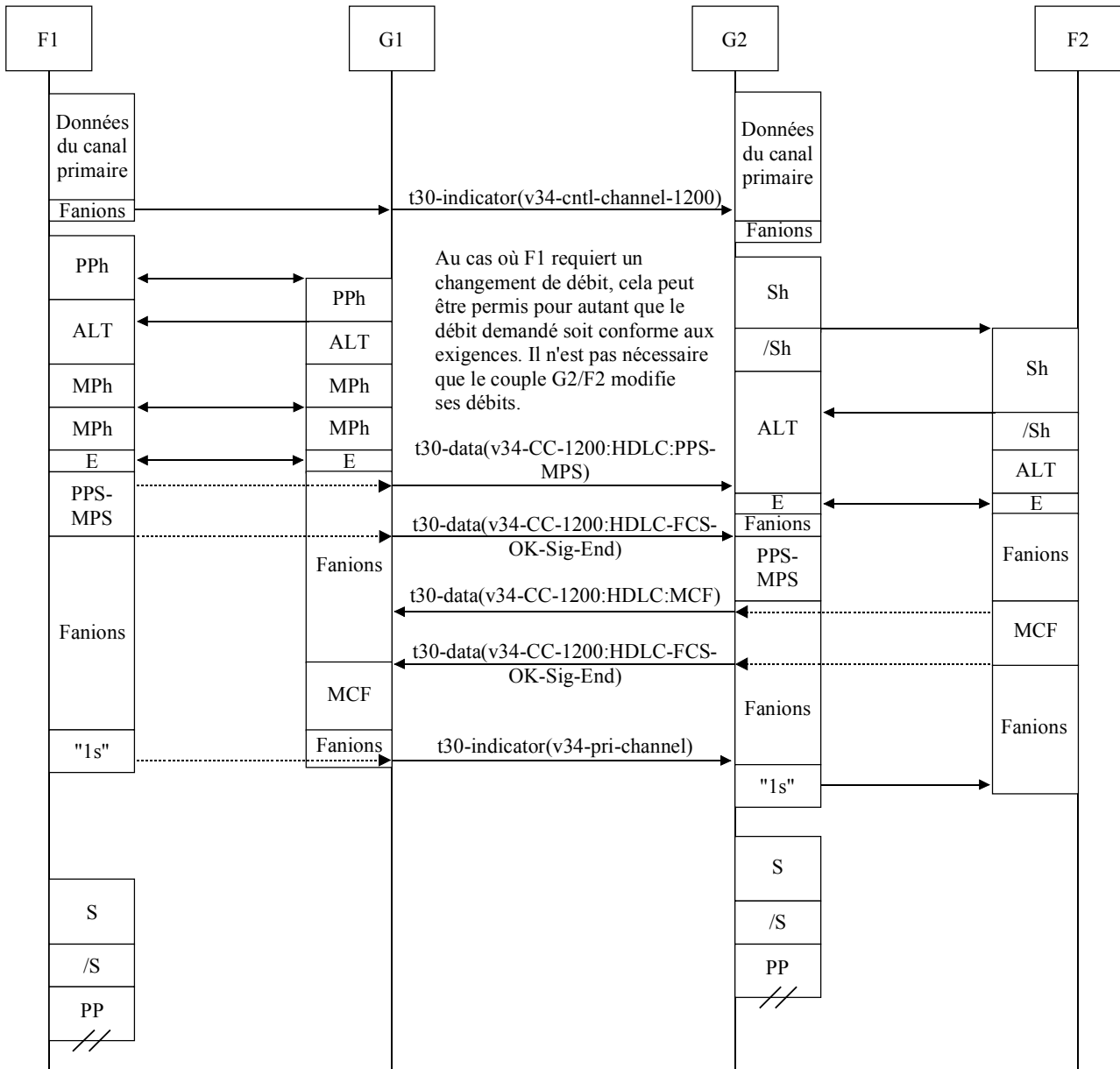
Figure IV.6/T.38 – Séquence de changement de débit quand le télécopieur G3 émetteur lance le reconditionnement
