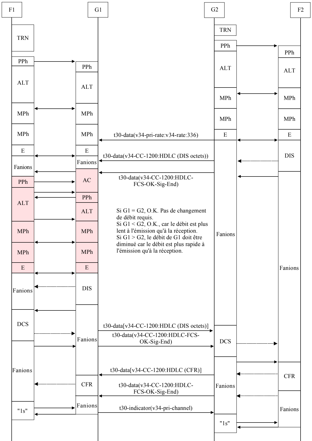
Figure IV.2/T.38 – Négociation du débit et démarrage du canal de commande
