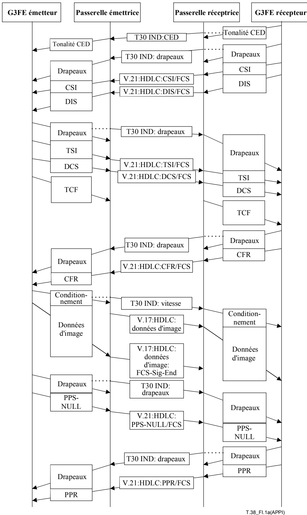
Figure I.1/T.38 – Deux dispositifs de télécopie du Groupe 3 communiquant via des passerelles (feuille 1 de 2)
