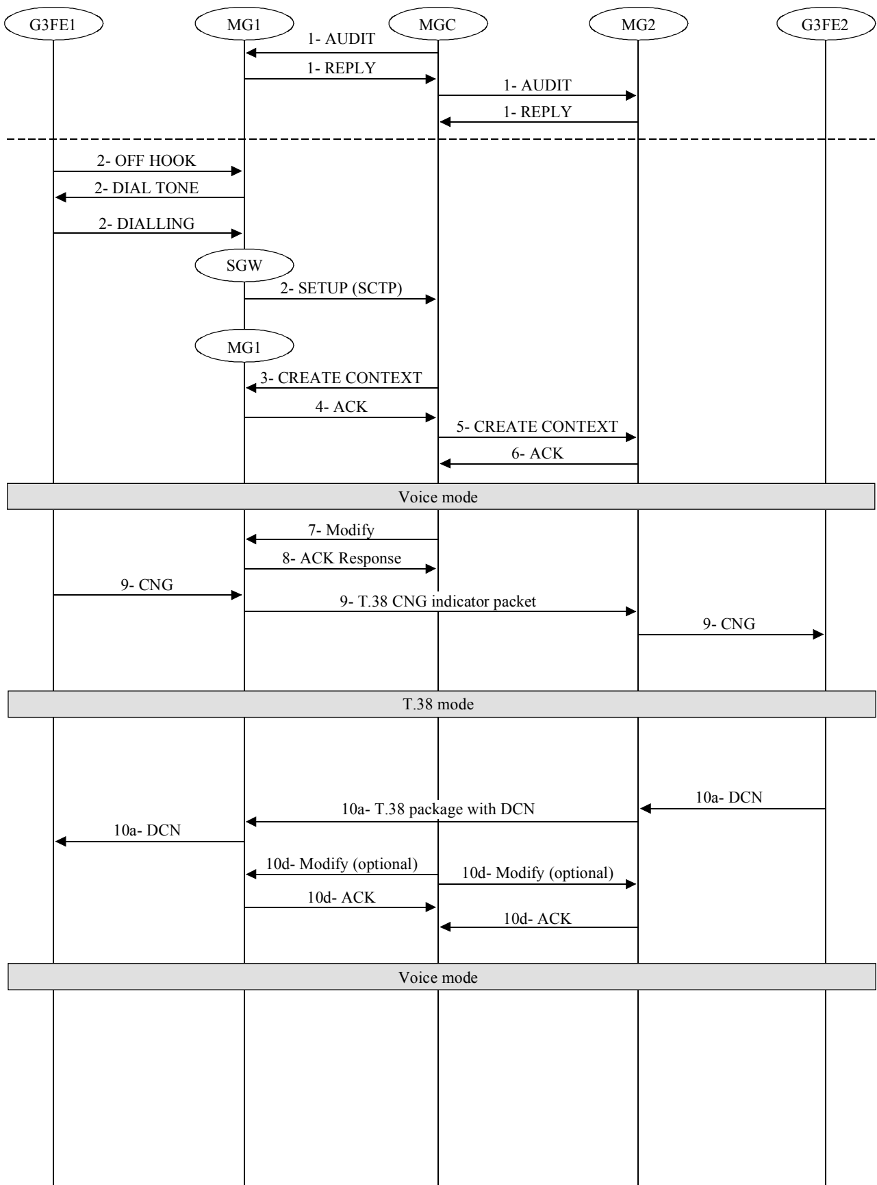
Figure III.3/T.38 – Appel vocal à télécopieur avec points d'extrémité H.248 acceptant le passage autonome entre les modes VoIP et FoIP
