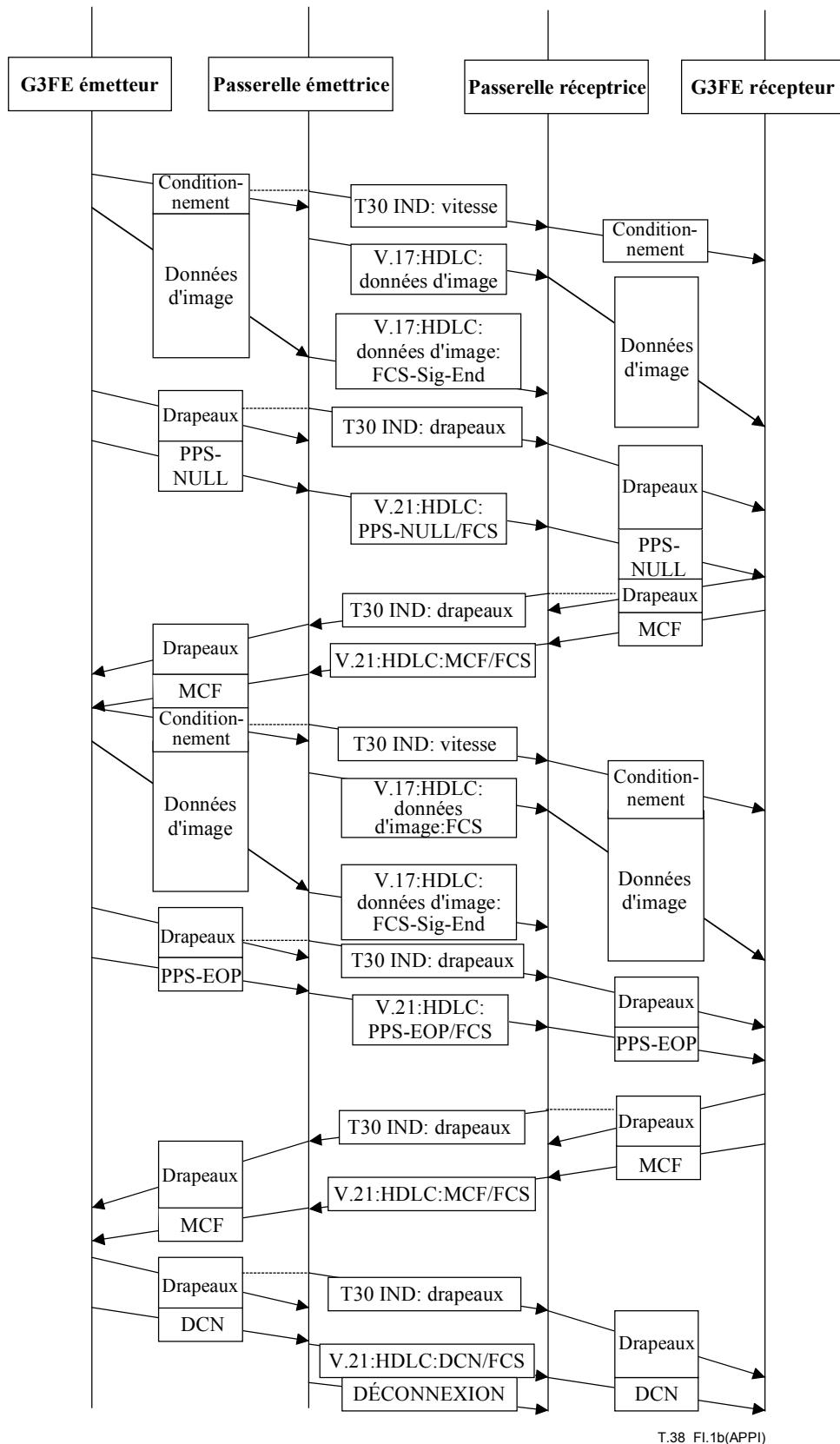
Figure I.1/T.38 – Deux dispositifs de télécopie du Groupe 3 communiquant via des passerelles (feuille 2 de 2)
