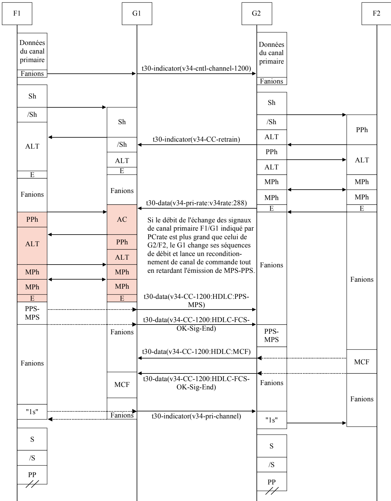
Figure IV.5/T.38 – Séquence de changement de débit quand le télécopieur G3 récepteur lance le reconditionnement
