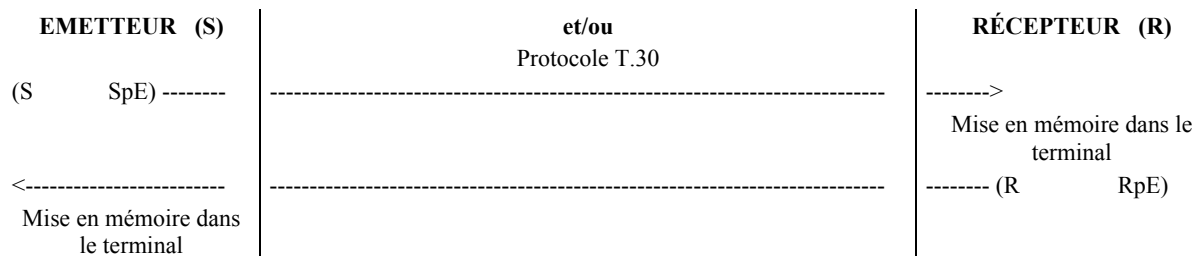
Figure H.3/T.30 – Mécanisme du mode enregistrement
