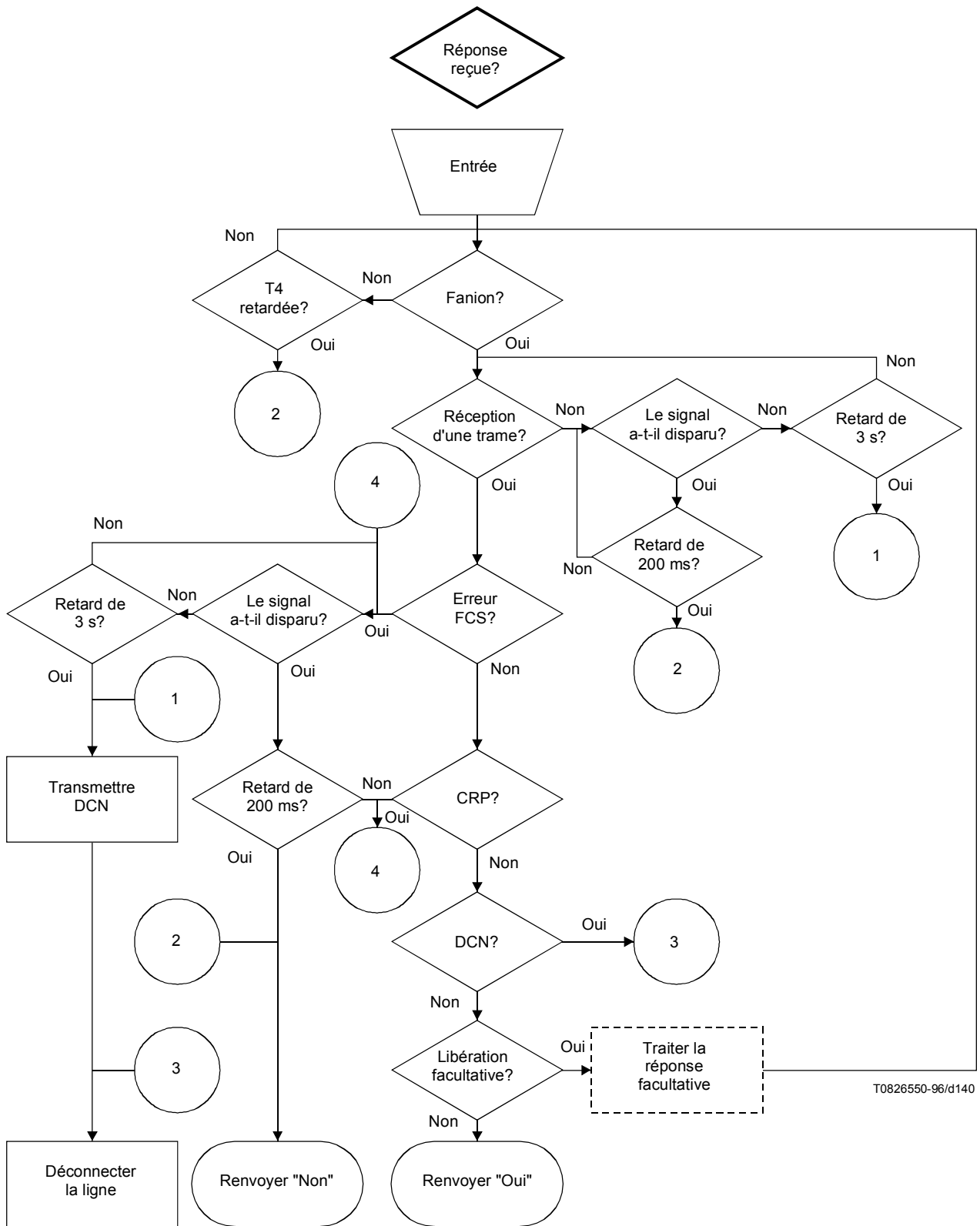
Figure G.7/T.30 (feuille 18 de 20)
