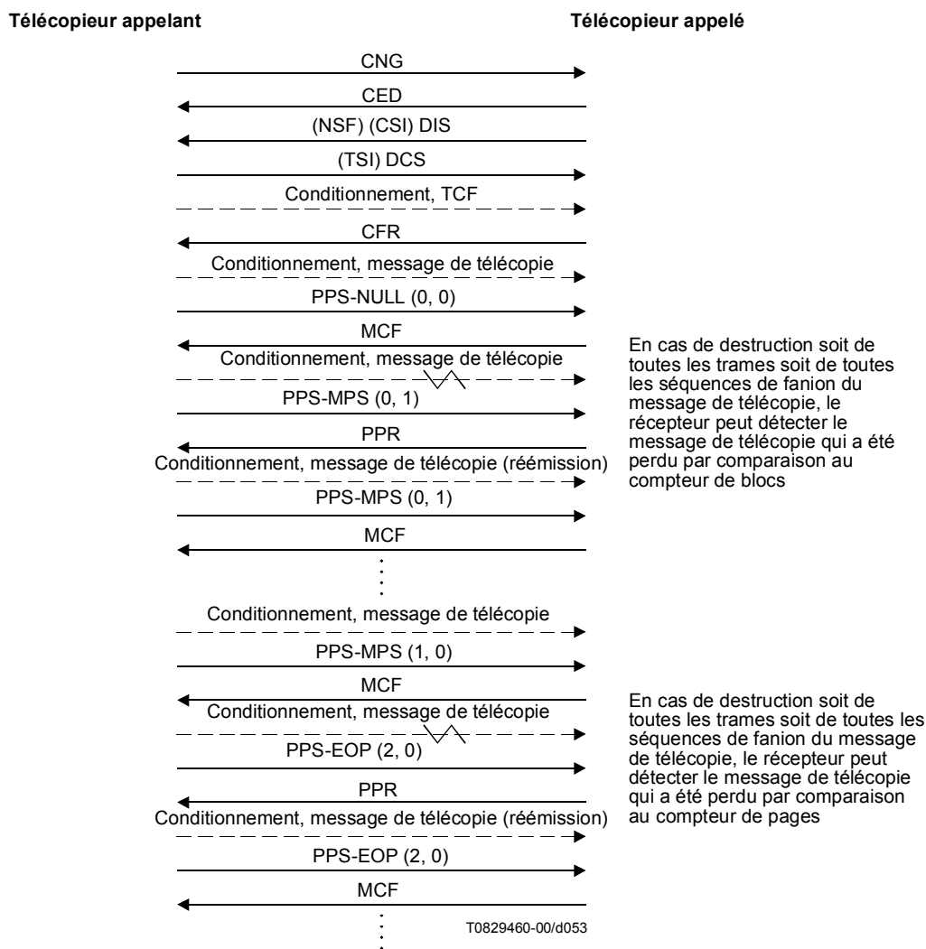
Figure A.7/T.30 (feuille 13 de 13)
