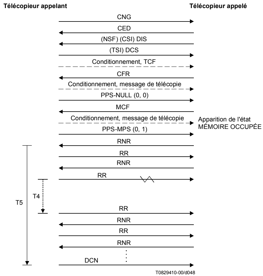
Figure A.7/T.30 (feuille 8 de 13)
