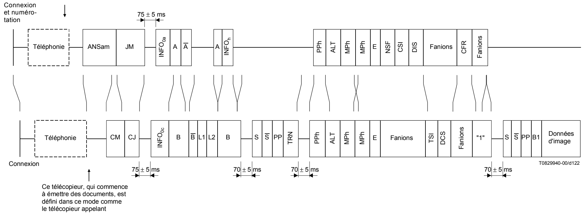
Figure F.5-14/T.30 – Communication manuelle après la phase téléphonique
