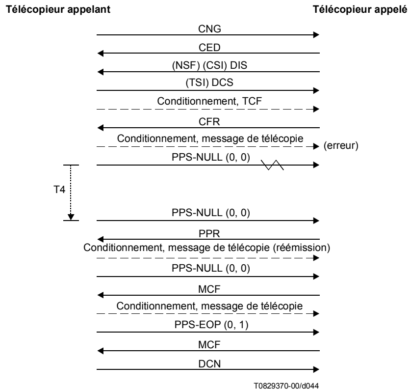
Figure A.7/T.30 (feuille 4 de 13)
