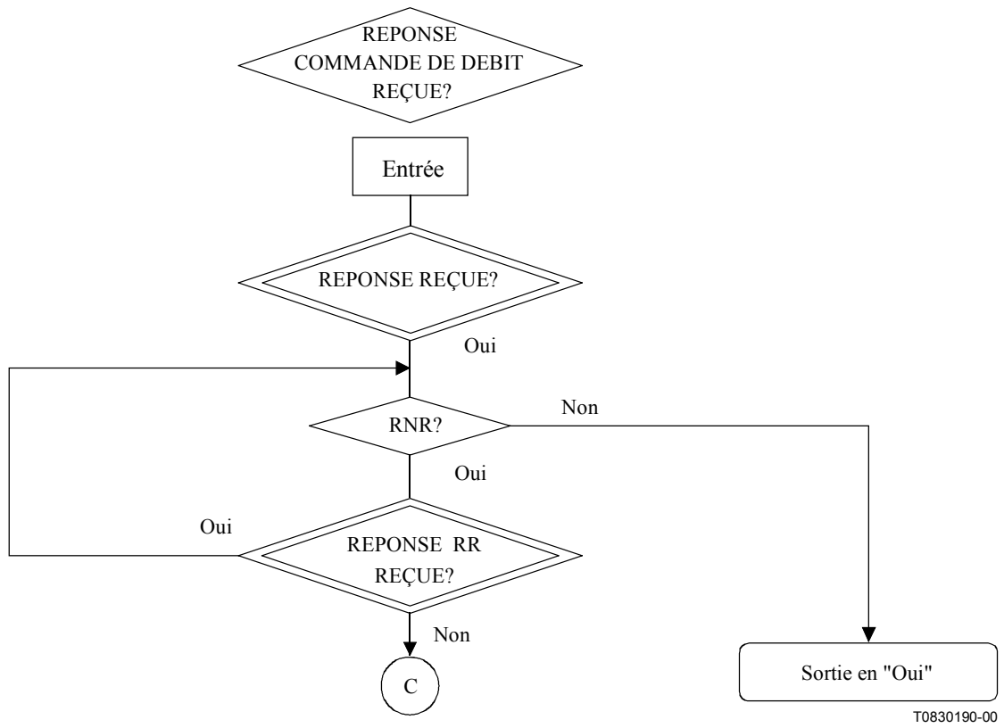
Figure 5-2w/T.30 – Réception de réponse dans le mode facultatif de commande de débit
