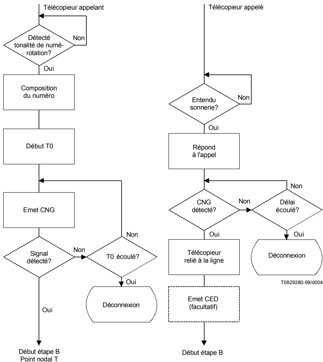
Figure 4/T.30 – Etablissement de la communication, mode opératoire 3
