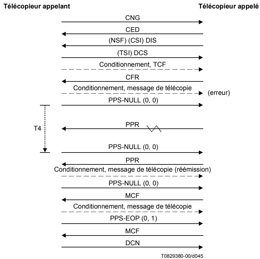
Figure A.7/T.30 (feuille 5 de 13)
