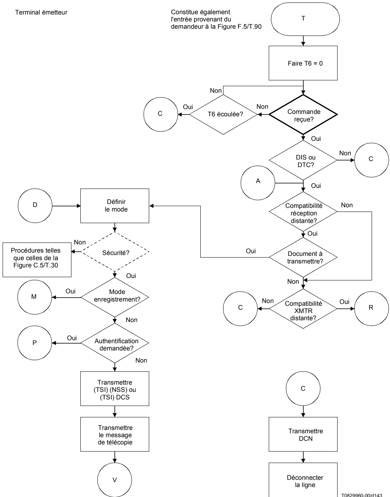
Figure G.8-1/T.30 – Mode duplex (feuille 1 de 3) (utilisée à la place de la Figure C.5)
