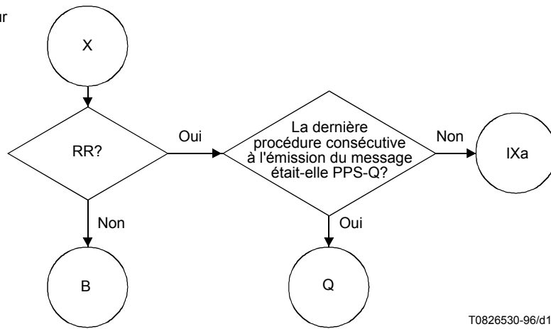
Figure G.7/T.30 (feuille 16 de 20)
