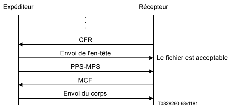
Figure V.4/T.30 – Fichier transmis acceptable pour un récepteur
