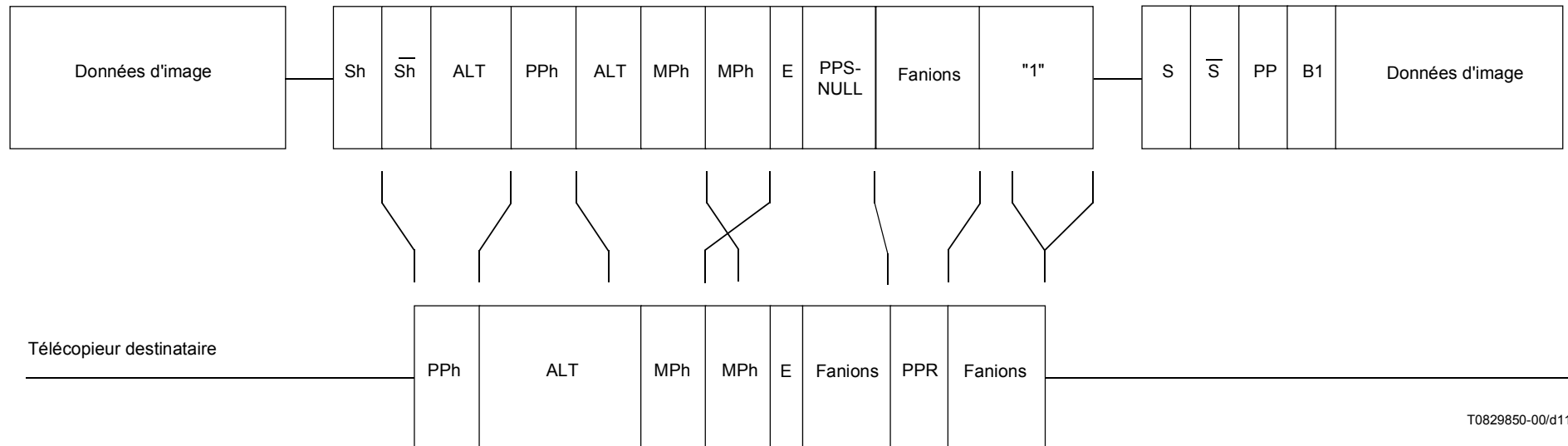
Figure F.5-6/T.30 – Changement du débit de données entre pages partielles
