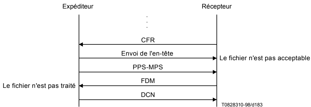
Figure V.6/T.30 – Fichier transmis non traité par un expéditeur
