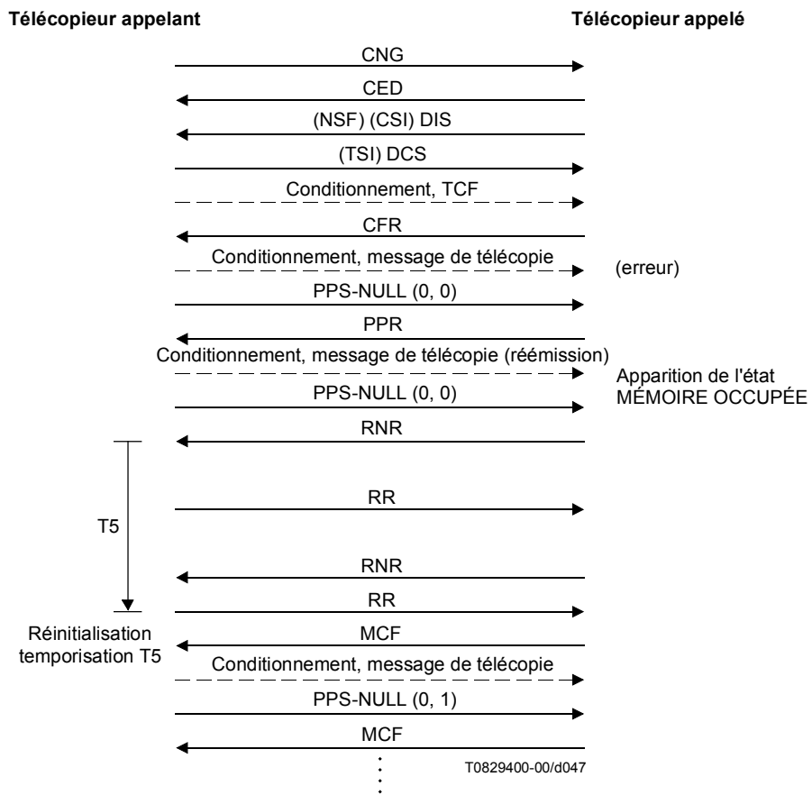
Figure A.7/T.30 (feuille 7 de 13)
