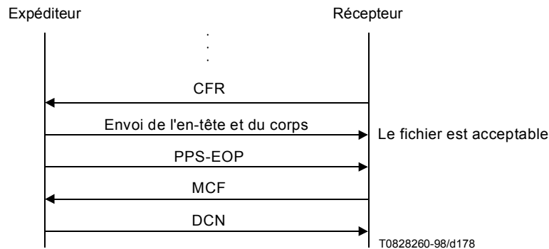
Figure V.1/T.30 – Fichier émis acceptable par un récepteur
