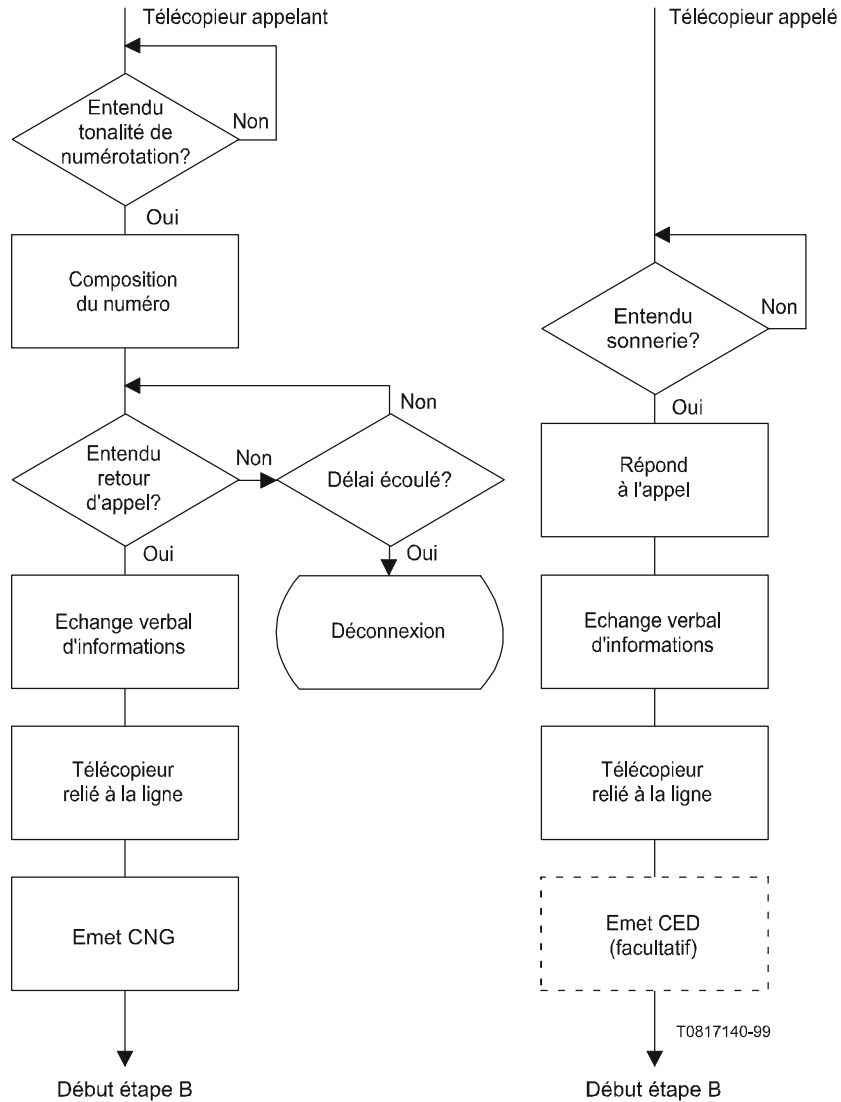
Figure 2/T.30 – Etablissement de la communication, mode opératoire 1
