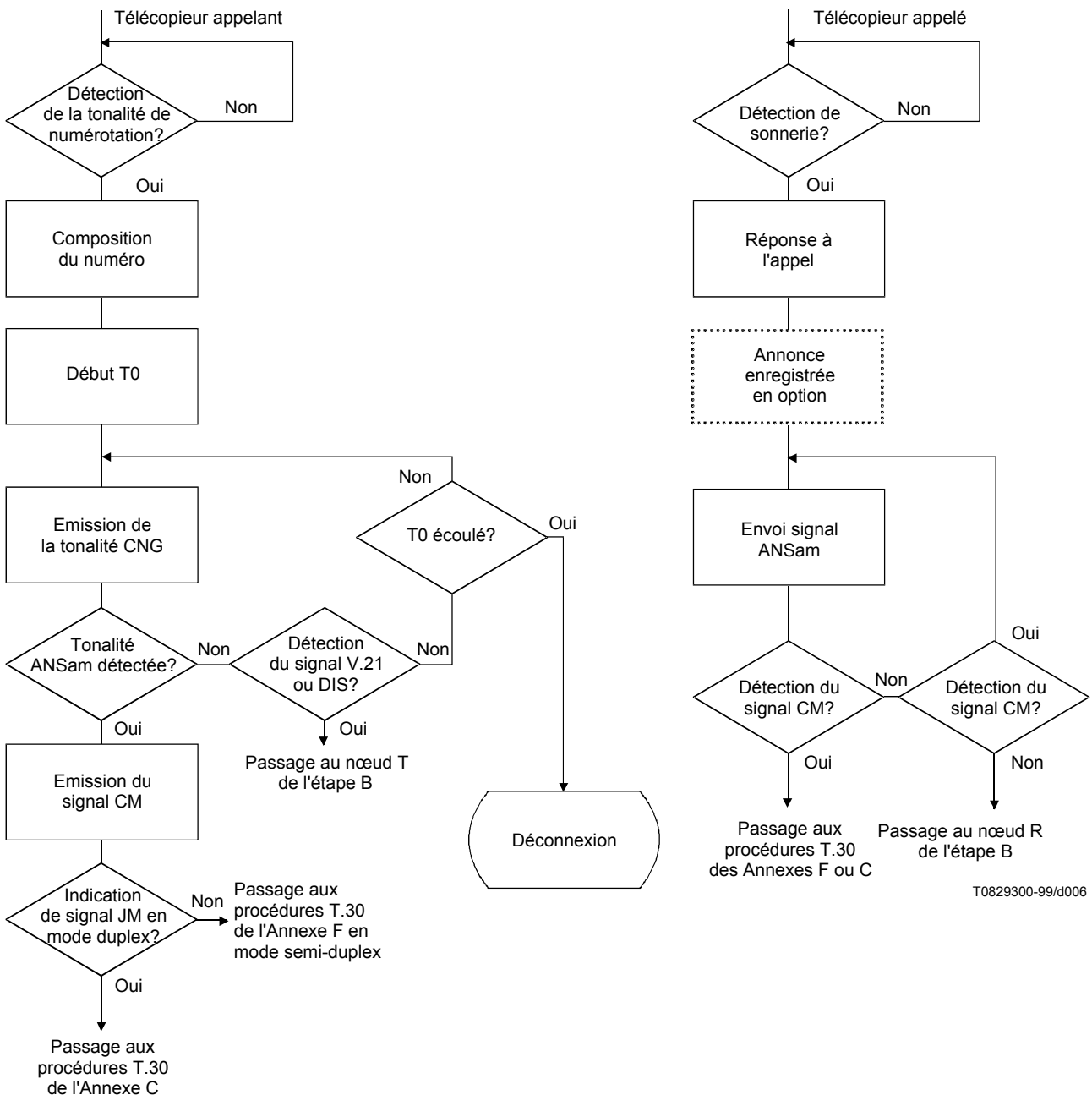
Figure 6a/T.30 – Etablissement de l'appel, méthode de fonctionnement 4 bis a
