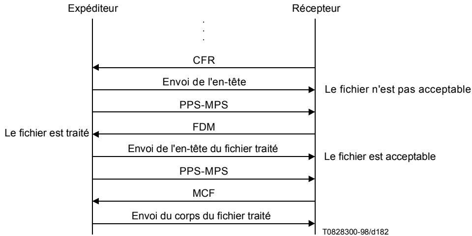
Figure V.5/T.30 – Fichier transmis traité par un expéditeur
