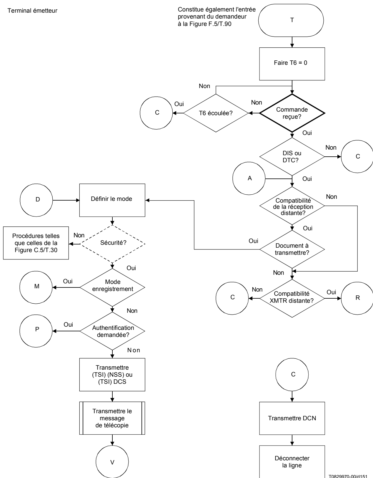
Figure G.8-5/T.30 – Mode duplex (feuille 1 de 3) (utilisée à la place de la Figure C.14)
