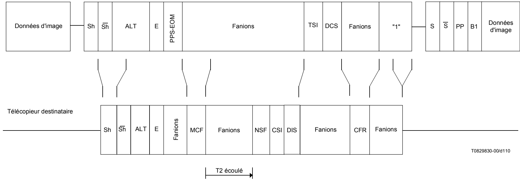
Figure F.5-4/T.30 – Changement de mode (sans changement de débit de données)
