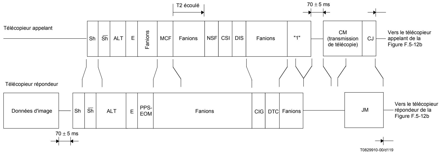
Figure F.5-12a/T.30 – Relève successive à une émission (passage du mode relève au mode émission dans le terminal appelant [1/2])
