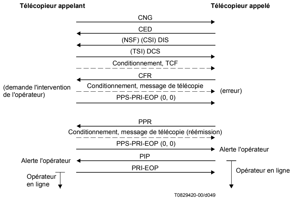
Figure A.7/T.30 (feuille 9 de 13)
