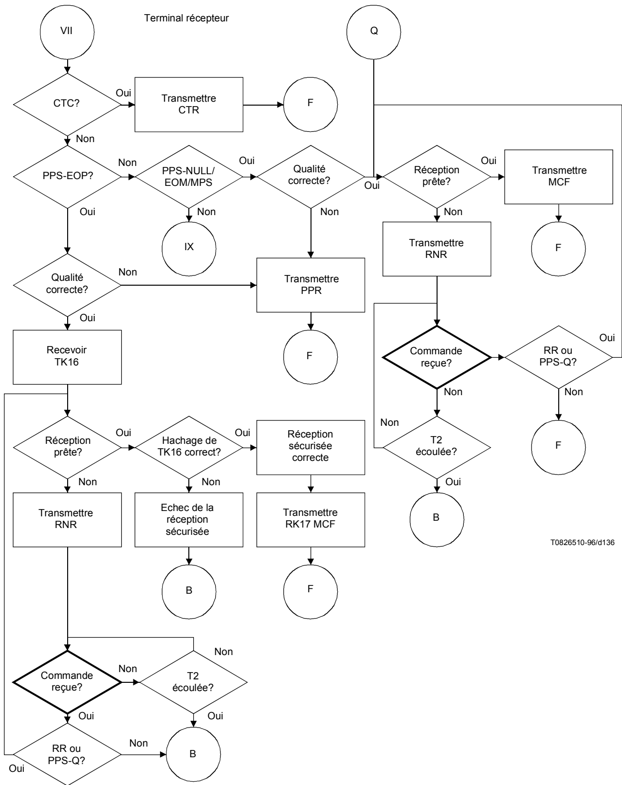
Figure G.7/T.30 (feuille 14 de 20)
