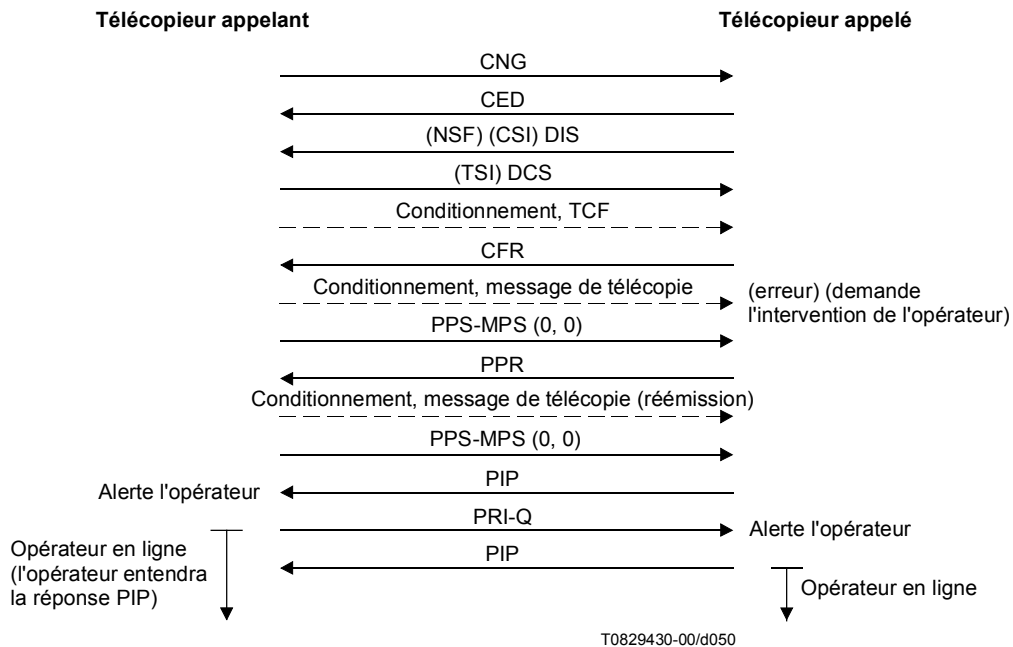
Figure A.7/T.30 (feuille 10 de 13)
