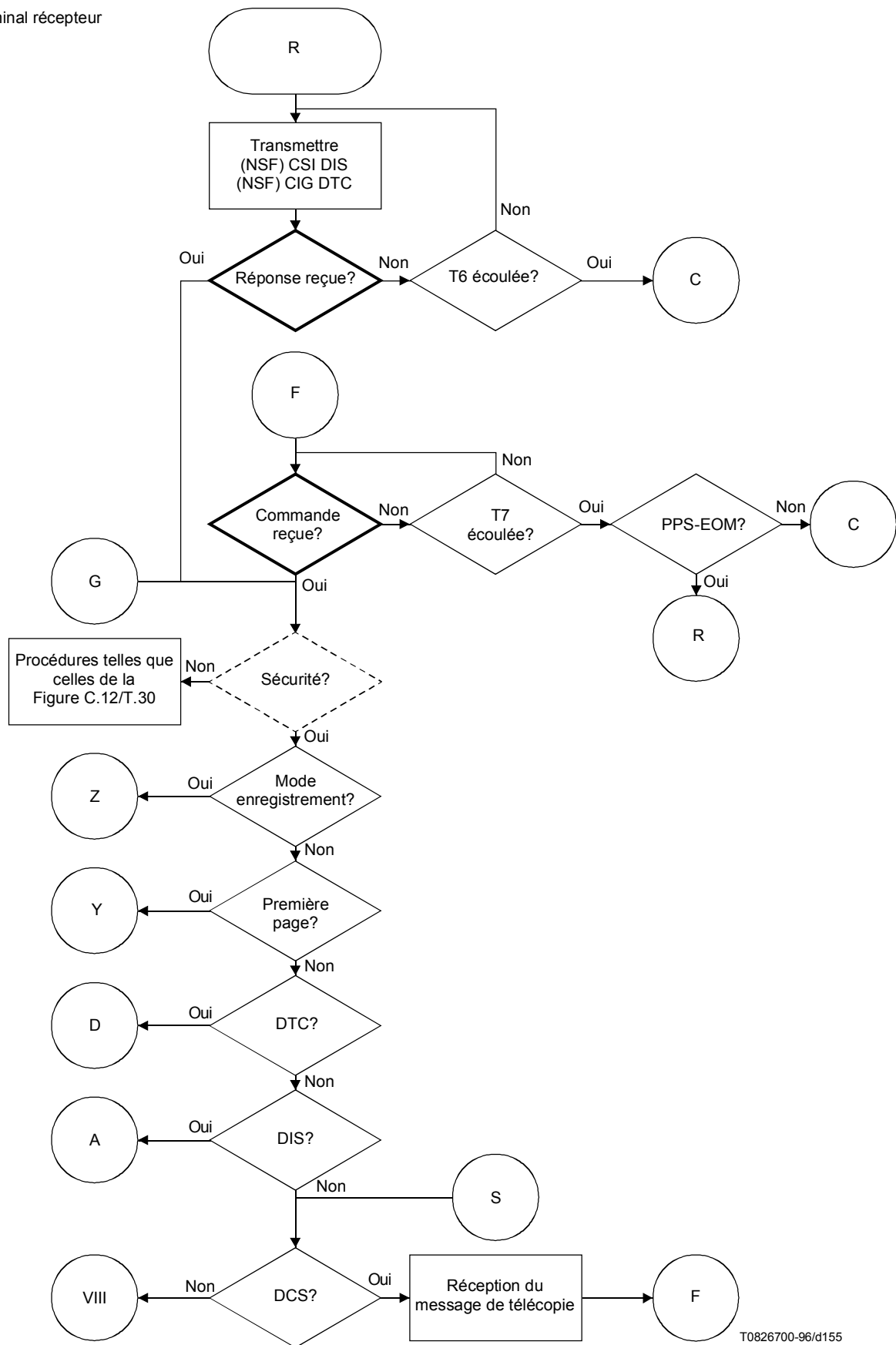
Figure G.8-7/T.30 – Mode duplex (utilisée à la place de la Figure C.21)
