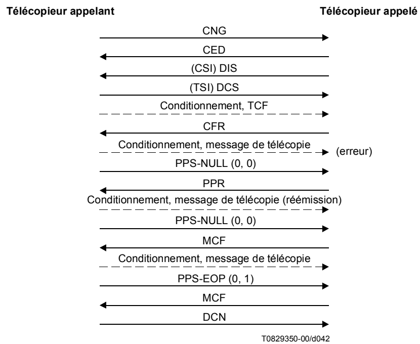
Figure A.7/T.30 (feuille 2 de 13)
