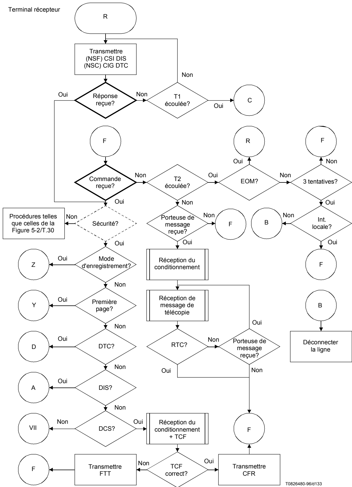
Figure G.7/T.30 (feuille 11 de 20)
