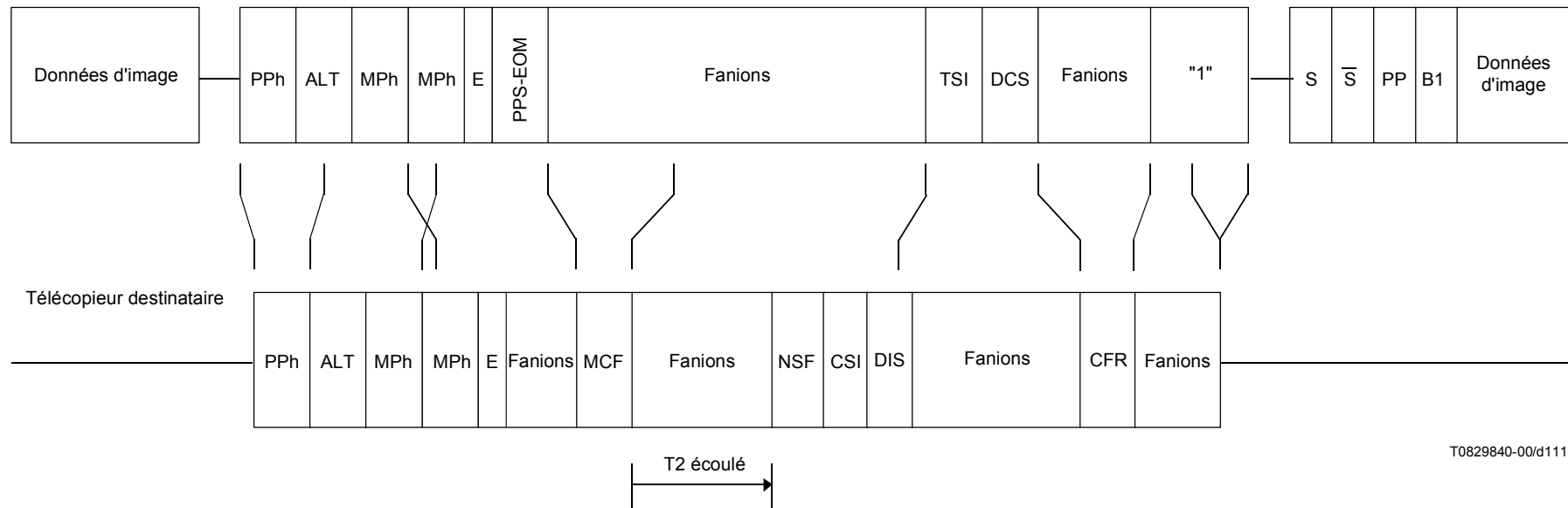
Figure F.5-5/T.30 – Changement de mode (avec changement du débit des données provenant du télécopieur émetteur)
