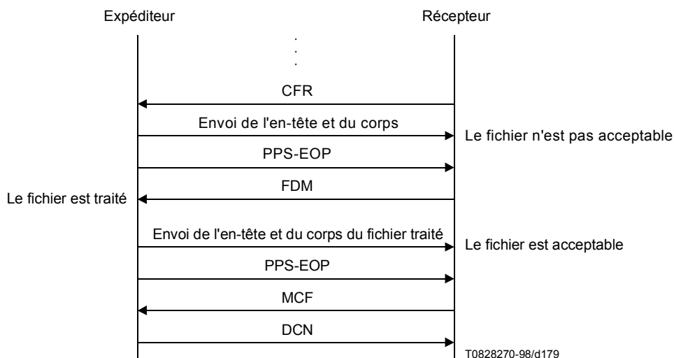
Figure V.2/T.30 – Fichier transmis traité par un expéditeur
