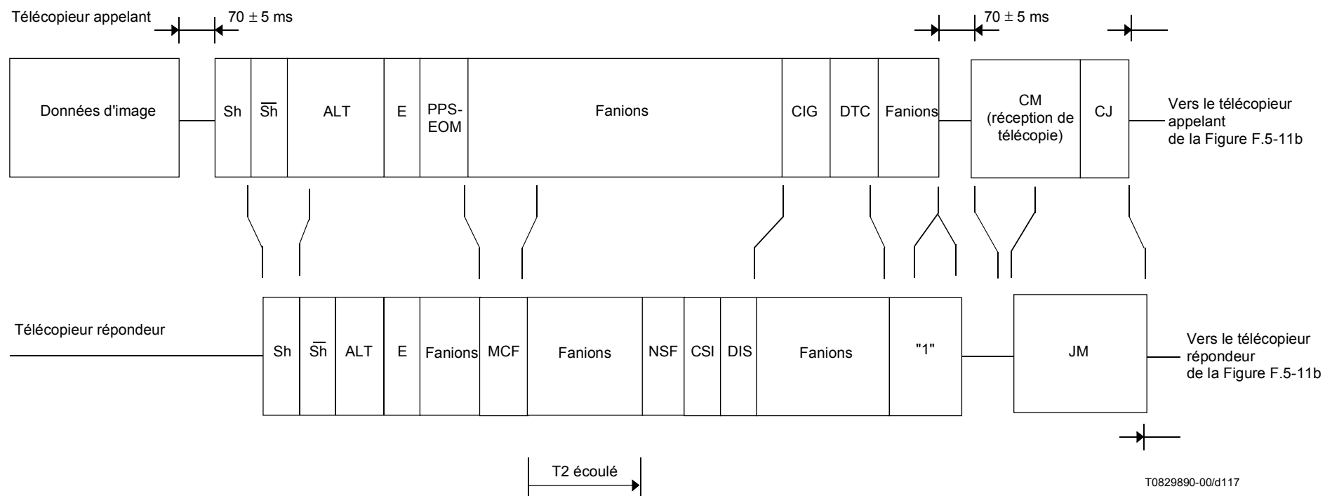
Figure F.5-11a/T.30 – Relève successive à une émission (passage du mode émission au mode relève dans le terminal appelant [1/2])
