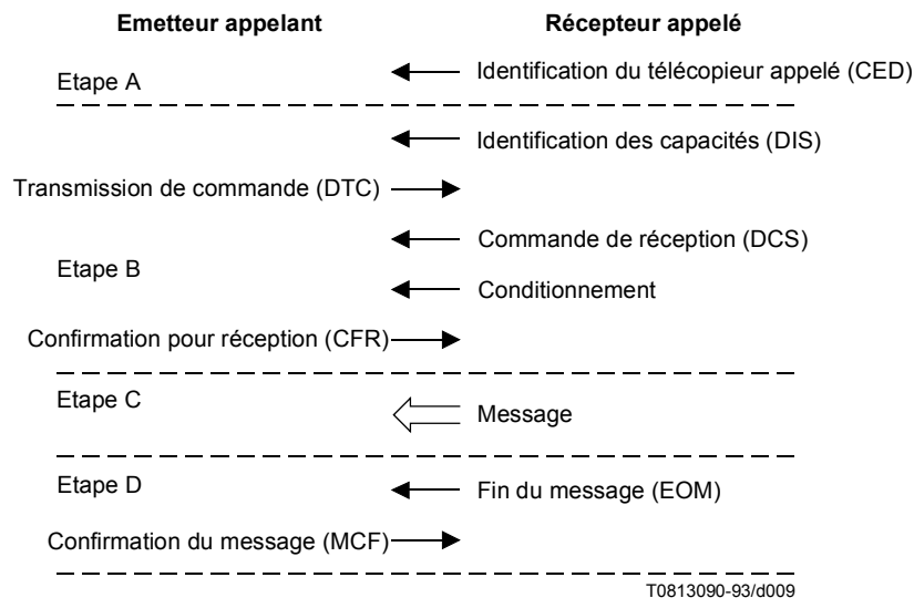
Figure 8/T.30 – Le télécopieur appelant reçoit
