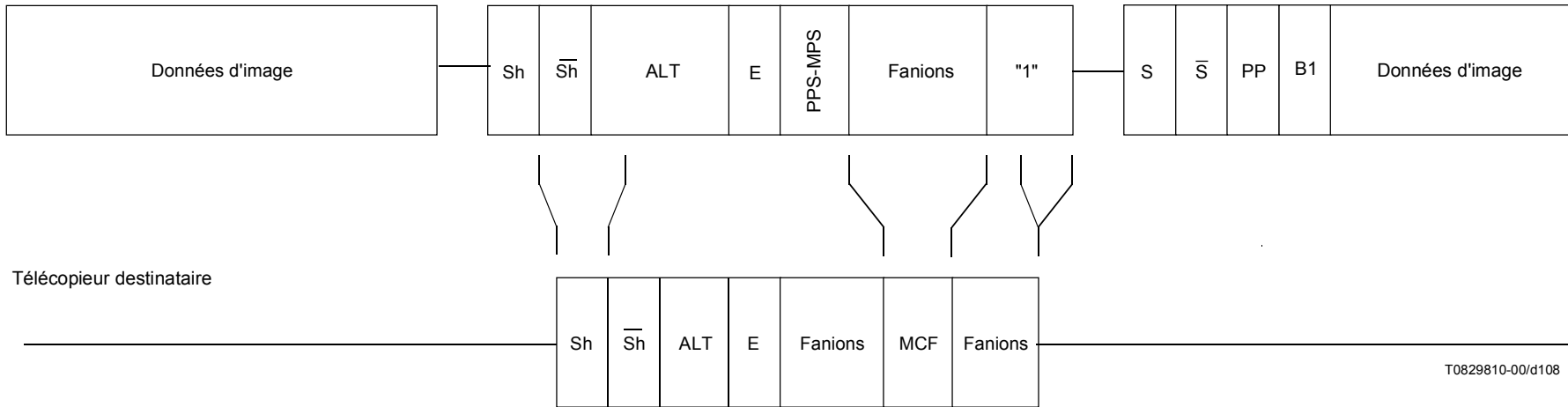
Figure F.5-2/T.30 – Entre pages
