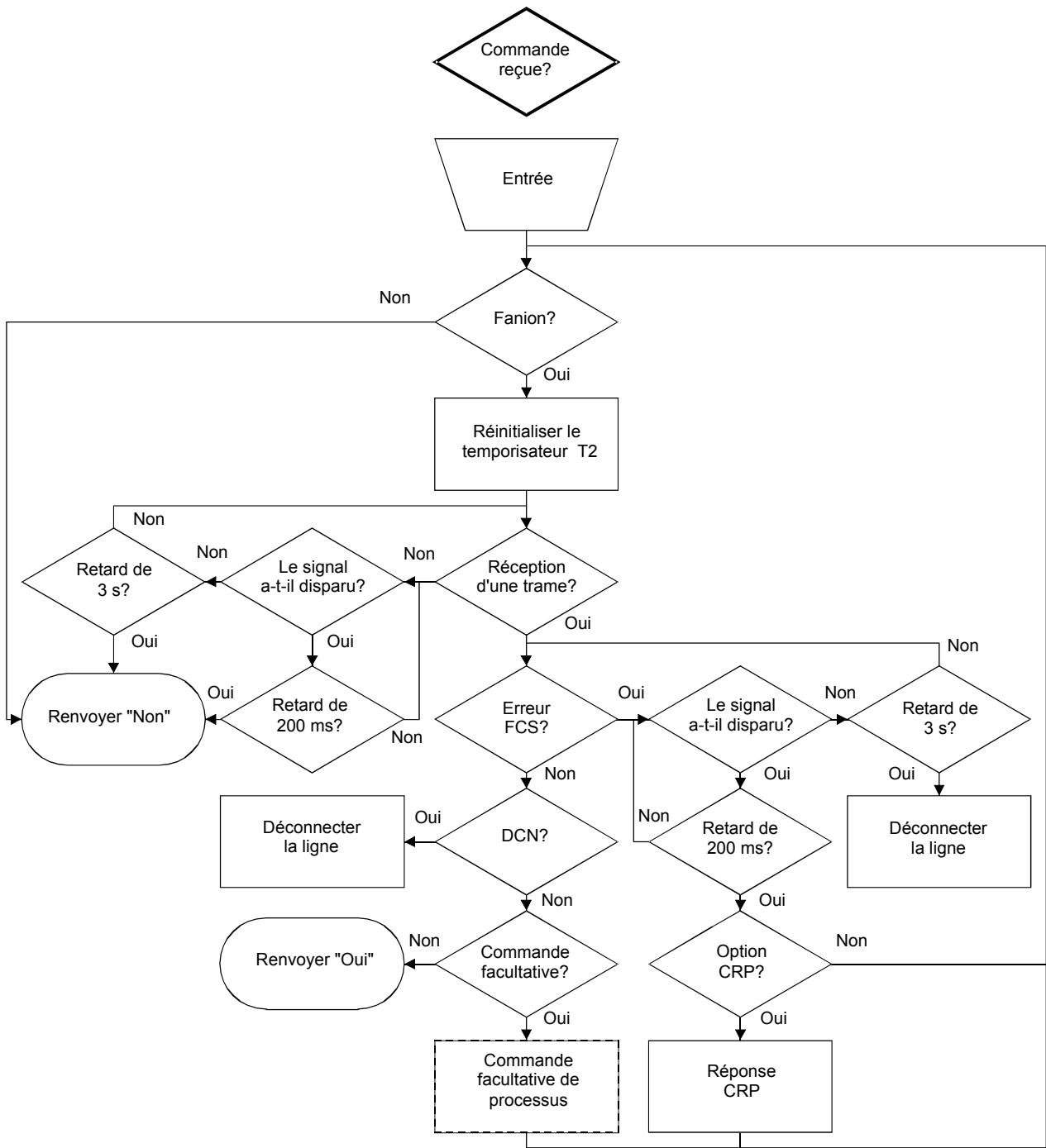
Figure G.7/T.30 (feuille 17 de 20)
