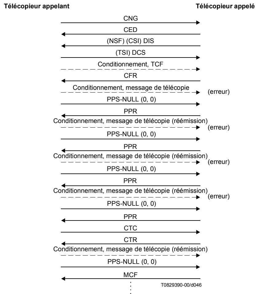
Figure A.7/T.30 (feuille 6 de 13)
