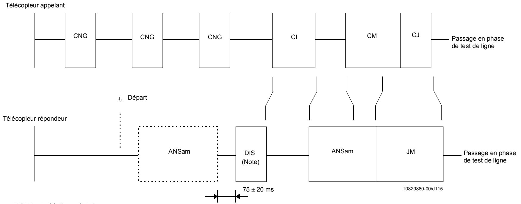
Figure F.5-9/T.30 – Réception manuelle
