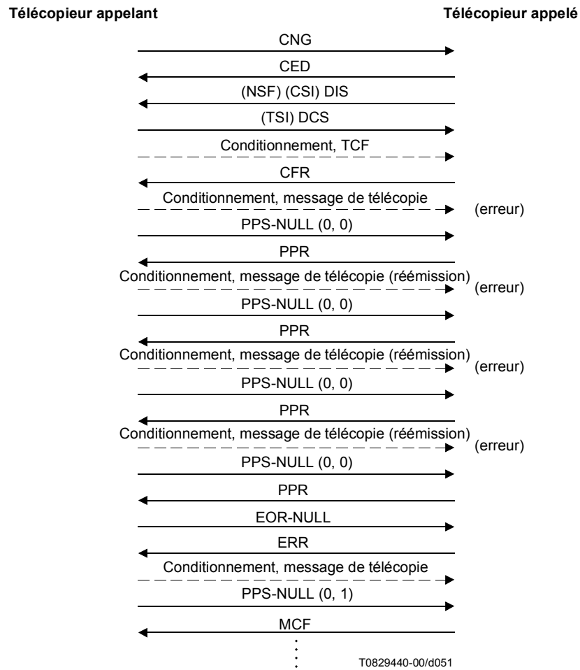
Figure A.7/T.30 (feuille 11 de 13)
