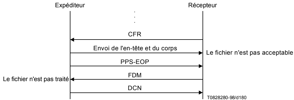
Figure V.3/T.30 – Fichier transmis non traité par un expéditeur
