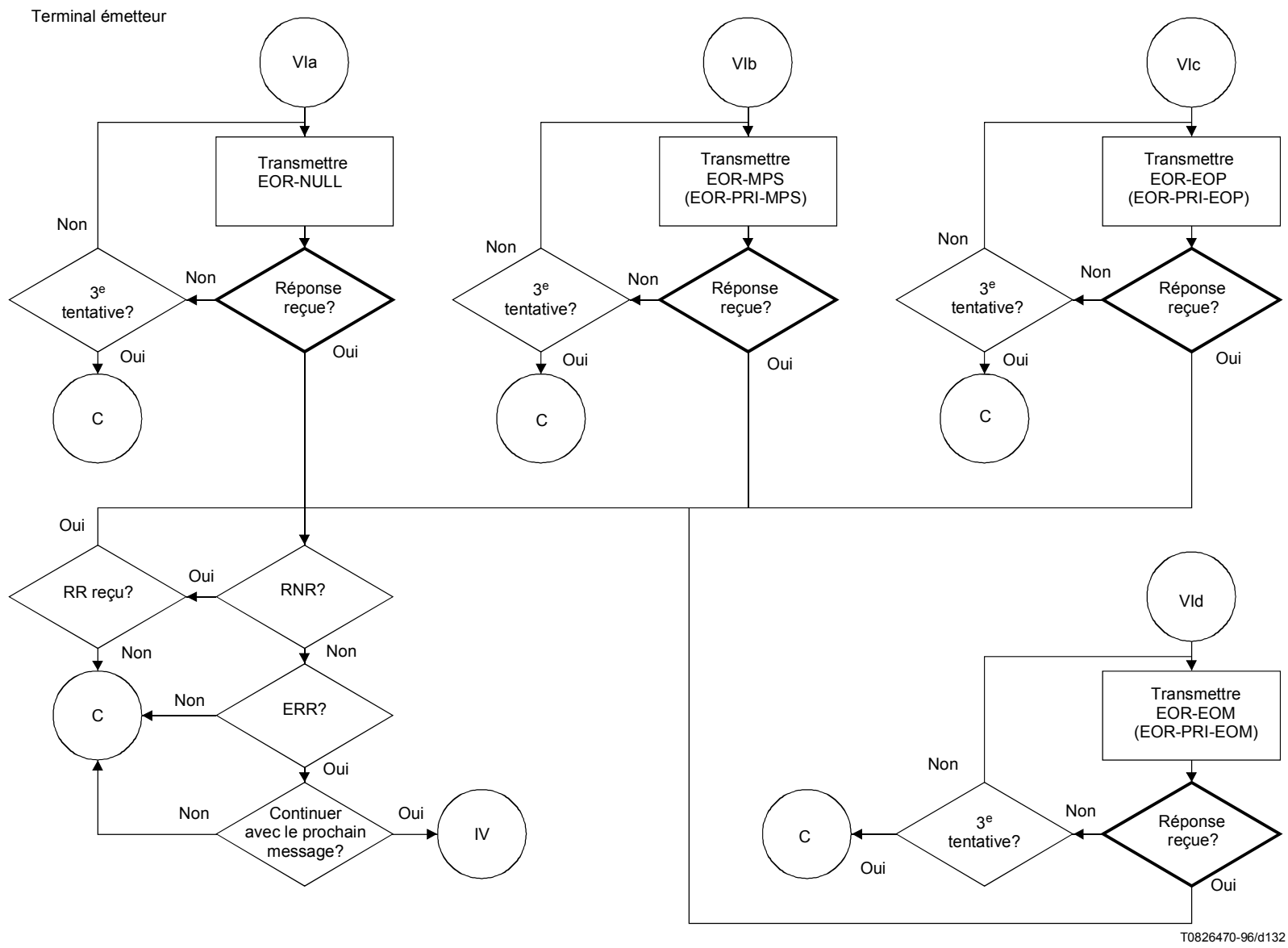
Figure G.7/T.30 (feuille 10 de 20)
