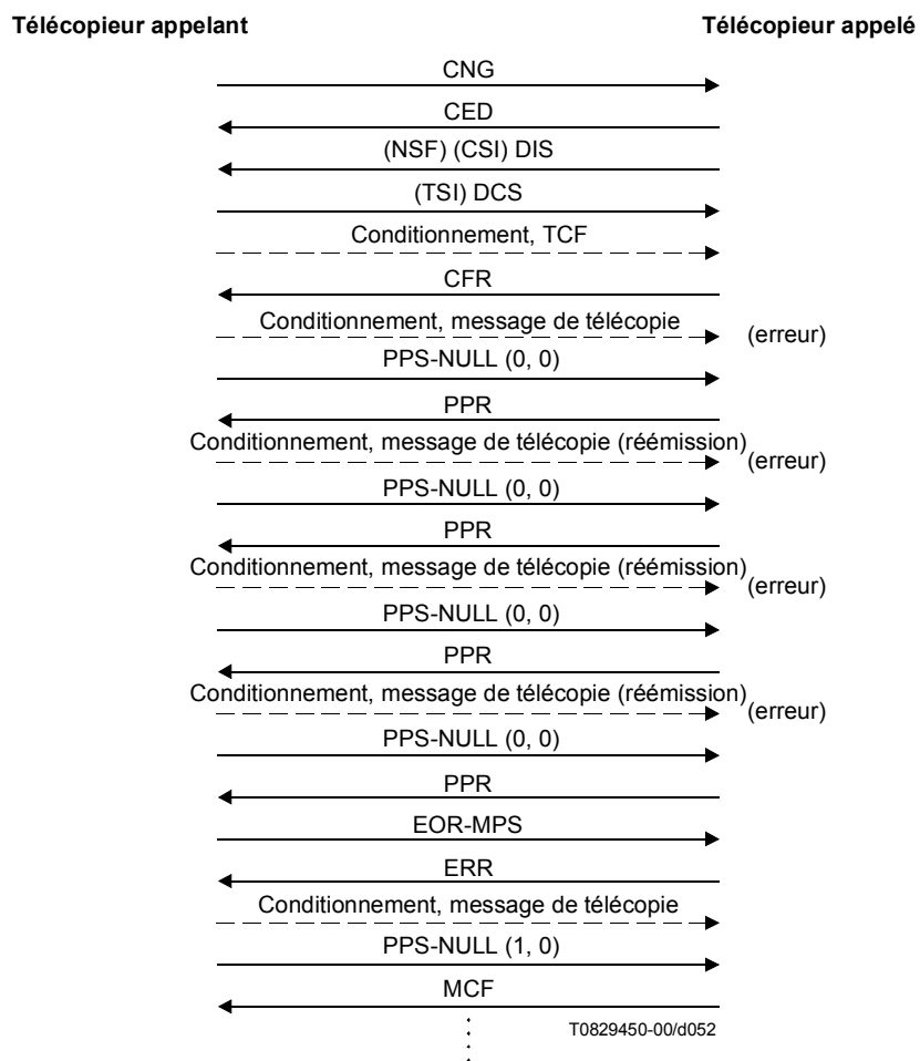
Figure A.7/T.30 (feuille 12 de 13)
