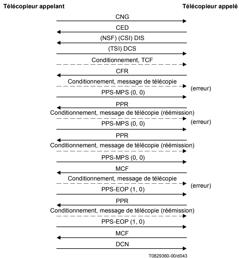
Figure A.7/T.30 (feuille 3 de 13)
