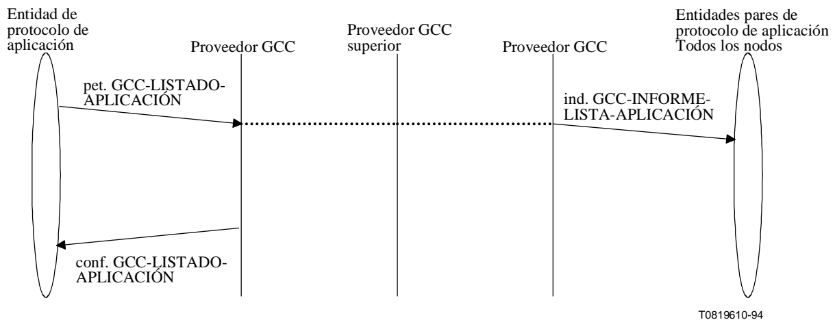
Figura 7-19/T.124 – GCC-LISTADO-APLICACIÓN – Secuencia de primitivas
