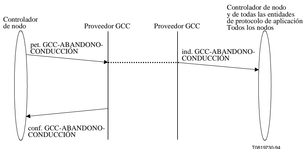
Figura 7-31/T.124 – GCC-ABANDONO-CONDUCCIÓN (iniciada por el usuario) – Secuencia de primitivas
