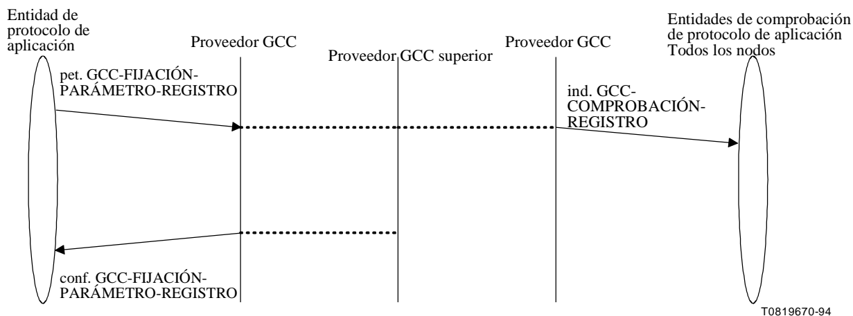
Figura 7-25/T.124 – GCC-FIJACIÓN-PARÁMETRO-REGISTRO – Secuencia de primitivas
