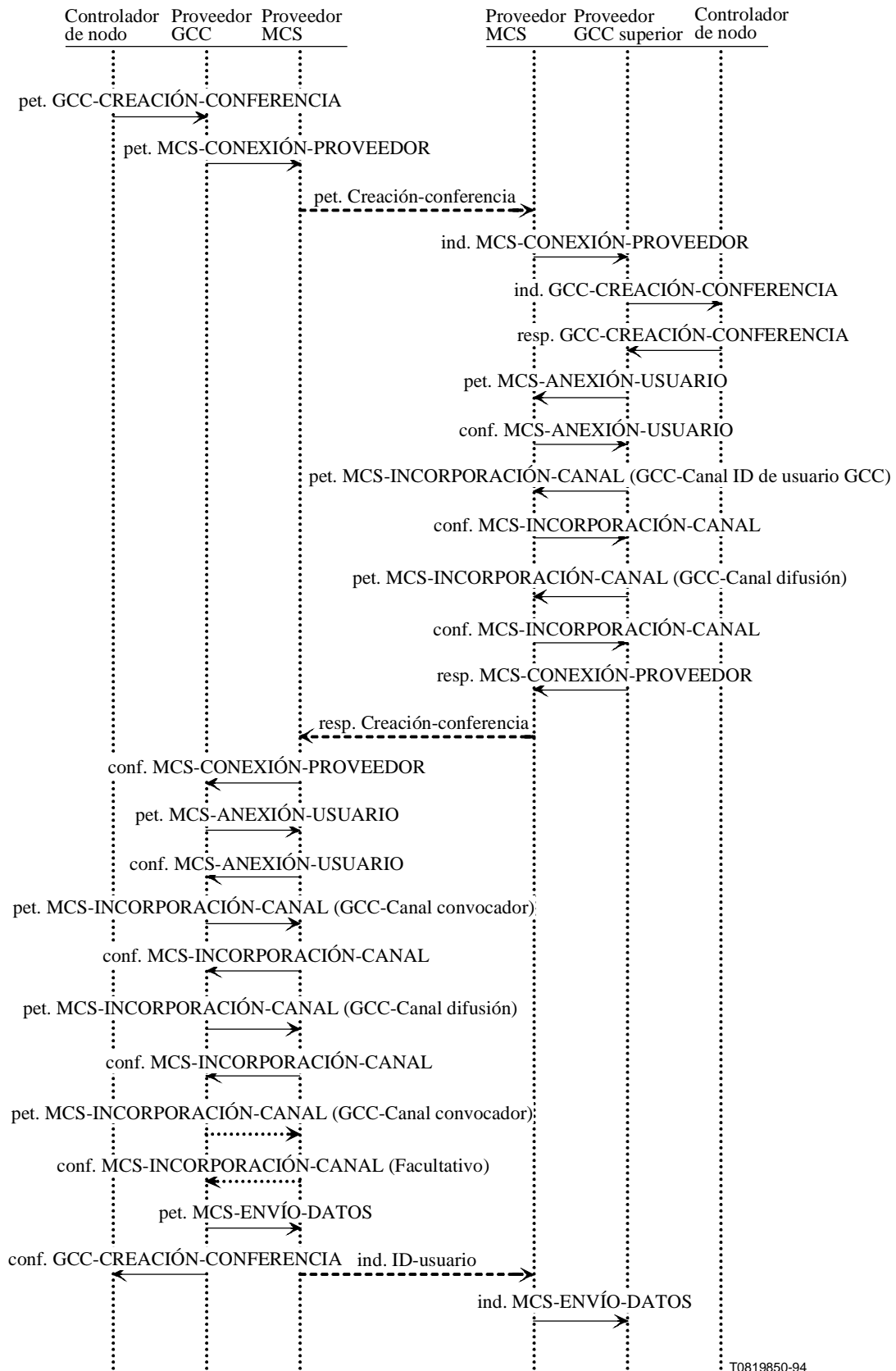
Figura 8-1/T.124 – Cómo se crea una conferencia
