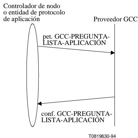
Figura 7-21/T.124 – GCC-PREGUNTA-LISTA-APLICACIÓN – Secuencia de primitivas
