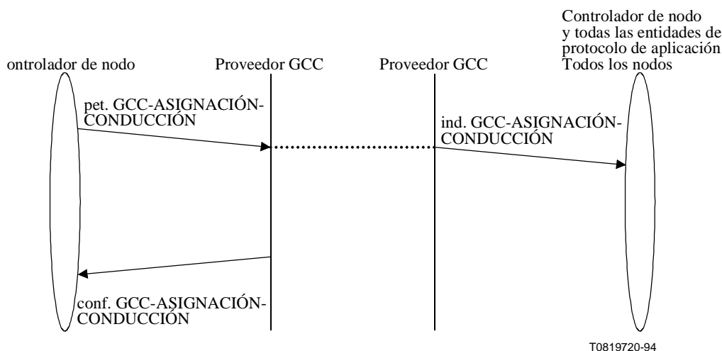
Figura 7-30/T.124 – GCC-ASIGNACIÓN-CONDUCCIÓN – Secuencia de primitivas
