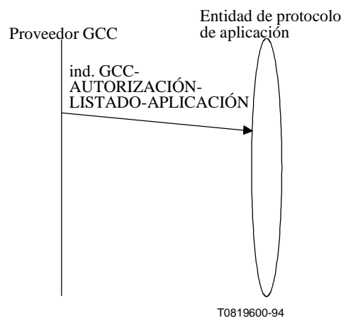
Figura 7-18/T.124 – GCC-AUTORIZACIÓN-LISTADO-APLICACIÓN – Secuencia de primitivas
