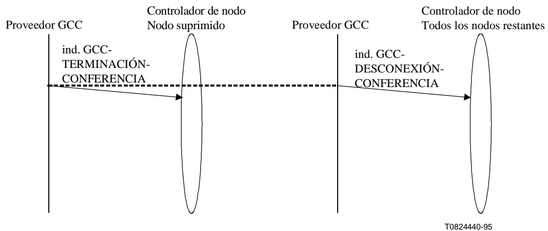
Figura 7-11/T.124 – GCC-TERMINACIÓN-CONFERENCIA (terminación por error) – Secuencia de primitivas
