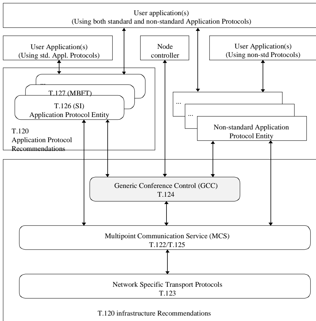
Figura 1-1/T.124 – Alcance de la Recomendación T.124
