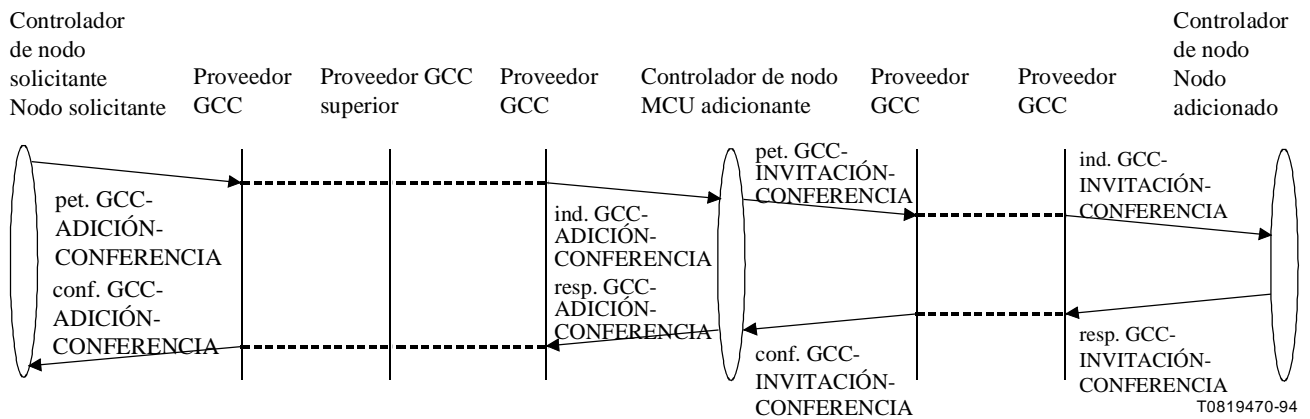
Figura 7-5/T.124 – GCC-ADICIÓN-CONFERENCIA (caso directo) – Secuencia de primitivas
