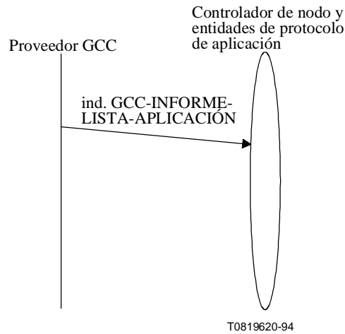
Figura 7-20/T.124 – GCC-INFORME-LISTA-APLICACIÓN – Secuencia de primitivas
