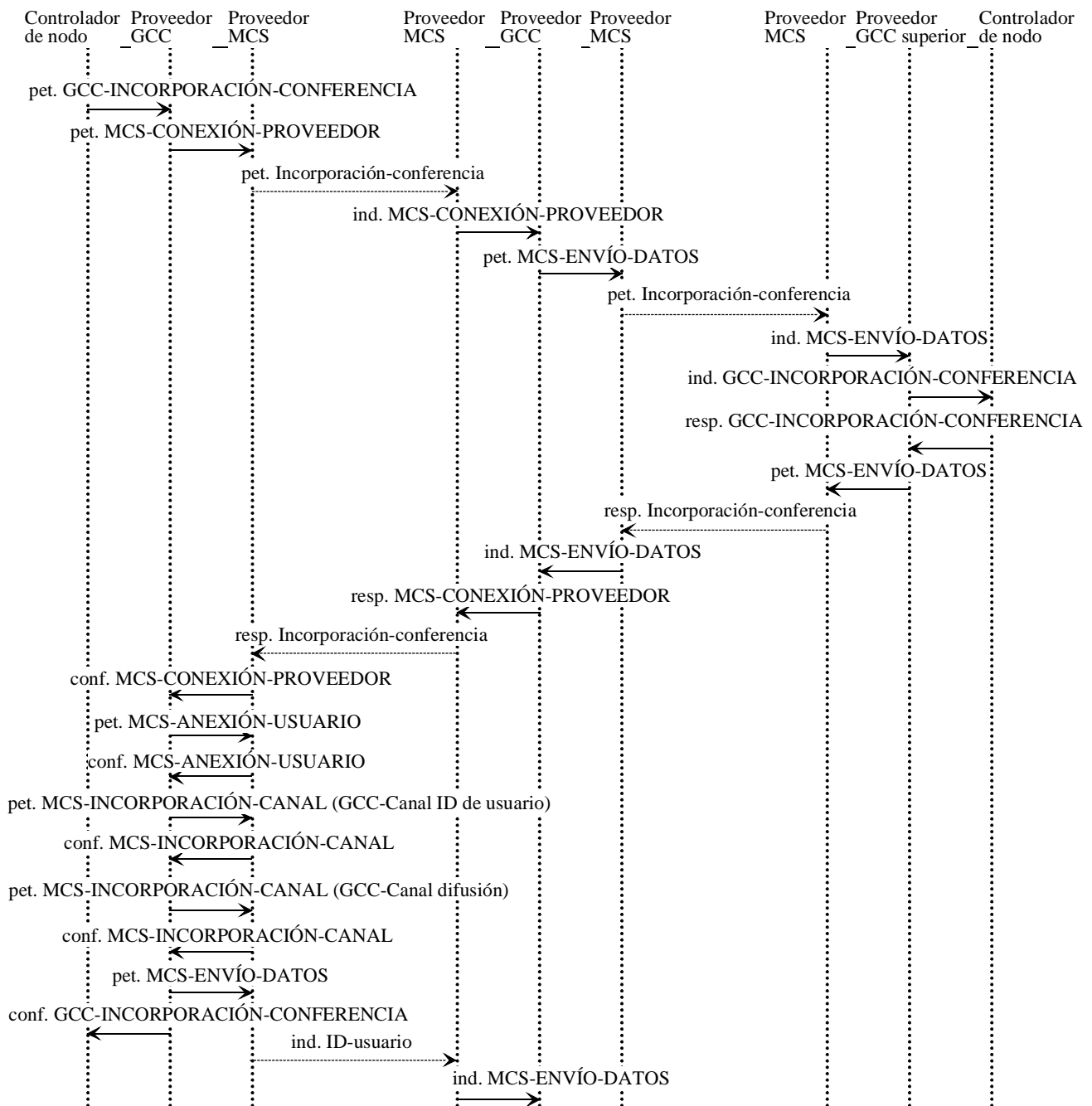
Figura 8-3/T.124 – Cómo incorporarse a una conferencia sin conexión directa al proveedor GCC superior
