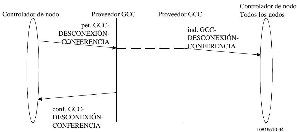
Figura 7-9/T.124 – GCC-DESCONEXIÓN-CONFERENCIA (iniciada por el cliente) – Secuencia de primitivas
