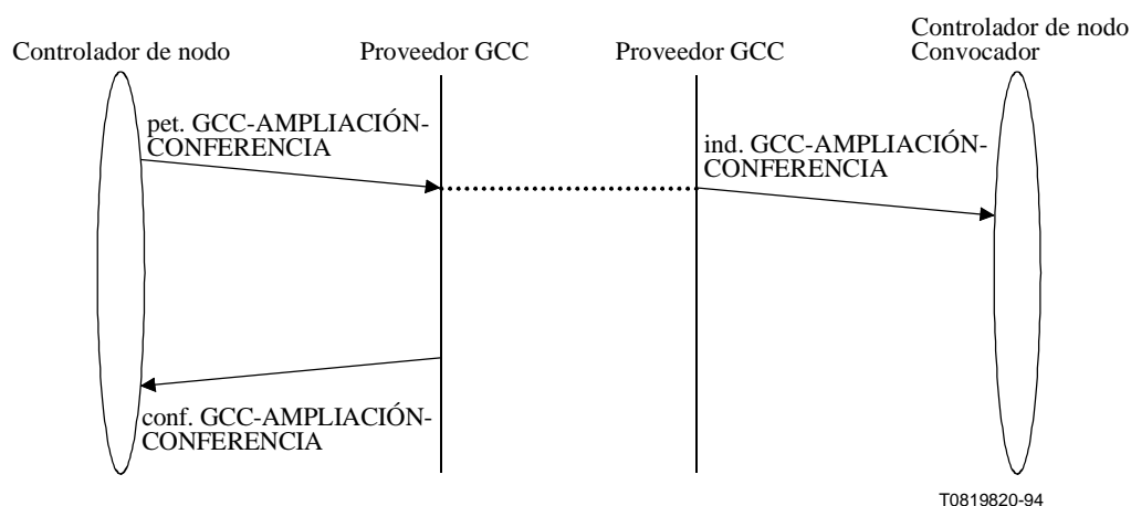
Figura 7-40/T.124 – GCC-AMPLIACIÓN-CONFERENCIA – Secuencia de primitivas
