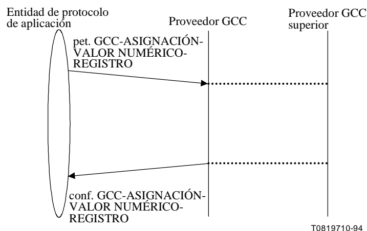
Figura 7-29/T.124 – GCC-ASIGNACIÓN-VALOR NUMÉRICO-REGISTRO – Secuencia de primitivas
