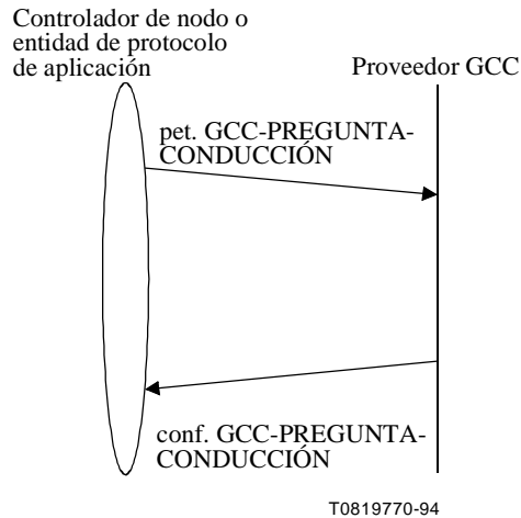
Figura 7-35/T.124 – GCC-PREGUNTA-CONDUCCIÓN – Secuencia de primitivas
