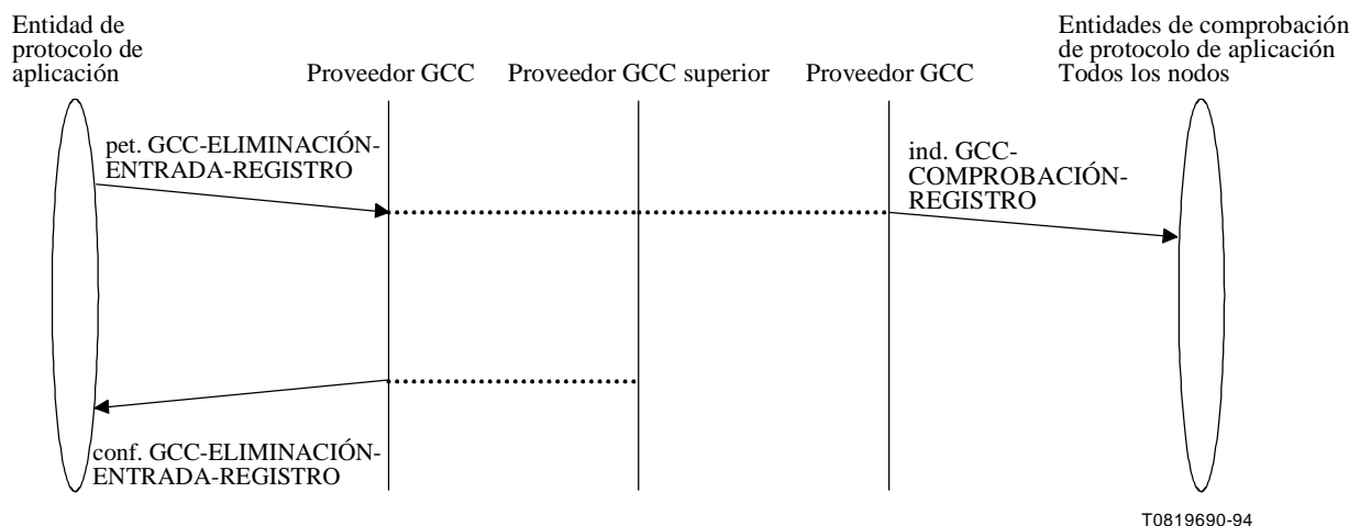
Figura 7-27/T.124 – GCC-ELIMINACIÓN-ENTRADA-REGISTRO – Secuencia de primitivas
