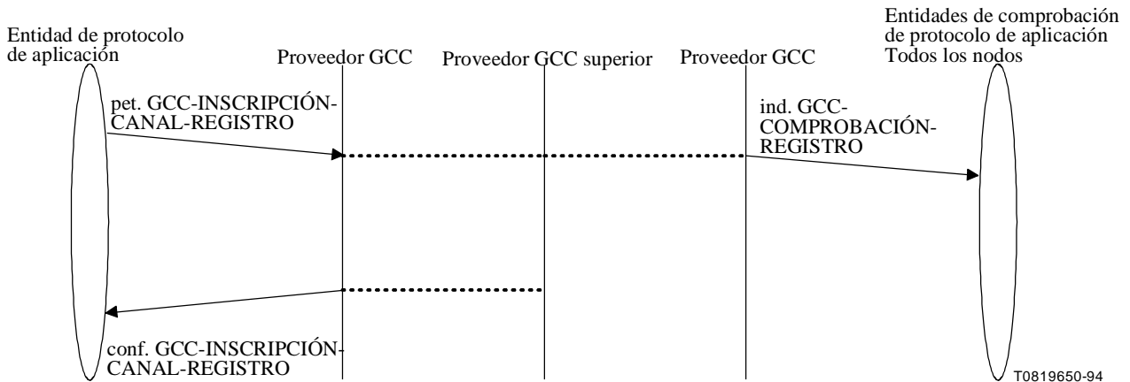
Figura 7-23/T.124 – GCC-INSCRIPCIÓN-CANAL-REGISTRO – Secuencia de primitivas
