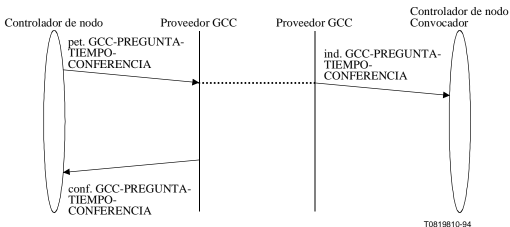
Figura 7-39/T.124 – GCC-PREGUNTA-TIEMPO-CONFERENCIA – Secuencia de primitivas
