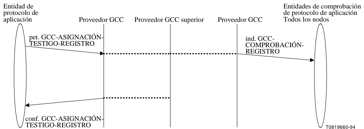
Figura 7-24/T.124 – GCC-ASIGNACIÓN-TESTIGO-REGISTRO – Secuencia de primitivas
