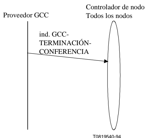
Figura 7-12/T.124 – GCC-TERMINACIÓN-CONFERENCIA (terminación automática) – Secuencia de primitivas
