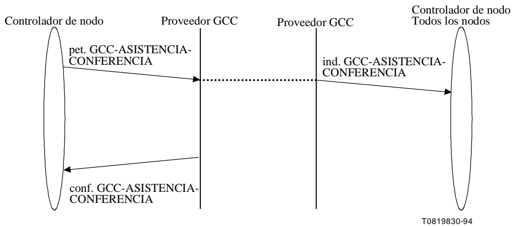
Figura 7-41/T.124 – GCC-ASISTENCIA-CONFERENCIA – Secuencia de primitivas
