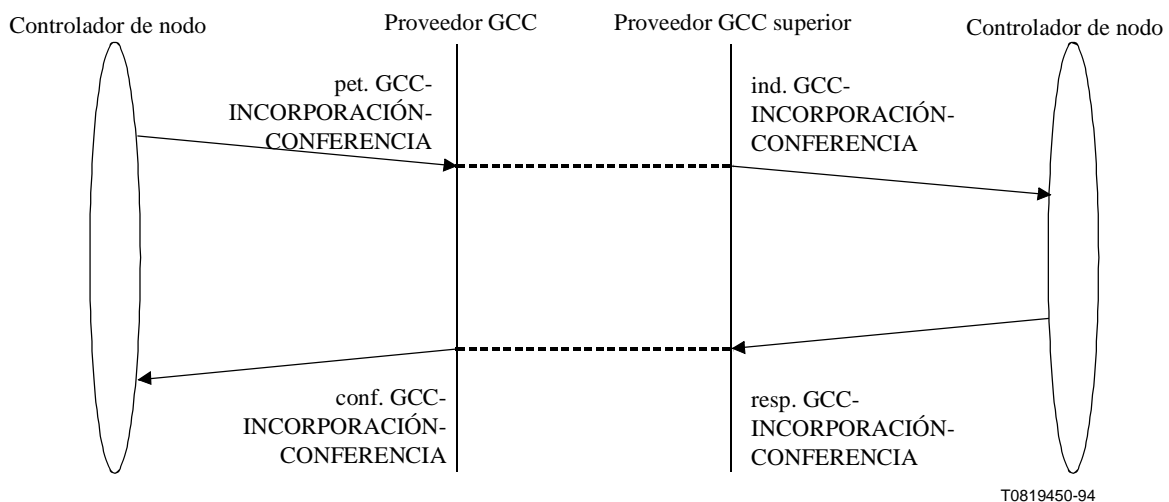
Figura 7-3/T.124 – GCC-INCORPORACIÓN-CONFERENCIA – Secuencia de primitivas
