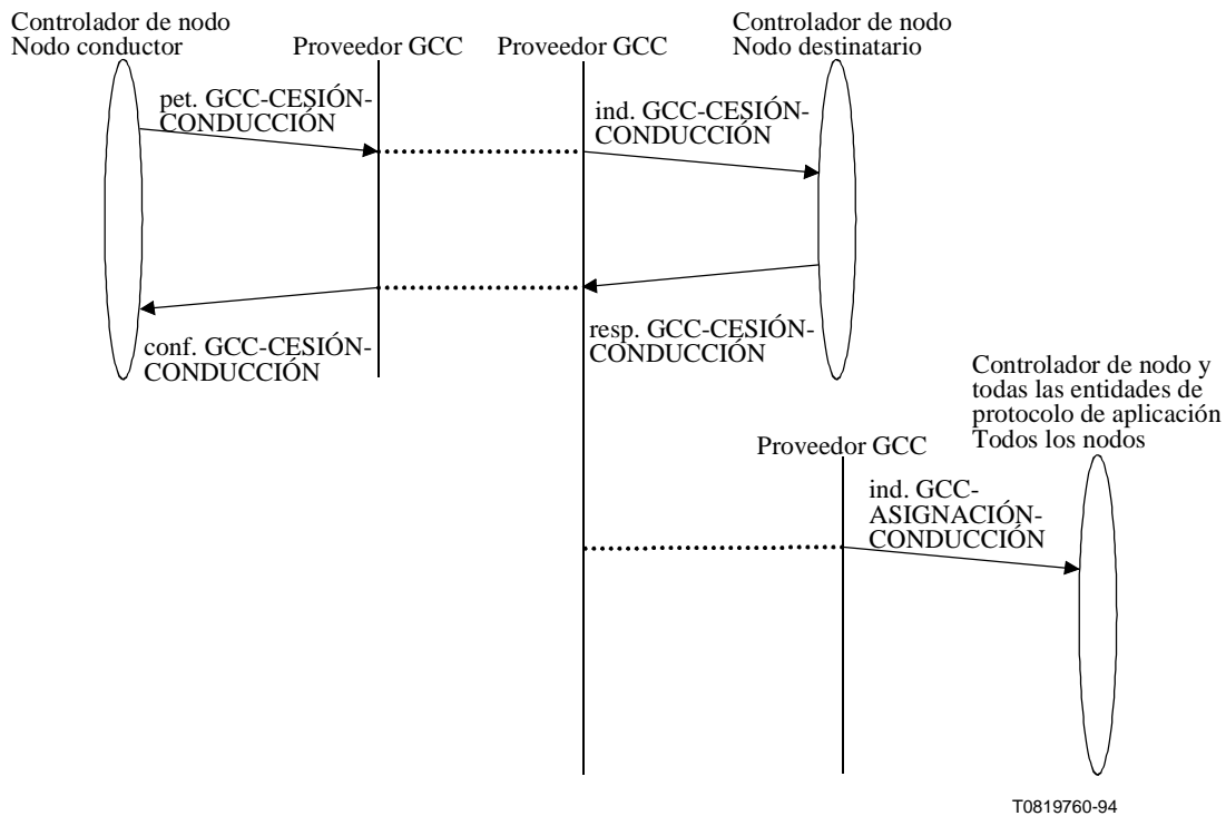
Figura 7-34/T.124 – GCC-CESIÓN-CONDUCCIÓN – Secuencia de primitivas
