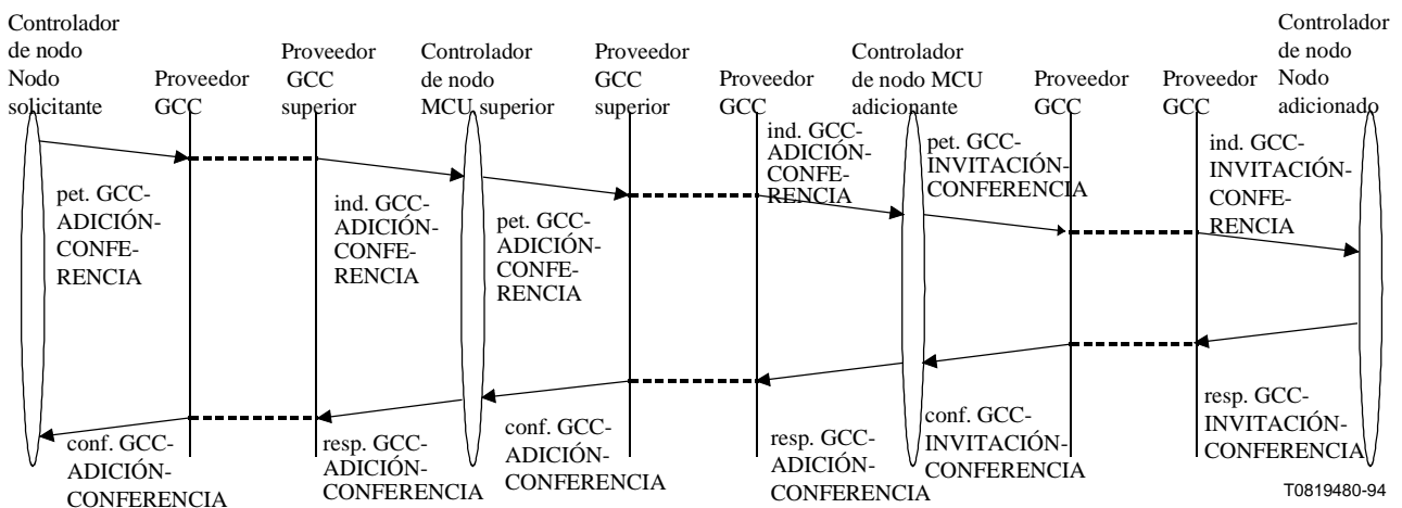
Figura 7-6/T.124 – GCC-ADICIÓN-CONFERENCIA (caso indirecto) – Secuencia de primitivas
