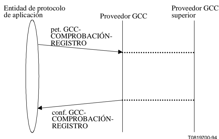
Figura 7-28/T.124 – GCC-COMPROBACIÓN-REGISTRO – Secuencia de primitivas
