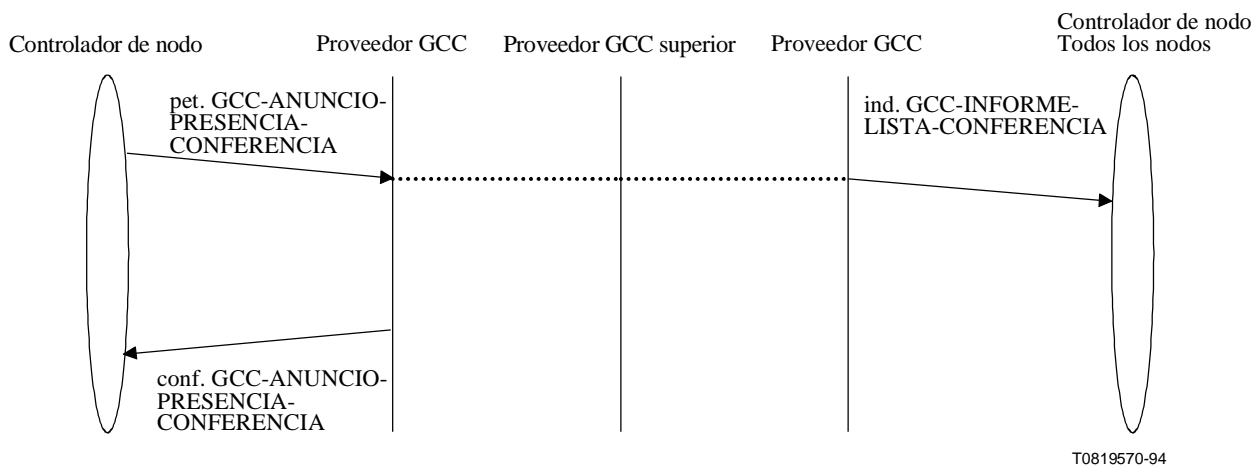
Figura 7-15/T.124 – GCC-ANUNCIO-PRESENCIA-CONFERENCIA – Secuencia de primitivas
