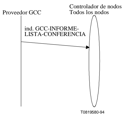
Figura 7-16/T.124 – GCC-INFORME-LISTA-CONFERENCIA – Secuencia de primitivas
