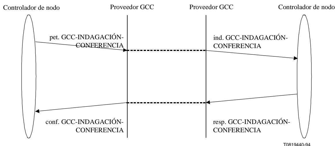
Figura 7-2/T.124 – GCC-INDAGACIÓN-CONFERENCIA – Secuencia de primitivas
