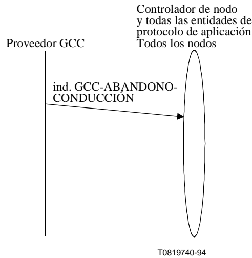
Figura 7-32/T.124 – GCC-ABANDONO-CONDUCCIÓN (iniciada por GCC) – Secuencia de primitivas
