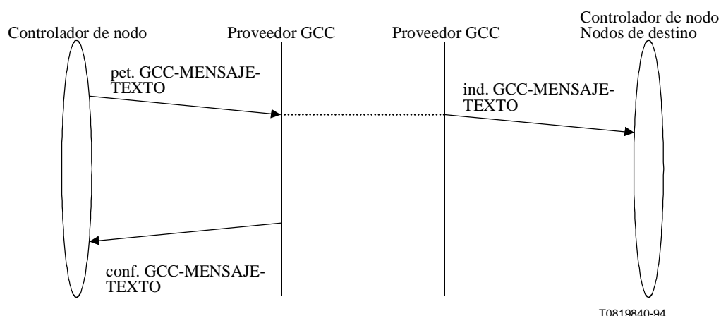
Figura 7-42/T.124 – GCC-MENSAJE-TEXTO – Secuencia de primitivas
