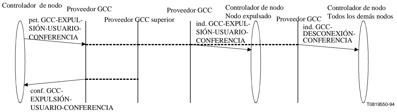
Figura 7-13/T.124 – GCC-EXPULSIÓN-USUARIO-CONFERENCIA – Secuencia de primitivas
