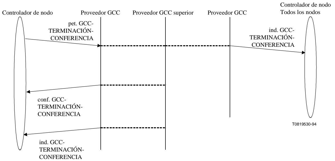
Figura 7-10/T.124 – GCC-TERMINACIÓN-CONFERENCIA (iniciada por el cliente) – Secuencia de primitivas
