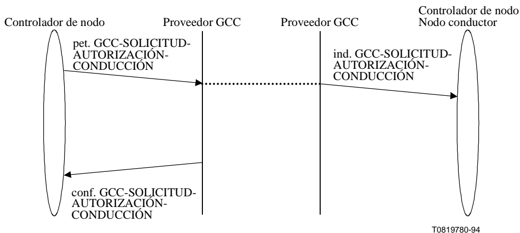
Figura 7-36/T.124 – GCC-SOLICITUD-AUTORIZACIÓN-CONDUCCIÓN – Secuencia de primitivas
