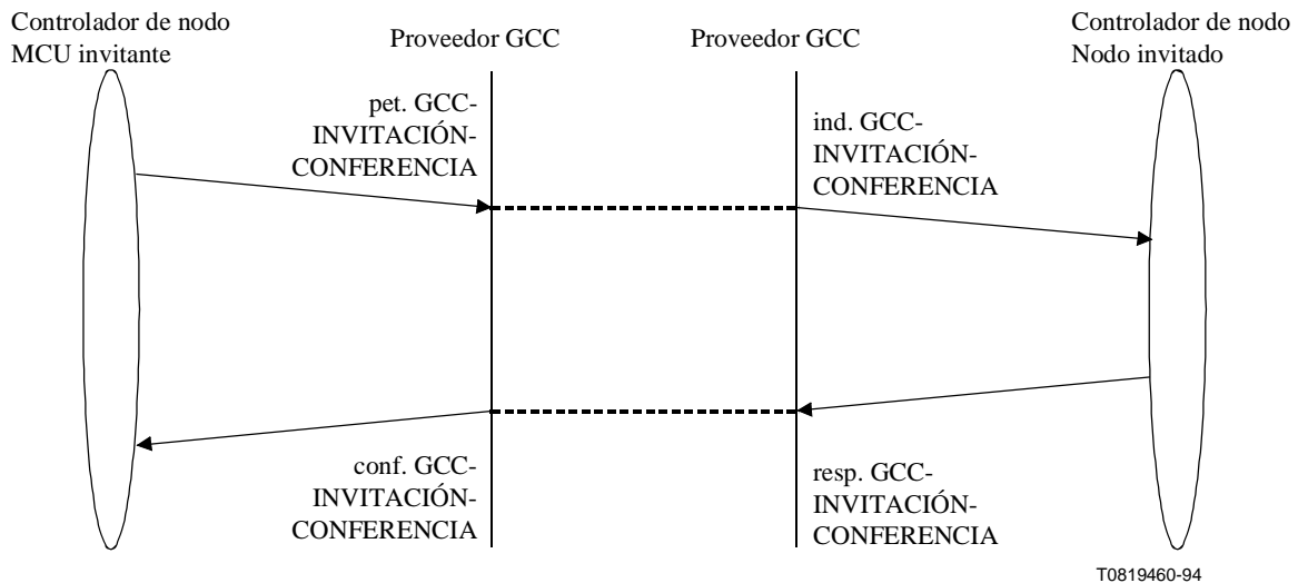
Figura 7-4/T.124 – GCC-INVITACIÓN-CONFERENCIA – Secuencia de primitivas
