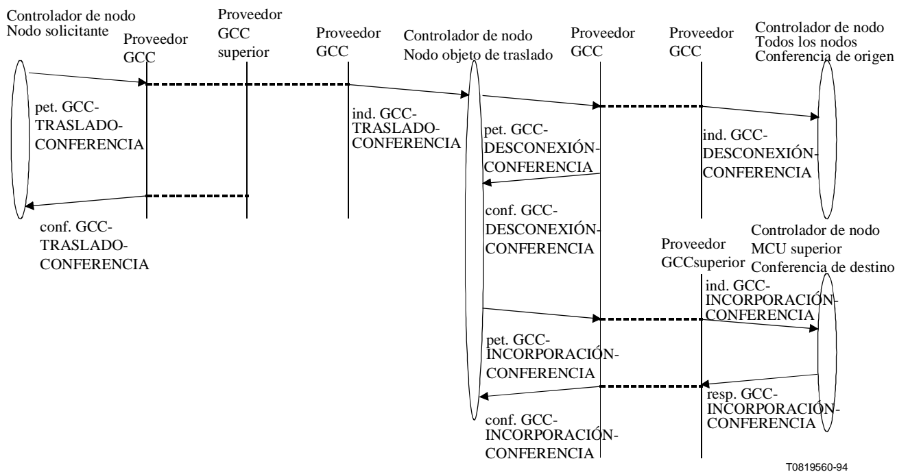
Figura 7-14/T.124 – GCC-TRASLADO-CONFERENCIA – Secuencia de primitivas
