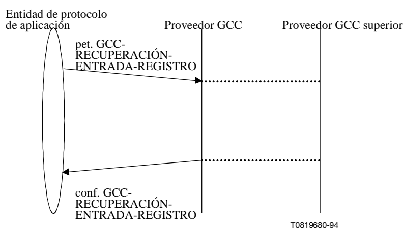
Figura 7-26/T.124 – GCC-RECUPERACIÓN-ENTRADA-REGISTRO – Secuencia de primitivas
