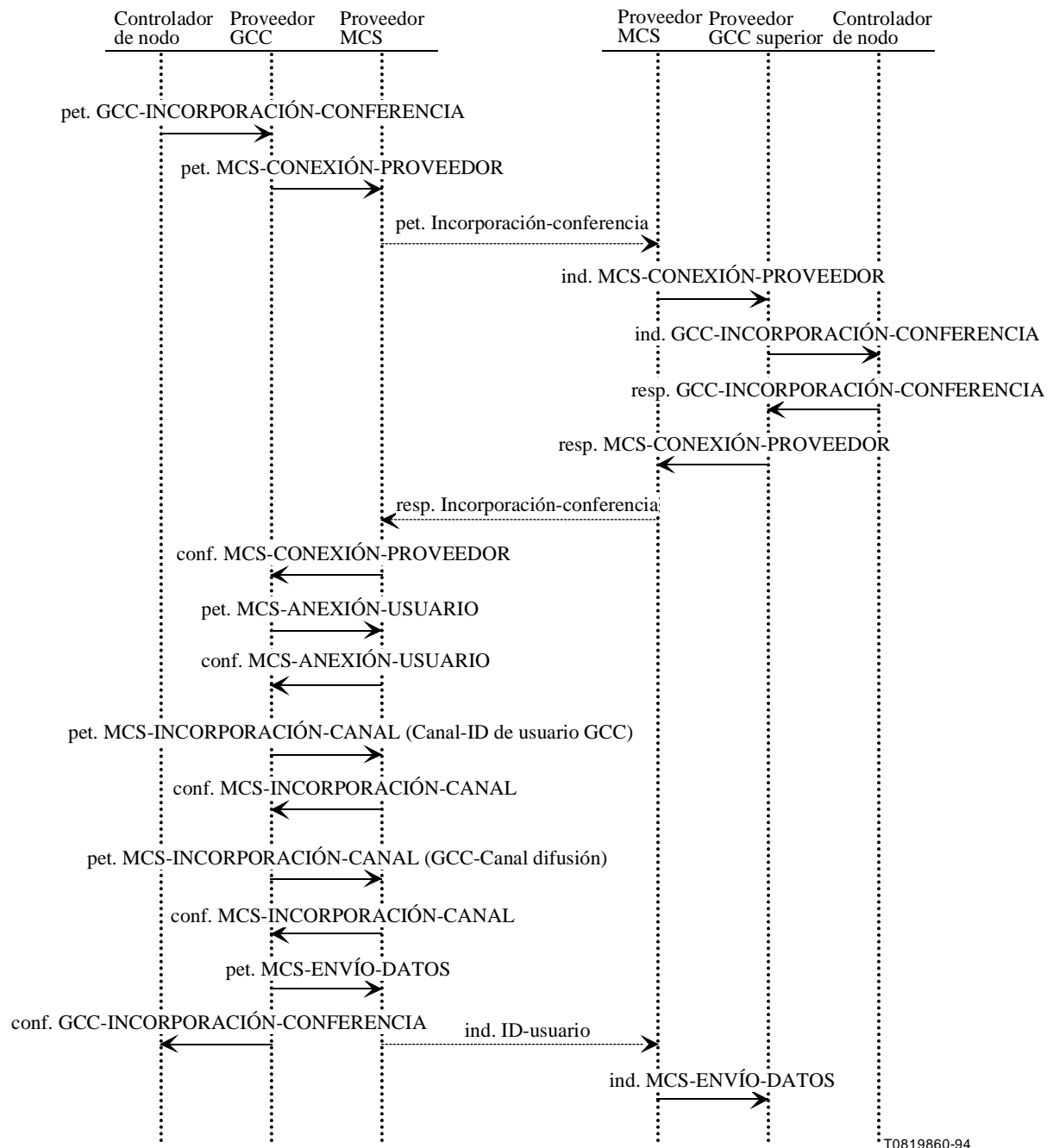
Figura 8-2/T.124 – Cómo incorporarse a una conferencia con conexión directa al proveedor GCC superior
