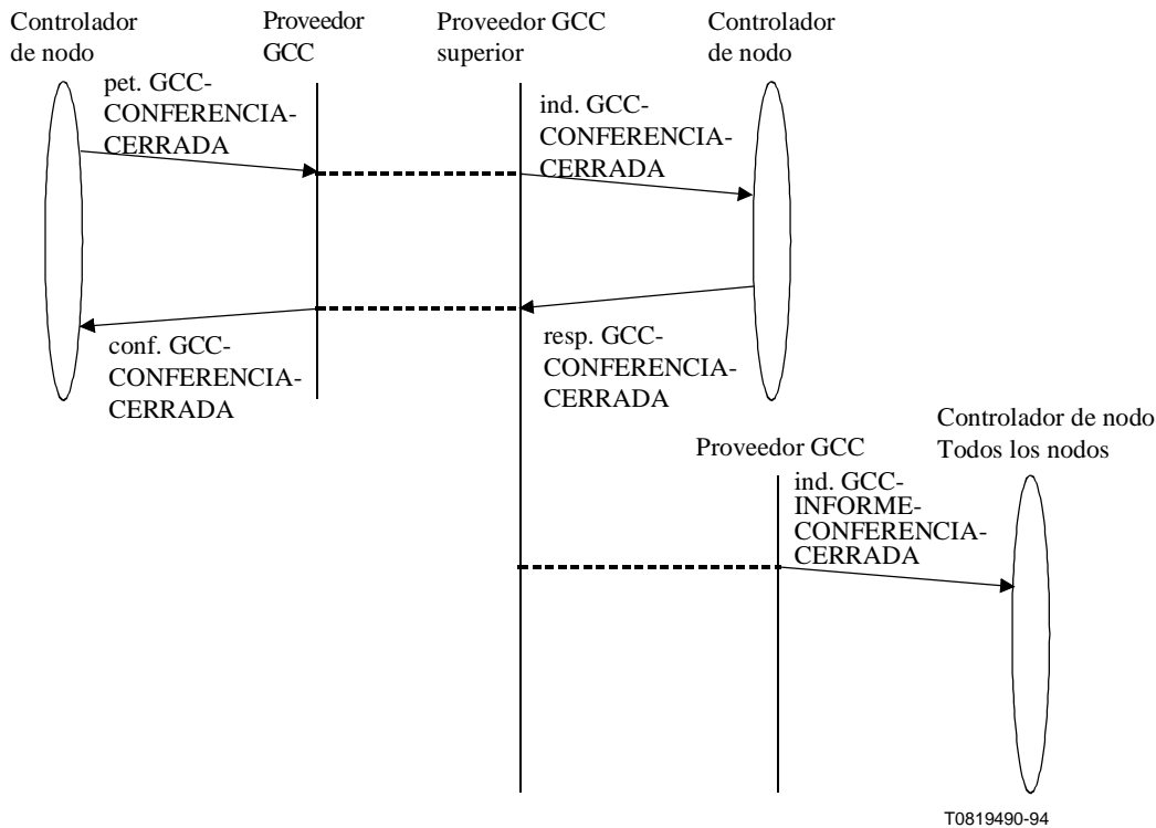
Figura 7-7/T.124 – GCC-CONFERENCIA-CERRADA – Secuencia de primitivas
