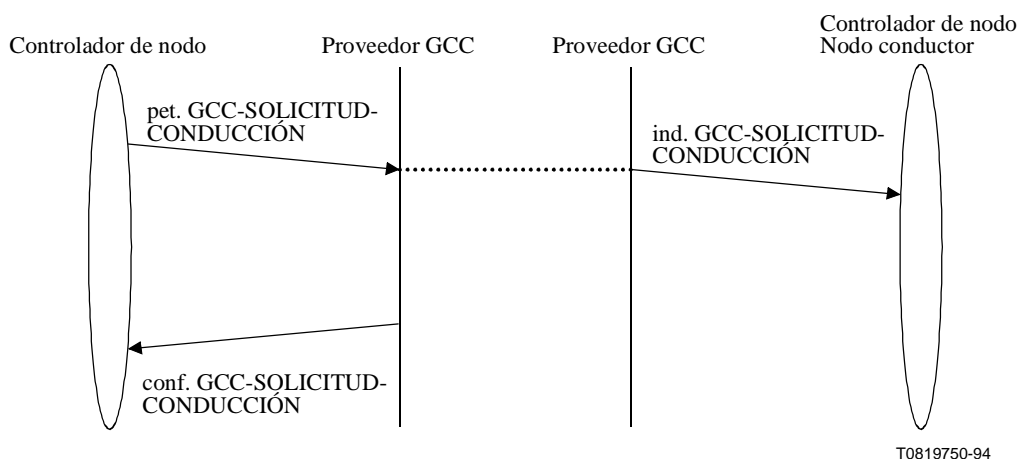
Figura 7-33/T.124 – GCC-SOLICITUD-CONDUCCIÓN – Secuencia de primitivas
