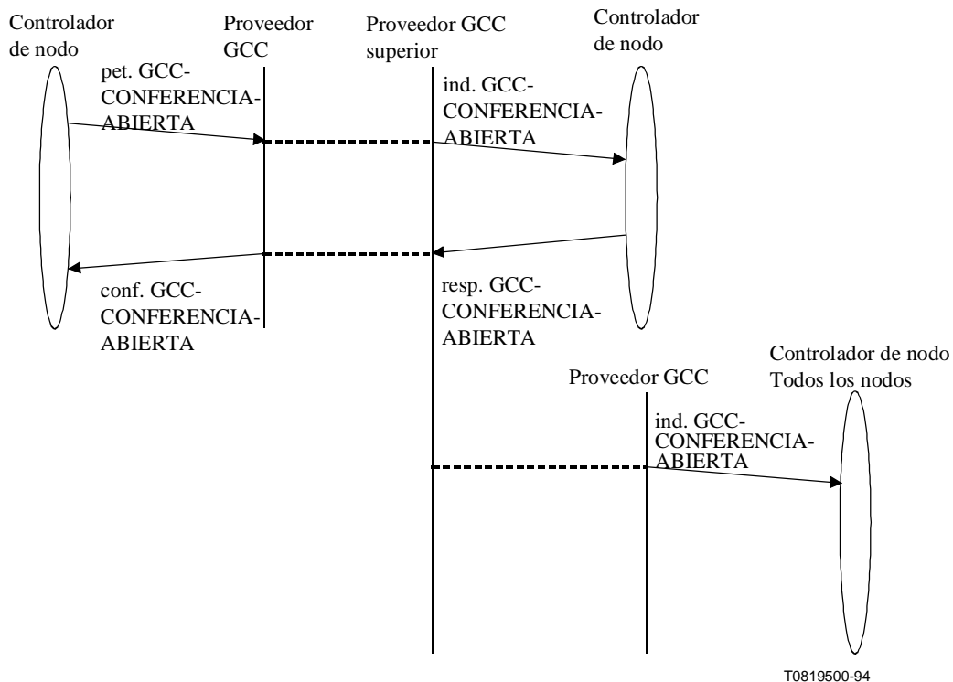
Figura 7-8/T.124 – GCC-CONFERENCIA-ABIERTA – Secuencia de primitivas
