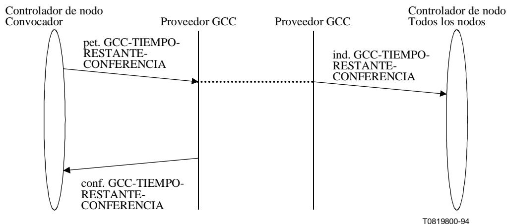
Figura 7-38/T.124 – GCC-TIEMPO-RESTANTE-CONFERENCIA – Secuencia de primitivas
