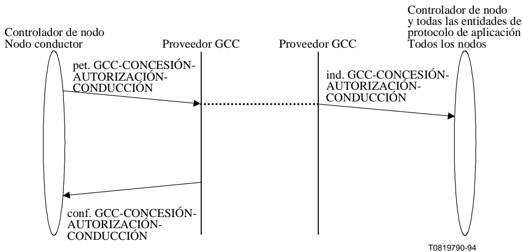
Figura 7-37/T.124 – GCC-CONCESIÓN-AUTORIZACIÓN-CONDUCCIÓN – Secuencia de primitivas
