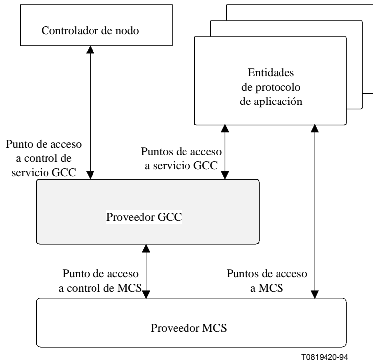
Figura 6-2/T.124 – Modelo de sistema que muestra los puntos de acceso a servicio GCC y la relación con MCS
