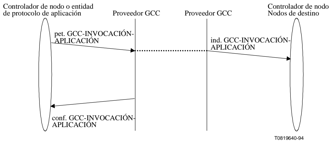
Figura 7-22/T.124 – GCC-INVOCACIÓN-APLICACIÓN – Secuencia de primitivas
