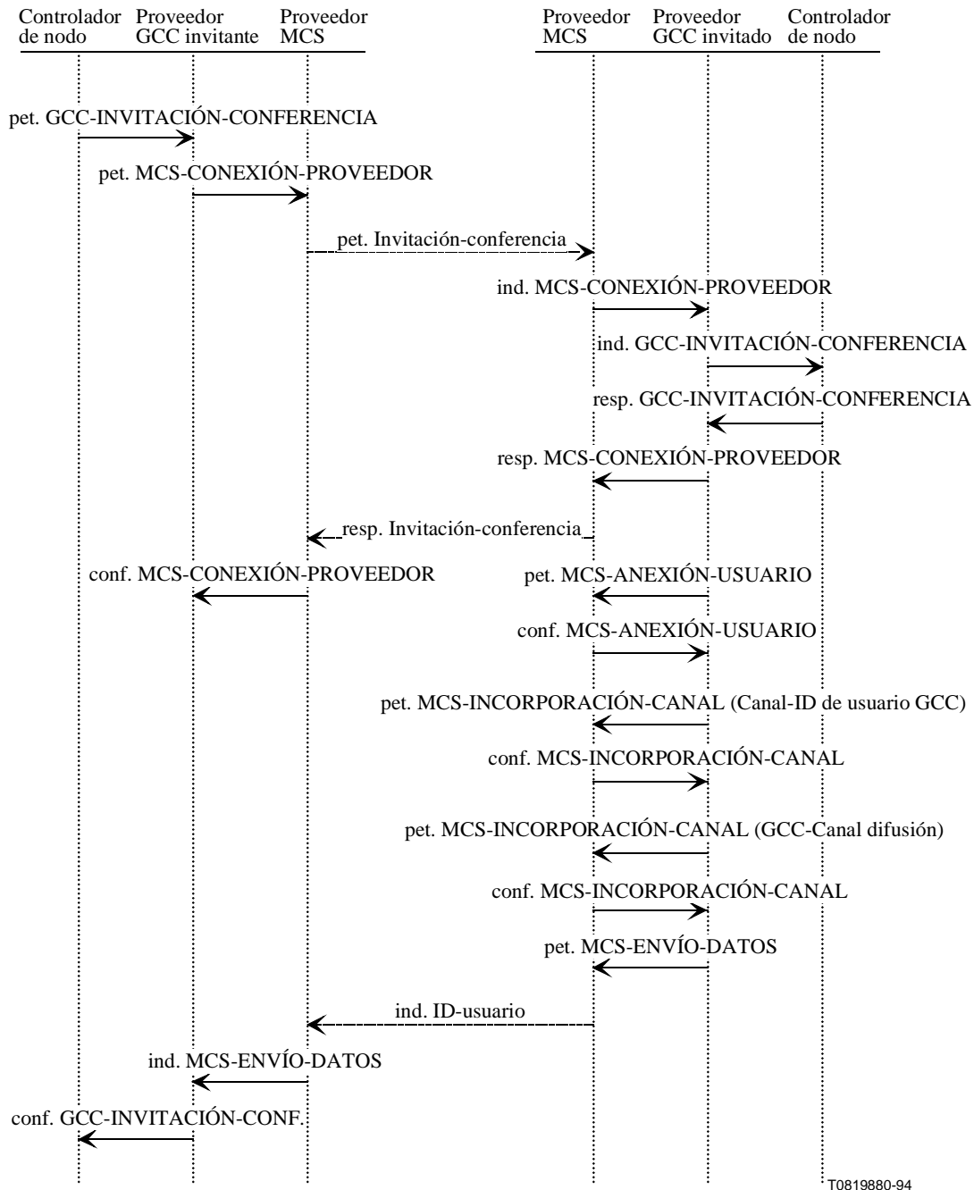
Figura 8-4/T.124 – Cómo invitar a un nodo a una conferencia
