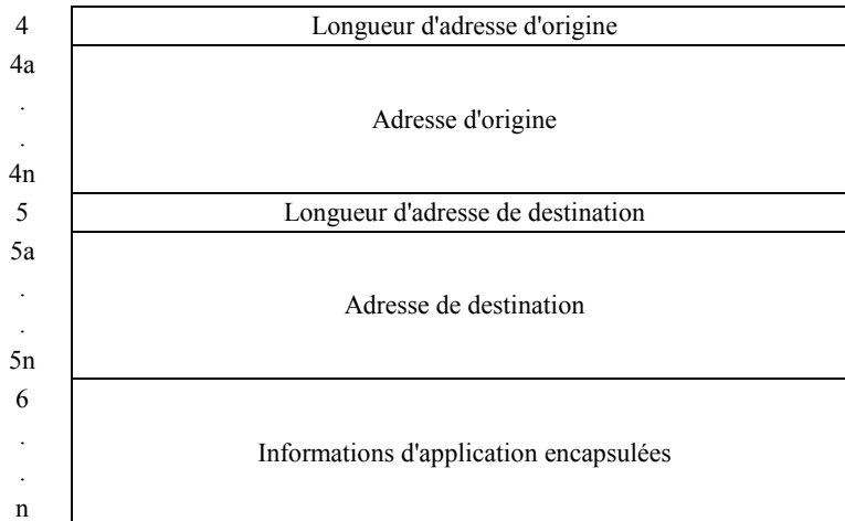
Figure 77.2/Q.763 – Contenu du champ d'information d'utilisateur du mécanisme APM pour les applications d'utilisateur du mécanisme APM'2000'
