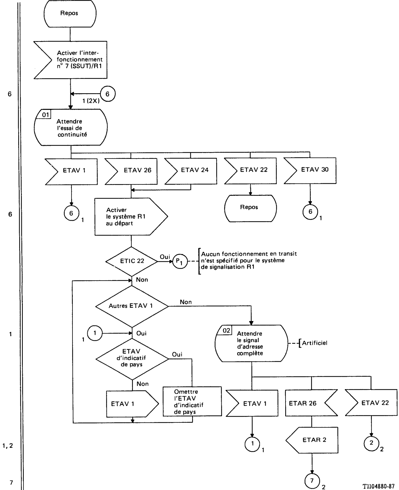
FIGURE 3/Q.665 (feuillet 1 sur 2) Interfonctionnement n° 7 (SSUT) vers R1
