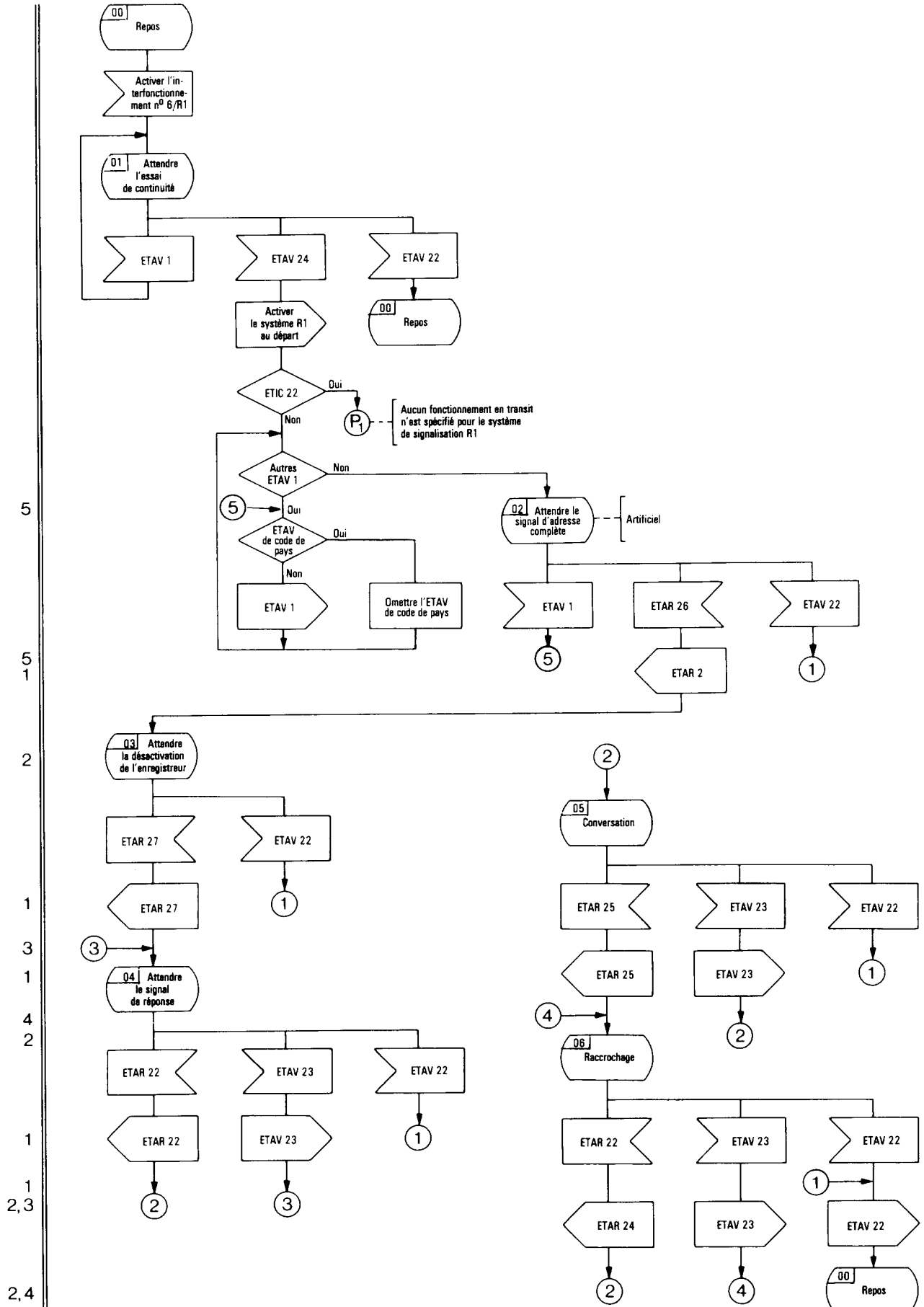
FIGURE 3/Q.654 Interfonctionnement n° 6 vers R1
