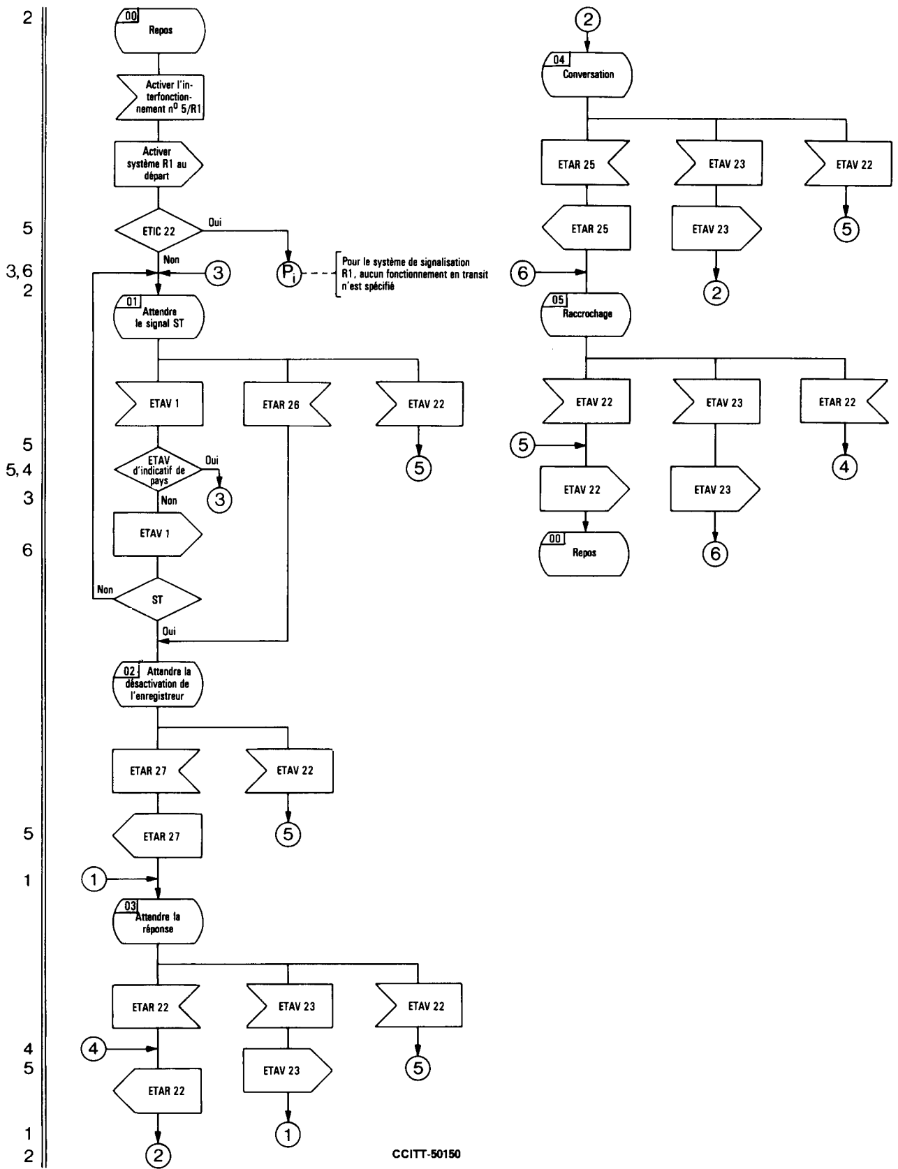
FIGURE 3/Q.644 Interfonctionnement n° 5 vers R1
