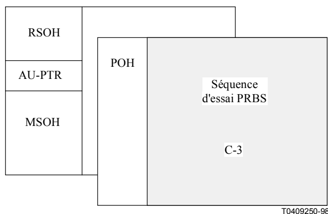
Figure A.2/O.172 – Structure de signal d'essai pour la mesure de la gigue de l'interface STM-0
