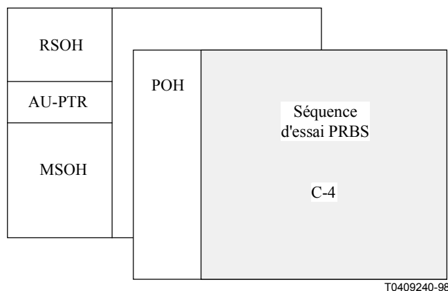
Figure A.1/O.172 – Structure de signal d'essai pour la mesure de la gigue de l'interface STM-1
