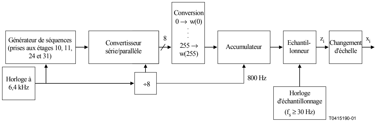
Figure V.2/O.172 – Autre source de bruit TIE utilisée pour vérifier les algorithmes de calcul d'écart MTIE et TDEV
