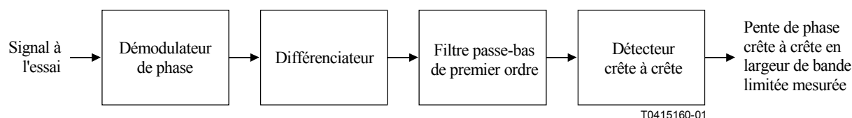
Figure B.1/O.172 – Fonction de mesure de la pente de phase
