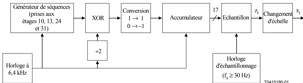
Figure V.1/O.172 – Source de bruit TIE utilisée pour la vérification des algorithmes de calcul d'écart MTIE et TDEV
