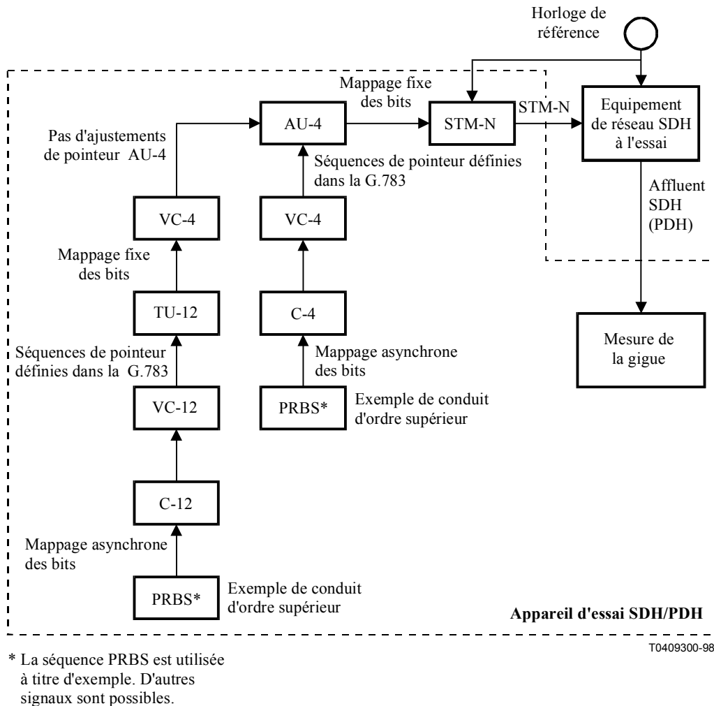
Figure III.1/O.172 – Schéma de principe du montage pour la production de séquences d'essai de pointeur
