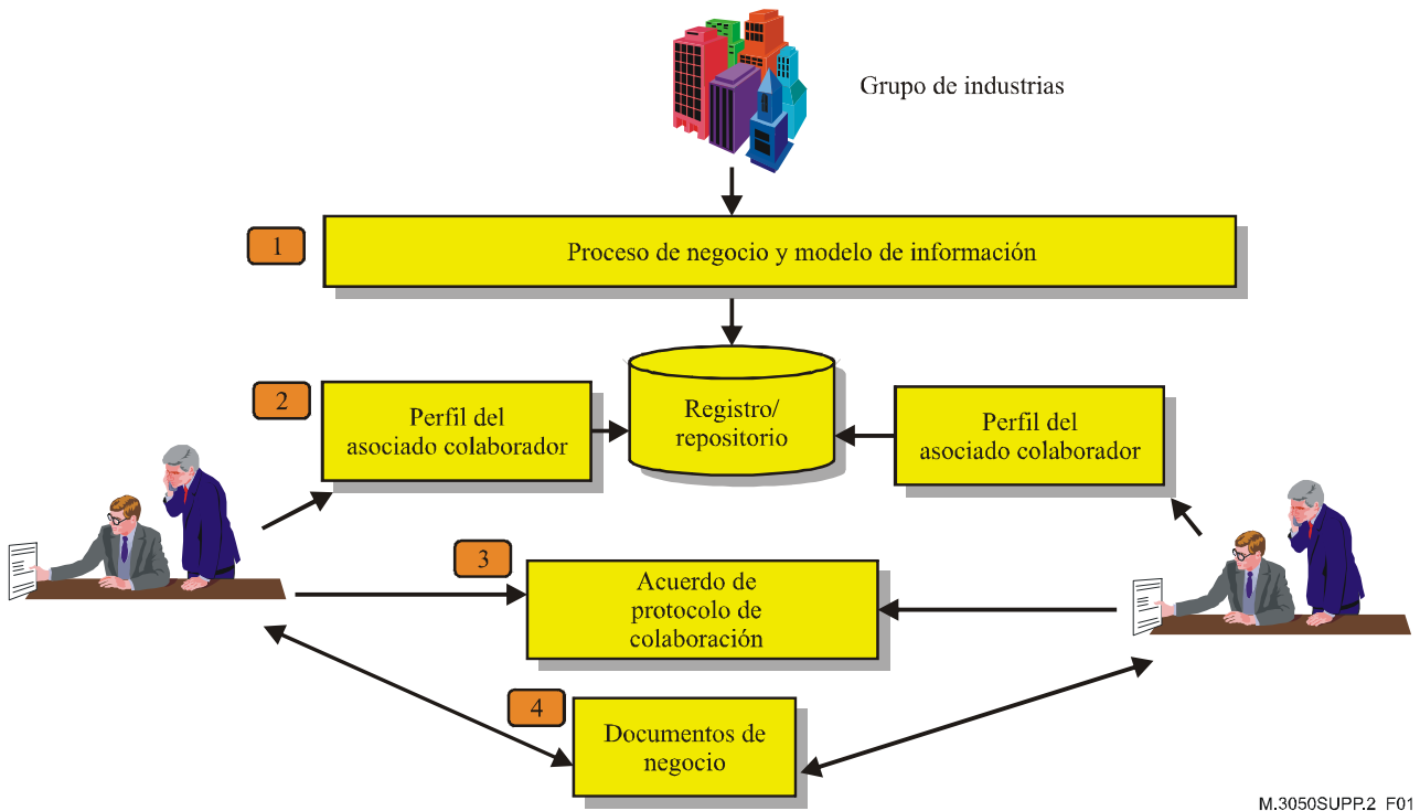
Figura 1 – Repositorio ebXML
