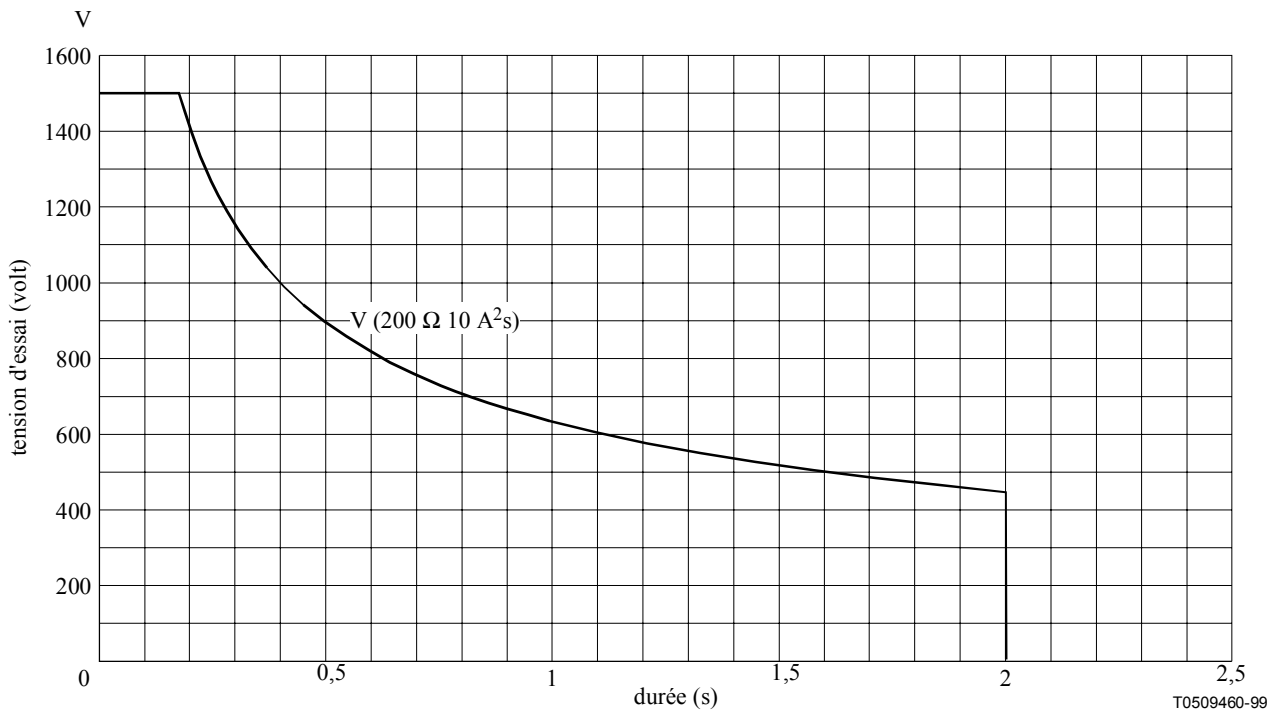
Figure 1/K.20 – Tension d'essai en fonction de la durée pour obtenir 10 A^2s avec 200 \Omega
