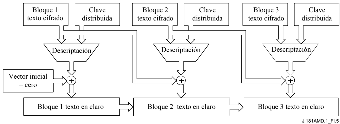
Figura I.5/J.181 – Ejemplo de descripción DES con CBC
