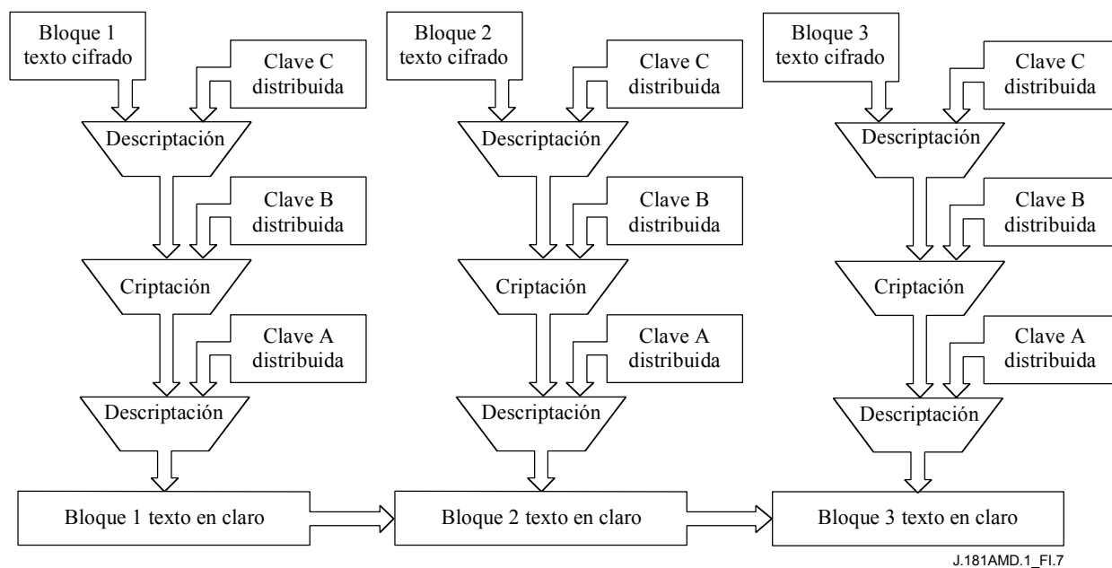
Figura I.7/J.181 – Ejemplo de descryptación DES triple con ECB
