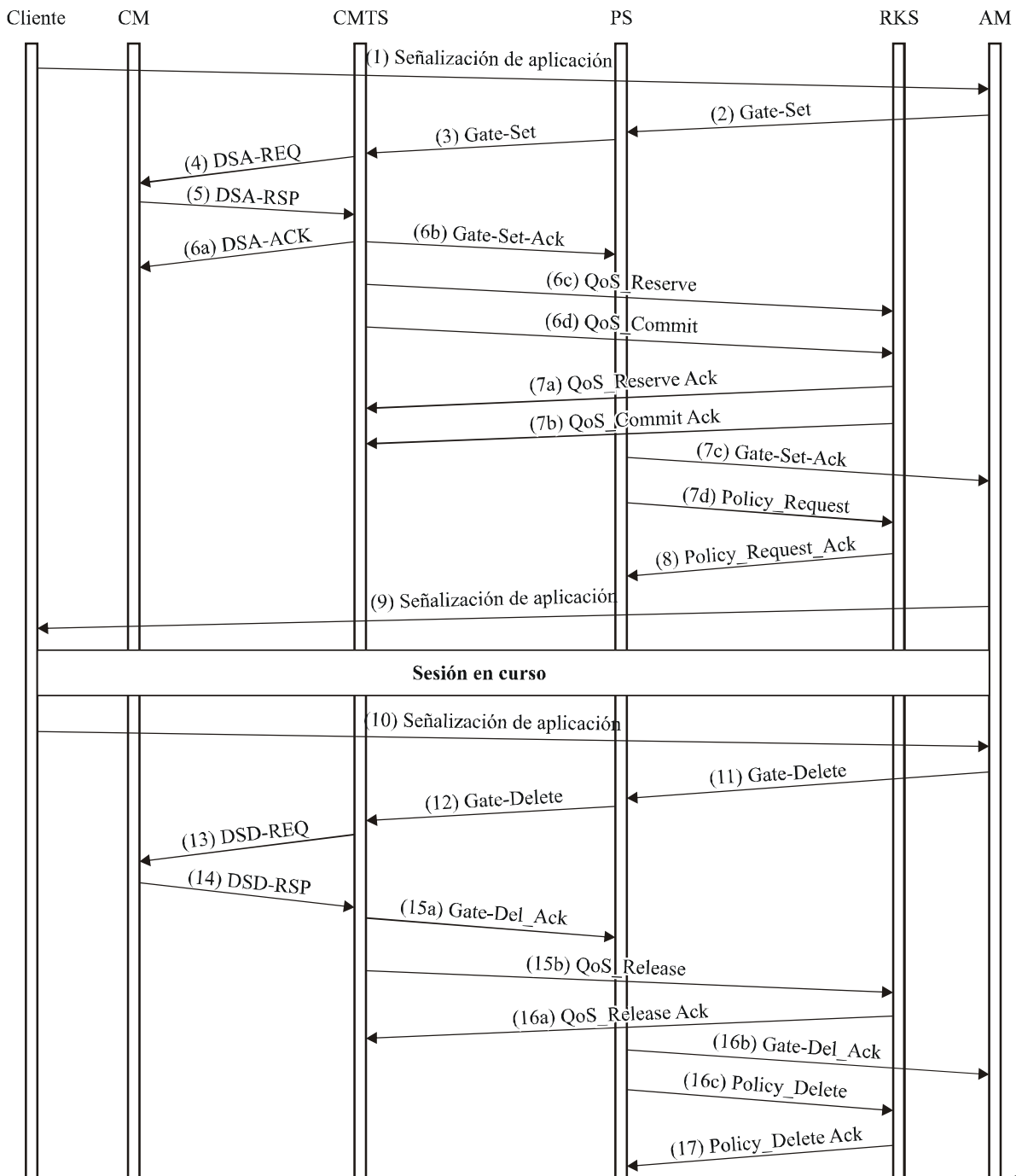
Figura 9/J.179 – Secuencia de mensajes detallada
