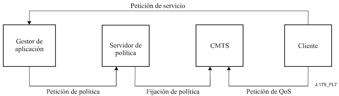
Figura I.7/J.179 – Marco de autorización del escenario 2
