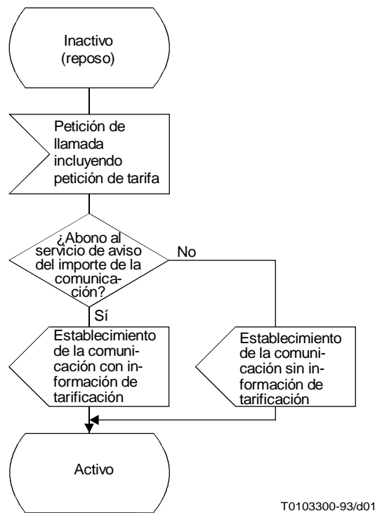
FIGURA 1/I.256.2a Información de tarificación – Petición de tarifa al establecerse la comunicación
