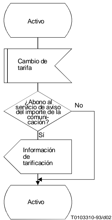
FIGURA 2/I.256.2a Información de tarificación – Cambio de la tarifa en la fase activa de una llamada
