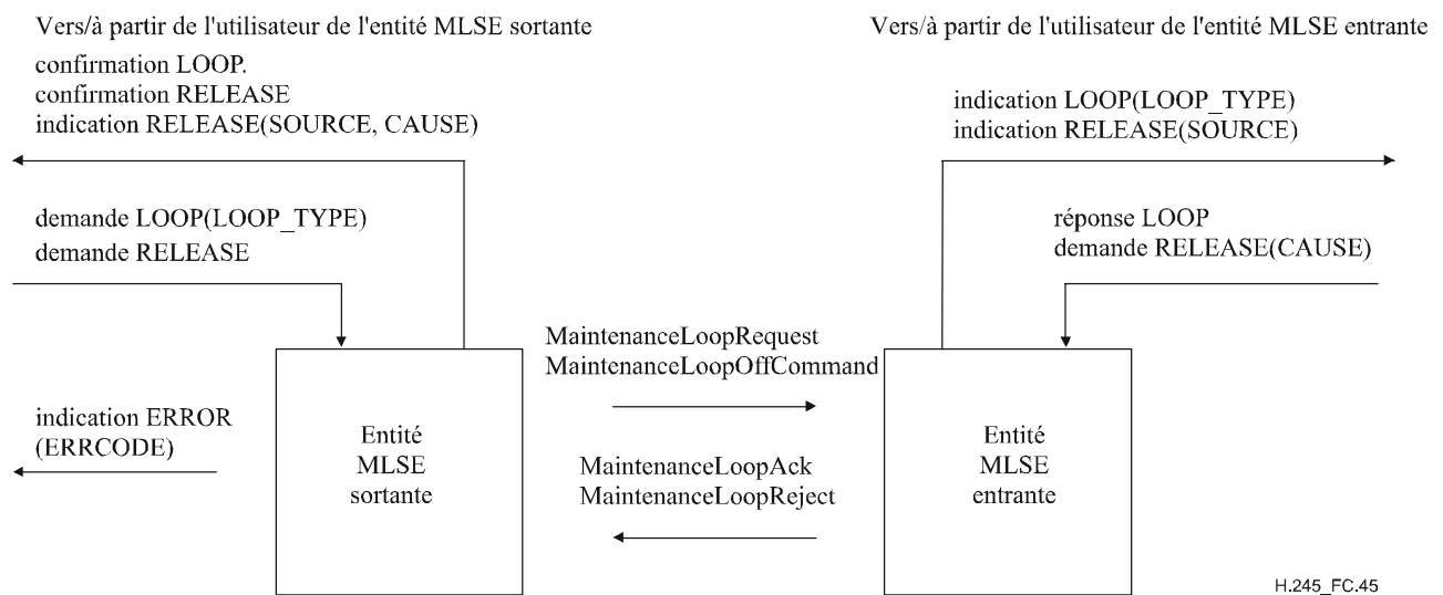
Figure C.45/H.245 – Primitives et messages dans l'entité de signalisation de boucle de maintenance
