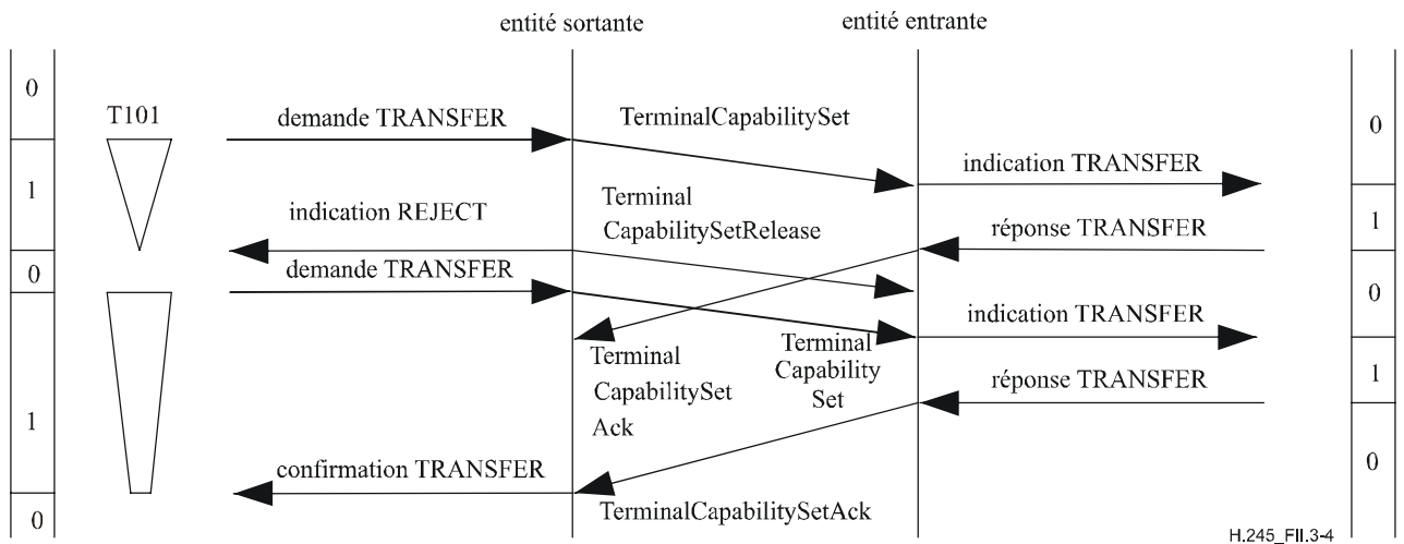
Figure II.3-3/H.245 – Echange de capacités avec expiration de la temporisation T101
