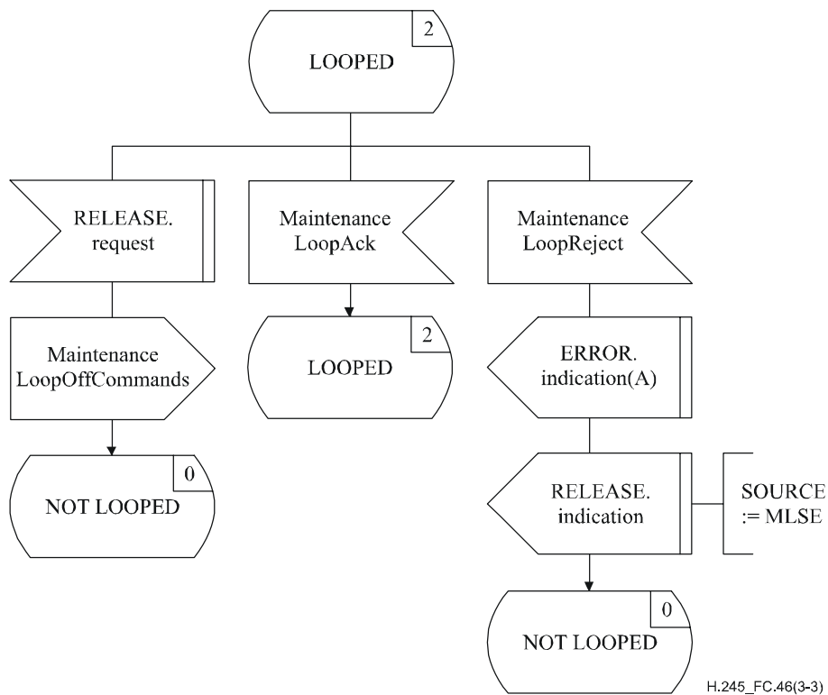
Figure C.46/H.245 – Diagramme SDL de l'entité MLSE sortante (feuille 3 de 3)
