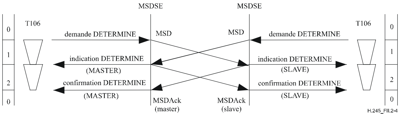
Figure II.2-4/H.245 – Désignation maître-esclave – Désignation simultanée
