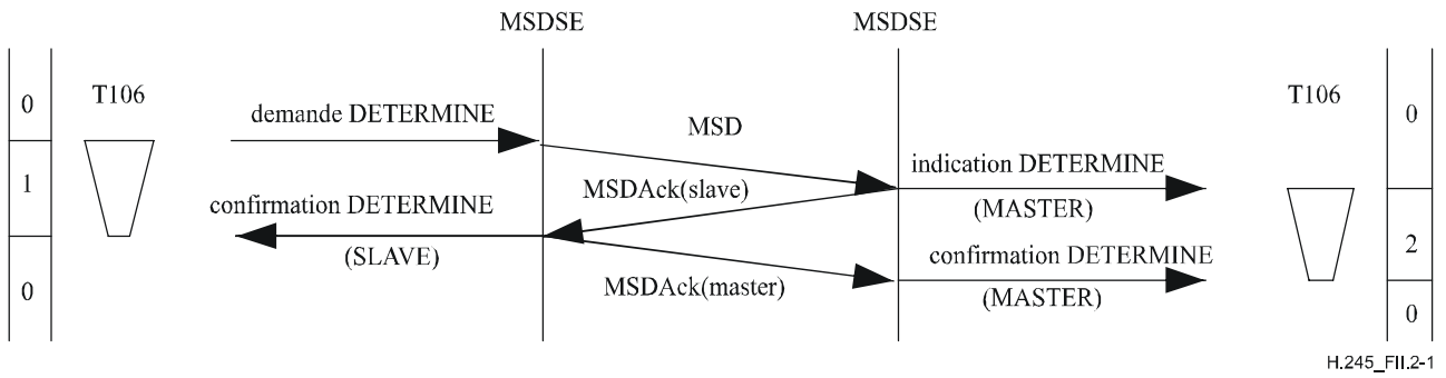
Figure II.2-1/H.245 – Désignation maître-esclave – Terminal maître dans l'entité MSDSE distante
