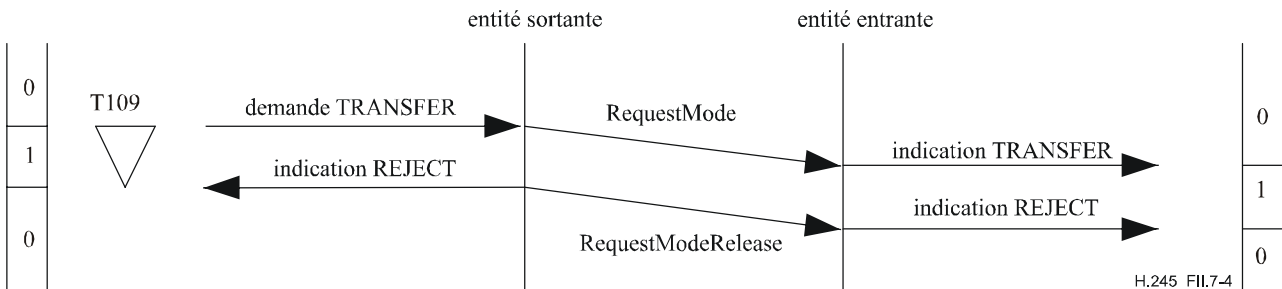
Figure II.7-3/H.245 – Demande de mode avec deuxième demande de mode avant acquittement de la première demande
