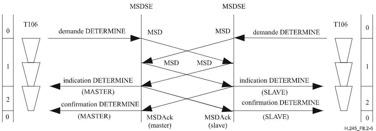
Figure II.2-5/H.245 – Désignation maître-esclave – Désignation simultanée mais avec retour de résultat indéterminé à la première tentative
