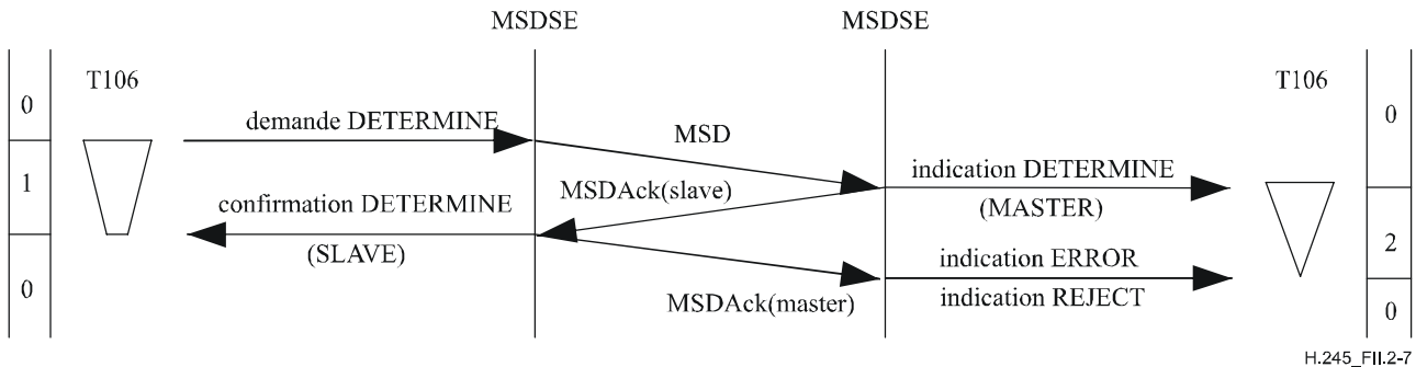
Figure II.2-7/H.245 – Désignation maître-esclave – Temporisation distante T106 à expiration avec terminal maître du côté distant
