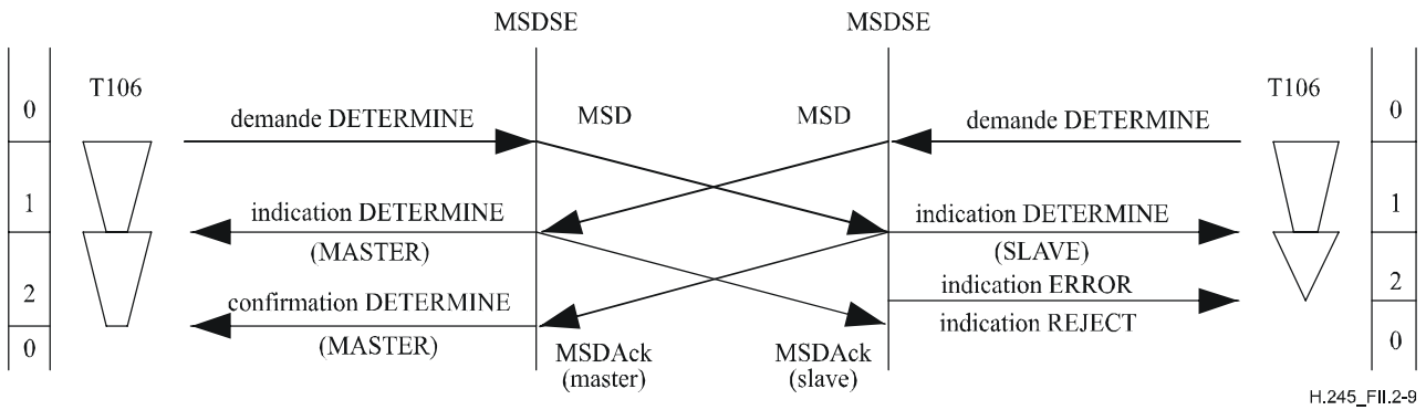
Figure II.2-9/H.245 – Désignation maître-esclave – Procédures de désignation simultanées avec expiration de la temporisation T106 au cours de l'état INCOMING AWAITING ACKNOWLEDGEMENT
