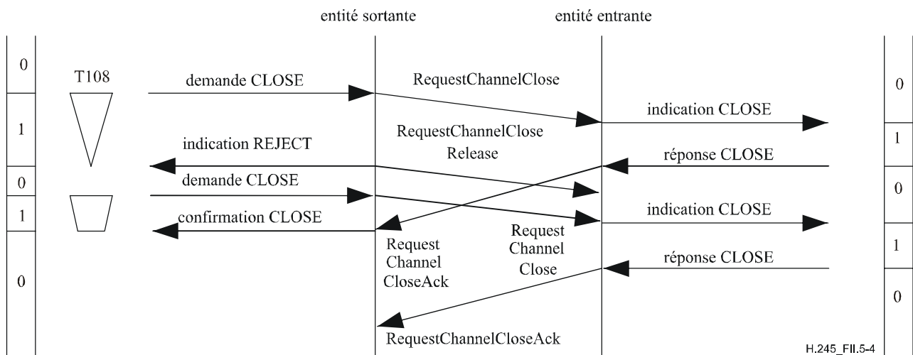
Figure II.5-3/H.245 – Demande de fermeture de voie logique avec expiration de la temporisation T108
