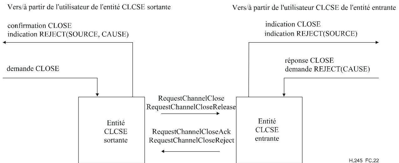
Figure C.22/H.245 – Primitives et messages dans l'entité de signalisation de fermeture de voie logique (CLCSE)
