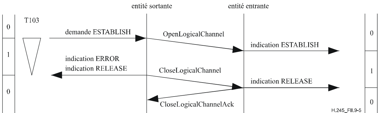
Figure II.9-5/H.245 – Demande d'établissement de voie logique bidirectionnelle avec fin de temporisation T103 du côté sortant par suite d'une réaction lente de l'utilisateur de l'entité B-LCSE entrante homologue
