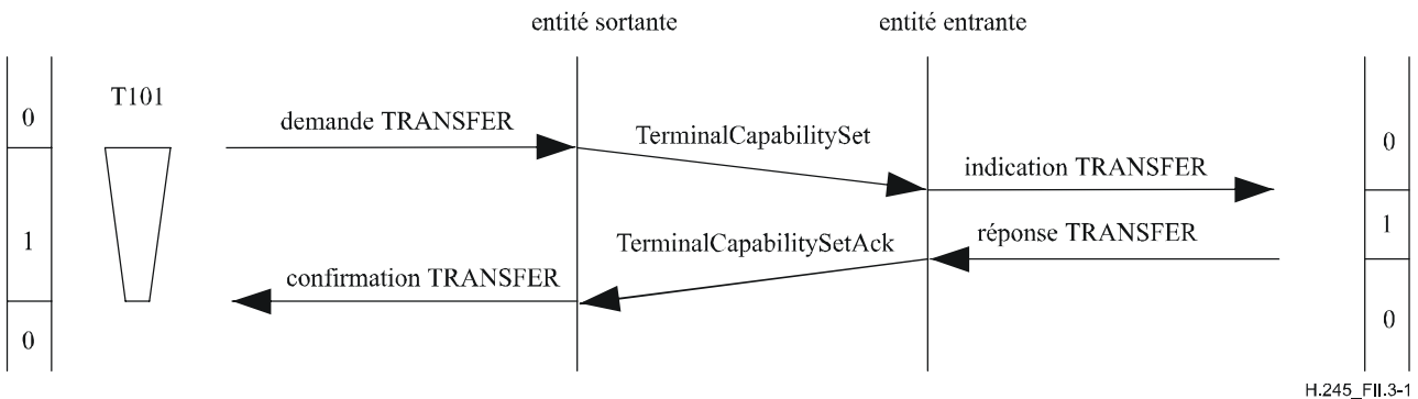
Figure II.3-1/H.245 – Echange de capacités avec acceptation provenant de l'utilisateur de l'entité CESE homologue entrante
