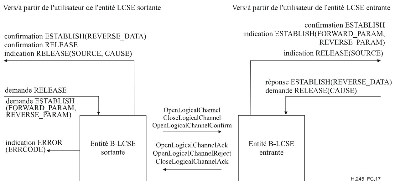
Figure C.17/H.245 – Primitives et messages dans l'entité de signalisation de voie logique bidirectionnelle
