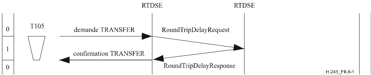
Figure II.8-1/H.245 – Procédure de détermination du temps de propagation aller et retour
