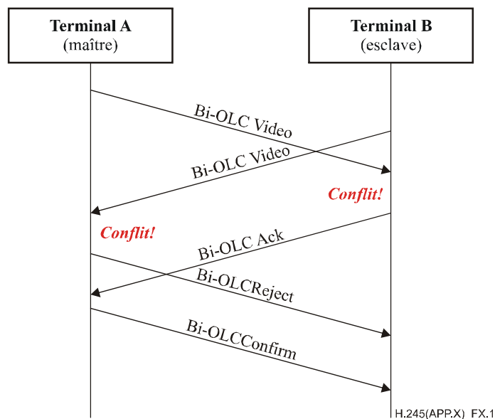
Figure X.1/H.245 – Les deux terminaux utilisent des messages bidirectionnels d'ouverture OLC
