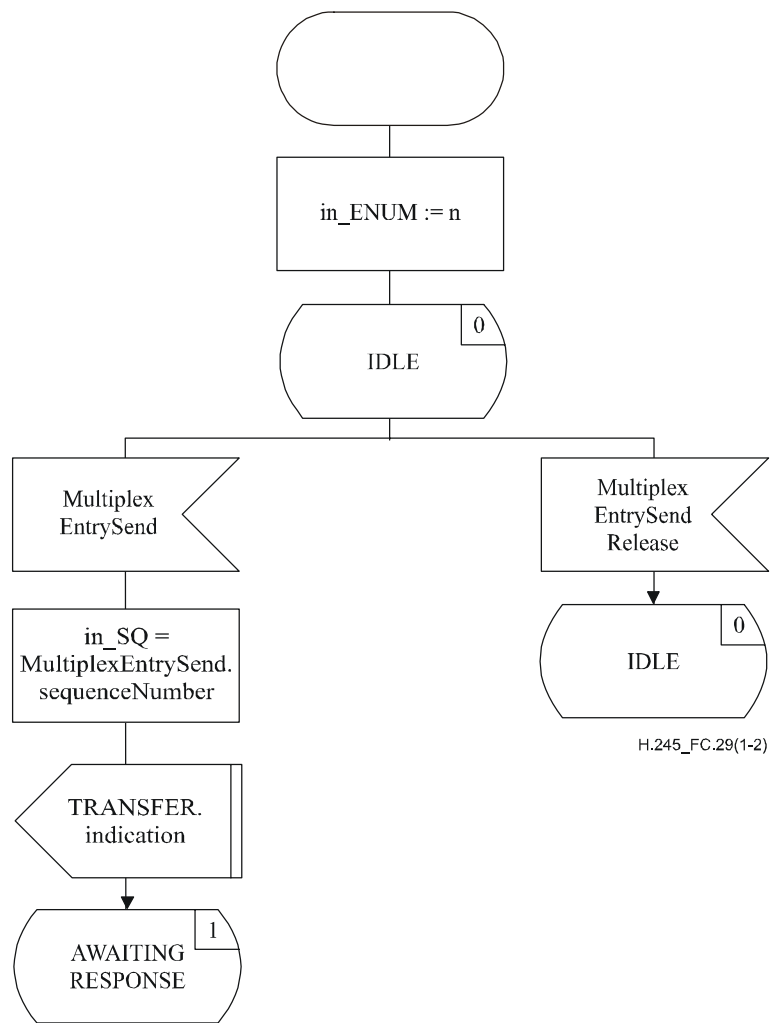
Figure C.29/H.245 – Diagramme SDL dans l'entité MTSE entrante (feuille 1 de 2)
