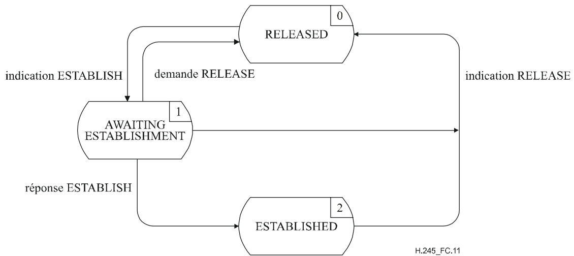
Figure C.11/H.245 – Diagramme de changement d'état pour la séquence de primitives d'une entité LCSE entrante
