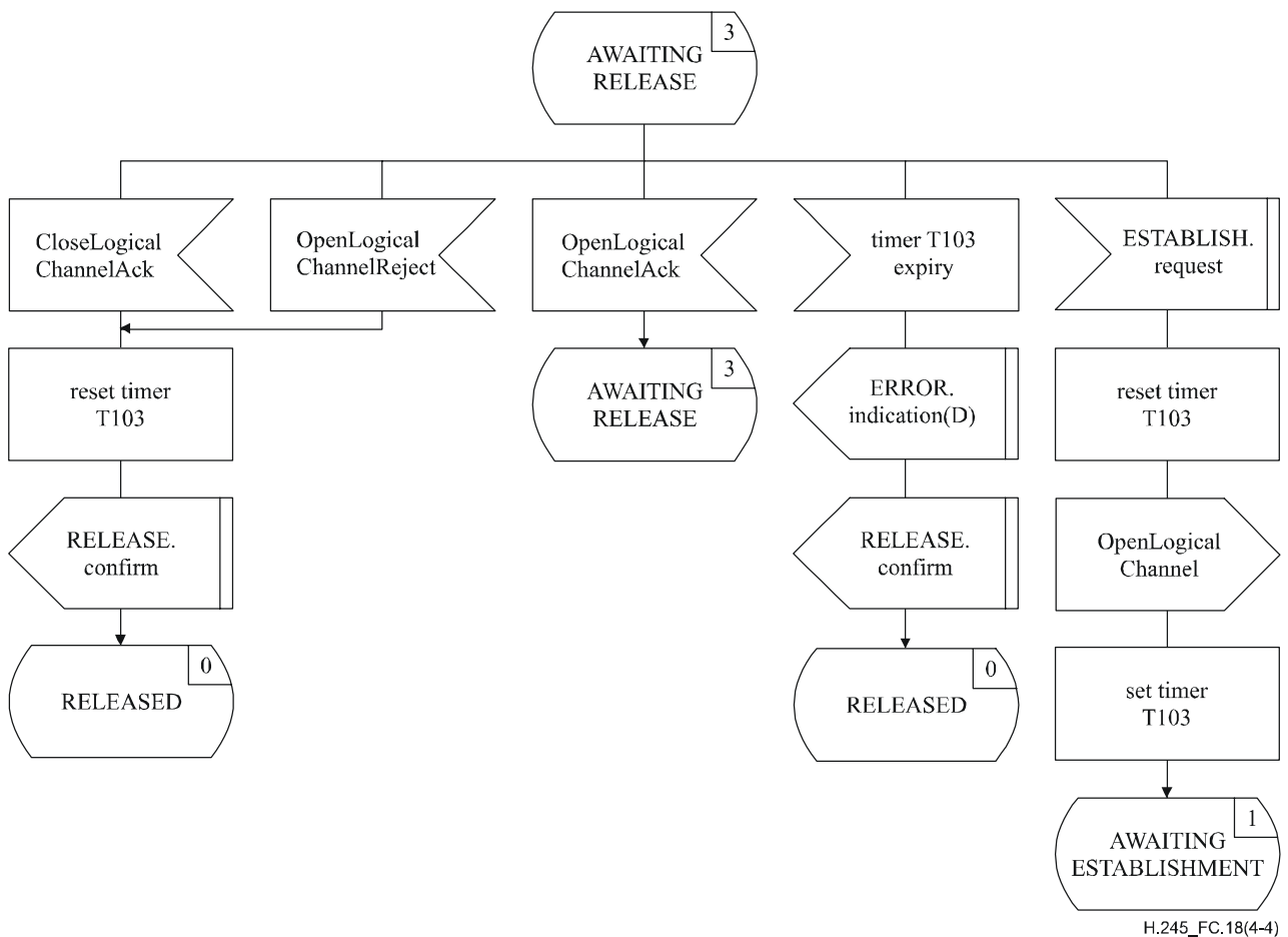
Figure C.18/H.245 – Diagramme SDL de l'entité B-LCSE sortante (feuille 4 de 4)
