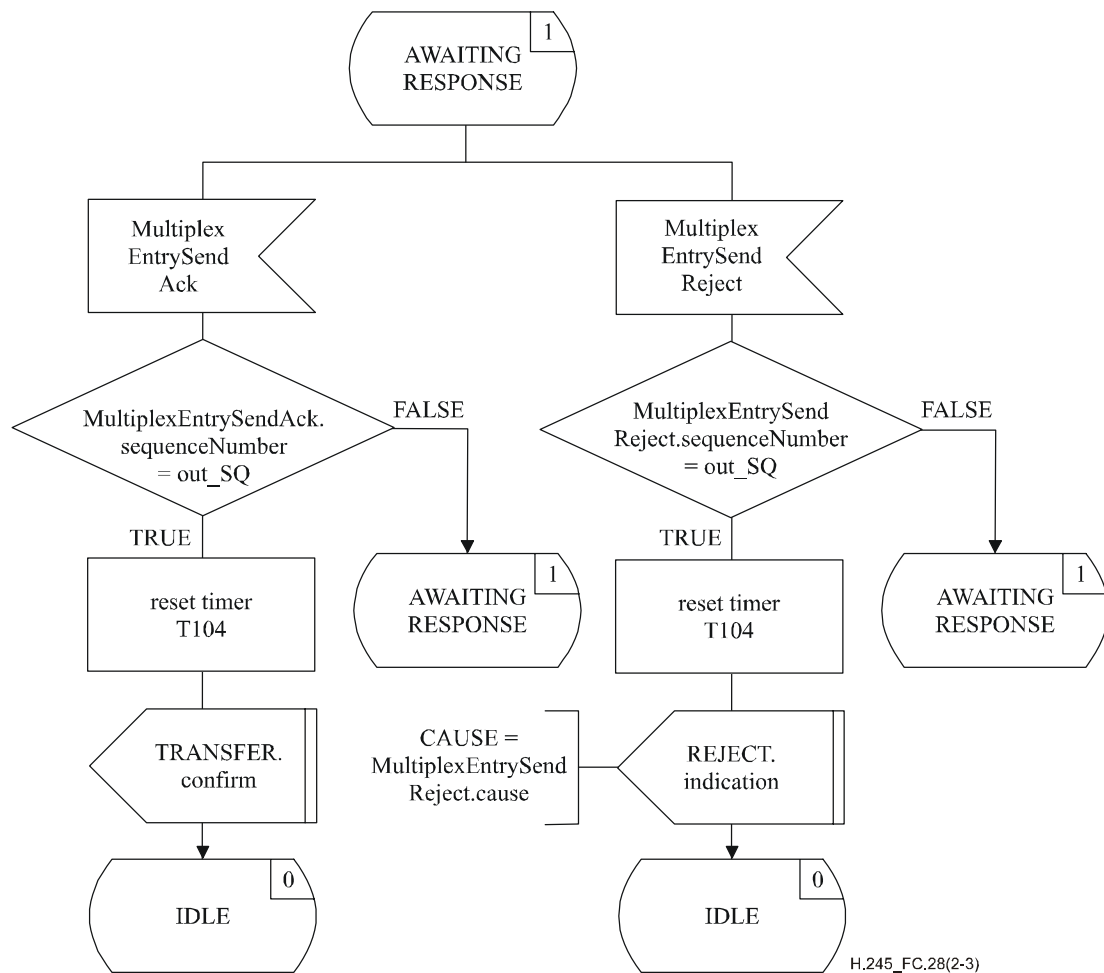
Figure C.28/H.245 – Diagramme SDL dans l'entité MTSE sortante (feuille 2 de 3)
