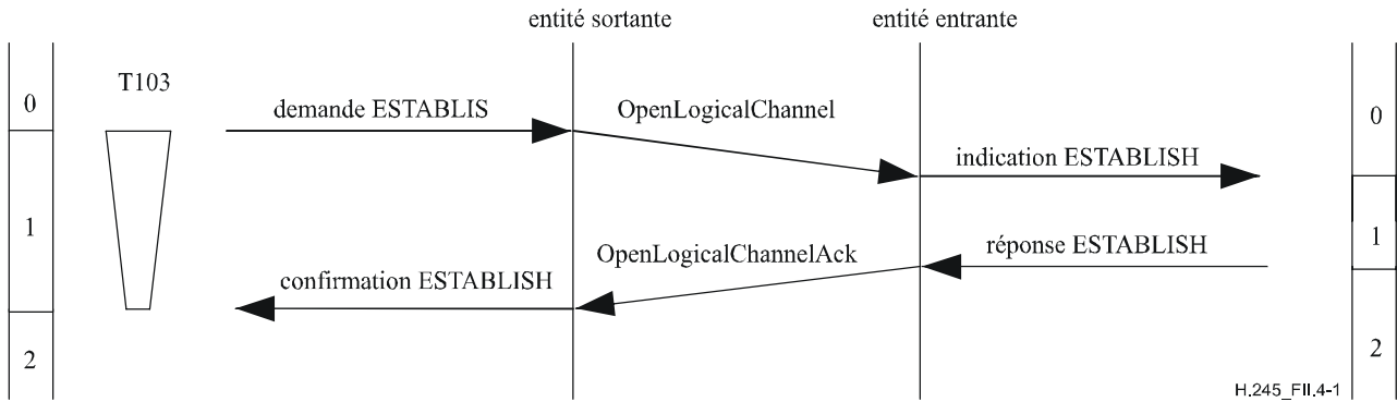
Figure II.4-1/H.245 – Etablissement de voie logique
