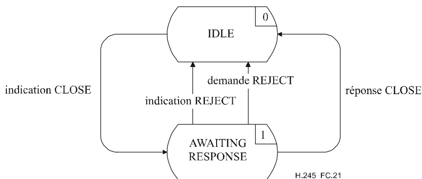
Figure C.21/H.245 – Diagramme de changement d'état pour la séquence de primitives de l'entité CLCSE entrante
