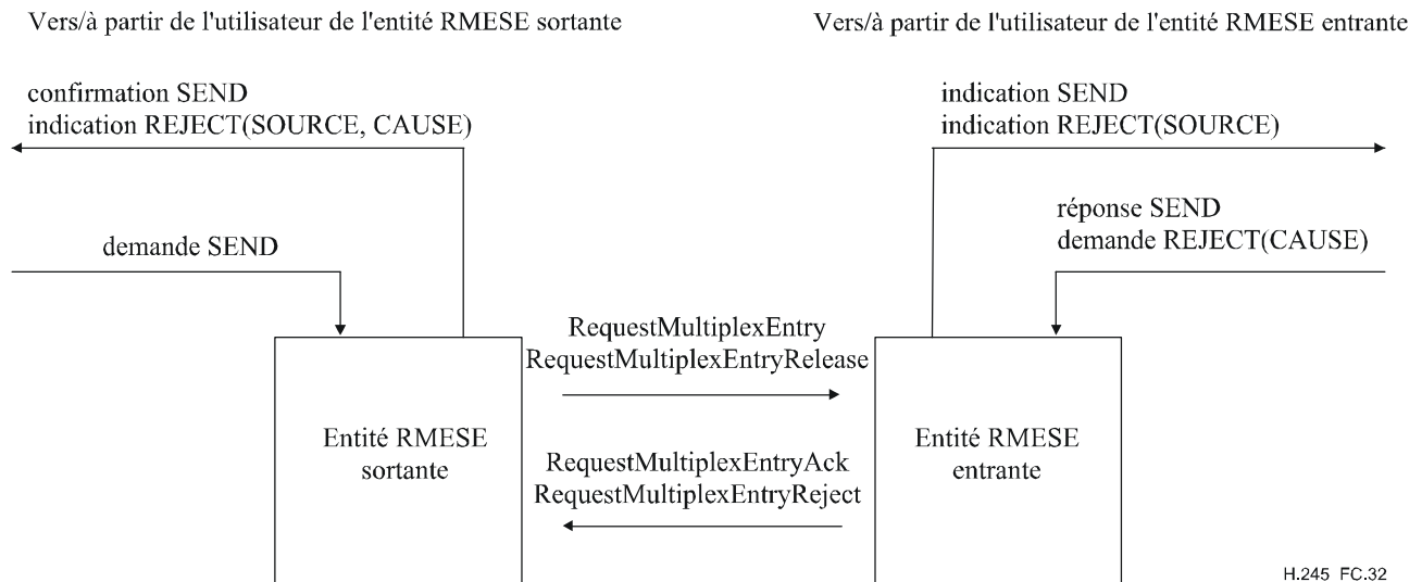
Figure C.32/H.245 – Primitives et messages de l'entité de signalisation de demande d'entrée de multiplexage
