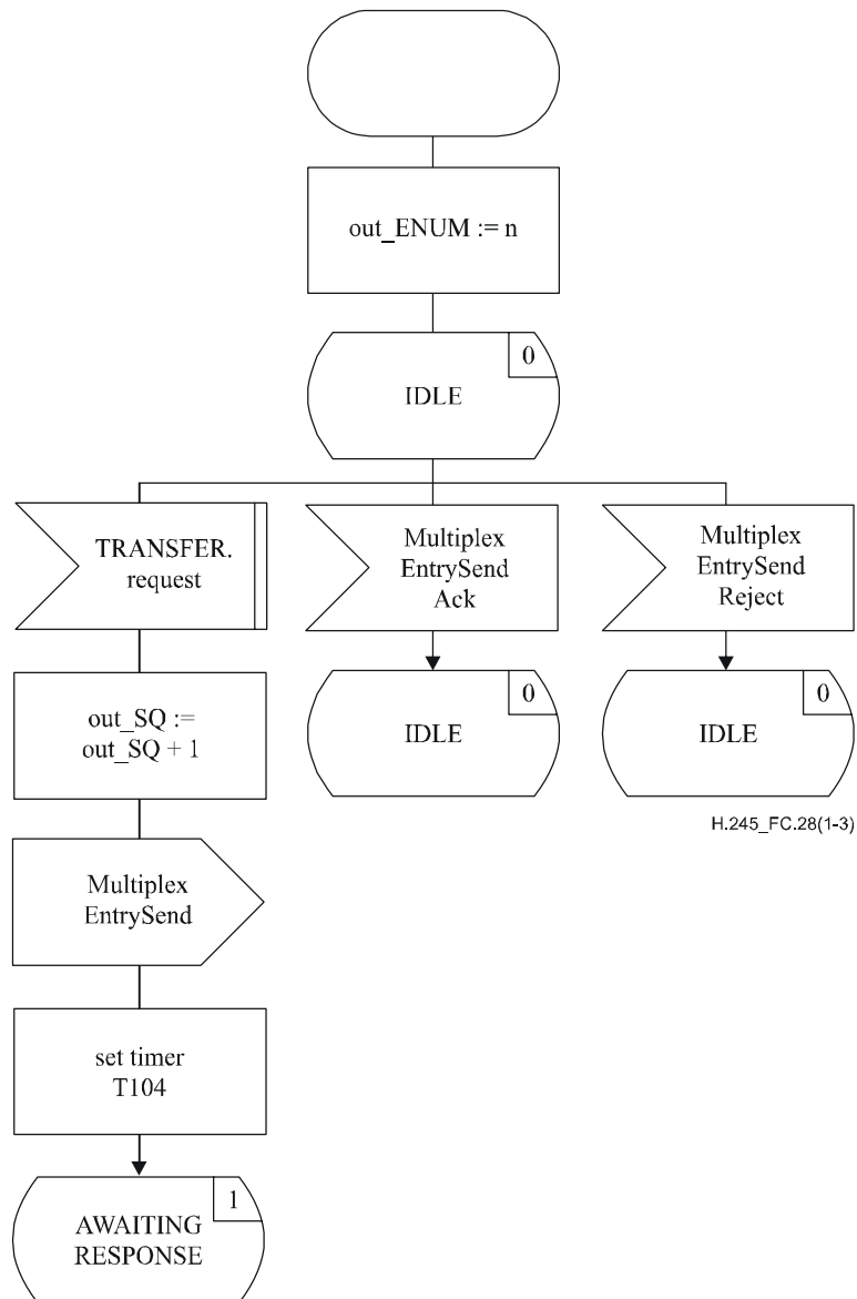
Figure C.28/H.245 – Diagramme SDL dans l'entité MTSE sortante (feuille 1 de 3)
