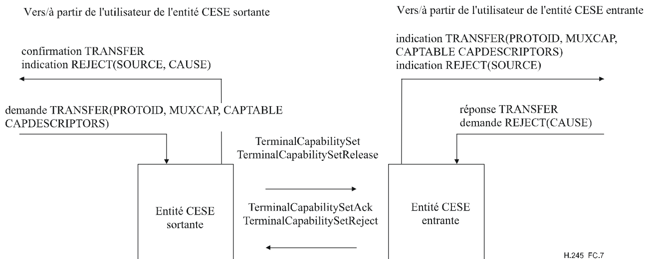
Figure C.7/H.245 – Primitives et messages dans l'entité de signalisation d'échange de capacités (CESE)
