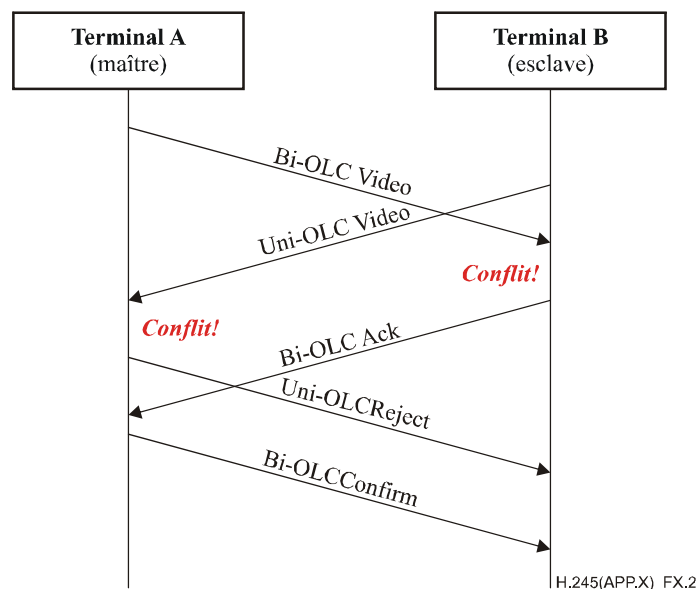
Figure X.2/H.245 – Le terminal maître propose des messages bidirectionnels d'ouverture OLC et le terminal esclave propose des messages unidirectionnels d'ouverture OLC
