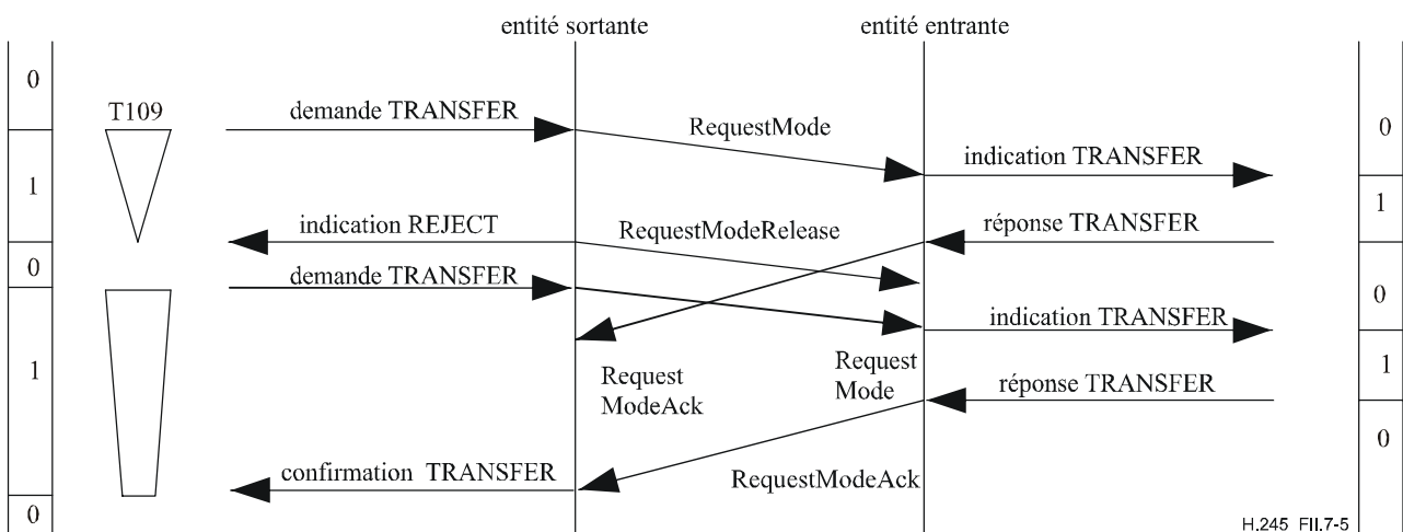
Figure II.7-4/H.245 – Demande de mode avec expiration de la temporisation T109
