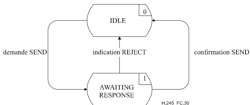
Figure C.30/H.245 – Diagramme de changement d'état pour la séquence de primitives dans l'entité RMESE sortante
