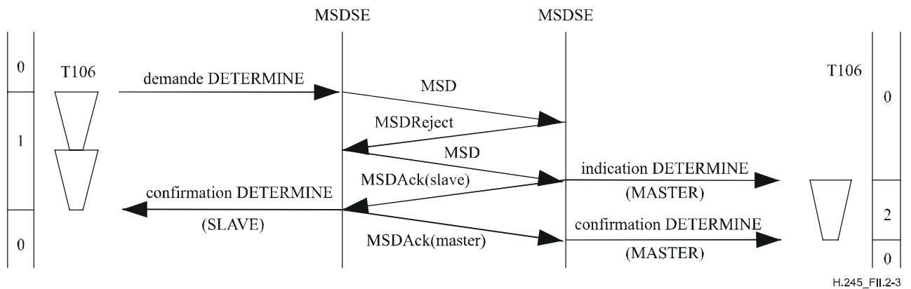
Figure II.2-3/H.245 – Désignation maître-esclave – La première tentative a donné un résultat indéterminé. La deuxième tentative a abouti
