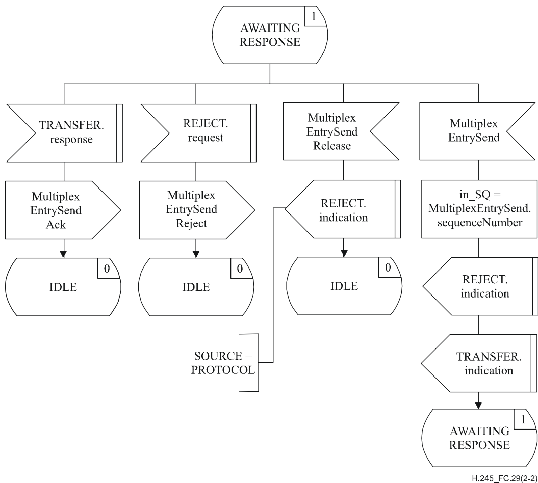
Figure C.29/H.245 – Diagramme SDL dans l'entité MTSE entrante (feuille 2 de 2)
