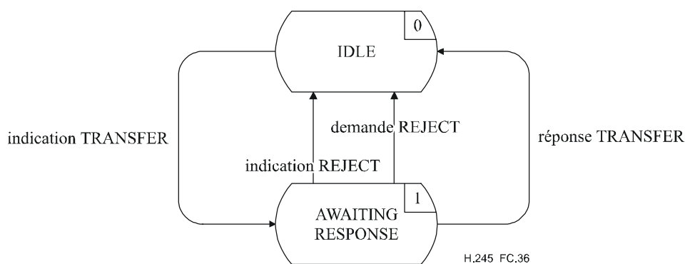
Figure C.36/H.245 – Diagramme de changement d'état pour la séquence de primitives de l'entité MRSE entrante
