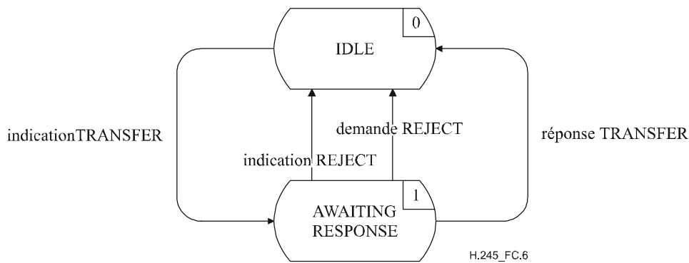
Figure C.6/H.245 – Diagramme de changement d'état pour la séquence de primitives d'une entité CESE entrante
