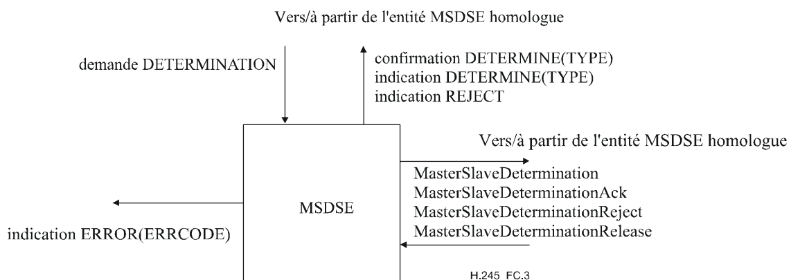
Figure C.3/H.245 – Primitives et messages dans l'entité MSDSE
