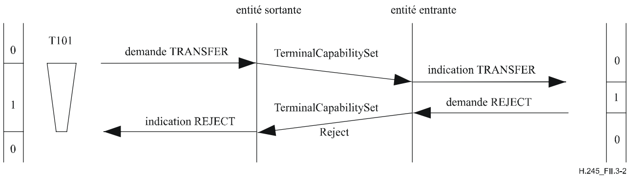
Figure II.3-2/H.245 – Echange de capacités avec rejet provenant de l'utilisateur de l'entité CESE homologue entrante
