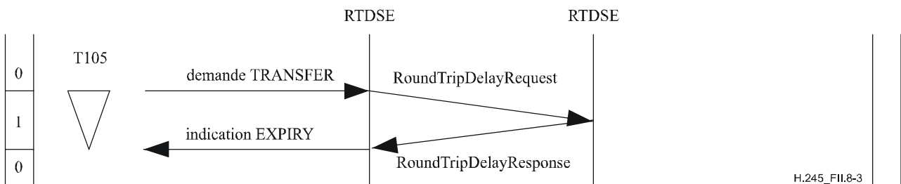
Figure II.8-3/H.245 – Procédure de détermination du temps de propagation aller et retour avec expiration de la temporisation T105
