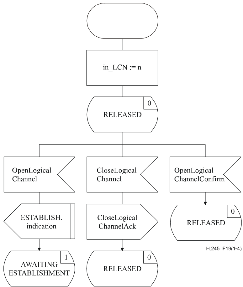
Figure C.19/H.245 – Diagramme SDL de l'entité B-LCSE entrante (feuille 1 de 4)
