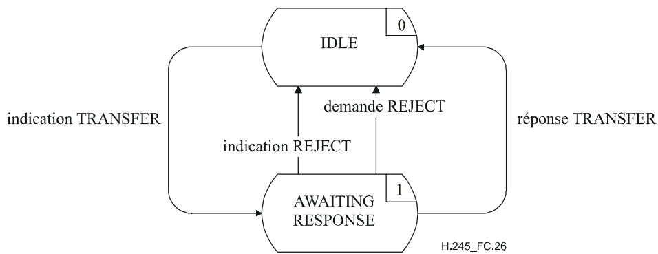
Figure C.26/H.245 – Diagramme de changement d'état pour la séquence de primitives dans l'entité MTSE entrante
