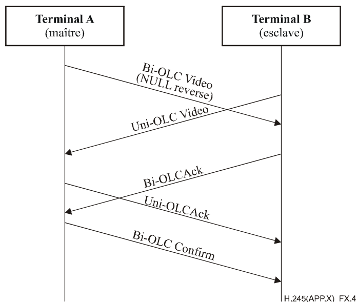
Figure X.4/H.245 – Le terminal maître propose des messages bidirectionnels d'ouverture OLC avec type nullData et le terminal esclave propose des messages unidirectionnels d'ouverture OLC
