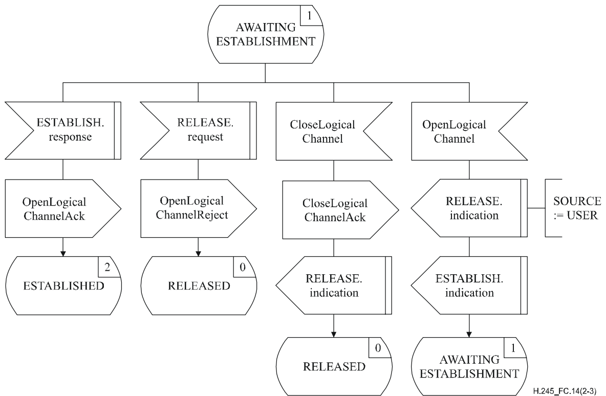
Figure C.14/H.245 – Diagramme SDL de l'entité LCSE entrante (feuille 2 de 3)
