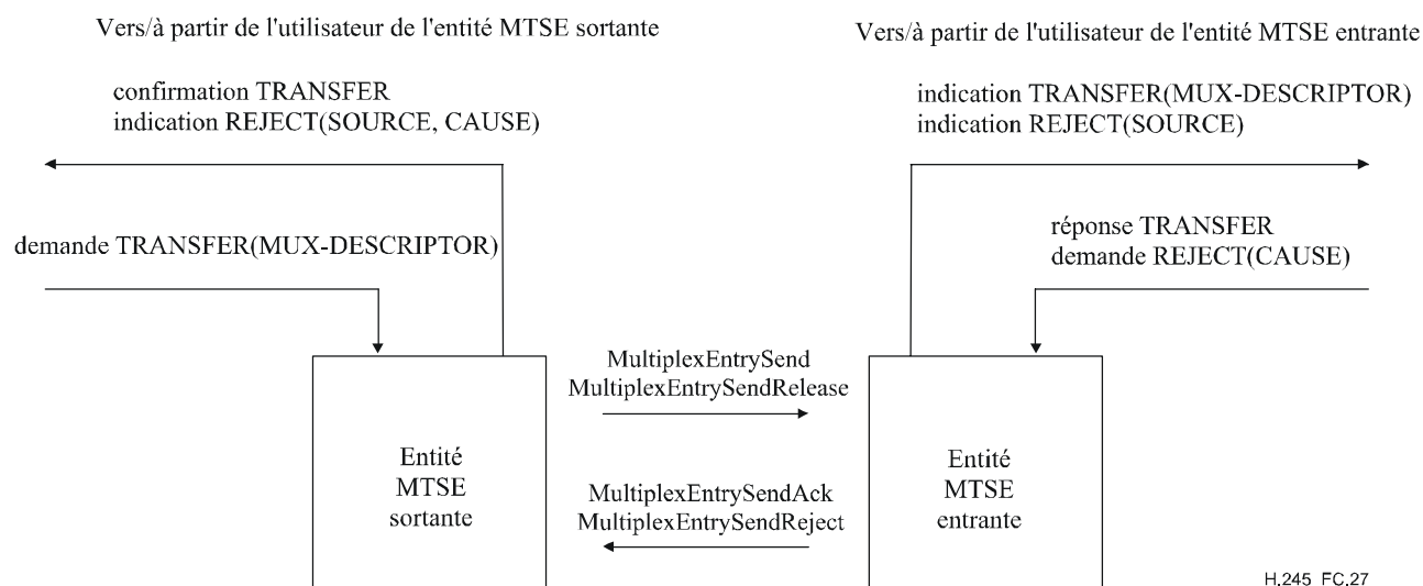
Figure C.27/H.245 – Primitives et messages dans l'entité de signalisation de tableau de multiplexage (MTSE)
