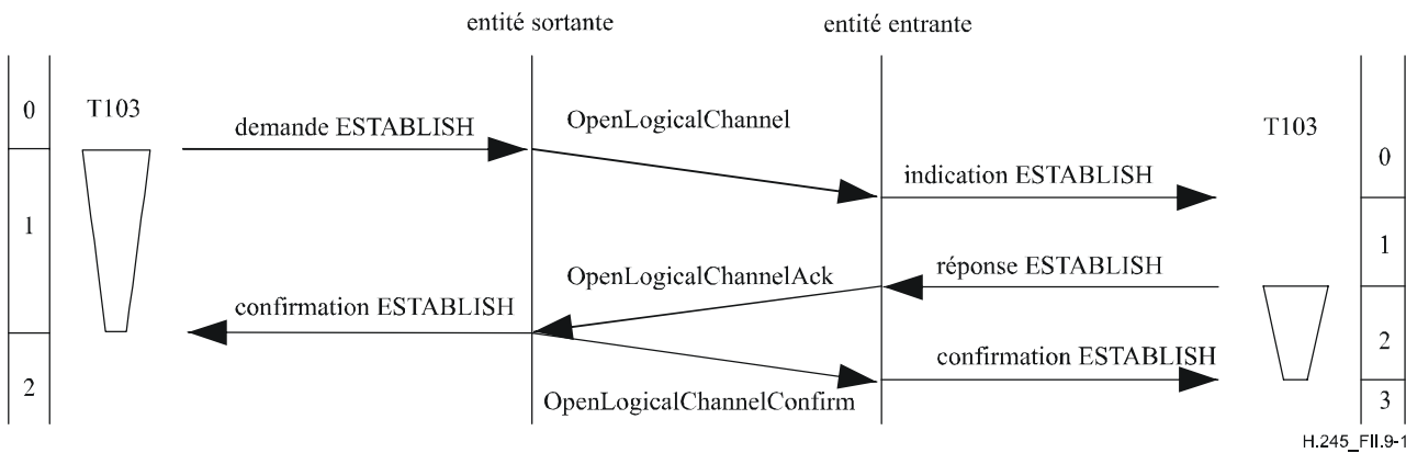
Figure II.9-1/H.245 – Etablissement de voie logique bidirectionnelle
