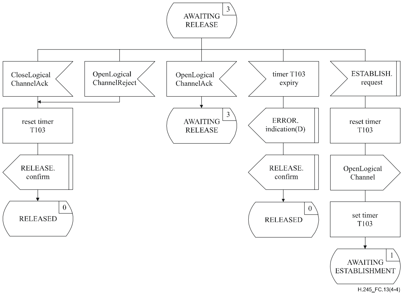
Figure C.13/H.245 – Diagramme SDL de l'entité LCSE sortante (feuille 4 de 4)
