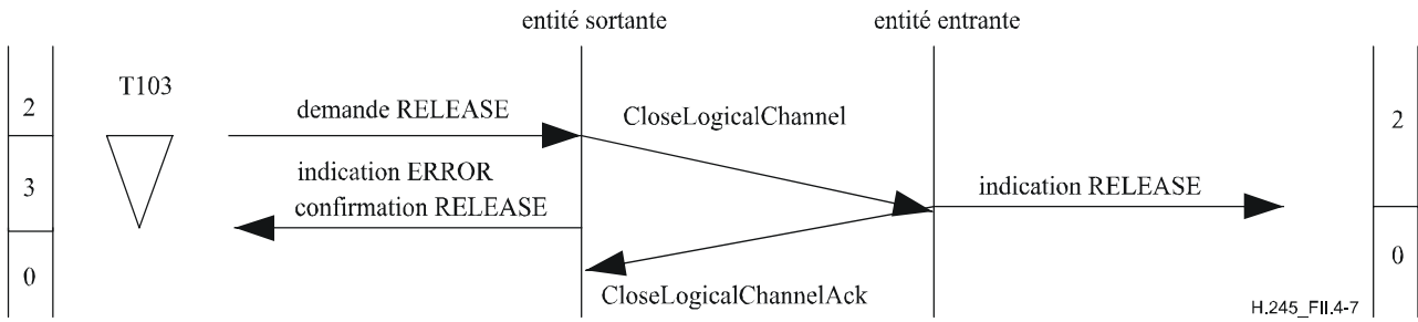
Figure II.4-7/H.245 – Demande de libération de voie logique avec expiration de la temporisation T103
