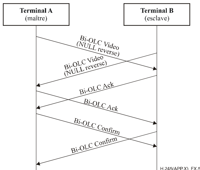
Figure X.5/H.245 – Les deux terminaux proposent des messages bidirectionnels d'ouverture OLC avec type nullData
