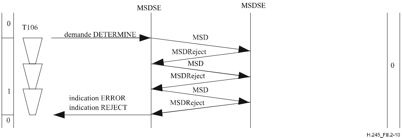
Figure II.2-10/H.245 – Désignation maître-esclave – Résultat indéterminé avec N100 = 3
