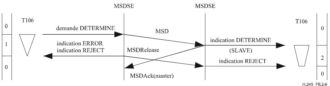
Figure II.2-6/H.245 – Désignation maître-esclave – Temporisation locale T106 à expiration avec terminal asservi du côté distant
