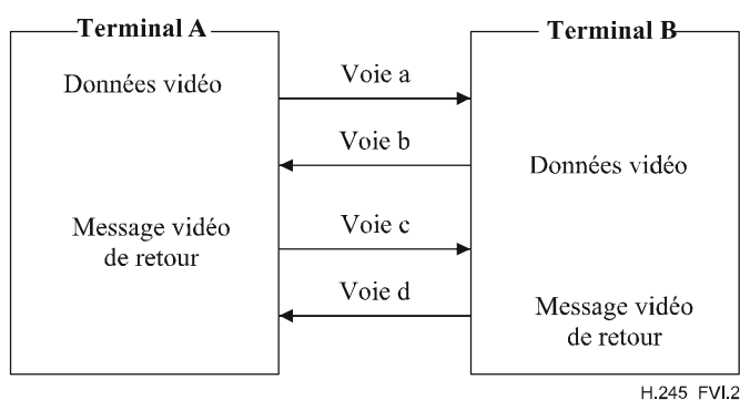
Figure VI.2/H.245 – Voies logiques pour le mode voie logique séparée
