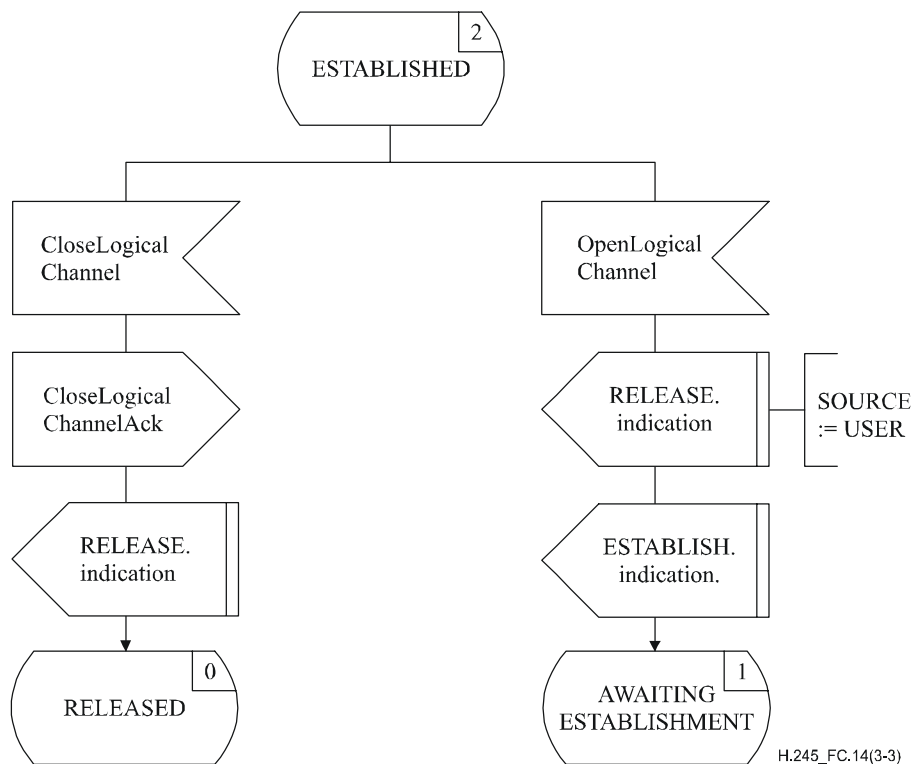
Figure C.14/H.245 – Diagramme SDL de l'entité LCSE entrante (feuille 3 de 3)
