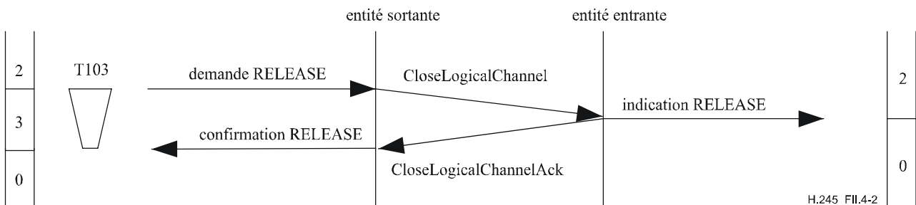
Figure II.4-2/H.245 – Libération de voie logique
