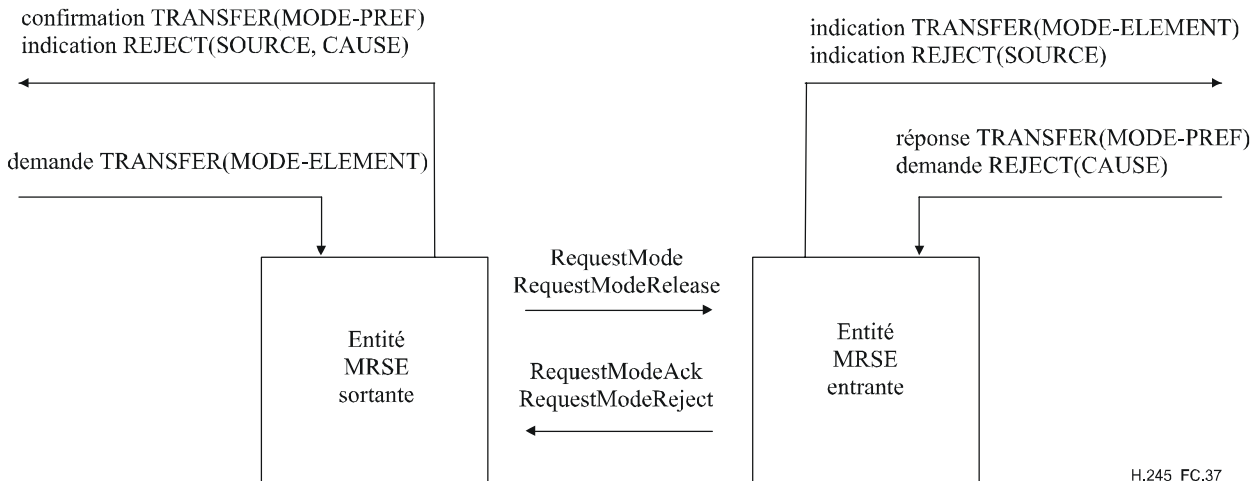
Figure C.37/H.245 – Primitives et messages dans l'entité de signalisation de demande de mode
