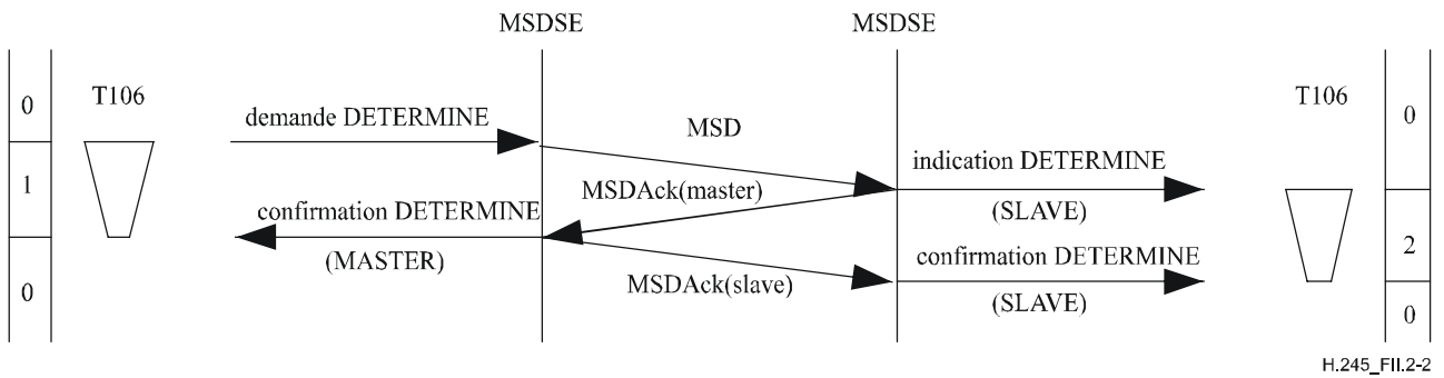
Figure II.2-2/H.245 – Désignation maître-esclave – Terminal asservi dans l'entité MSDSE distante
