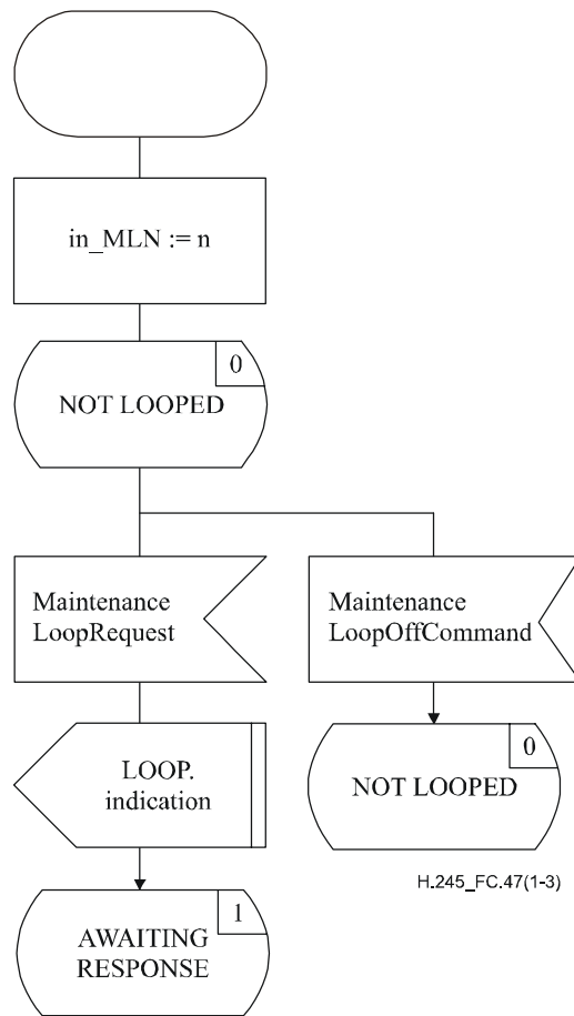
Figure C.47/H.245 – Diagramme SDL de l'entité MLSE entrante (feuille 1 de 3)
