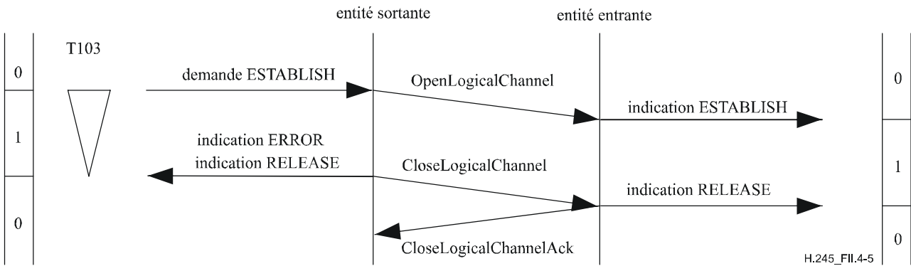
Figure II.4-5/H.245 – Demande d'établissement de voie logique avec expiration de la temporisation T103 en raison d'un retard de la réponse provenant de l'utilisateur d'entité LCSE homologue entrante
