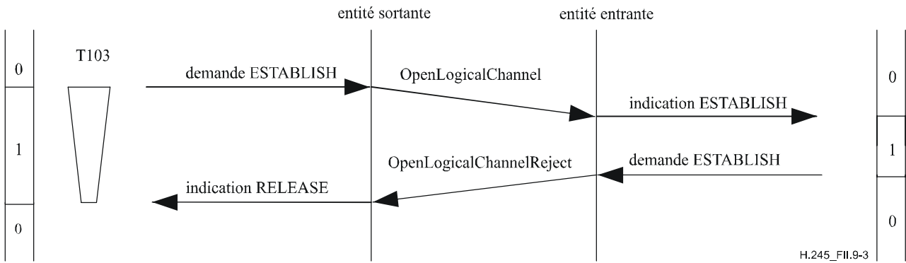
Figure II.9-3/H.245 – Rejet d'établissement de voie logique bidirectionnelle par l'utilisateur de l'entité B-LCSE homologue
