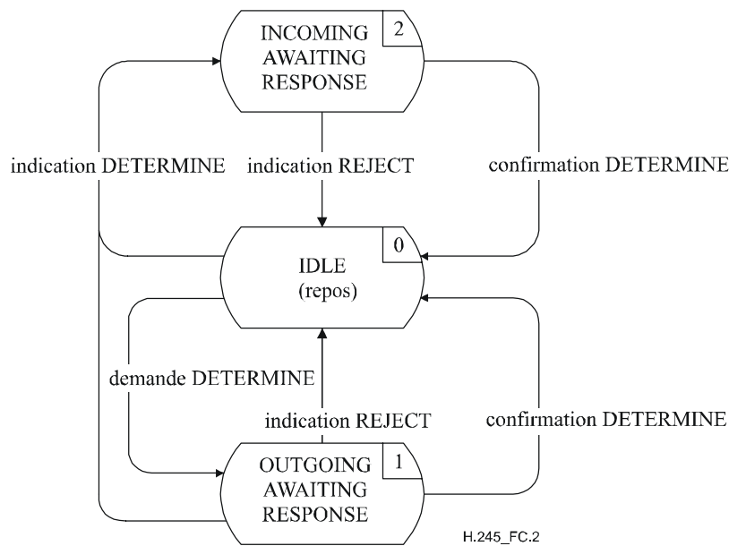
Figure C.2/H.245 – Diagramme de changement d'état pour la séquence de primitives dans l'entité MSDSE
