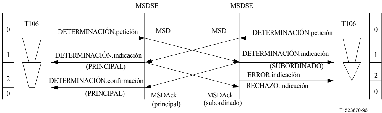
Figura II.2-9/H.245 – Determinación principal-subordinado – Procedimientos de determinación simultánea con expiración del temporizador T106 durante el estado ESPERA DE ACUSE DE RECIBO EN ENTRADA
