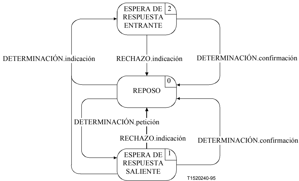
Figura C.2/H.245 – Diagrama de transición de estados para la secuencia de las primitivas en la MSDSE
