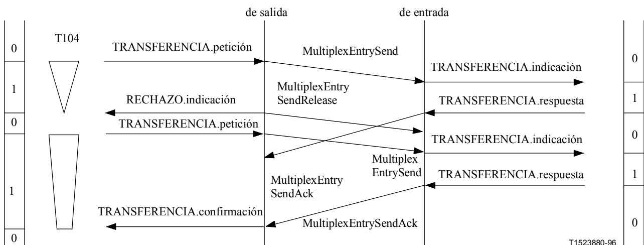
Figura II.6-5/H.245 – Petición de envío de tabla múltiplex con expiración del temporizador T104 seguida de una segunda petición de envío de tabla múltiplex
