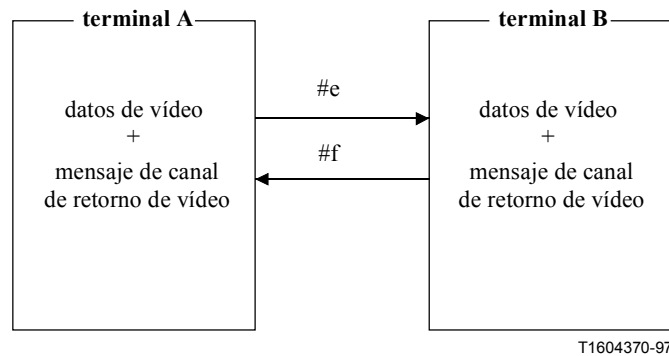
Figura VI.3/H.245 – Canales lógicos para modo múltiplex de vídeo
