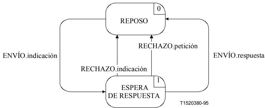
Figura C.31/H.245 – Diagrama de transición de estados para la secuencia de primitivas en una RMESE de entrada
