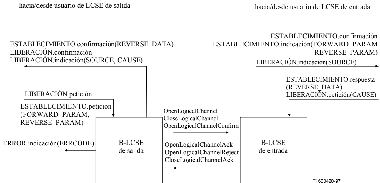
Figura C.17/H.245 – Primitivas y mensajes en la entidad de señalización de canal lógico bidireccional
