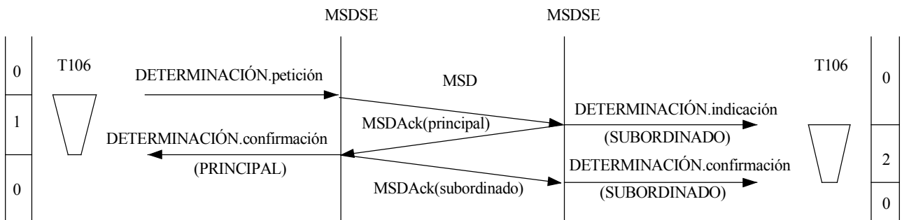
Figura II.2-2/H.245 – Determinación principal-subordinado – Subordinado en la MSDSE distante
