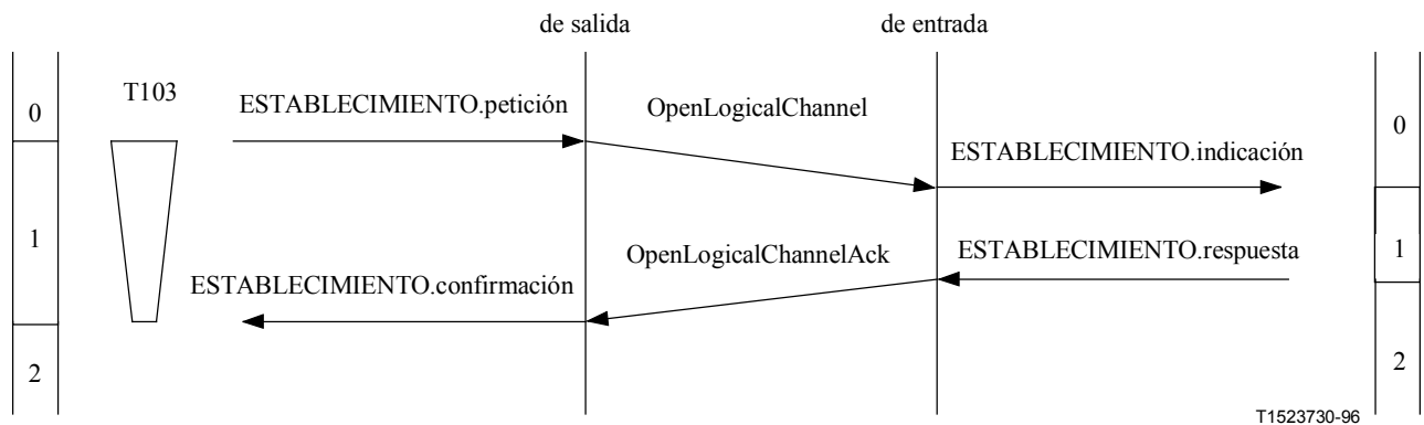
Figura II.4-1/H.245 – Establecimiento de canal lógico
