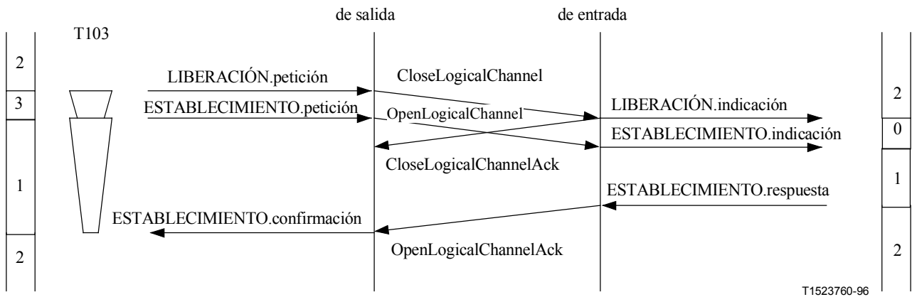
Figura II.4-4/H.245 – Liberación de canal lógico seguida de nuevo establecimiento inmediato
