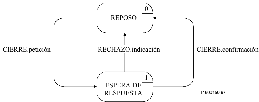
Figura C.20/H.245 – Diagrama de transición de estados para la secuencia de primitivas en una CLCSE de salida
