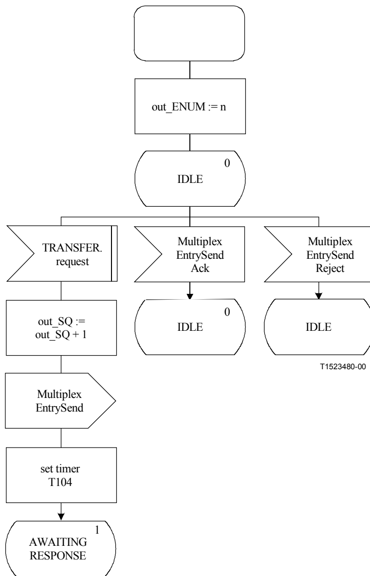
Figura C.28/H.245 – Diagrama SDL de la MTSE de salida (hoja 1 de 3)
