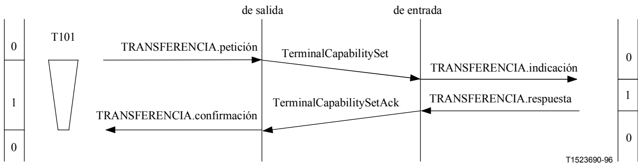
Figura II.3-1/H.245 – Intercambio de capacidades con aceptación por el usuario de la CESE de entrada par
