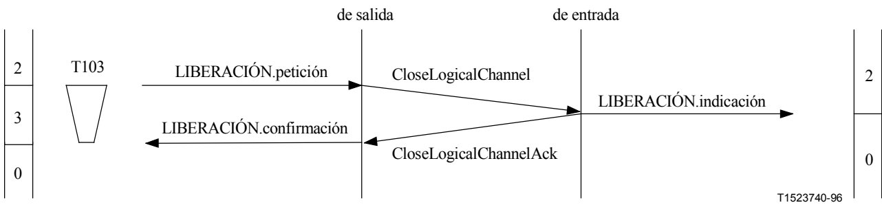
Figura II.4-2/H.245 – Liberación de canal lógico
