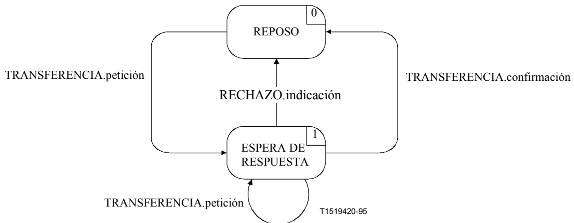
Figura C.25/H.245 – Diagrama de transición de estados para la secuencia de primitivas en una MTSE de salida
