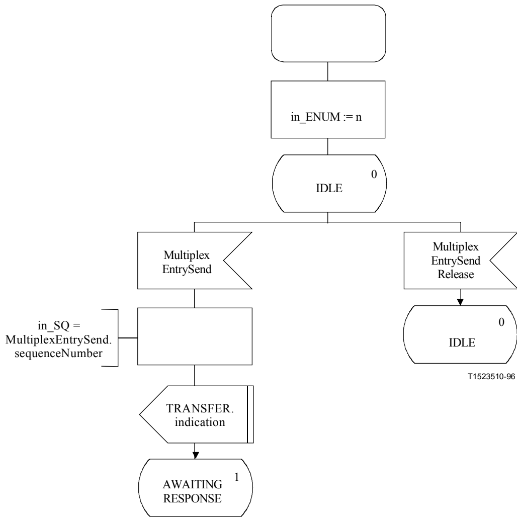
Figura C.29/H.245 – Diagrama SDL de la MTSE de entrada (hoja 1 de 2)
