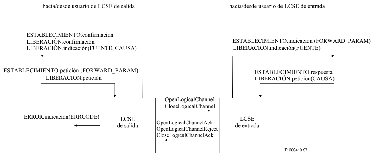
Figura C.12/H.245 – Primitivas y mensajes en la entidad de señalización de canal lógico
