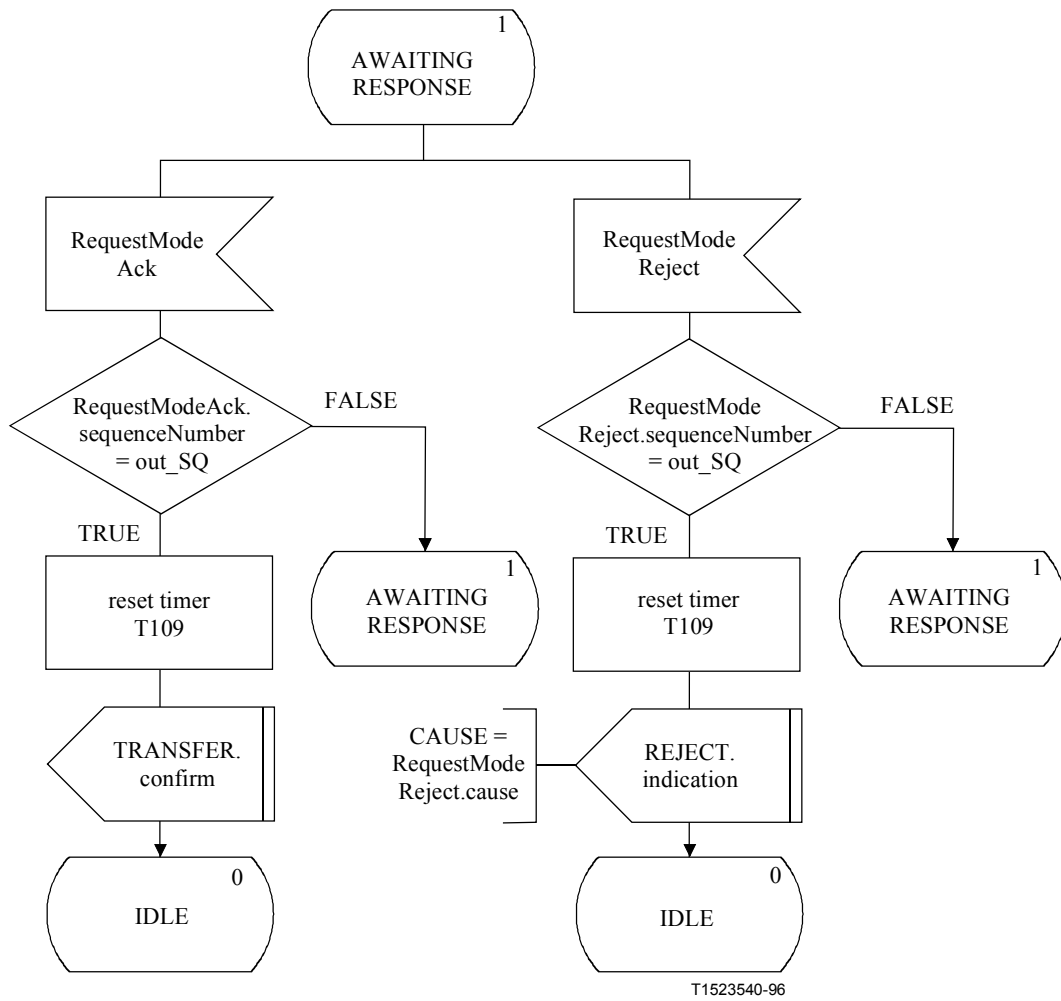
Figura C.38/H.245 – Diagrama SDL de la MRSE de salida (hoja 2 de 3)
