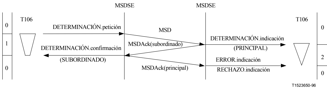
Figura II.2-7/H.245 – Determinación principal-subordinado – Expiración del temporizador distante T106 con director en el extremo distante
