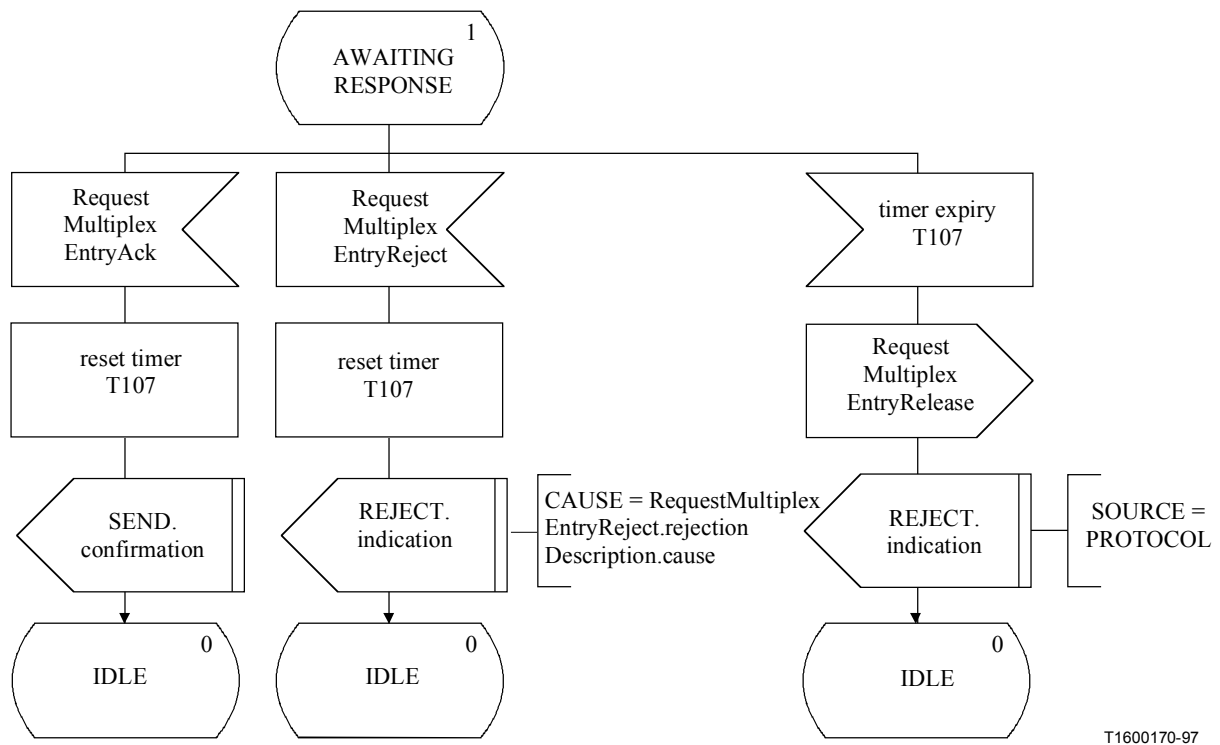
Figura C.33/H.245 – Diagrama SDL de la RMESSE de salida (hoja 2 de 2)
