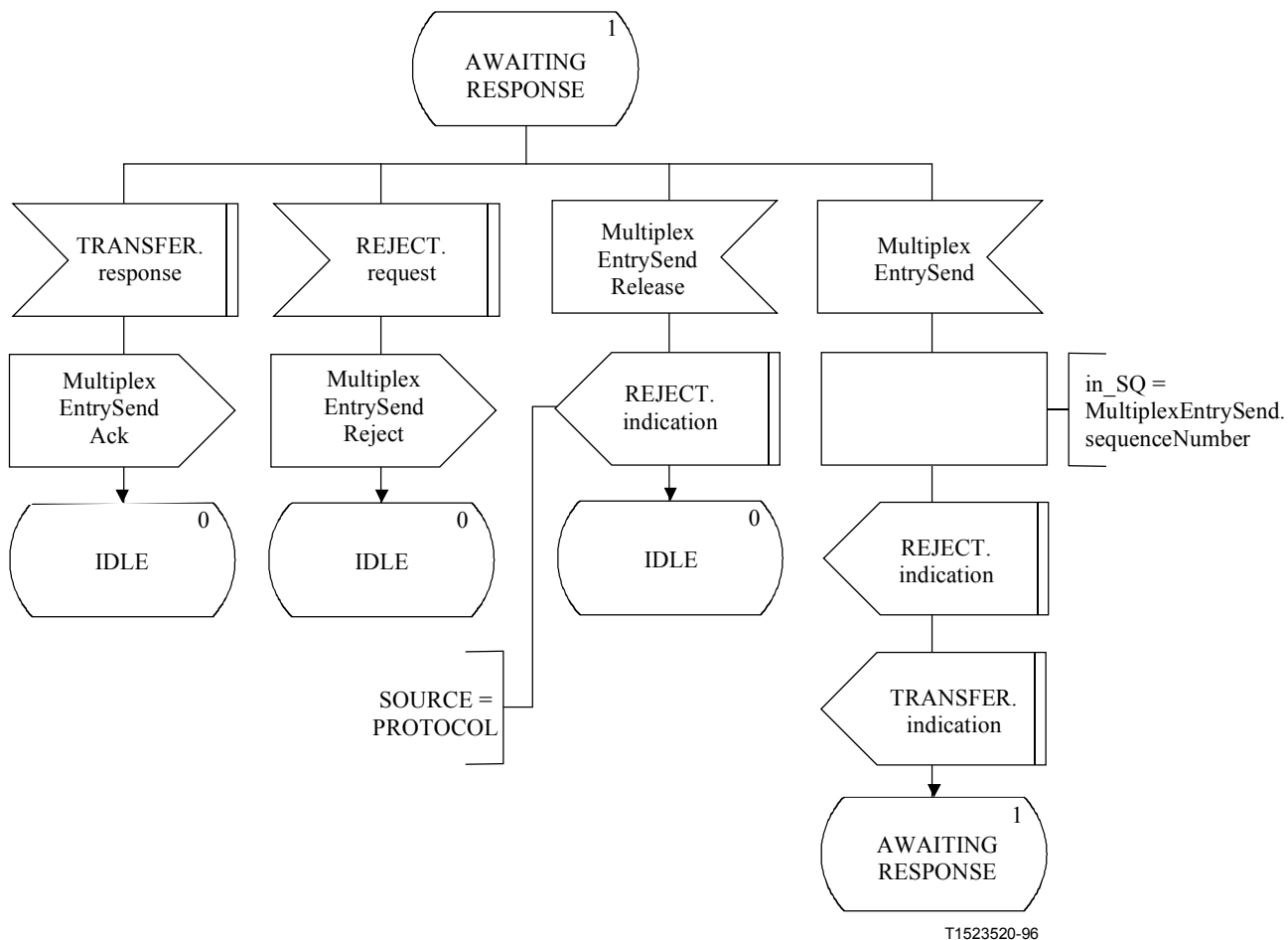
Figura C.29/H.245 – Diagrama SDL de la MTSE de entrada (hoja 2 de 2)
