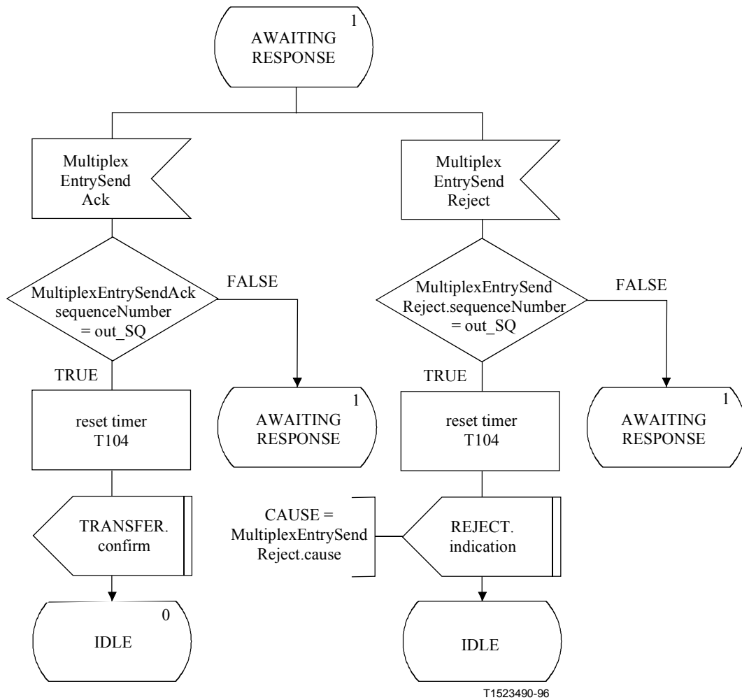
Figura C.28/H.245 – Diagrama SDL de la MTSE de salida (hoja 2 de 3)
