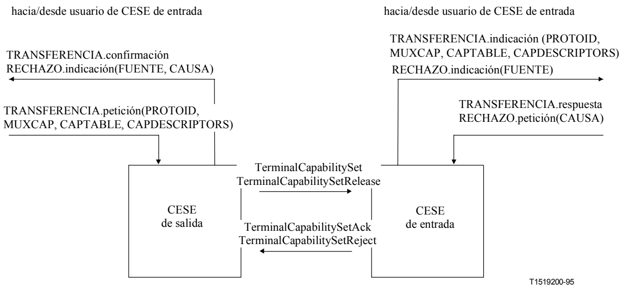
Figura C.7/H.245 – Primitivas y mensajes en la entidad de señalización de intercambio de capacidad
