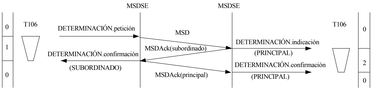
Figura II.2-1/H.245 – Determinación principal-subordinado – Principal en la MSDSE distante
