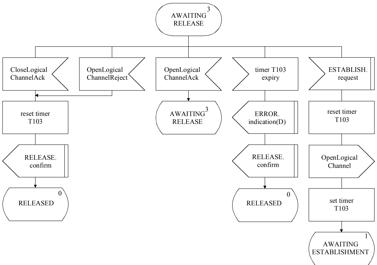
Figura C.18/H.245 – Diagrama SDL de la B-LCSE de salida (hoja 4 de 4)
