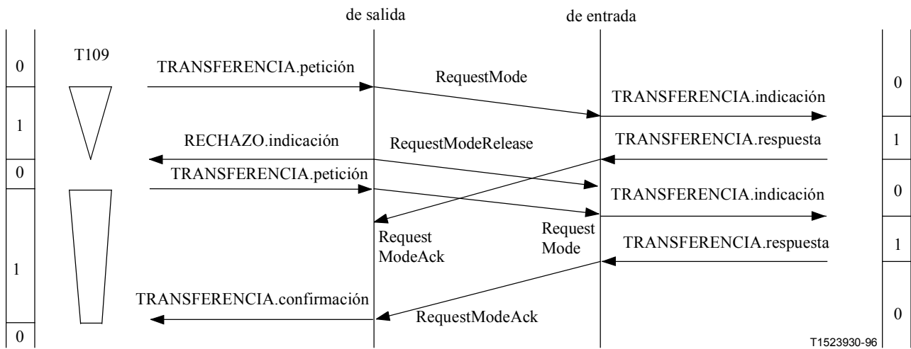
Figura II.7-5/H.245 – Petición de modo con expiración del temporizador T109 seguida de una segunda petición de modo
