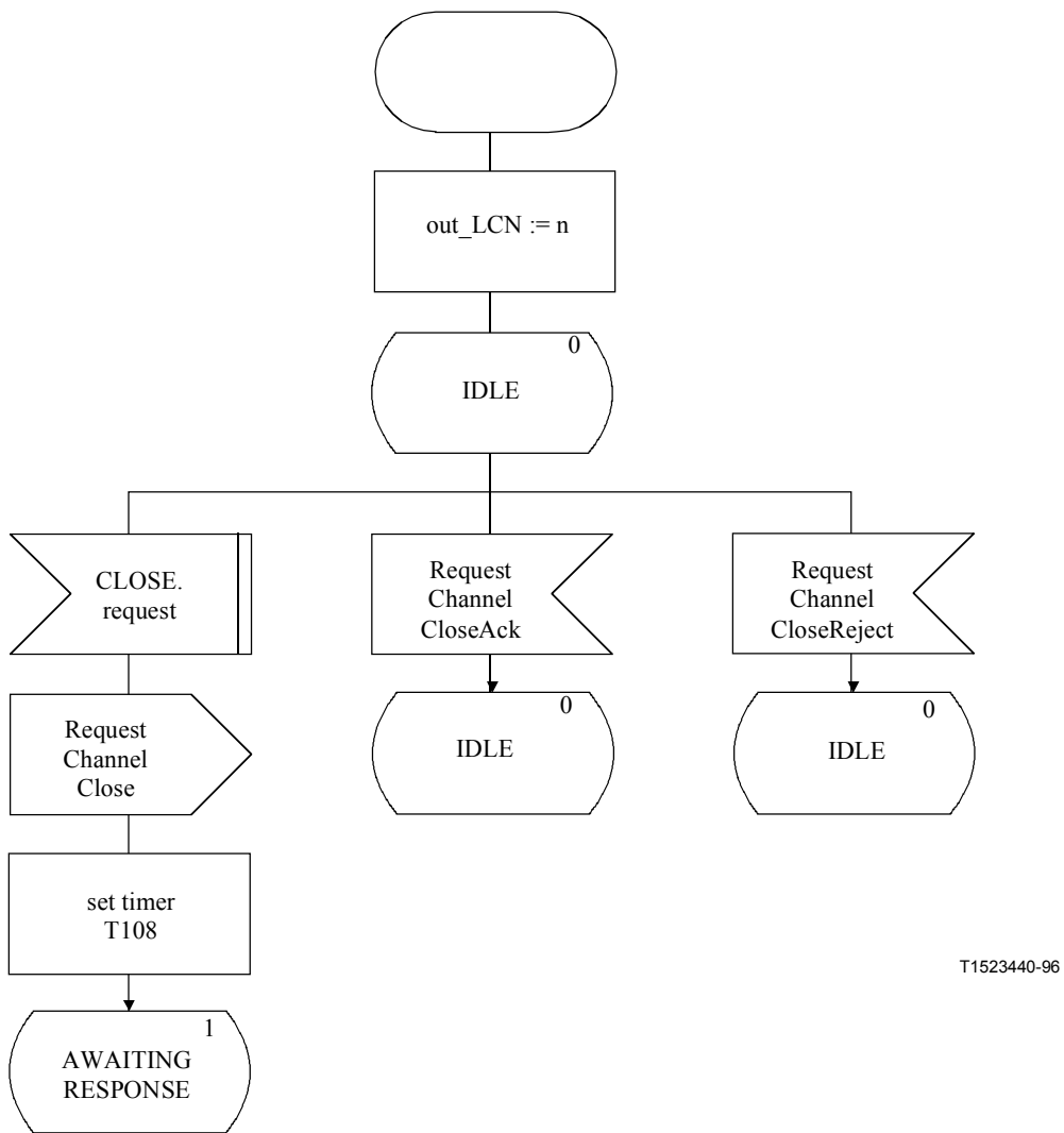
Figura C.23/H.245 – Diagrama SDL de la CLCSE de salida (hoja 1 de 2)
