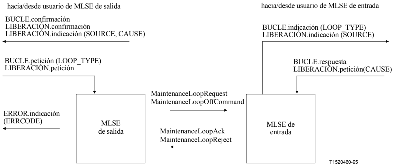
Figura C.45/H.245 – Primitivas y mensajes en la entidad de señalización de bucle de mantenimiento
