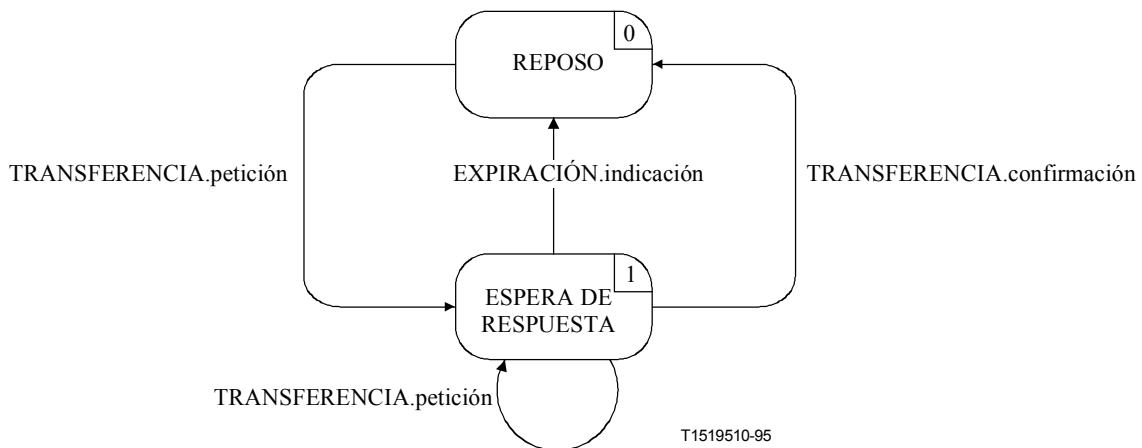
Figura C.40/H.245 – Diagrama de transición de estados para la secuencia de primitivas en la RTDSE
