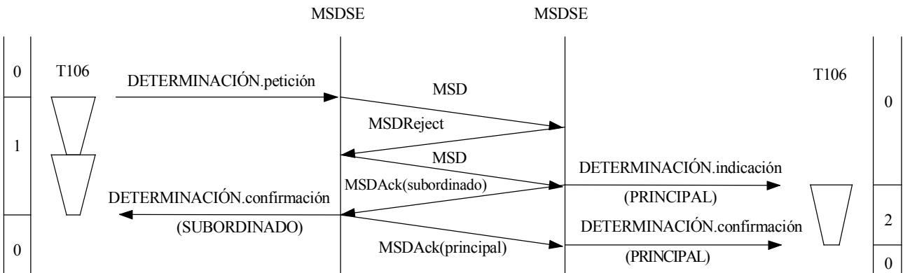
Figura II.2-3/H.245 – Determinación principal-subordinado – El primer intento produjo un resultado indeterminado. El segundo intento tuvo éxito
