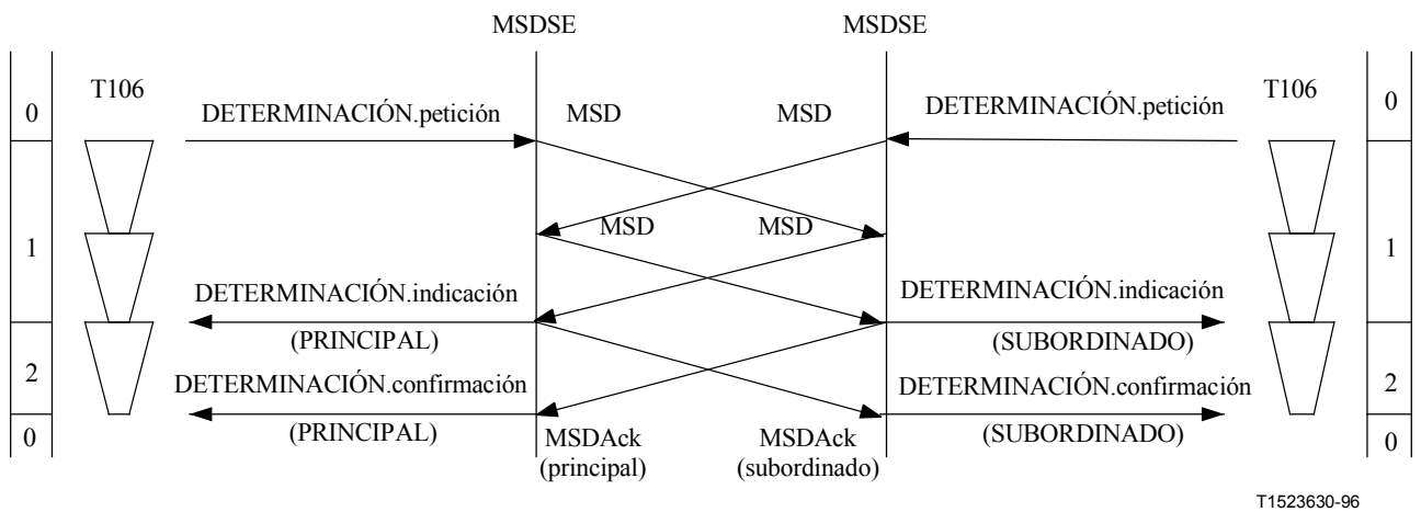
Figura II.2-5/H.245 – Determinación principal-subordinado – Determinación simultánea, pero el primer intento produce un resultado indeterminado
