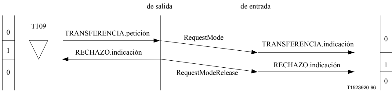
Figura II.7-4/H.245 – Petición de modo con expiración del temporizador T109
