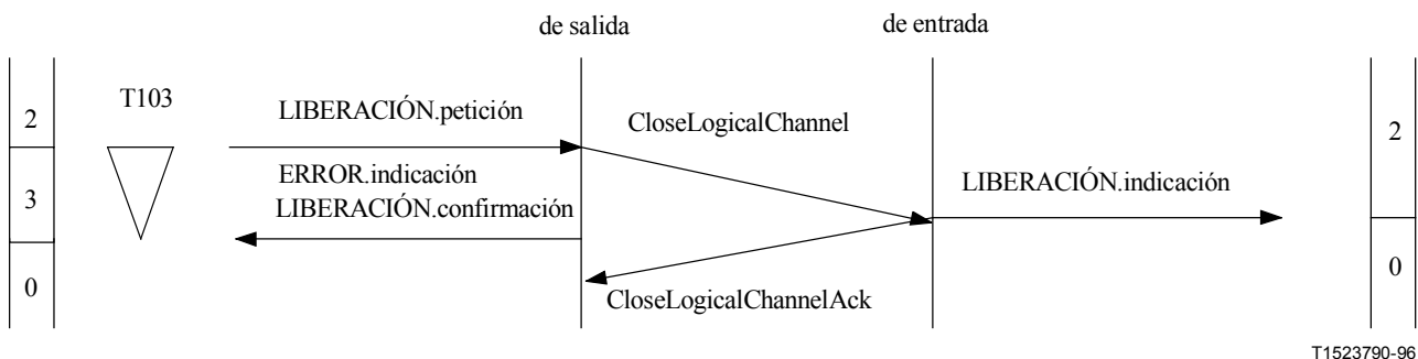
Figura II.4-7/H.245 – Petición de liberación de canal lógico con expiración del temporizador T103
