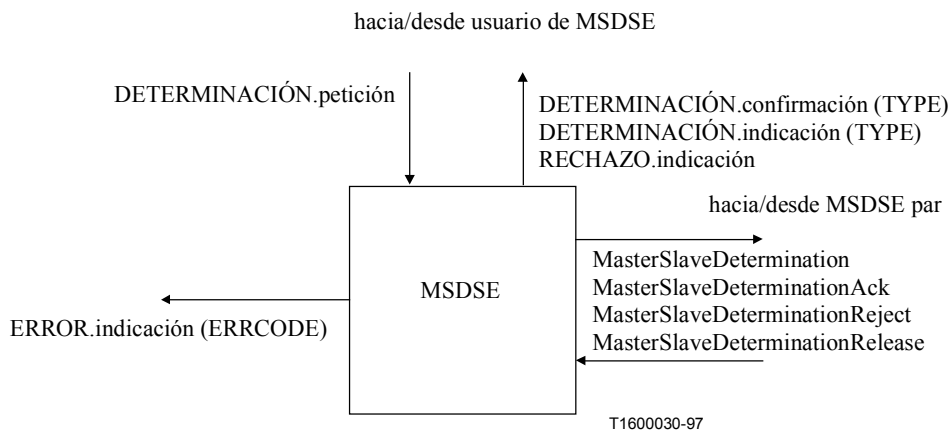
Figura C.3/H.245 – Primitivas y mensajes en la MSDSE
