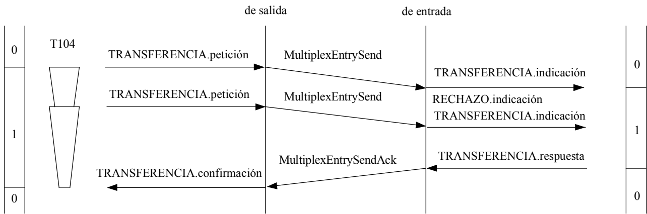
Figura II.6-3/H.245 – Petición de envío de tabla múltiplex con una segunda petición de envío de tabla múltiplex antes del acuse de recibo de la primera petición
