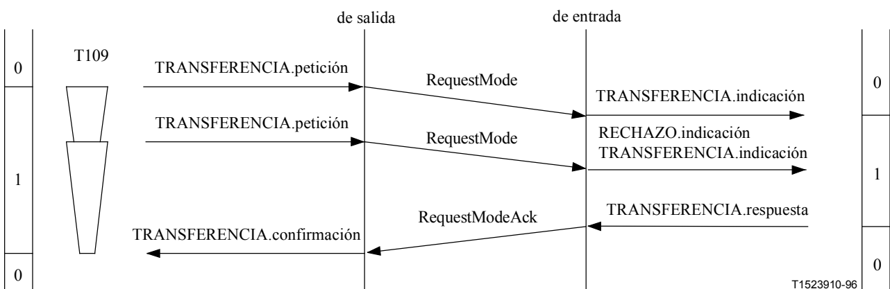
Figura II.7-3/H.245 – Petición de modo con una segunda petición de modo antes del acuse de recibo de la primera petición
