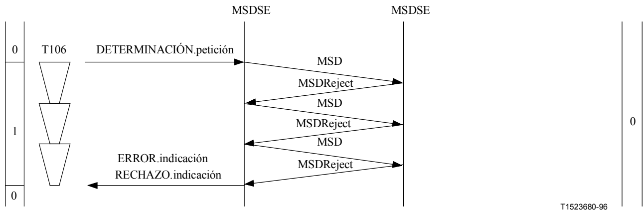
Figura II.2-10/H.245 – Determinación principal-subordinado – Resultado indeterminado con N100 = 3
