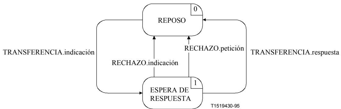
Figura C.26/H.245 – Diagrama de transición de estados para la secuencia de primitivas en una MTSE de entrada
