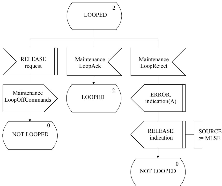
Figura C.46/H.245 – Diagrama SDL de la MLSE de salida (hoja 3 de 3)
