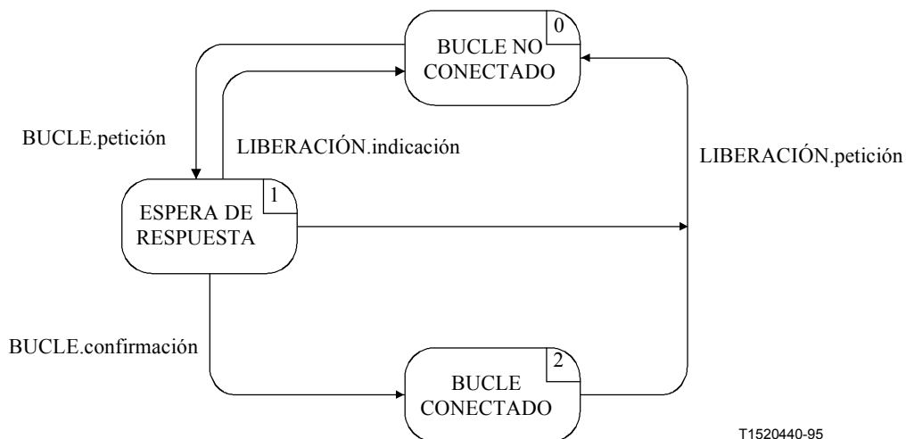
Figura C.43/H.245 – Diagrama de transición de estados para la secuencia de primitivas en la MLSE de salida
