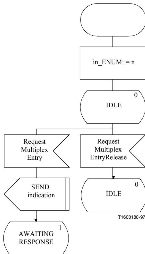
Figura C.34/H.245 – Diagrama SDL de la RMESSE de entrada (hoja 1 de 2)
