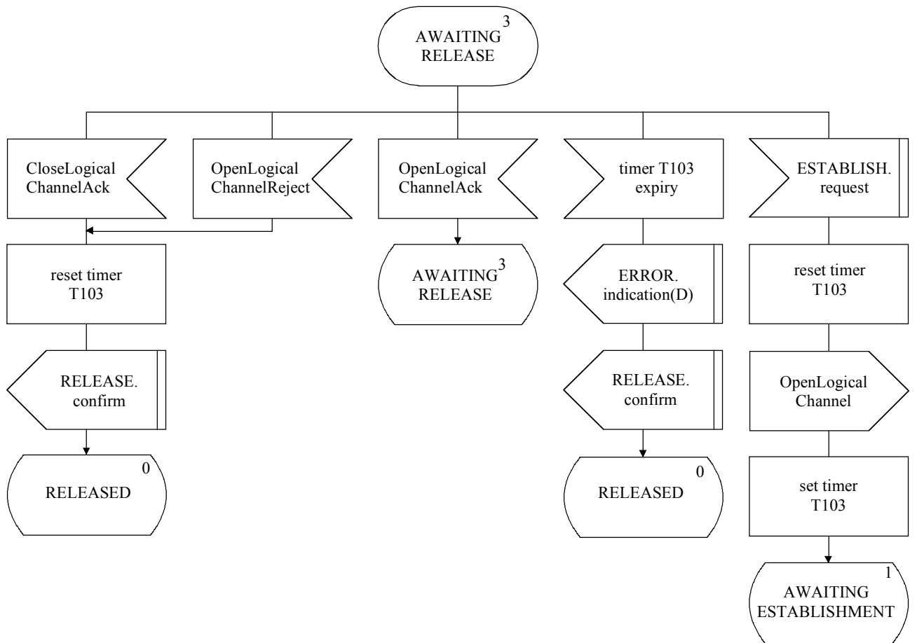
Figura C.13/H.245 – Diagrama SDL de la LCSE de salida (hoja 4 de 4)
