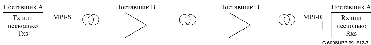
Рисунок 12-3 – Частичная поперечная совместимость физического уровня с многими пролетами
