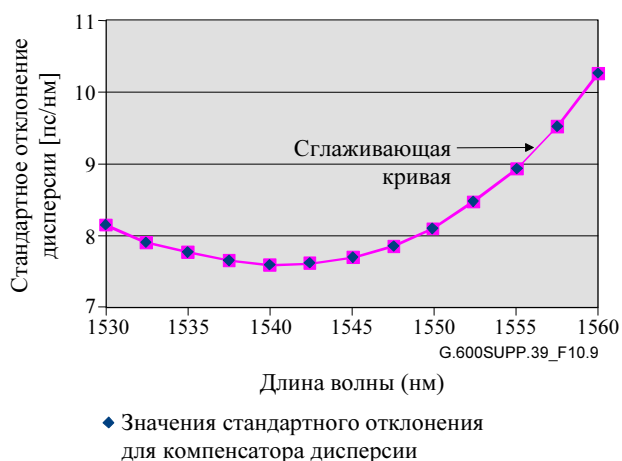
Рисунок 10-9 – Значения стандартного отклонения для компенсатора дисперсии
