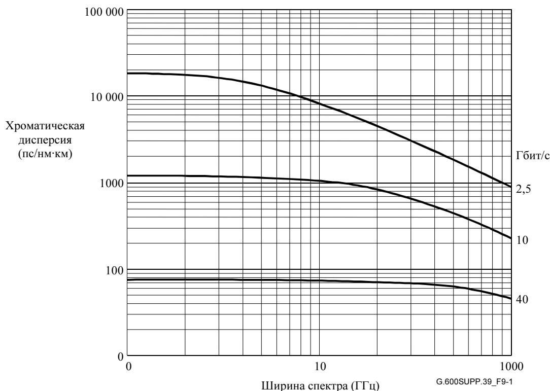
Рисунок 9-1 – Максимальная допустимая хроматическая дисперсия в зависимости от ширины спектра источника на 1550 нм для некоторых битовых скоростей NRZ без частотной модуляции при ухудшении по мощности 1 дБ
