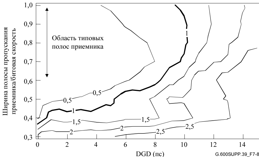
Рисунок 7-8 – Контурная схема для допуска на DGD (RZ-50%)
