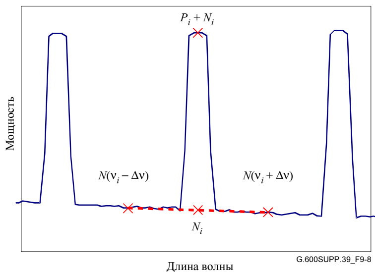
Рисунок 9-8 – Измерение OSNR в оптическом спектре
