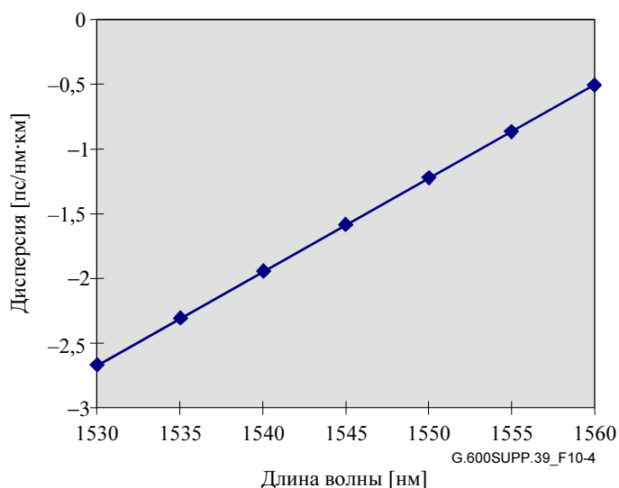
Рисунок 10-4 – Зависимость среднего коэффициента дисперсии от длины волны
