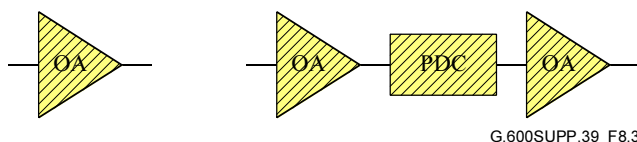
Рисунок 8-3 – Примеры схем реализации регенератора 1R
