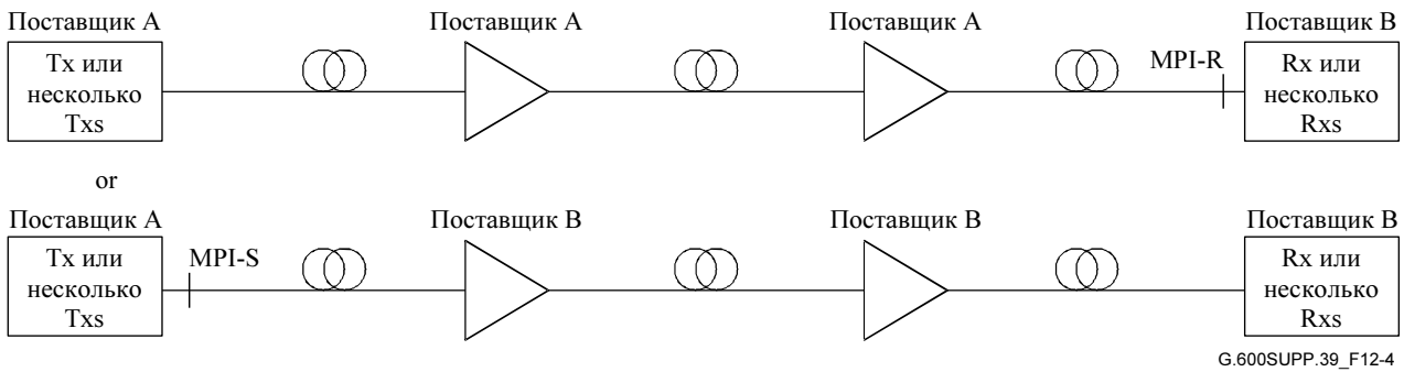
Рисунок 12-4 – Поперечная совместимость при одном интерфейсе и многих пролетах
