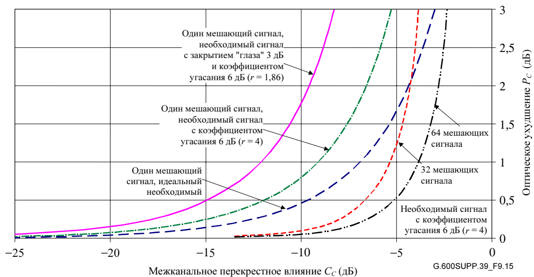
Рисунок 9-15 – График оптического ухудшения в зависимости от межканального перекрестного влияния
