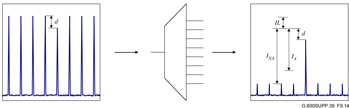
Рисунок 9-14 – Более реалистичный пример демультиплексора
