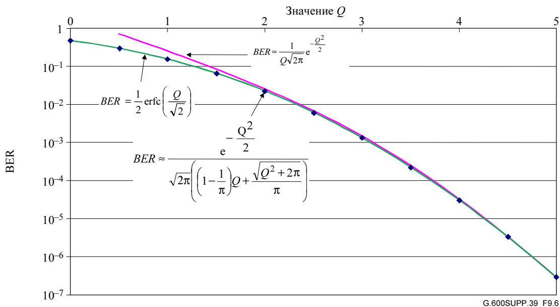
Рисунок 9-6 – Аппроксимации отношения КОБ и Q
