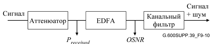
Рисунок 9-10 – Организация измерения OSNR
