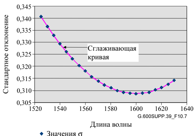
Рисунок 10-7 – Стандартное отклонение коэффициента хроматической дисперсии для волокна G.652
