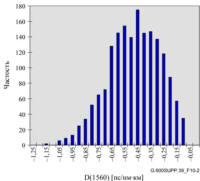
Рисунок 10-2 – Гистограмма значений коэффициента дисперсии на 1560 нм
