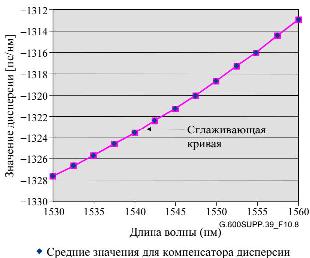
Рисунок 10-8 – Среднее значение для компенсатора дисперсии
