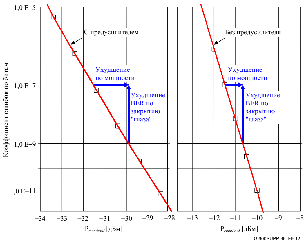
Рисунок 9-12 – Зависимость КОБ от принимаемой оптической мощности с оптическим предусилителем и без него
