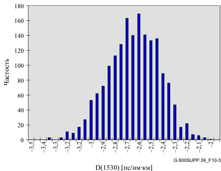
Рисунок 10-3 – Гистограмма значений коэффициента дисперсии на 1530 нм
