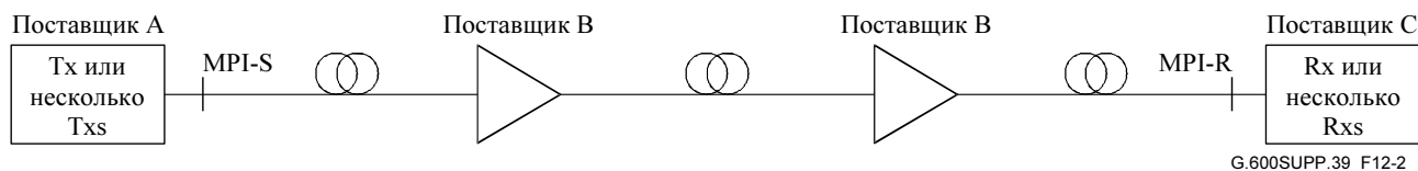
Рисунок 12-2 – Поперечная совместимость физического уровня с многими пролетами
