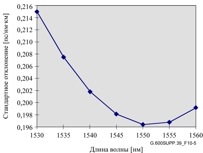
Рисунок 10-5 – Зависимость стандартного отклонения коэффициента дисперсии от длины волны
