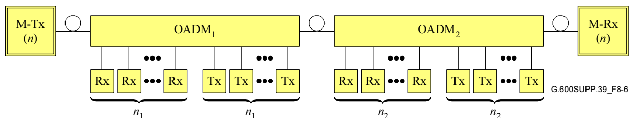
Рисунок 8-6 – Пример структуры "шина" с двумя OADM и с одним волокном для каждого добавляемого/ответвляемого канала WDM
