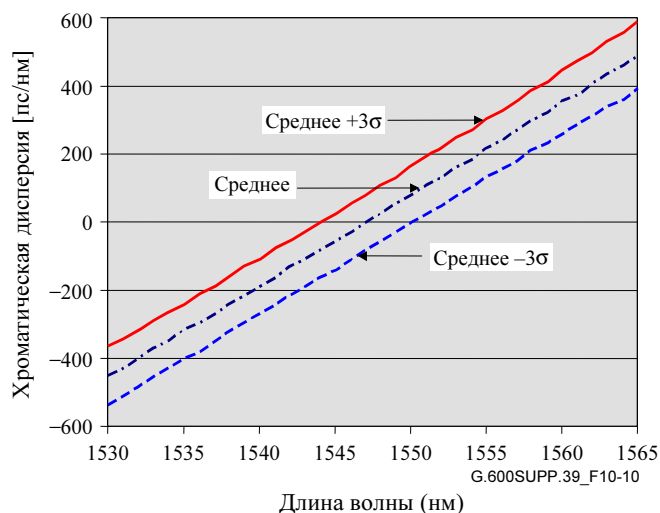
Рисунок 10-10 – Пределы 3 σ для комбинации волокна G.652 и компенсаторов
