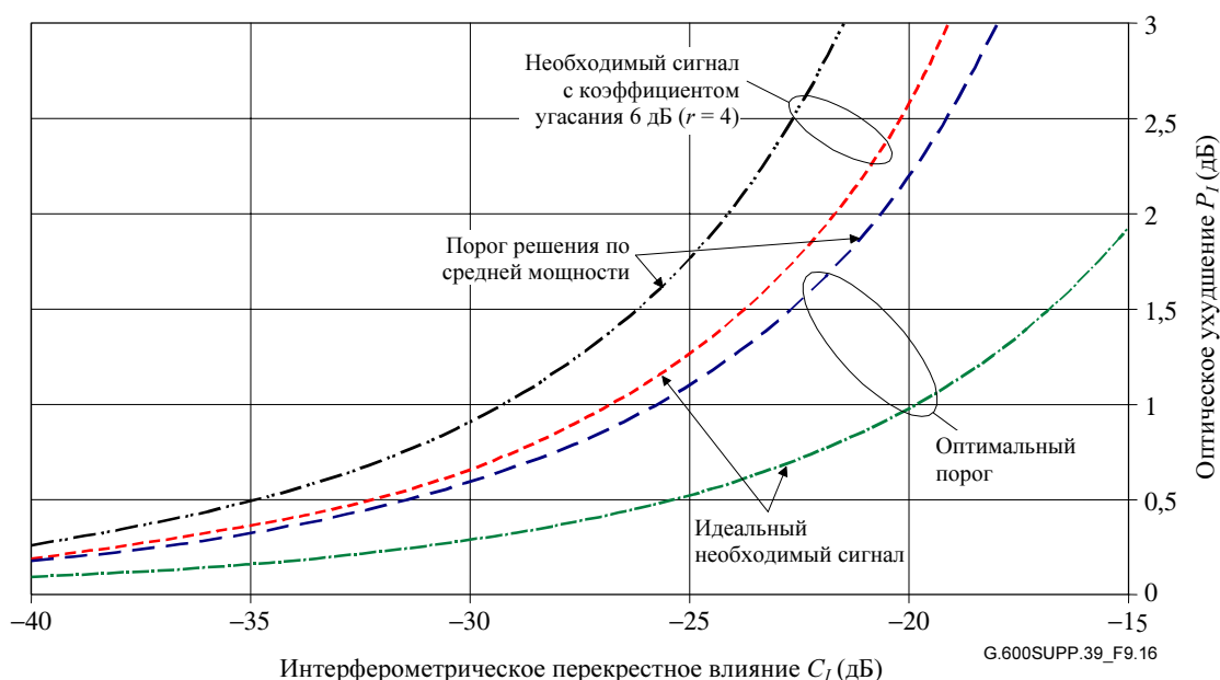
Рисунок 9-16 – График оптического ухудшения в зависимости от интерферометрического перекрестного влияния при одном мешающем сигнале (ограниченная модель)
