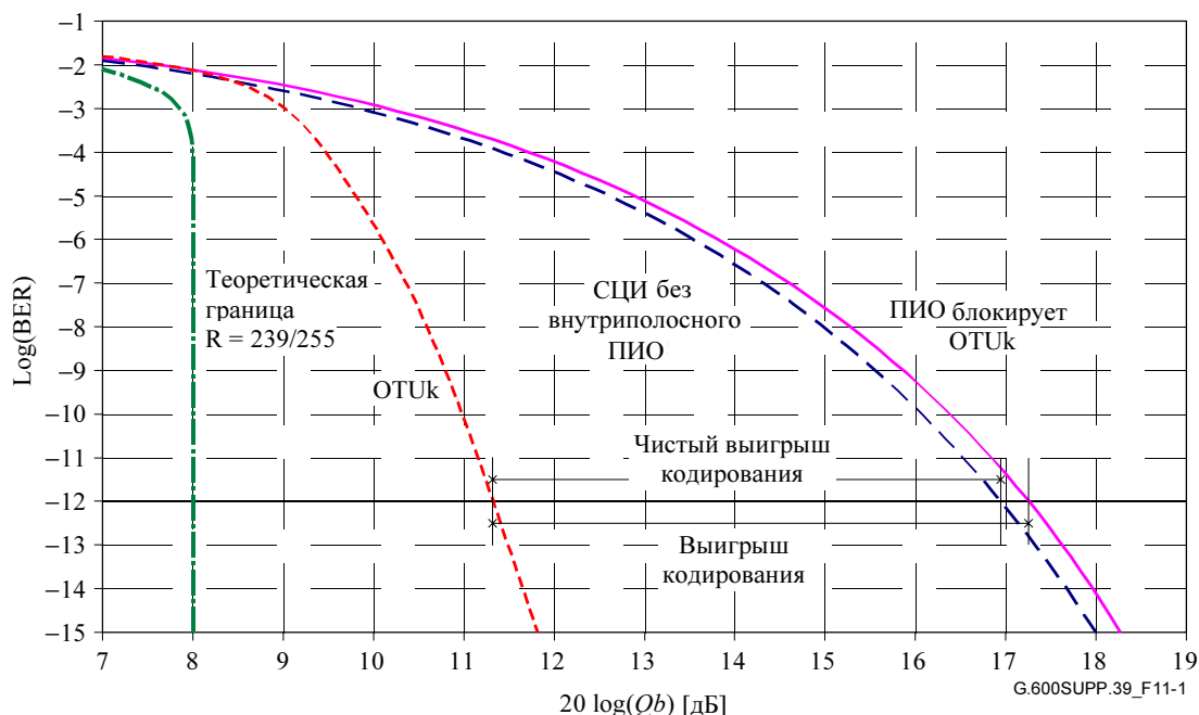
Рисунок 11-1 – Расчет рабочих характеристик схемы ПИО из G.709/Y.1331
