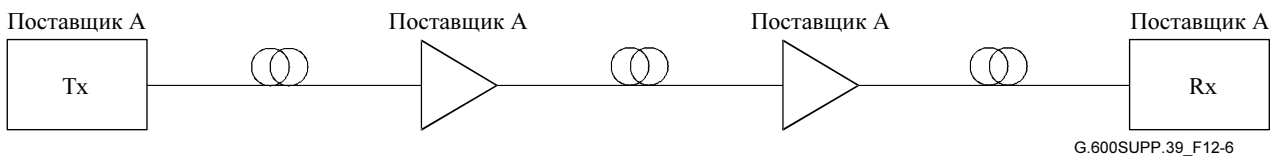
Рисунок 12-6 – Продольная совместимость физического уровня с многими участками
