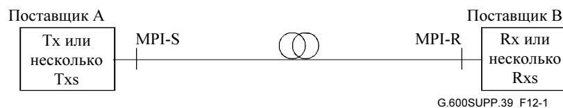
Рисунок 12-1 – Поперечная совместимость физического уровня с одним пролетом
