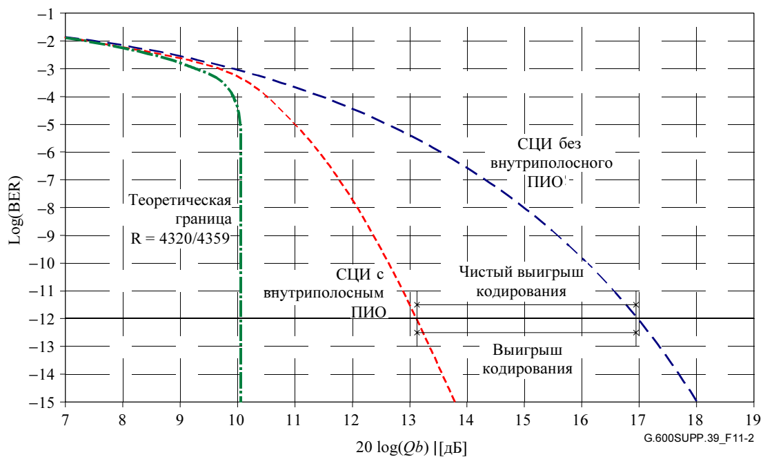
Рисунок 11-2 – Расчет рабочих характеристик схемы ПИО из G.707/Y.1322
