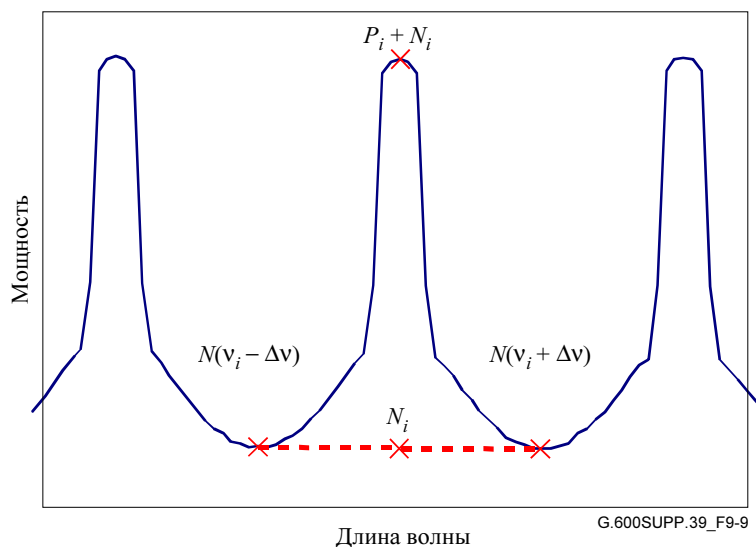
Рисунок 9-9 – Неправильное измерение OSNR из-за формирования шума
