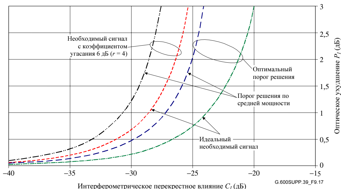
Рисунок 9-17 – График оптического ухудшения в зависимости от интерферометрического перекрестного влияния при многих мешающих сигналах (гауссова модель)
