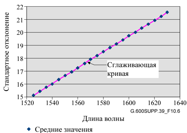
Рисунок 10-6 – Среднее значение коэффициента хроматической дисперсии для волокна G.652
