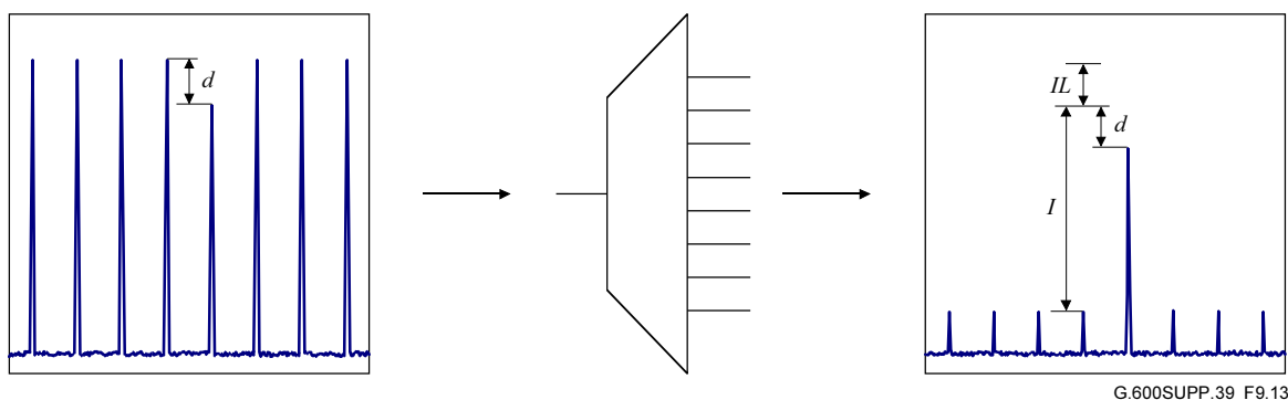
Рисунок 9-13 – Простой пример демультиплексора
