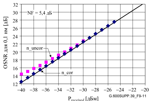
Рисунок 9-11 – OSNR в зависимости от измеренной принимаемой оптической мощности: с коррекцией шума ( n_{cor} ) и без коррекции шума ( n_{uncor} ) на канальной длине волны сигнала
