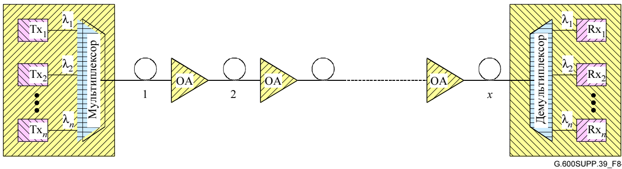
Рисунок 8-4 – Пример звена "точка-точка" с WDM
