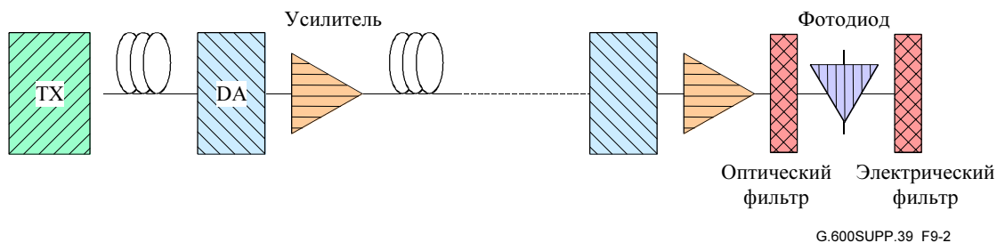
Рисунок 9-2 – Схема системы с повторяющейся посткомпенсацией
