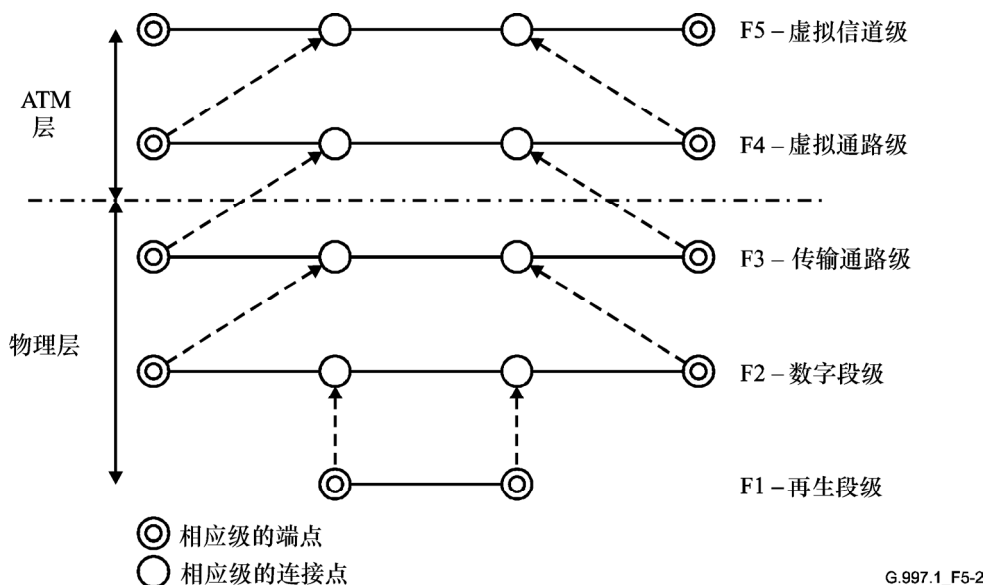
图 5-2/G.997.1—OAM 体系的分级及其与 ATM 层和物理层的关系
