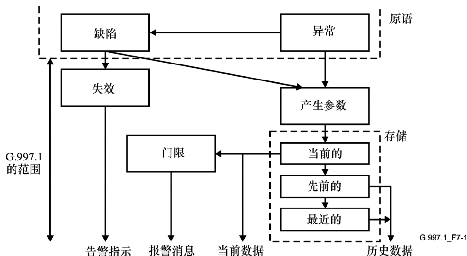
图 7-1/G.997.1—业务进行过程中的性能监控程序
