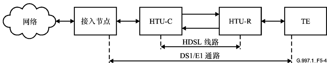
图 5-4/G.997.1—HDSL 线路和通路定义
