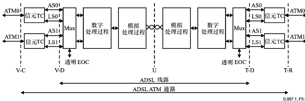
图 5-3/G.997.1—ADSL 线路和 ADSL ATM 通路定义
