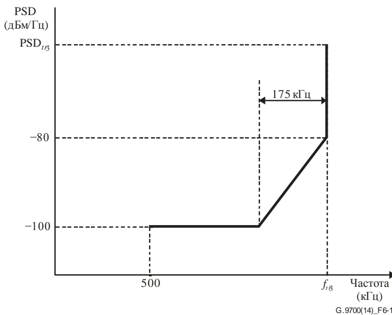
Рисунок 6-1 – Маска затухания на границе низких частот
