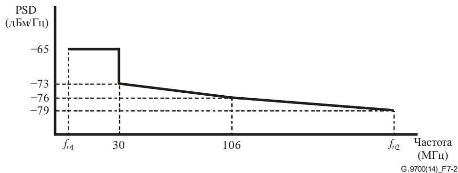
Рисунок 7-2 – Маска предельной PSD внутриполосных составляющих для профиля 212 МГц
