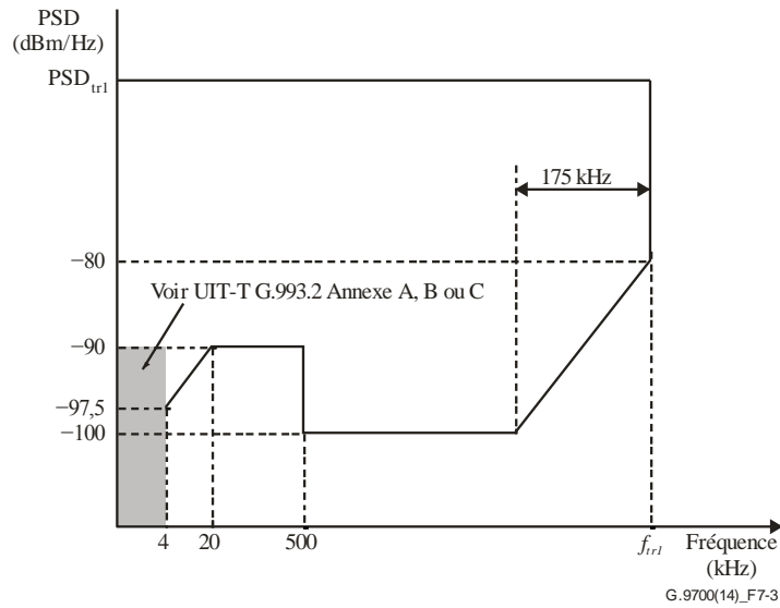
Figure 7-3 – Gabarit LPM hors bande côté basse fréquence
