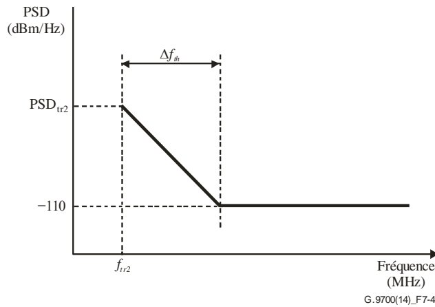
Figure 7-4 – Gabarit LPM hors bande côté haute fréquence
