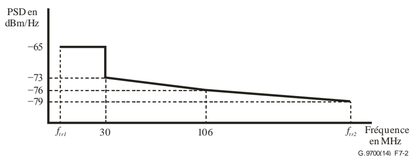
Figure 7-2 – Gabarit limite de densité PSD dans la bande pour le profil à 212 MHz
