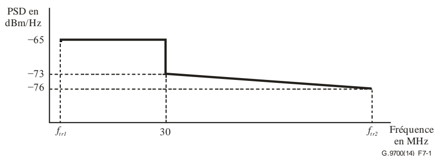
Figure 7-1 – Gabarit limite de densité PSD dans la bande pour le profil à 106 MHz
