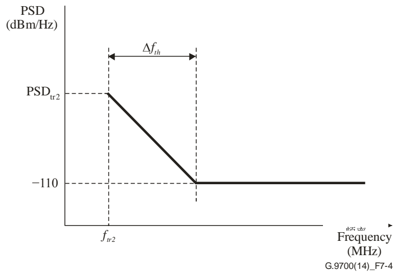
图 7-4 – 高频端的带外LPM
