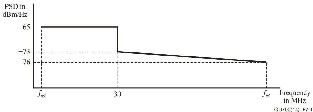
图 7-1 – 106 MHz剖面图的带内限制PSD掩膜
