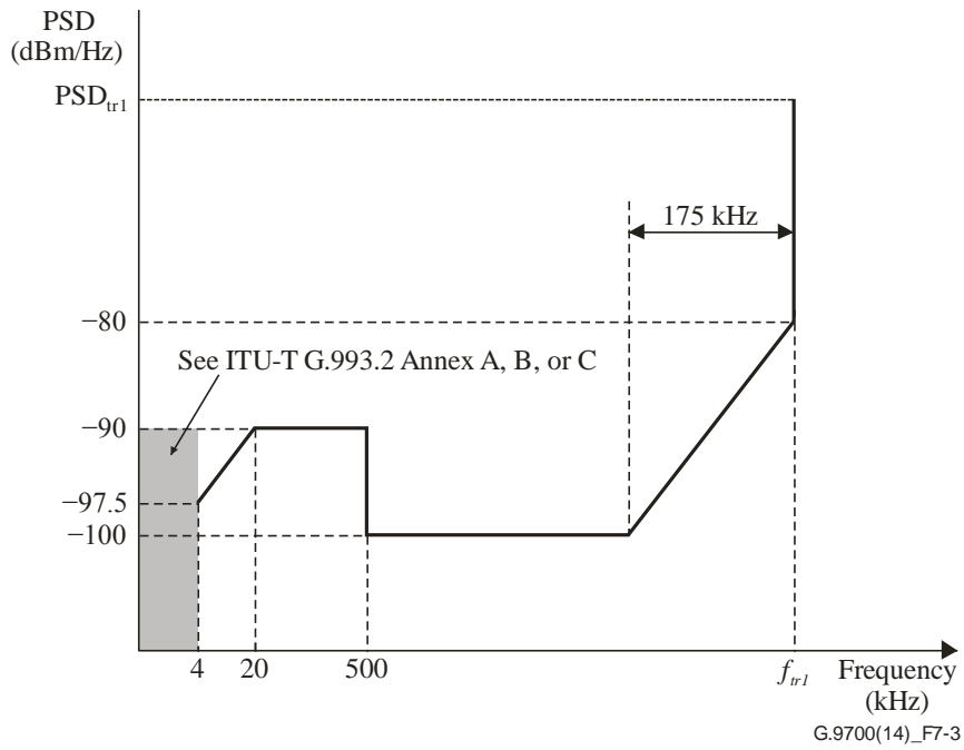
图 7-3 – 低频端的带外LPM
