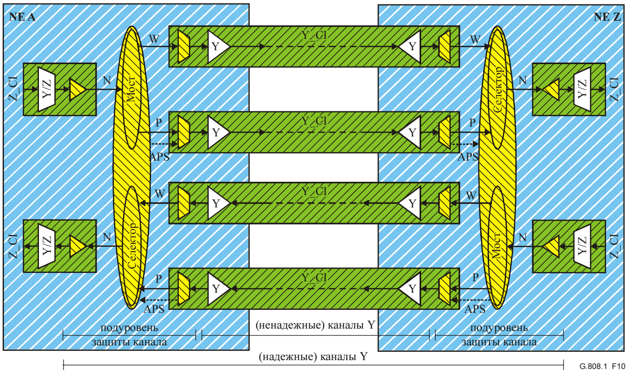
Рисунок 10/G.808.1 – Функциональная модель защиты канала 1+1/1:1
