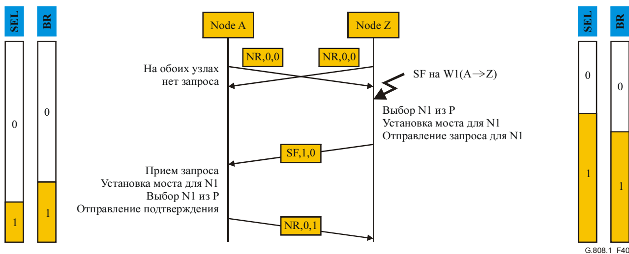
Рисунок 40/G.808.1 – Пример 1-этапного протокола
