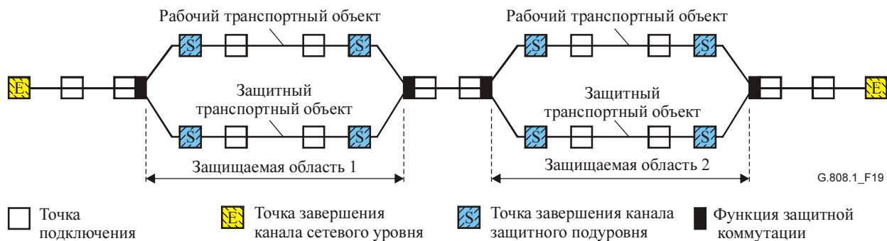
Рисунок 19/G.808.1 – Каскадная защита SNC/S
