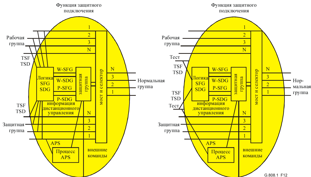
Рисунок 12/G.808.1 – Логика SFG/SDG в процессе групповой защиты
