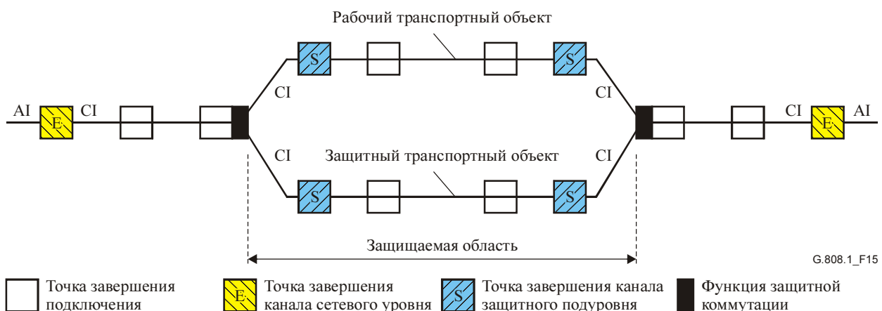
Рисунок 15/G.808.1 – Пример 1 защиты SNC/S
