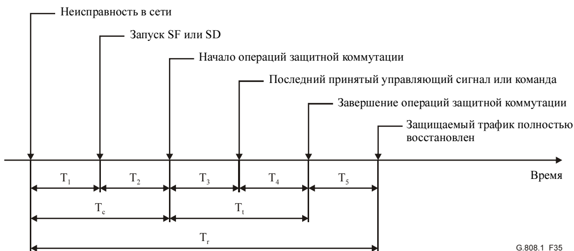
Рисунок 35/G.808.1 – Временная модель защитной коммутации
