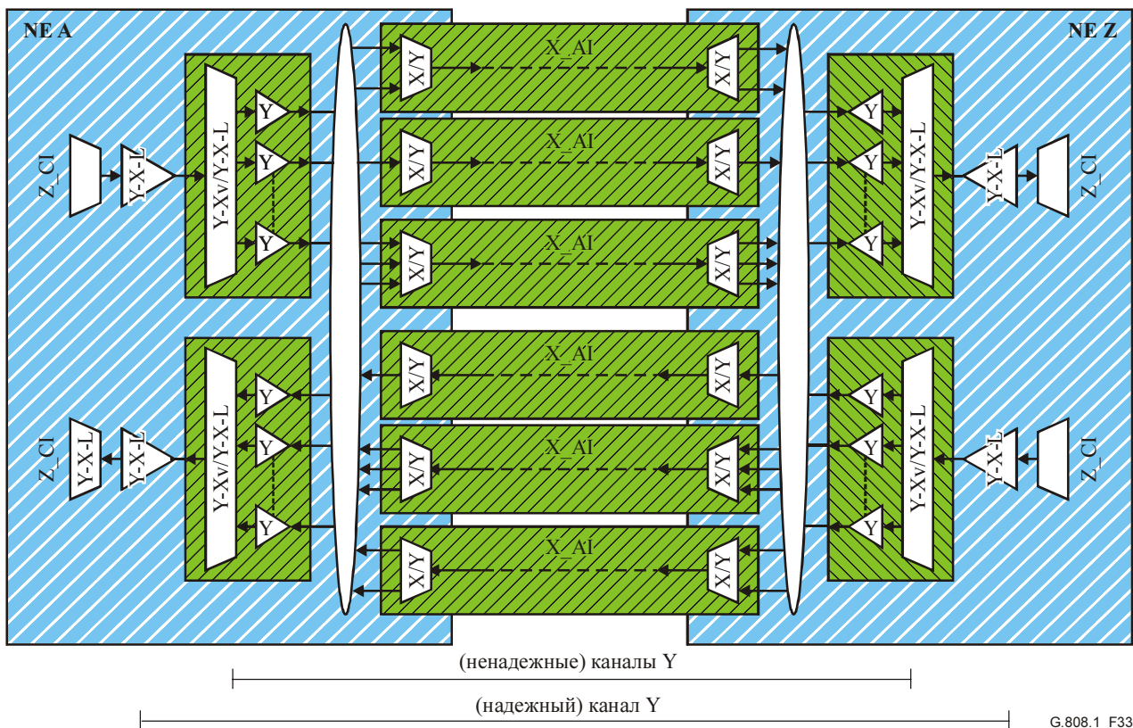
Рисунок 33/G.808.1 – Функциональная модель LCAS
