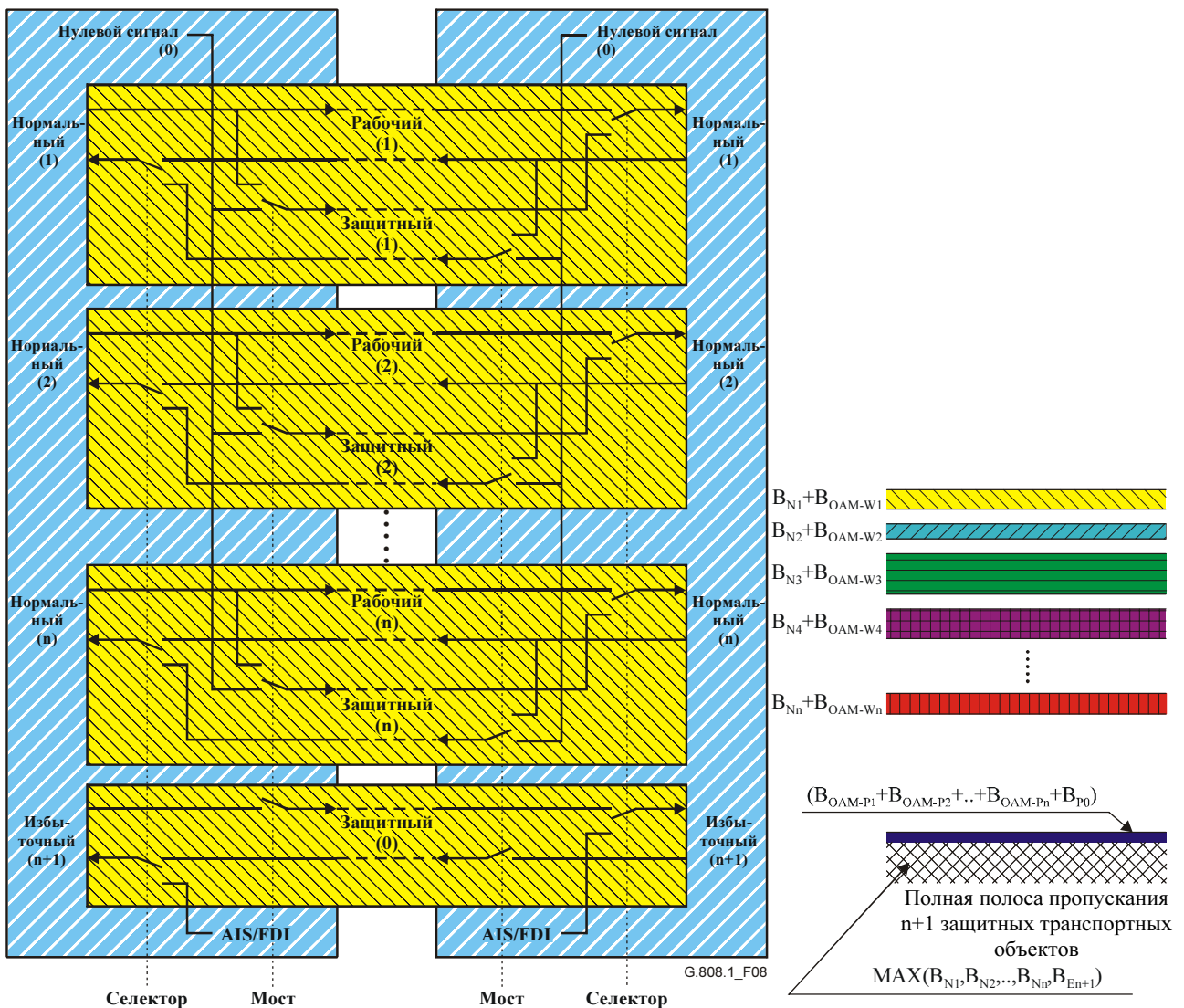
Рисунок 8/G.808.1 –Защитная архитектура (1:1) n при совместном использовании полосы пропускания
