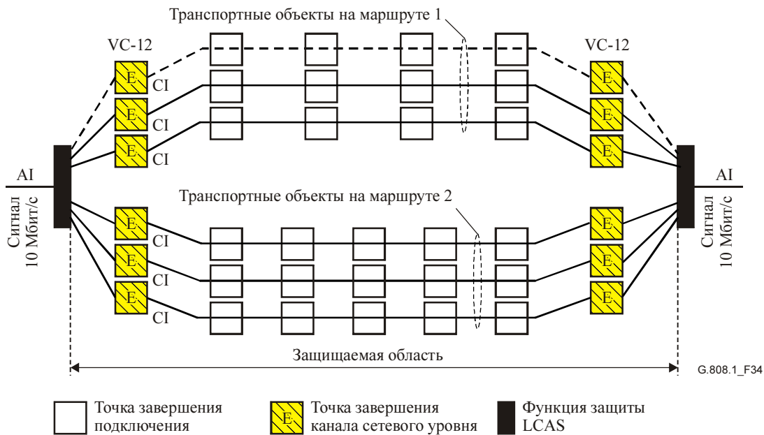
Рисунок 34/G.808.1 – Пример живучести LCAS для передачи сигнала 10 Мбит/с через VC-12-(X+Z)v (X=5, Z=0,1)
