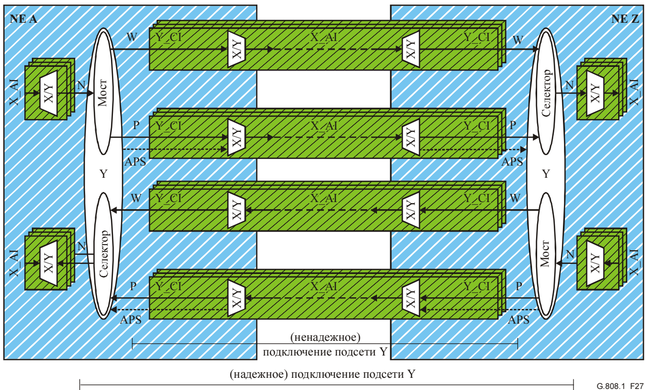
Рисунок 27/G.808.1 – Функциональная модель групповой защиты SNC/I 1+1
