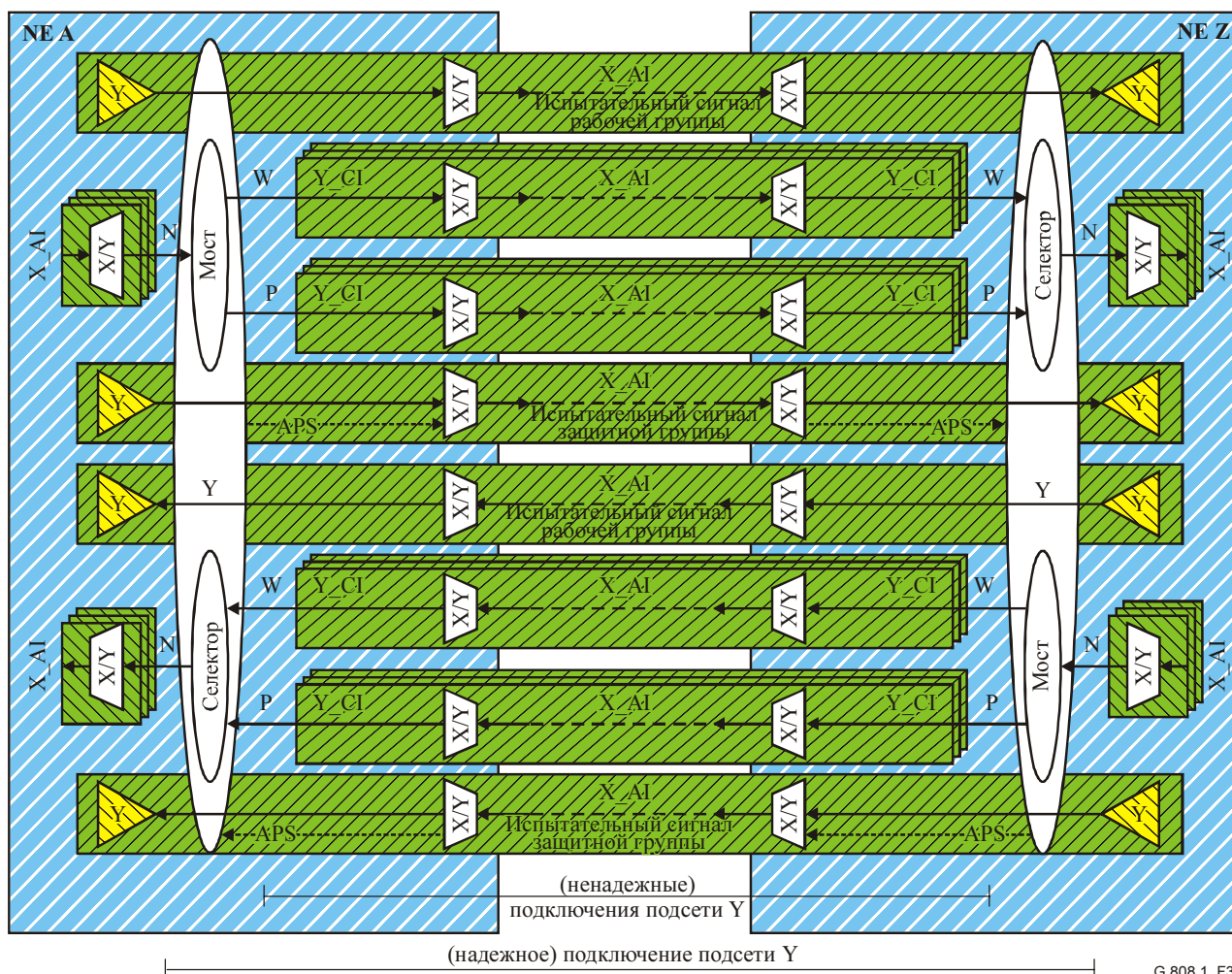
Рисунок 31/G.808.1 – Функциональная модель групповой защиты SNC/Te 1+1/1:1, использующая завершения канала сетевого уровня
