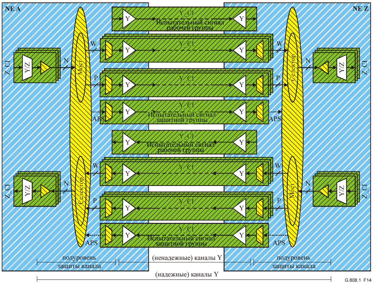
Рисунок 14/G.808.1 – Функциональная модель групповой защиты Т/канала 1+1/1:1
