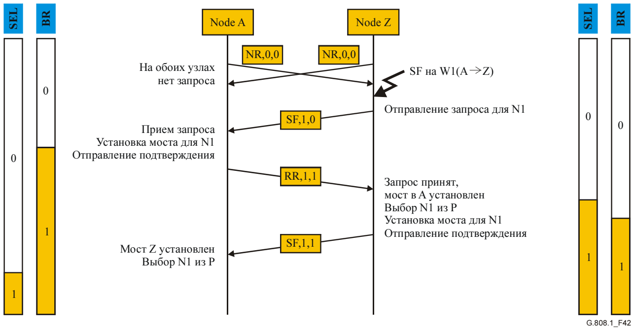
Рисунок 42/G.808.1 – Пример 3-этапного протокола
