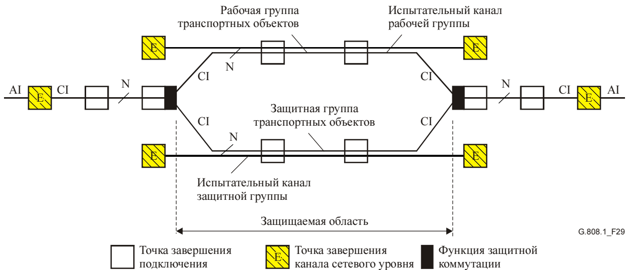
Рисунок 29/G.808.1 – Групповая защита SNC/Te 1:1 или 1+1, использующая завершения канала сетевого уровня
