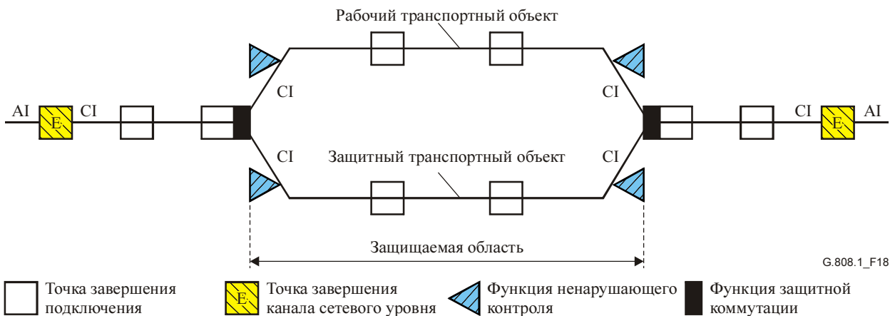
Рисунок 18/G.808.1 – Защита 1+1 SNC/N
