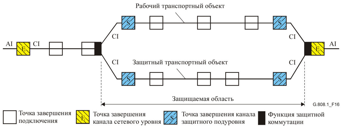
Рисунок 16/G.808.1 – Пример 2 защиты SNC/S
