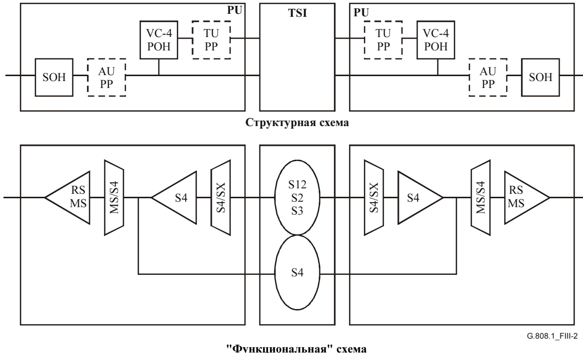
Рисунок III.2/G.808.1 – Отображение структурной схемы в функциональной: основная операция
