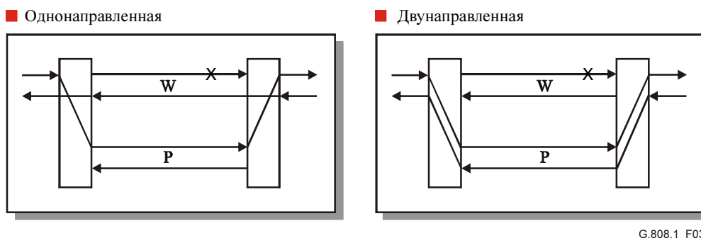
Рисунок 3/G.808.1 – Типы коммутации
