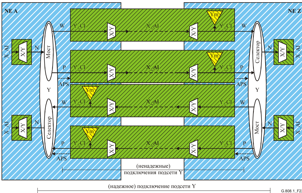
Рисунок 22/G.808.1 – Функциональная модель защиты SNC/Ne 1+1
