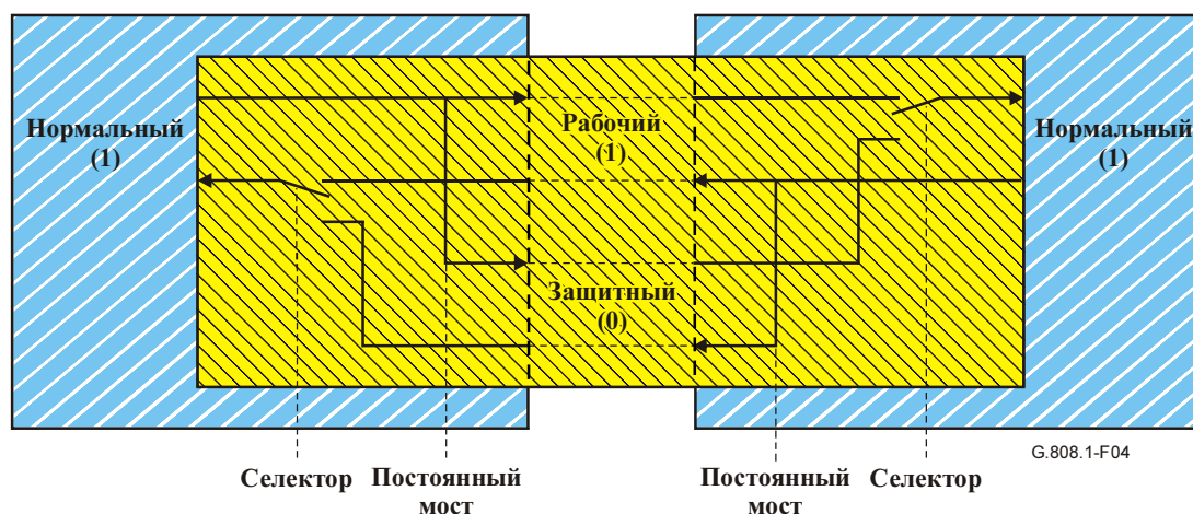
Рисунок 4/G.808.1 – Защитная архитектура 1+1
