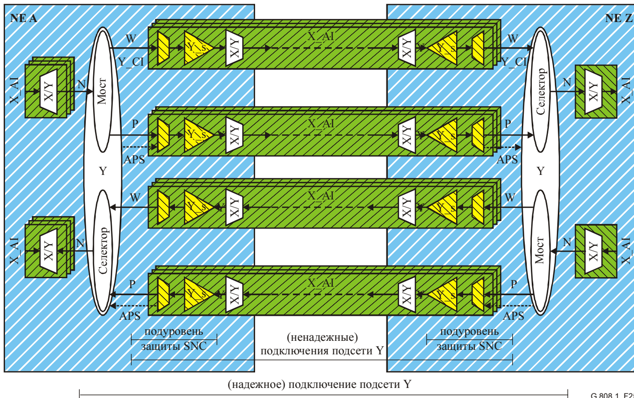
Рисунок 25/G.808.1 – Функциональная модель групповой защиты SNC/S 1+1/1:1
