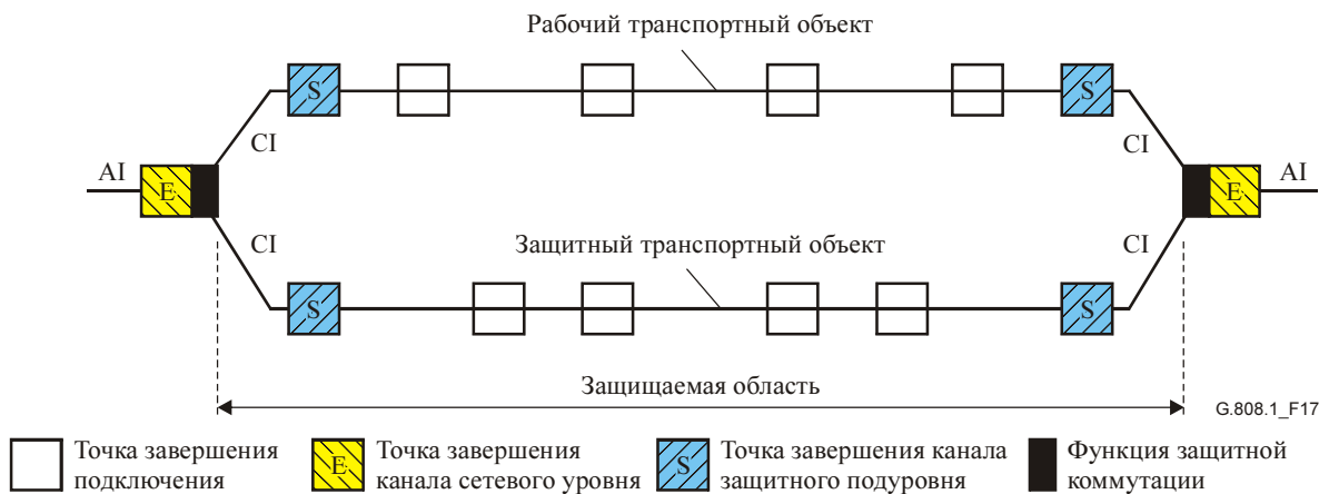
Рисунок 17/G.808.1 – Пример 3 защиты SNC/S
