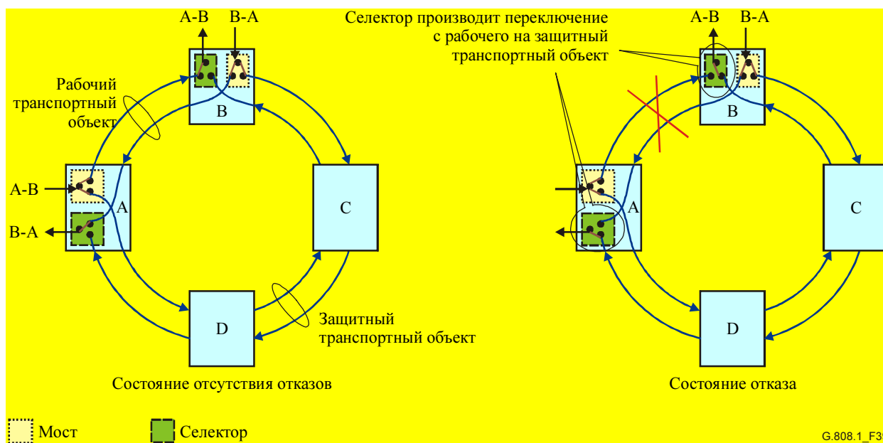
Рисунок 39/G.808.1 – Кольцо защиты подключения подсети (SNCP)
