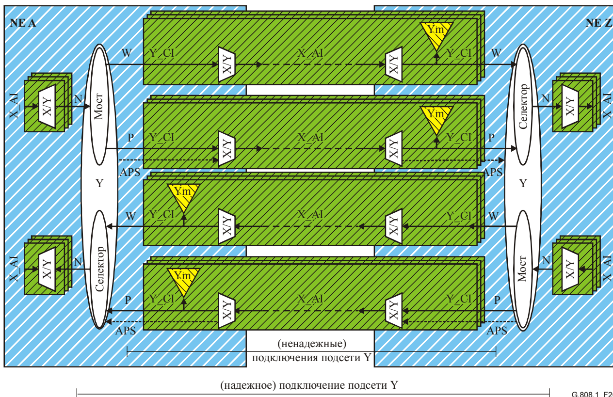
Рисунок 26/G.808.1 – Функциональная модель групповой защиты SNC/Ne 1+1
