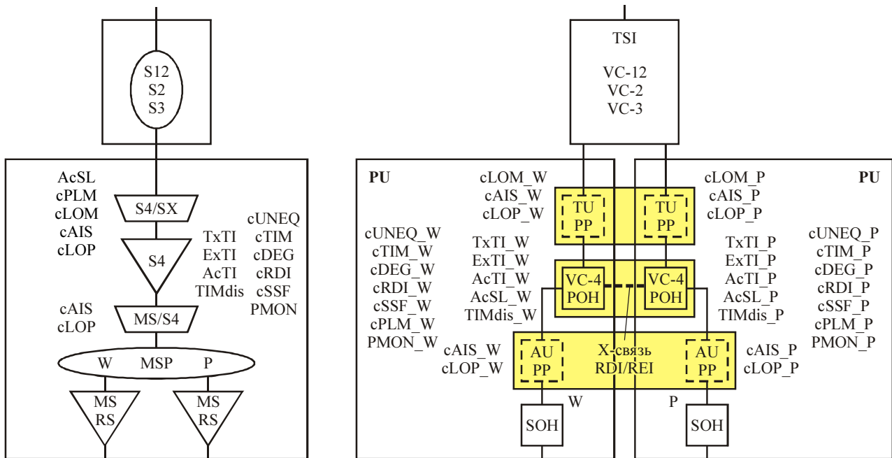
"Функциональная" схема
