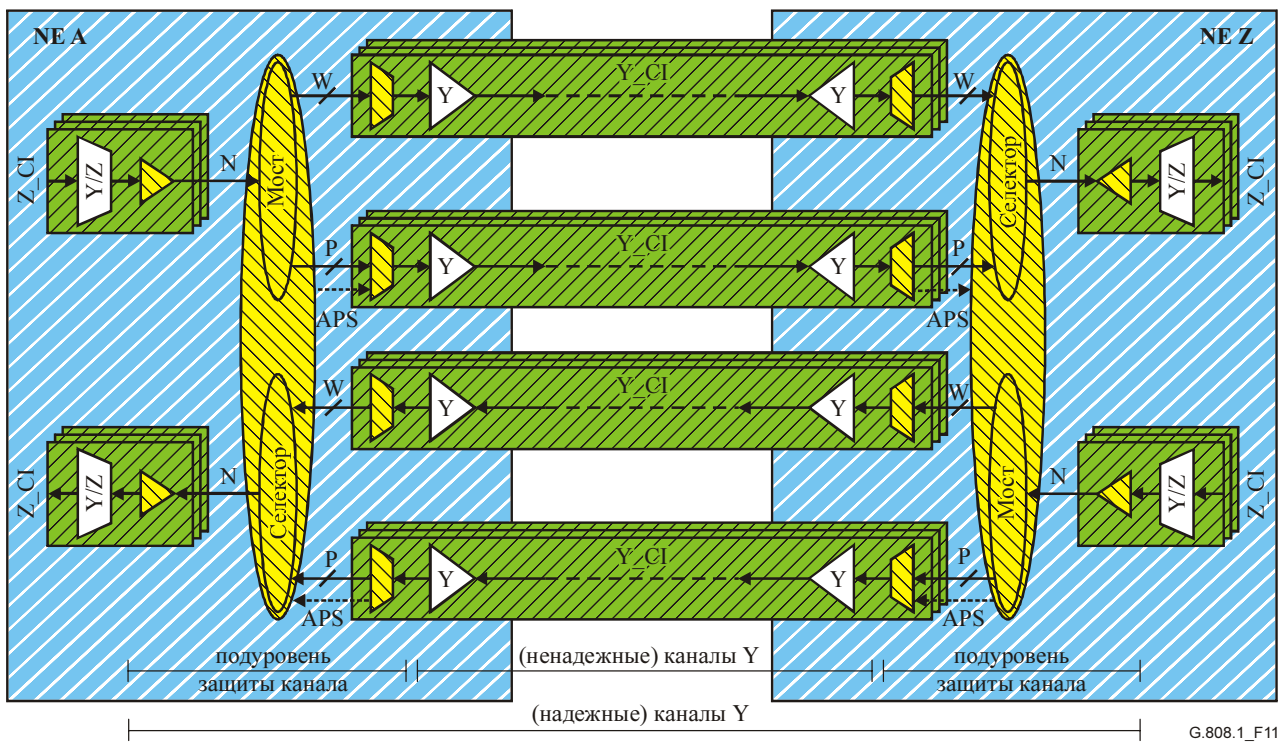
Рисунок 11/G.808.1 – Функциональная модель групповой защиты канала 1+1/1:1
