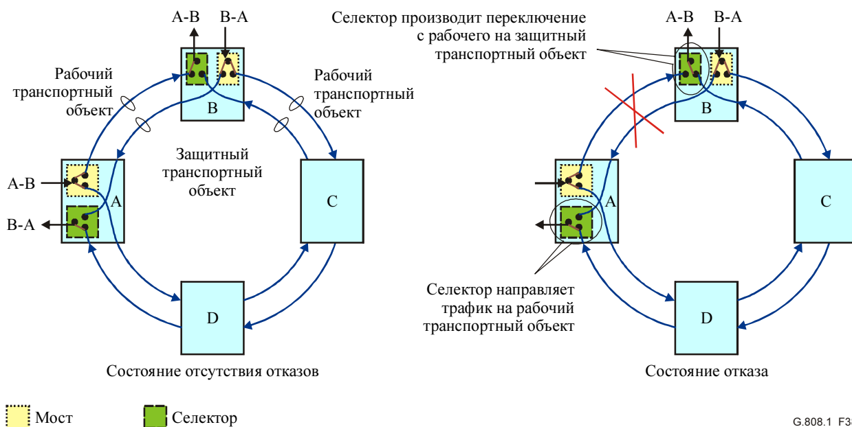
Рисунок 38/G.808.1 – Однонаправленное кольцо коммутации маршрута (UPSR)
