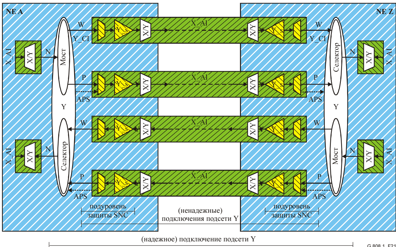
Рисунок 21/G.808.1 – Функциональная модель защиты SNC/S 1+1/1:1
