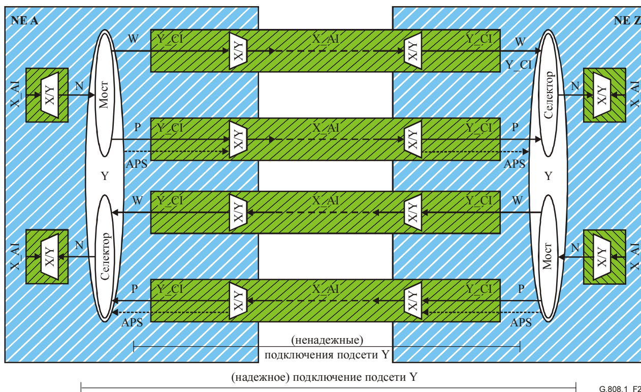
Рисунок 24/G.808.1 – Функциональная модель защиты SNC/I 1+1/1:1
