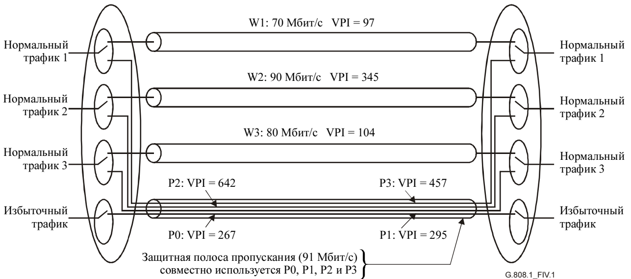
Рисунок IV.1/G.808.1 – Пример защиты (1:1) n
