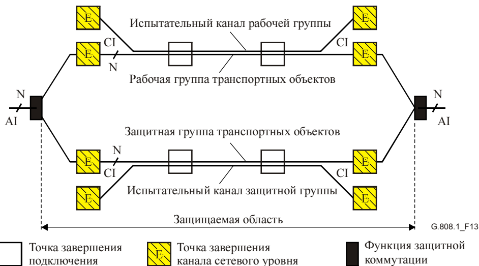
Рисунок 13/G.808.1 – Общая концепция групповой защиты канала/Т
