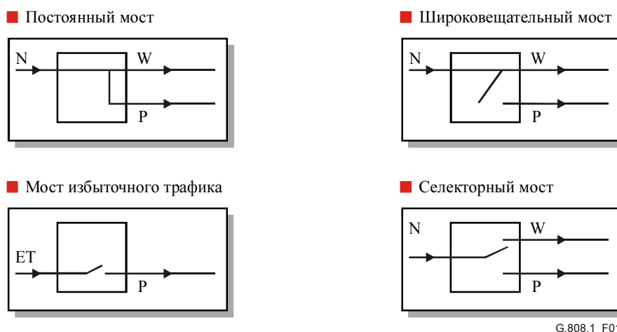
Рисунок 1/G.808.1 – Защитные мосты
