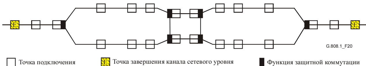
Рисунок 20/G.808.1 – Каскадная защита 1+1 SNC с соединениями подсетей, устойчивых к отказам
