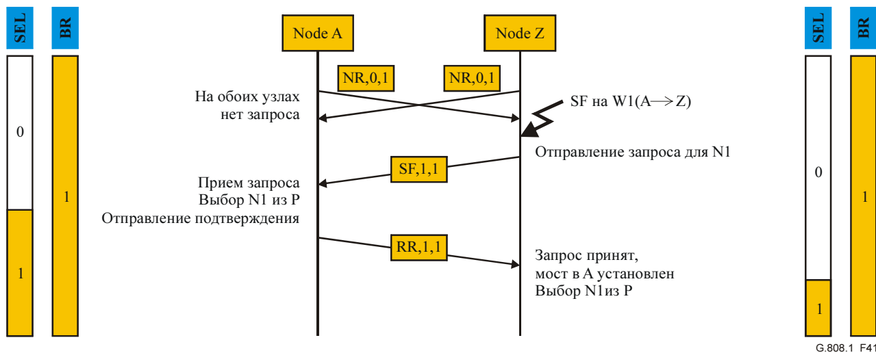
Рисунок 41/G.808.1 – Пример 2-этапного протокола
