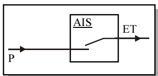
Рисунок 2/G.808.1 – Защитные селекторы
