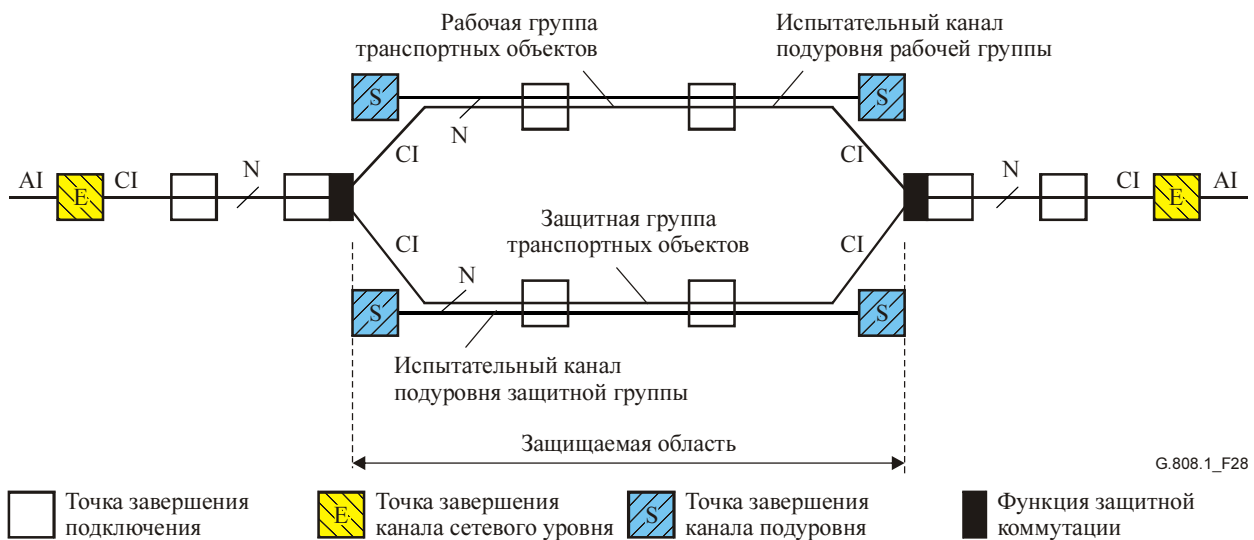
Рисунок 28/G.808.1 – Групповая защита SNC/Ts 1:1 или 1+1, использующая завершения канала подуровня
