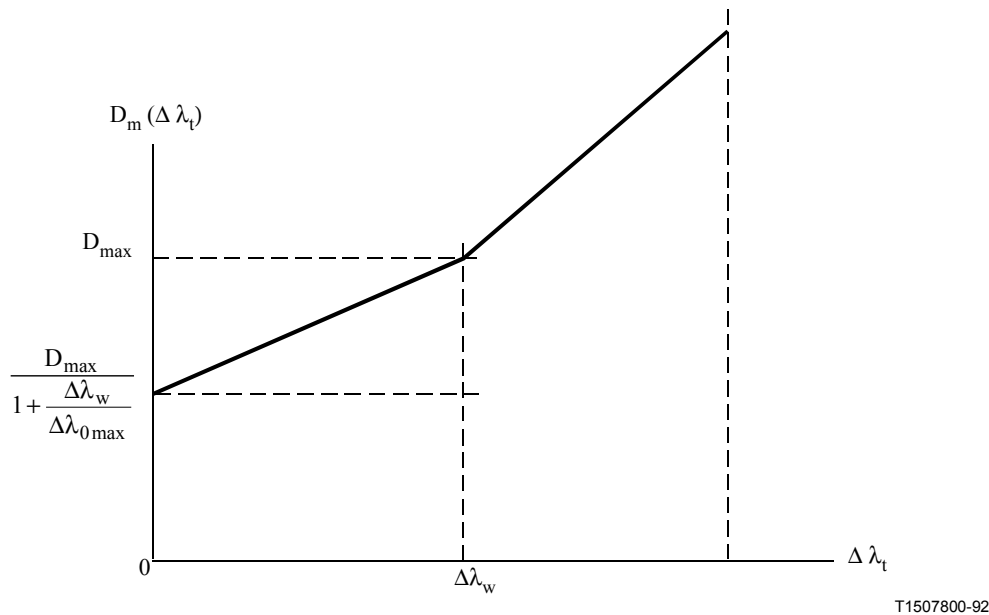
Figure 1/G.653 – Valeur absolue maximale du coefficient de dispersion
