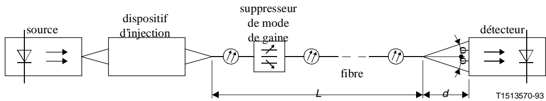
Figure 4/G.651 – Principe de mesure de la distribution de la lumière dans le champ lointain transmis
