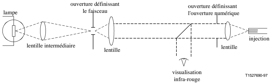
Figure 6/G.651 – Optique d'injection à ouverture limitée
