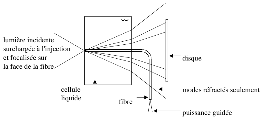
a) technique d'exploration du champ proche – Diagramme schématisique
