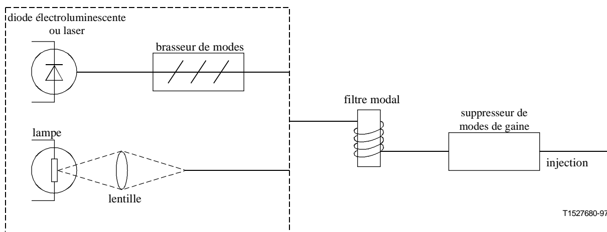
Figure 5/G.651 – Montage général pour l'injection
