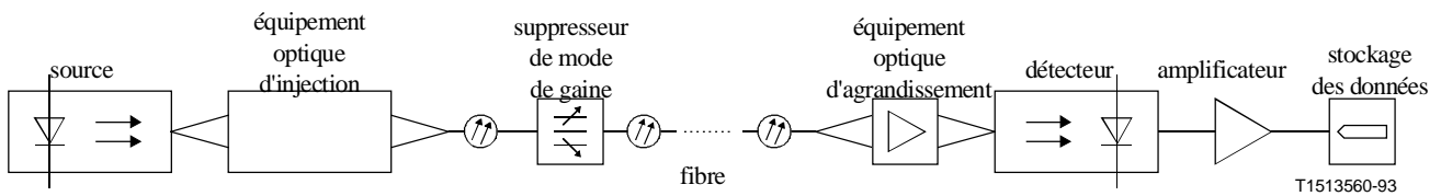
Figure 3/G.651 – Schéma type d'un banc de mesure par champ proche transmis
