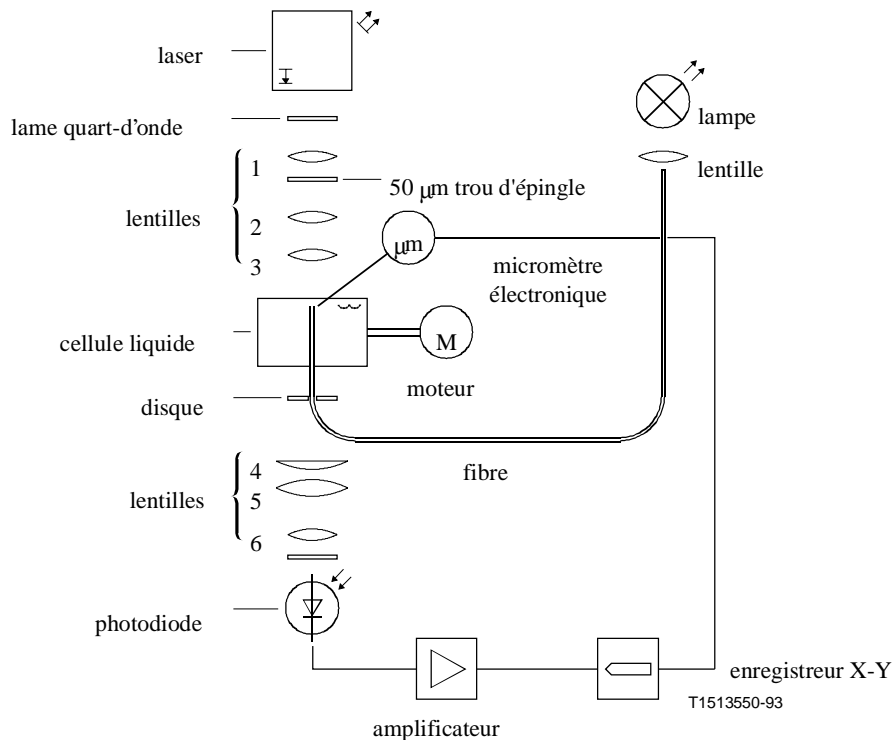
Figure 2/G.651 – Schéma type de l'équipement de mesure de l'exploration du champ proche réfracté
