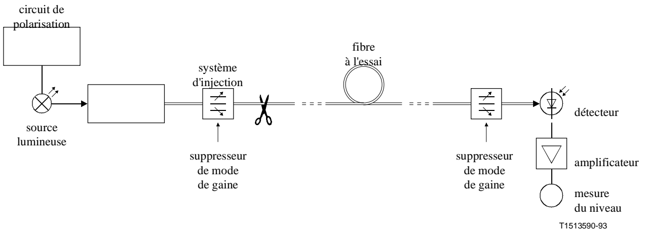
Figure 7/G.651 – Disposition du matériel d'essai pour mesurer l'affaiblissement ponctuel
