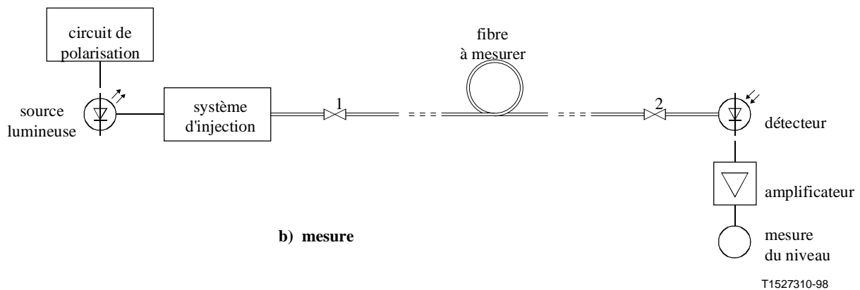
Figure 9/G.651 – Technique d'affaiblissement d'insertion
