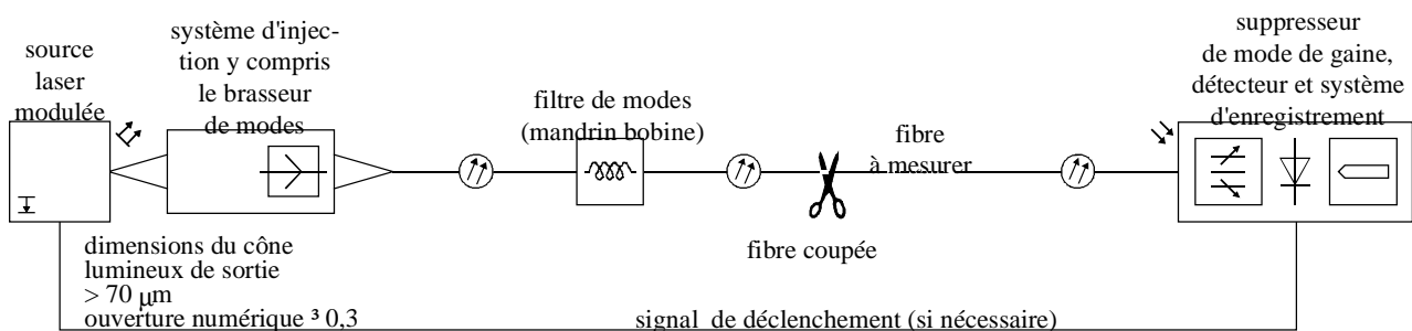
Figure 11/G.651 – Diagramme type de dispositif expérimental
