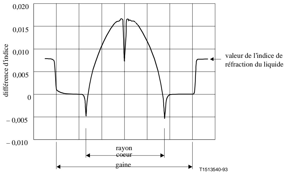
b) profil d'indice typique d'une fibre à gradient d'indice obtenu à l'aide de la technique d'exploration du champ réfracté proche
