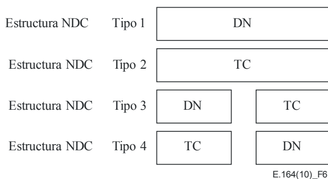
Figura 6 – Opciones para estructura de NDC
