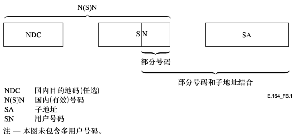
图 B.1—用ISDN号码寻址
