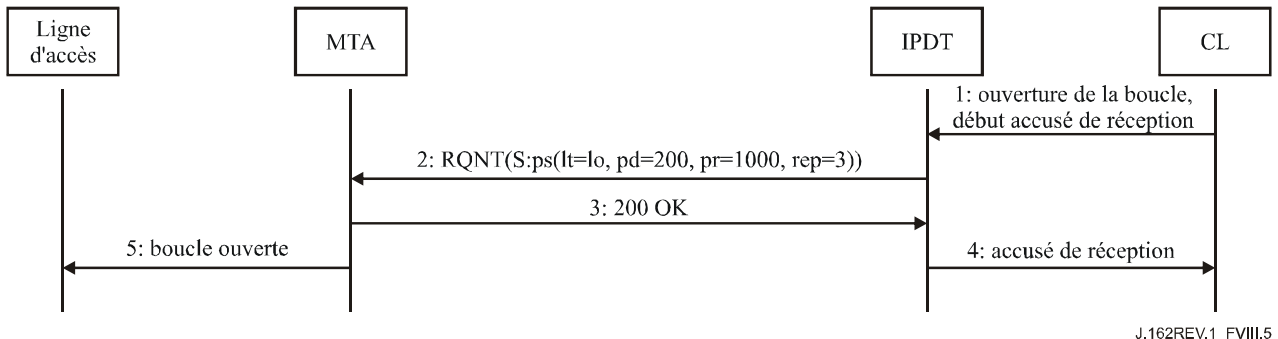
Figure VIII.5/J.162 – Signal à impulsions avec accusé de réception de départ
