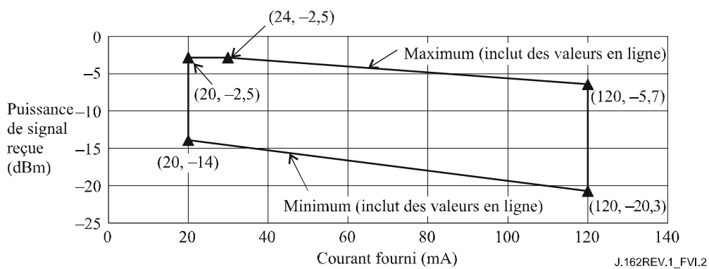
Figure VI.1/J.162 – Gamme de tolérance pour la puissance de réception du signal (basse fréquence de groupe)
