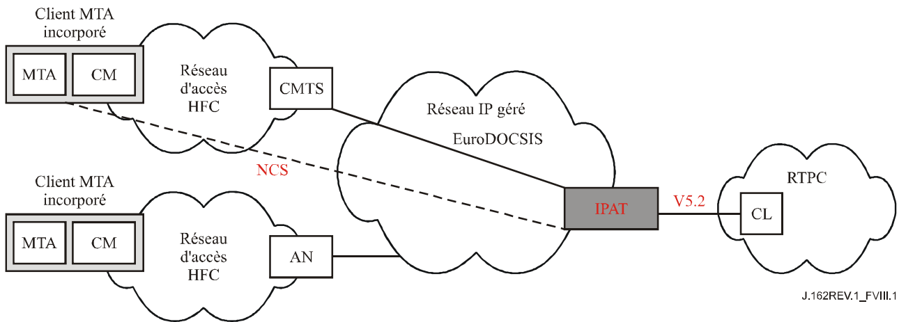
Figure VIII.1/J.162 – Modèle de référence pour le présent appendice
