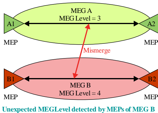
a) Bidirectional mismerge
