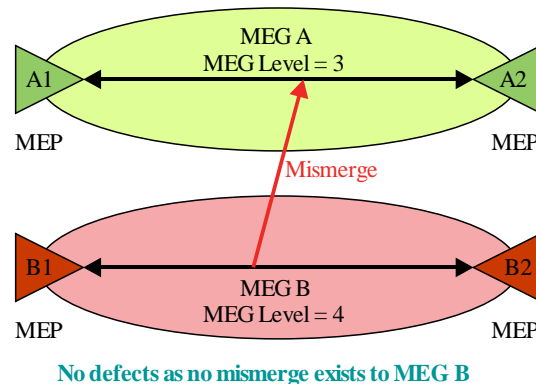
b) Unidirectional mismerge
