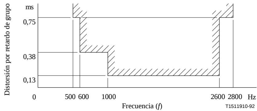
Figura 8/G.712 – Distorsión por retardo de grupo en función de la frecuencia para canales de analógico a cuatro hilos a digital (E4 ent a T sal o T ent a E4 sal )
