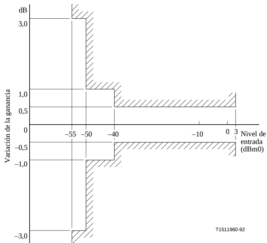
Figura 13/G.712 – Variación de la ganancia en función del nivel de entrada para canales de analógico a cuatro hilos a analógico a cuatro hilos y de analógico a dos hilos a analógico a dos hilos ( E4_{1ent} a E4_{2sal} y E2_{1ent} a E2_{2sal} )
