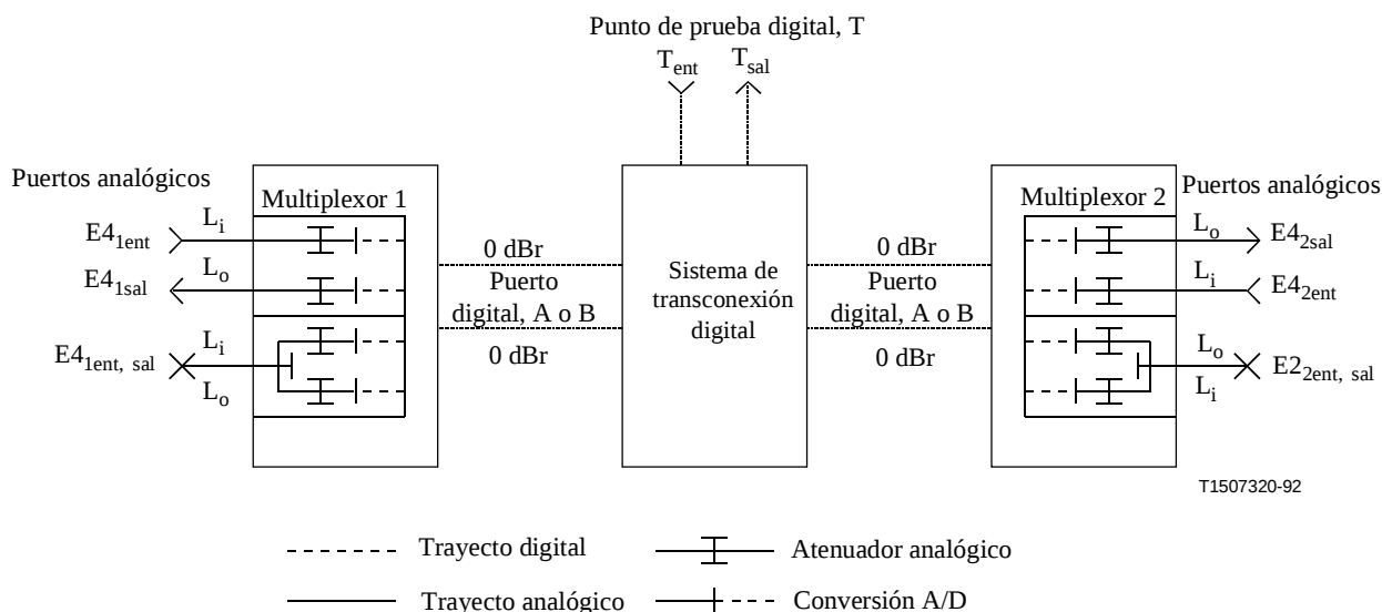
Figura 1/G.712 – Equipos y puertos de prueba a MIC
