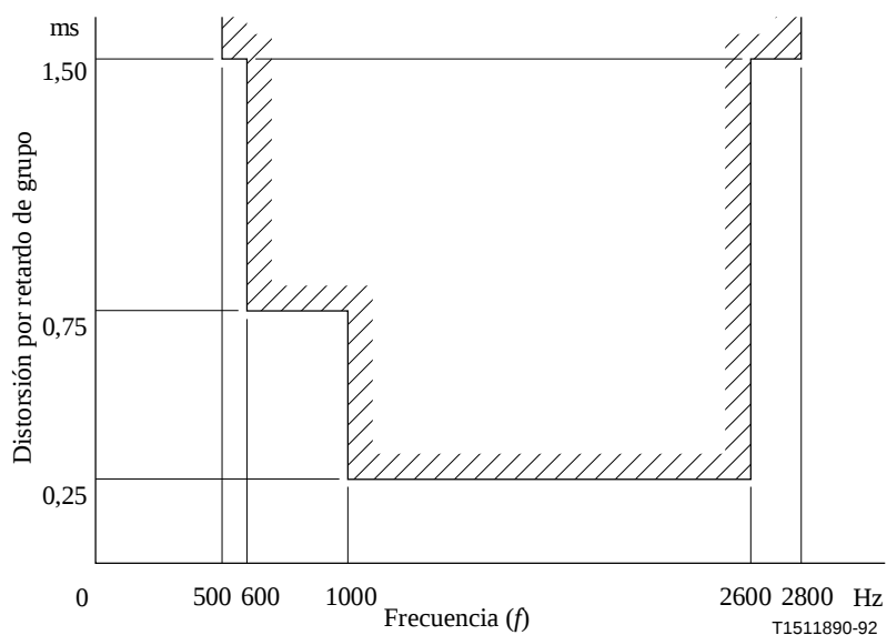
Figura 6/G.712 – Distorsión por retardo de grupo en función de la frecuencia para canales de analógico a analógico entre puertos a cuatro hilos ( E4_{1ent} a E4_{2sal} )
