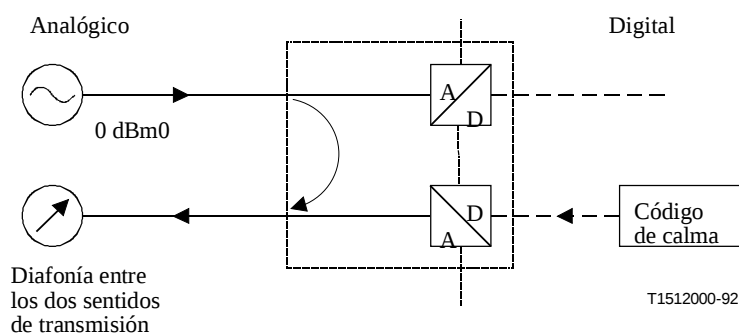
Figura 18/G.712 – Mediciones de diafonía en un puerto a cuatro hilos (E4) con una señal de prueba analógica entre un canal y el canal de retorno
