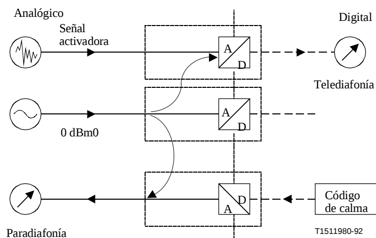
Figura 16/G.712 – Mediciones FEXT y NEXT con una señal de prueba analógica entre canales a cuatro hilos (E4)
