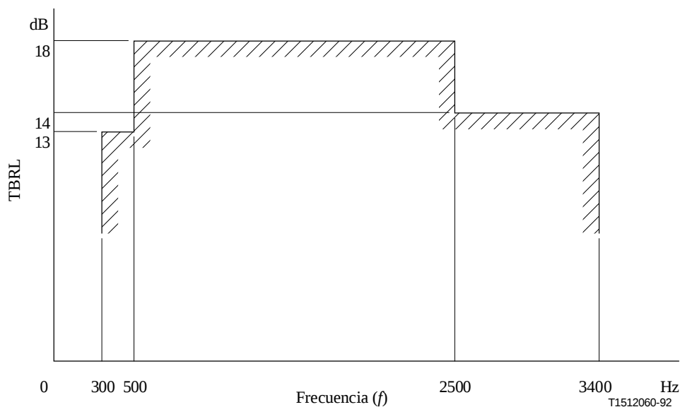
Figura 24/G.712 – Valores mínimos de la atenuación de equilibrado del terminal (provisional)
