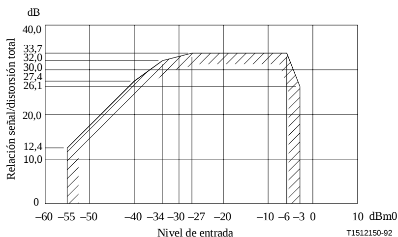
Figura I.9/G.712 – Relación señal/distorsión total en función del nivel de entrada de los canales de analógico a dos hilos a digital, lado codificación ( E_{2ent} a T_{sal} )
