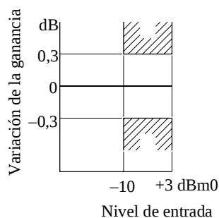
Figura I.4/G.712 – Variación de la ganancia en función del nivel de entrada de los canales de analógico a digital ( E4_{ent} a T_{sal} , T_{ent} a E4_{sal} , E2_{ent} a T_{sal} o T_{ent} a E2_{sal} )
