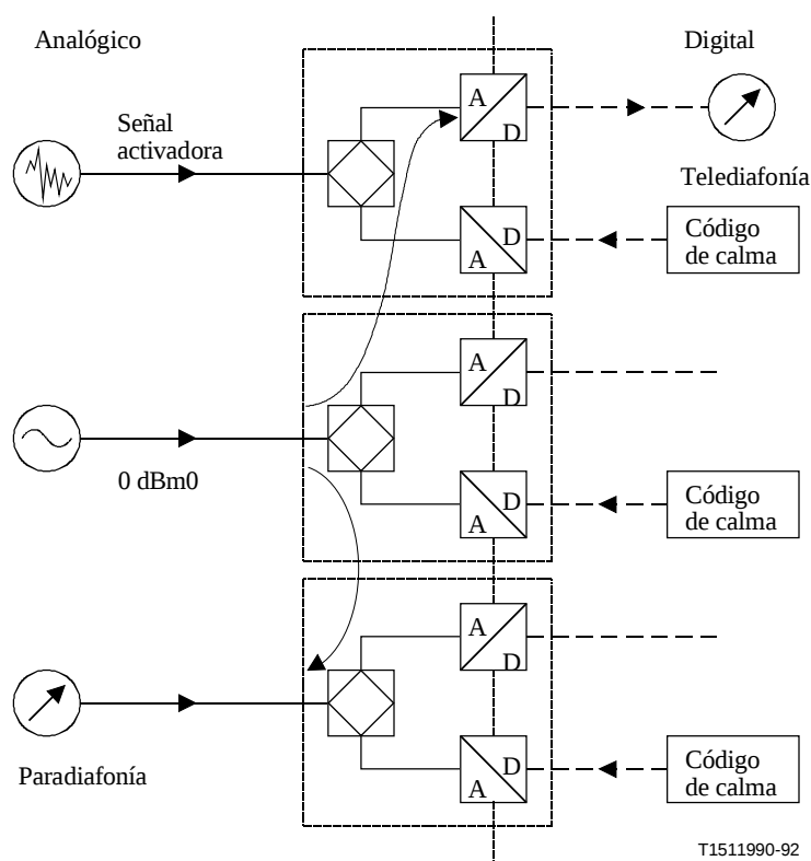
Figura 17/G.712 – Mediciones FEXT y NEXT con una señal de prueba analógica entre canales a dos hilos (E2)
