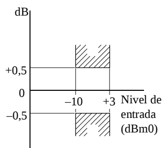
Figura I.3/G.712 – Variación de la ganancia en función del nivel de entrada de los canales de analógico a analógico entre puertos a cuatro hilos ( E4_{1ent} a E4_{2sal} ) a dos hilos ( E2_{1ent} a E2_{2sal} )
