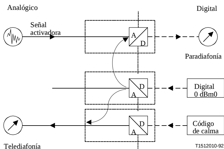
Figura 19/G.712 – Mediciones en puertos a cuatro hilos (E4) con una señal de prueba digital entre canales diferentes
