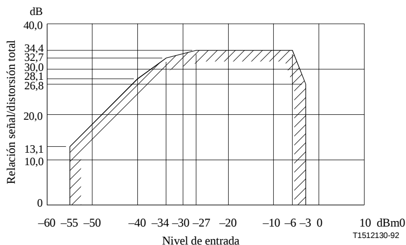
Figura I.7/G.712 – Relación señal/distorsión total en función del nivel de entrada de los canales de analógico a cuatro hilos a digital, lado codificación ( E_{4ent} a T_{sal} )
