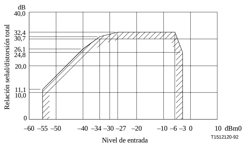
Figura I.6/G.712 – Relación señal/distorsión total en función del nivel de entrada de los canales a dos hilos de analógico a analógico ( E_{2_{1ent}} a E_{2_{2sal}} )
