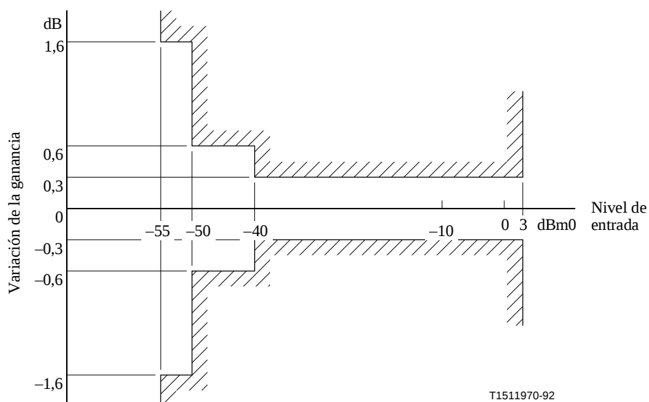
Figura 14/G.712 – Variación de la ganancia en función del nivel de entrada para canales de analógico a digital ( E4_{ent} a T_{sal} , T_{ent} a E4_{sal} , E2_{ent} a T_{sal} y T_{ent} a E2_{sal} )
