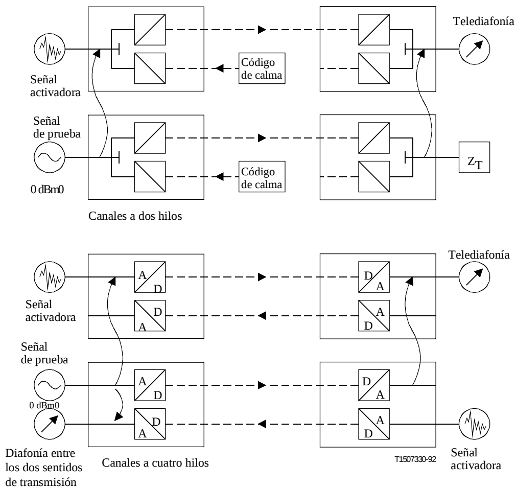
Figura 15/G.712 – Medición de la diafonía entre dos canales
