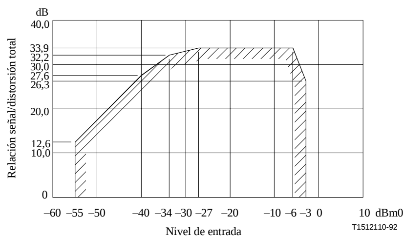
Figura I.5/G.712 – Relación señal/distorsión total en función del nivel de entrada de los canales a cuatro hilos de analógico a analógico ( E_{4_{1ent}} a E_{4_{2sal}} )
