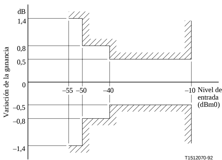
Figura I.1/G.712 – Variación de la ganancia en función del nivel de entrada de los canales de analógico a analógico entre puertos a cuatro hilos ( E4_{1ent} a E4_{2sal} ) o dos hilos ( E2_{1ent} a E2_{2sal} )
