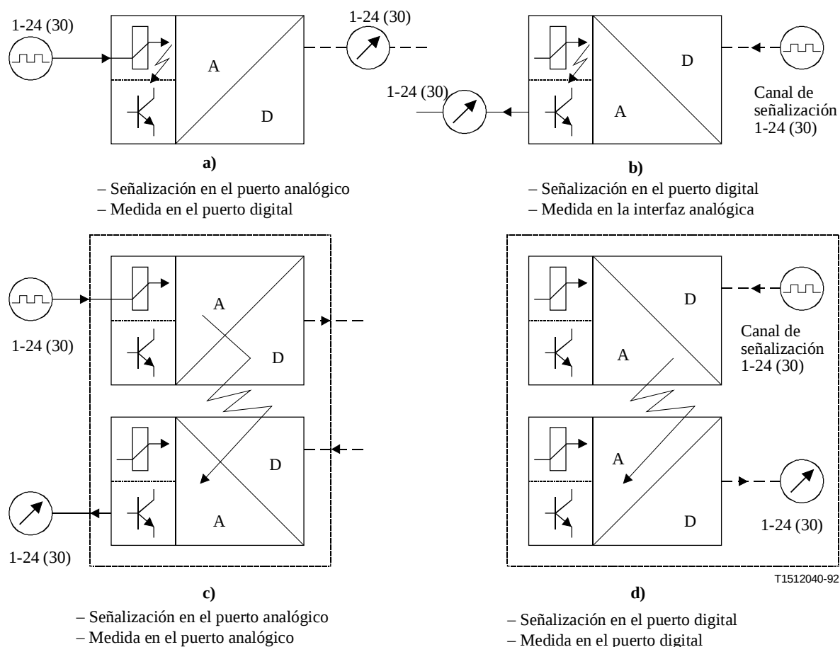
Figura 22/G.712 – Medición de las contribuciones de interferencia de la señalización
