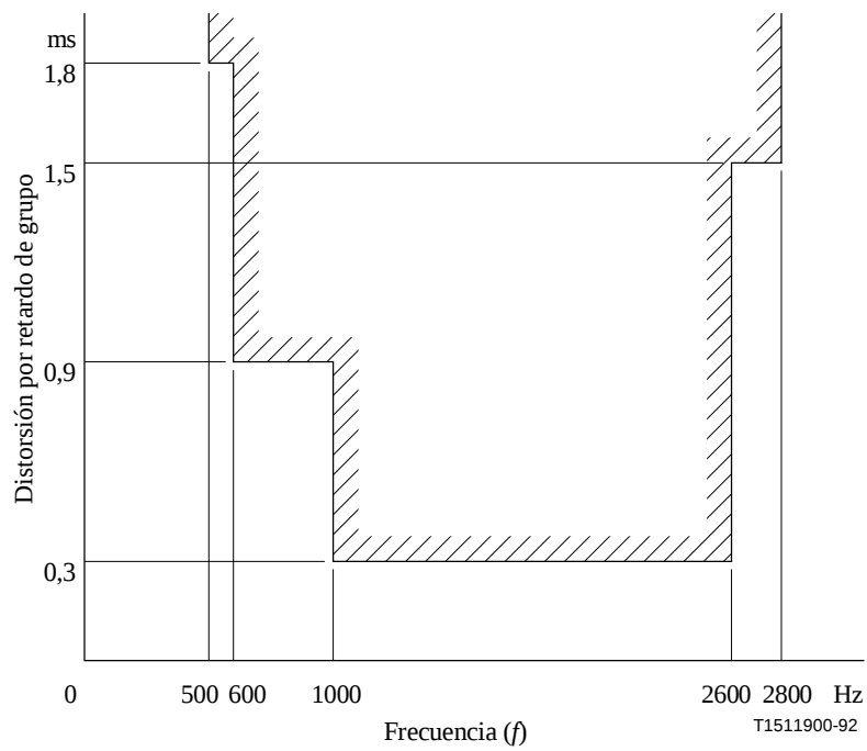
Figura 7/G.712 – Distorsión por retardo de grupo en función de la frecuencia para canales de analógico a analógico entre puertos a dos hilos (E2 1ent a E2 2sal )
