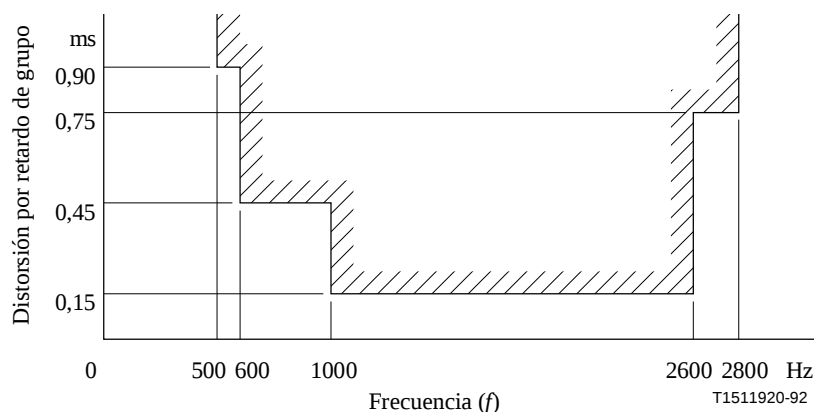
Figura 9/G.712 – Distorsión por retardo de grupo en función de la frecuencia para canales de analógico a dos hilos a digital (E2 ent a T sal o T ent a E2 sal )
