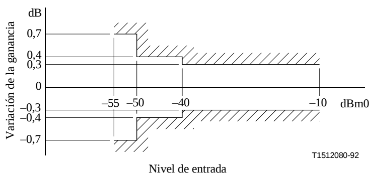
Figura I.2/G.712 – Variación de la ganancia en función del nivel de entrada de los canales de analógico a digital ( E4_{ent} a T_{sal} , T_{ent} a E4_{sal} , E2_{ent} a T_{sal} o T_{ent} a E2_{sal} )
