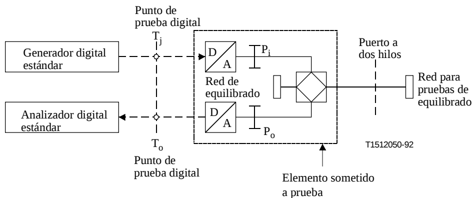
Figura 23/G.712 – Configuración para la medición de la pérdida del semibucle
