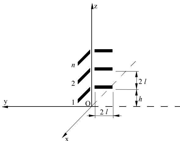
Quadrant antenna
