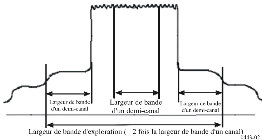
FIGURE 2 Rapport de puissance dans le canal adjacent en utilisant la largeur de bande d'un demi-canal
